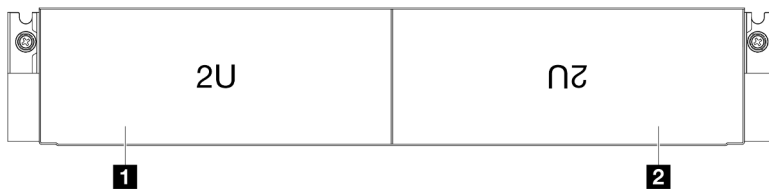
Figura 7. Vista anteriore dello chassis con due nodi 2U
