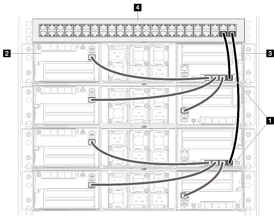
Figura 11. Configurazioni a più nodi o chassis con nodi 2U
