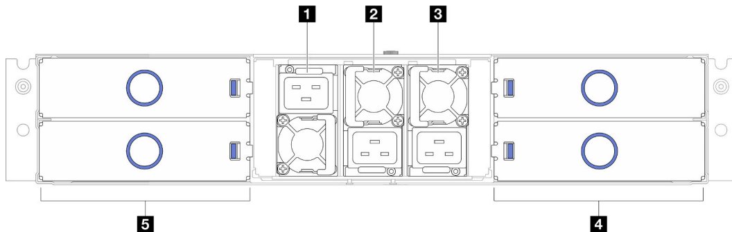
Figura 8. Vista posteriore chassis
