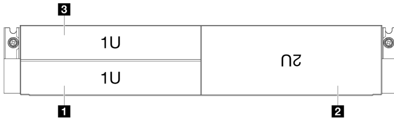
Figura 6. Vista anteriore dello chassis con due nodi 1U (vassoi sinistri) e un nodo 2U (vassoio destro, capovolto)
