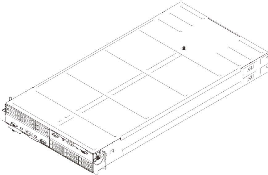
Figura 3. Chassis ThinkSystem D3 installato con due nodi SD550 V3
