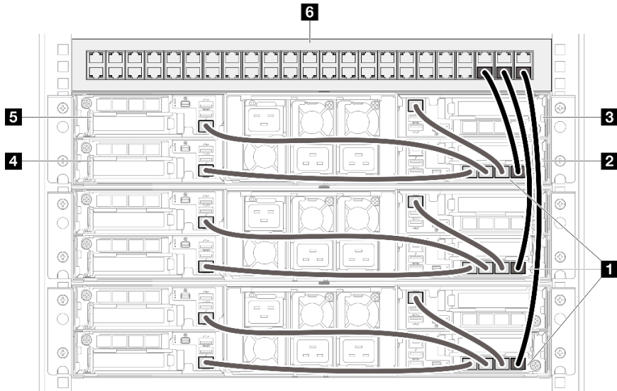
Figura 12. Configurazioni a più nodi o chassis con nodi 1U
