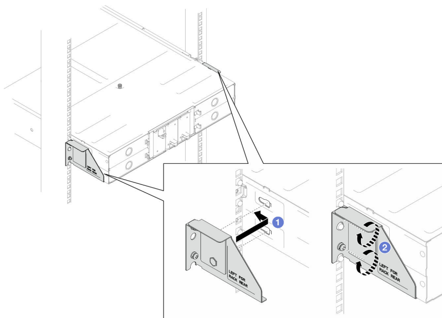
Figura 19. Installazione delle staffe di spedizione
