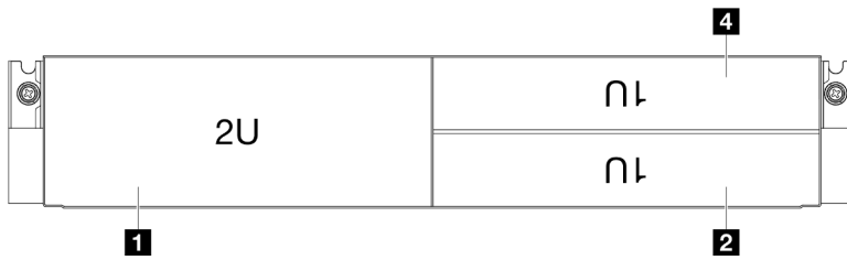
Figura 5. Vista anteriore dello chassis con un nodo 2U (vassoio sinistro) e due nodi 1U (vassoi destri, capovolti)
