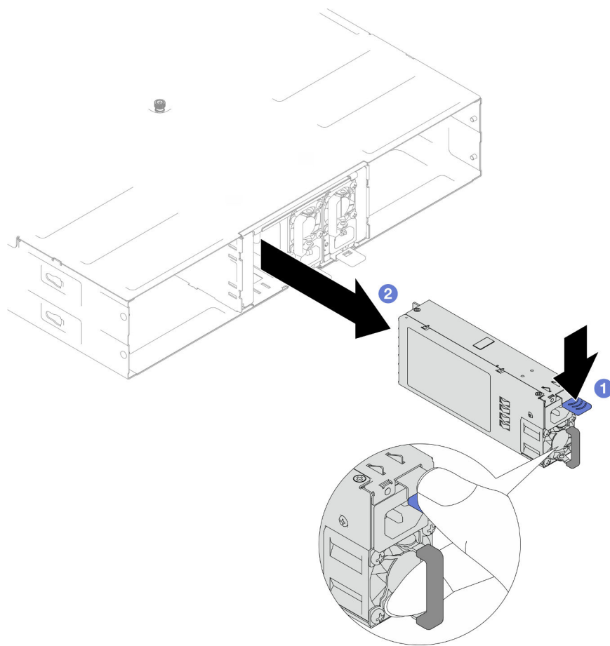
Figura 22. Rimozione di una PSU hot-swap
