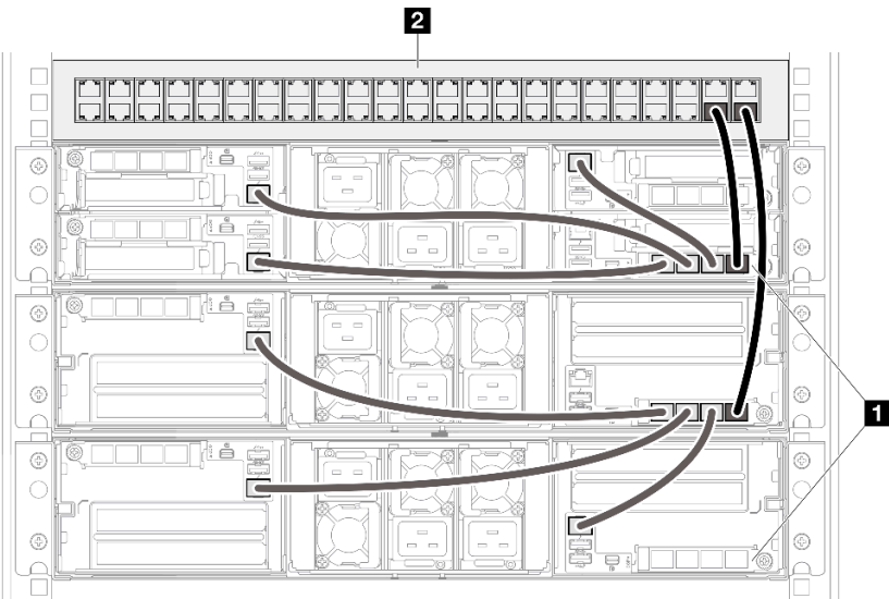
Figura 13. Configurazioni a più nodi o chassis con nodi 1U e 2U
