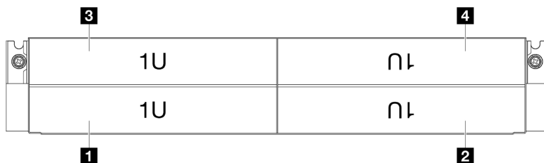
Figura 4. Vista anteriore dello chassis con quattro nodi 1U
