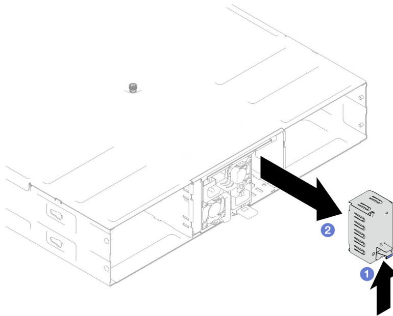
Abbildung 18. Entfernen einer PSU-Abdeckblende
