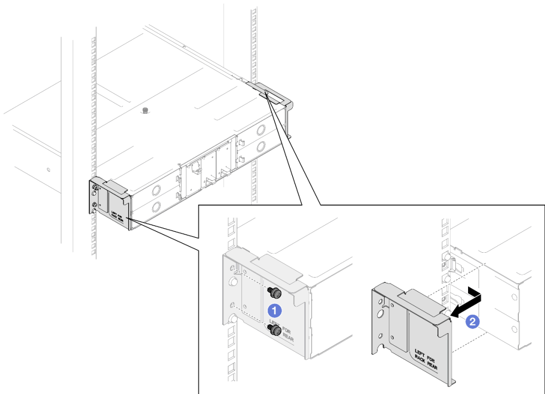
Abbildung 8. Entfernen von Transporthalterungen für 29 Zoll oder 28,31 Zoll tiefe Racks
