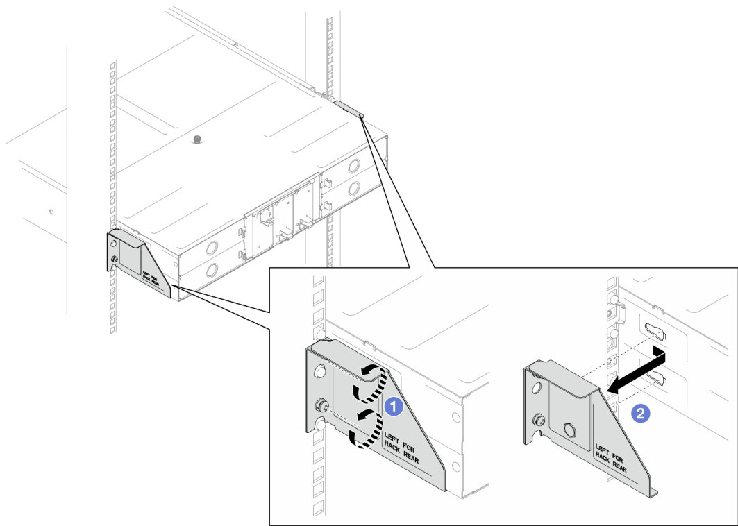
Abbildung 8. Entfernen von Transporthalterungen für 29 Zoll oder 28,31 Zoll tiefe Racks
