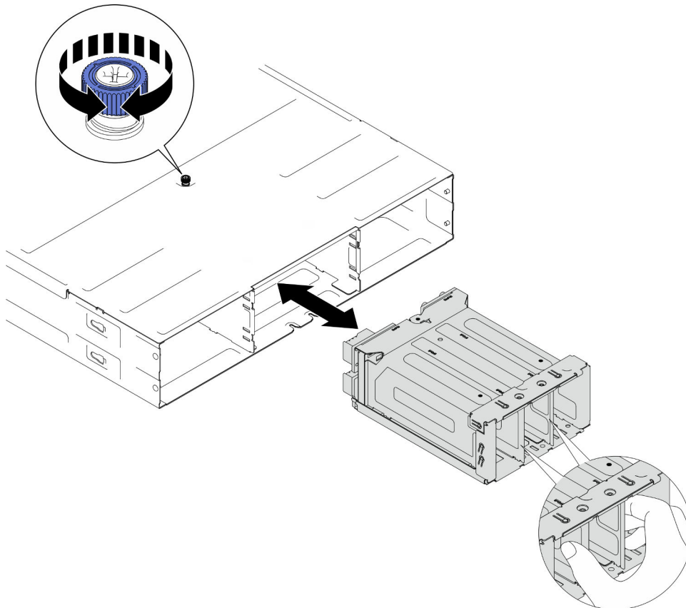
Abbildung 21. Entfernen des PSU-Rahmens
