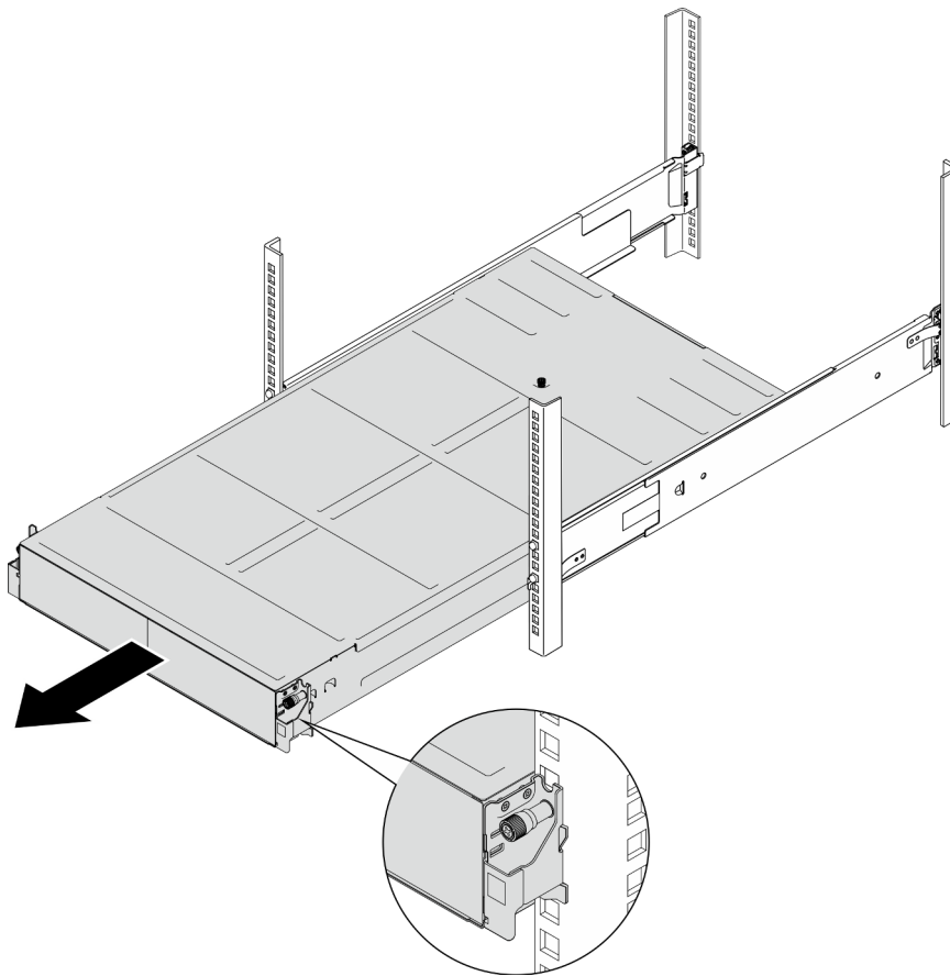
Abbildung 10. Entfernen des Gehäuses
