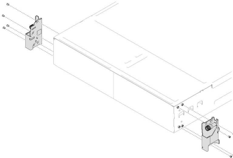
Abbildung 14. Entfernen der EIA-Halterungen
