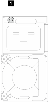
Abbildung 5. Netzteilanzeige
