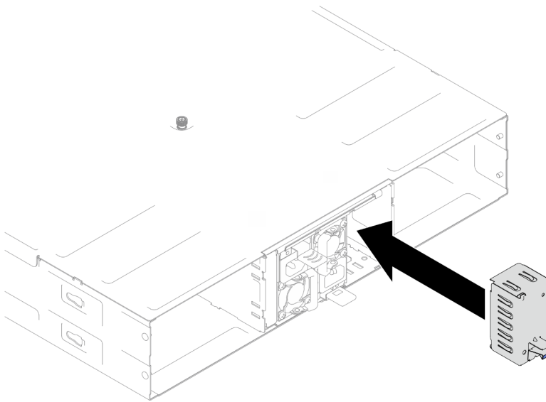
Abbildung 17. Installation einer PSU-Abdeckblende
