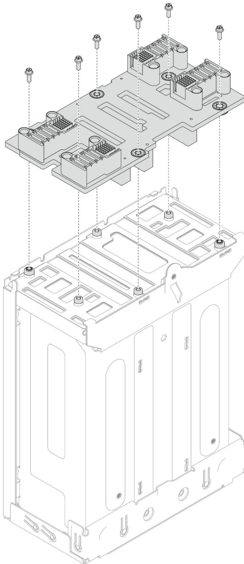
Abbildung 22. Entfernen der Gehäusemittelplatte
