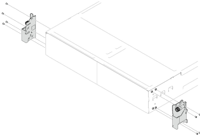
Abbildung 15. Installation der EIA-Halterung
