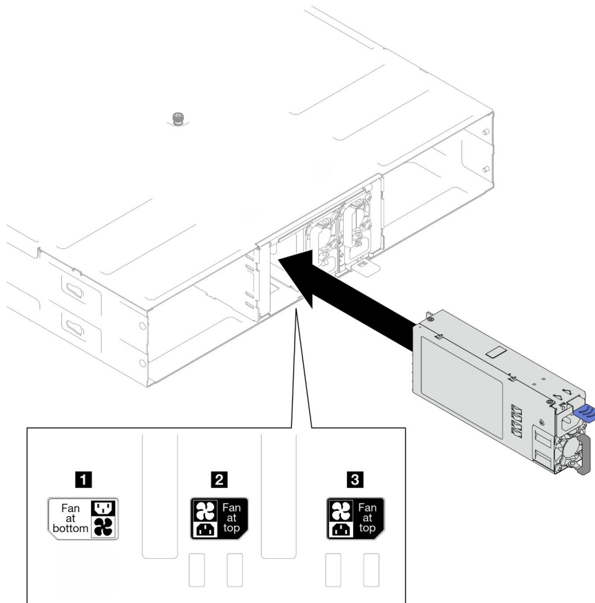
Abbildung 19. Installation eines Hot-Swap-Netzteils
