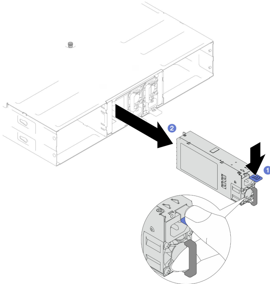
Abbildung 16. Entfernen eines Hot-Swap-PSUs
