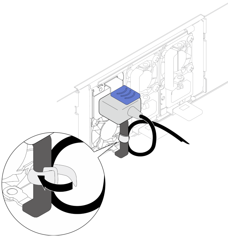
Abbildung 20. Verlegen und Befestigen des Netzkabels
