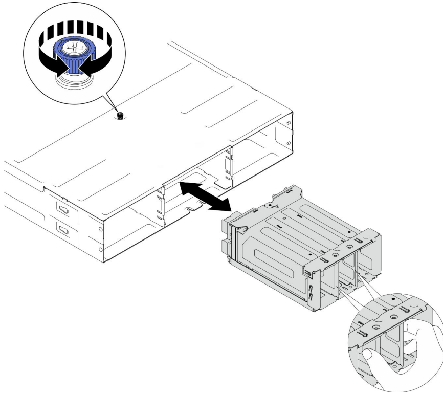
Abbildung 24. Installation des PSU-Rahmens
