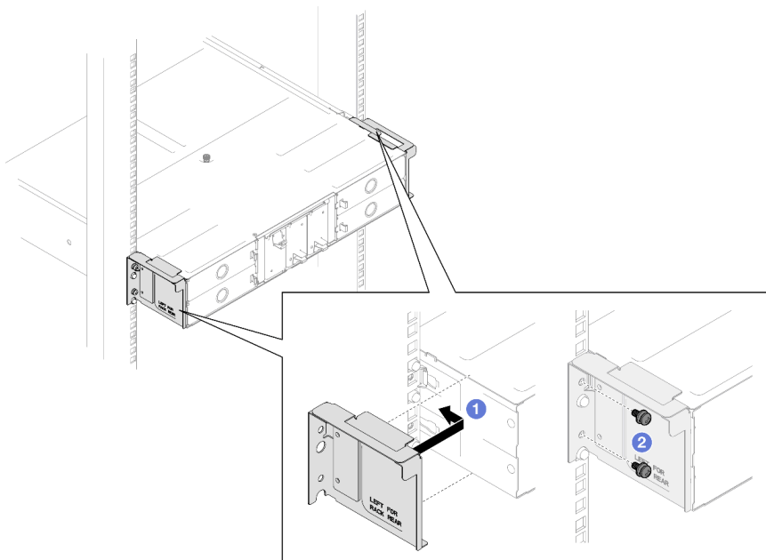
Abbildung 13. Installation von Transporthalterungen für 29,5 Zoll tiefe Racks
