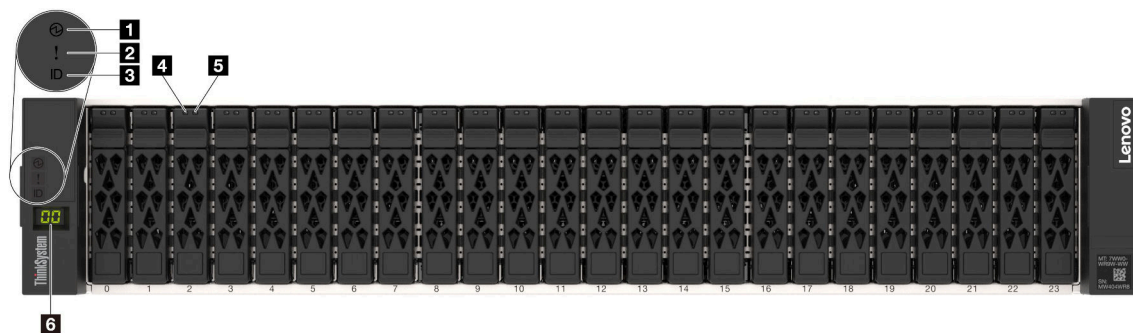
図 1. ベゼルなしの前面図
