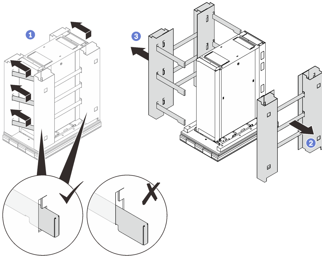
Figure 5. Retrait des cadres latéraux
