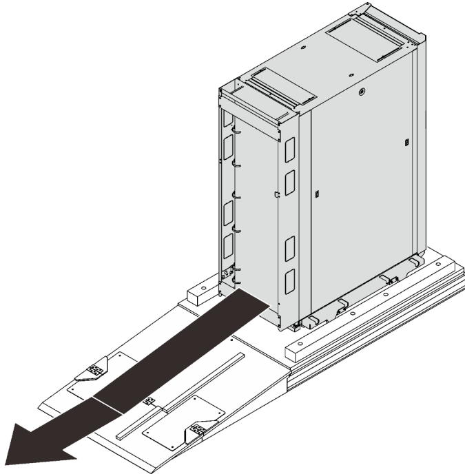
Figure 11. Déplacement de l'armoire
