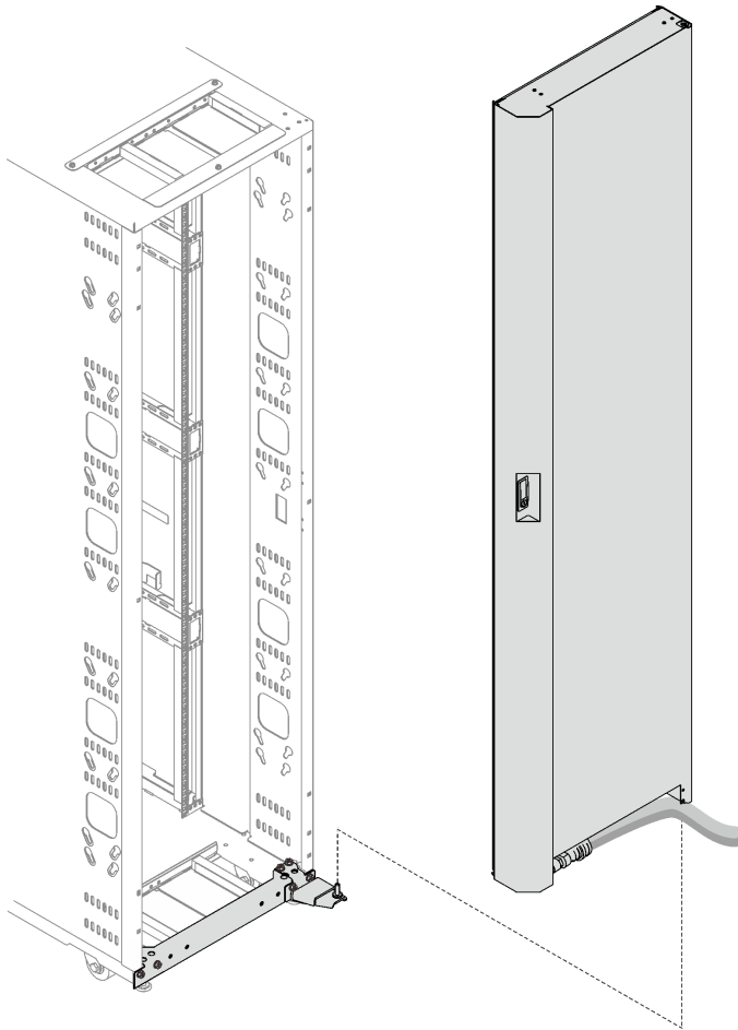
Figure 55. Retrait de l'échangeur de chaleur de l'armoire
