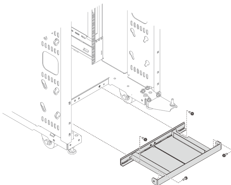
Figure 16. Installation de la grille d'aération inférieure
