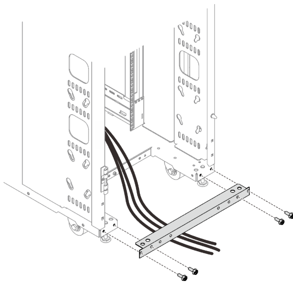
Figure 15. Retrait de la barre d'accès aux câbles
