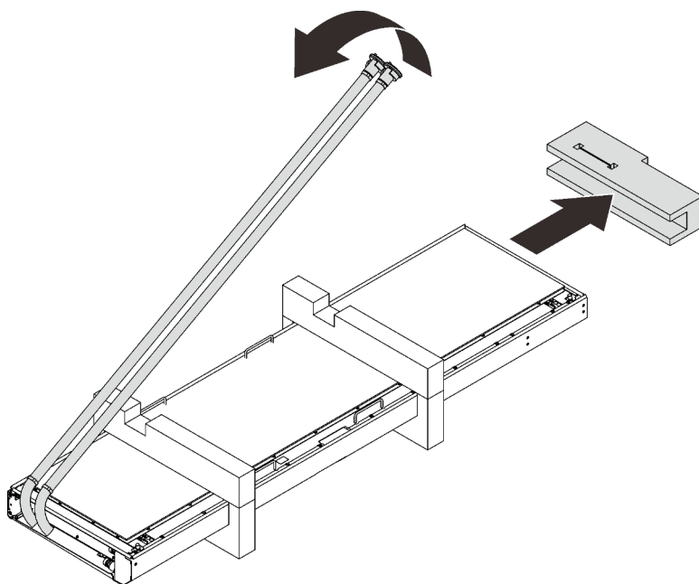
Figure 22. Retrait du matériau de retenue
