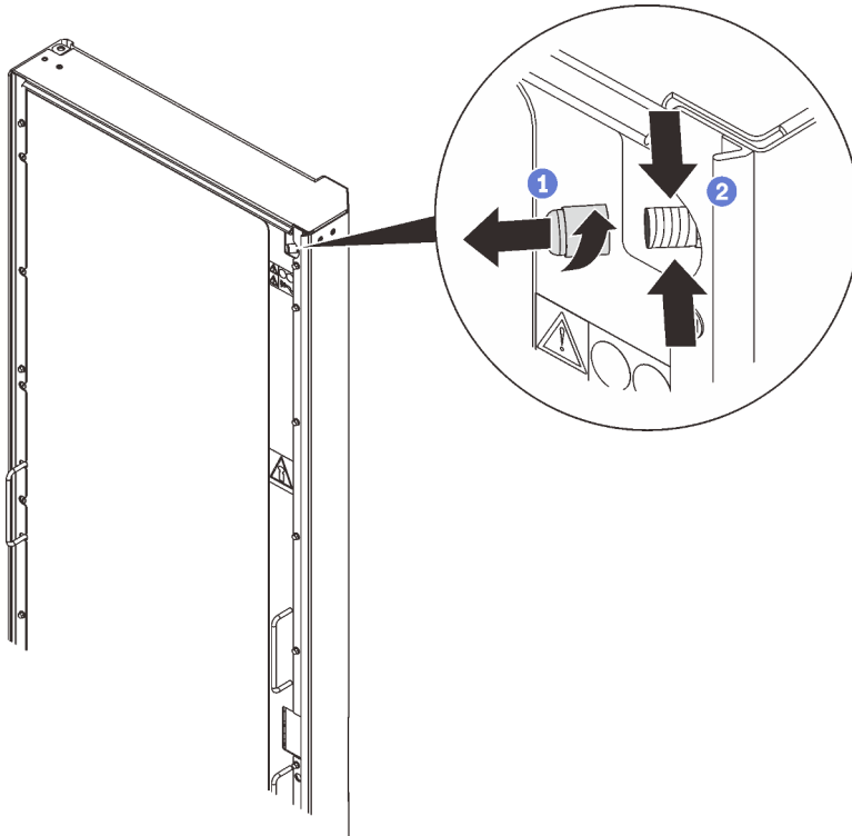
Figure 64. Purge de l'azote
