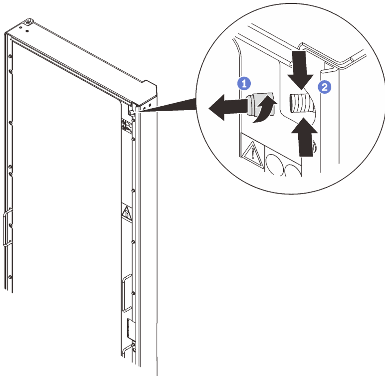
Figure 33. Purge de l'azote
