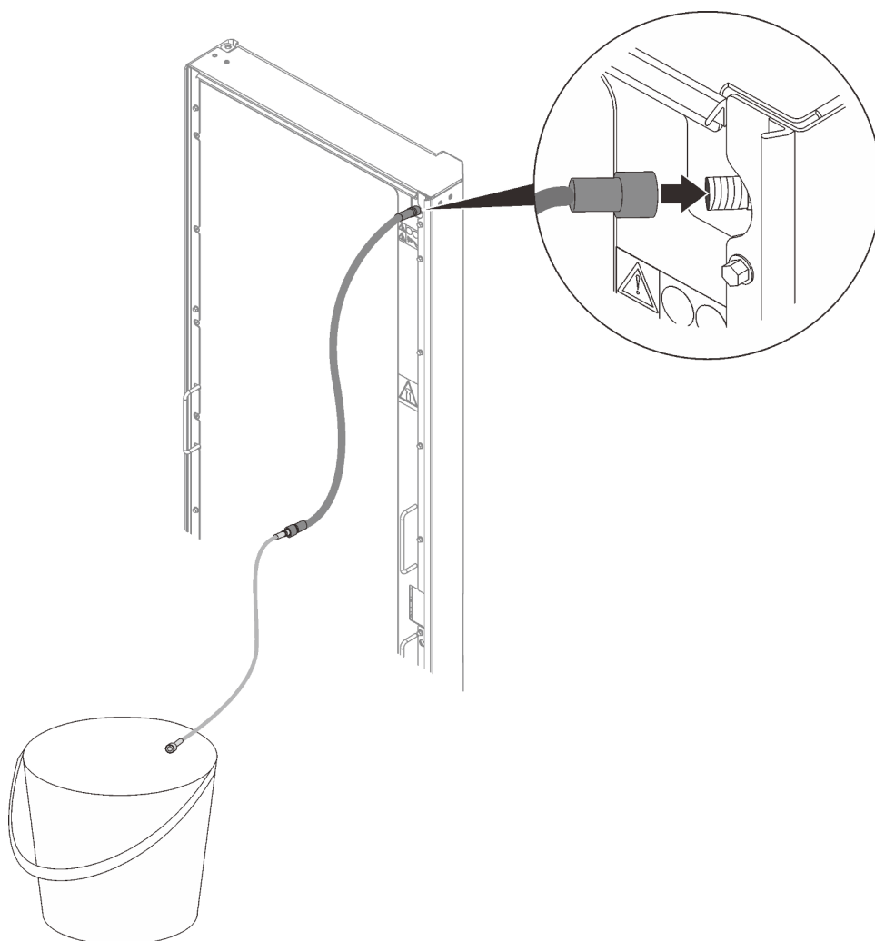
Figure 65. Installation de l'outil de purge d'air
