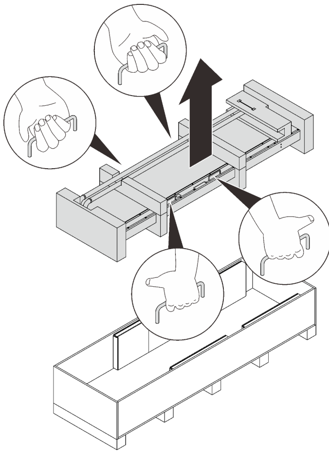
Figure 20. Retrait de l'échangeur de chaleur
