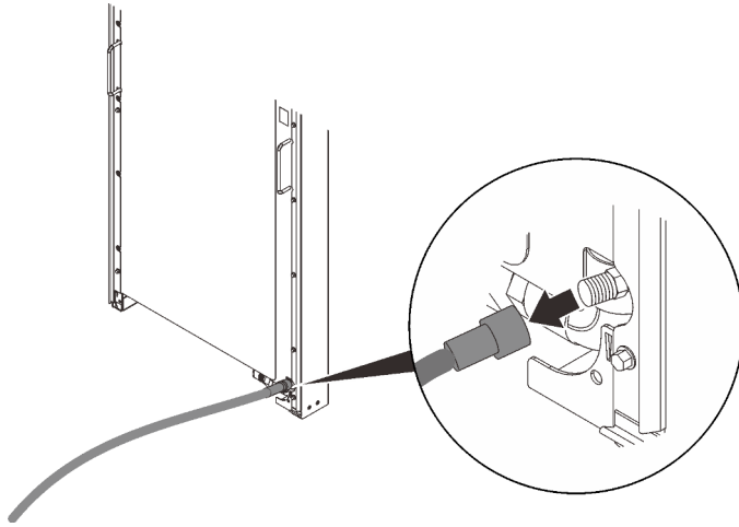
Figure 51. Retrait de l'outil de purge d'air
