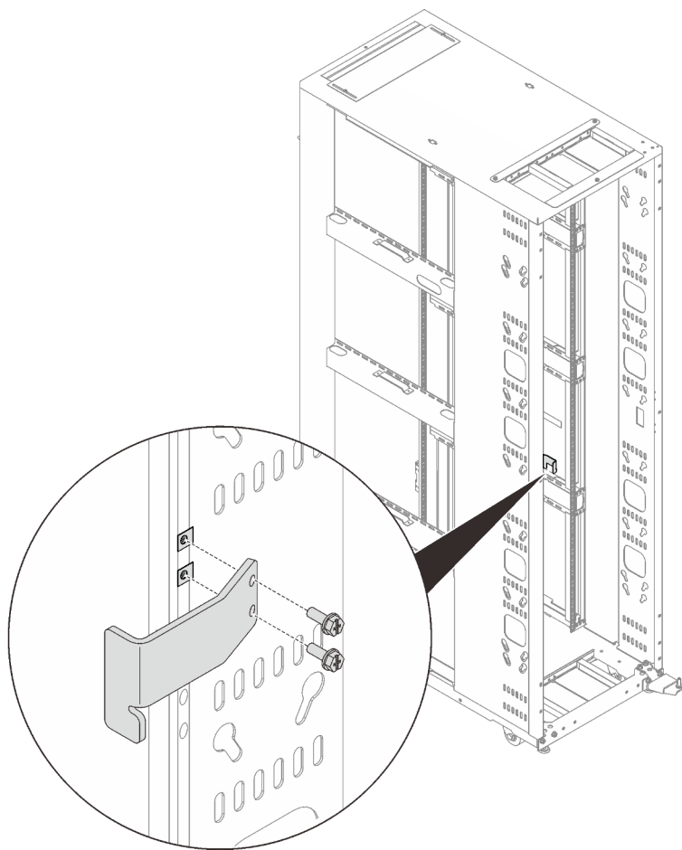
Figure 18. Installation de la plaque de verrouillage
