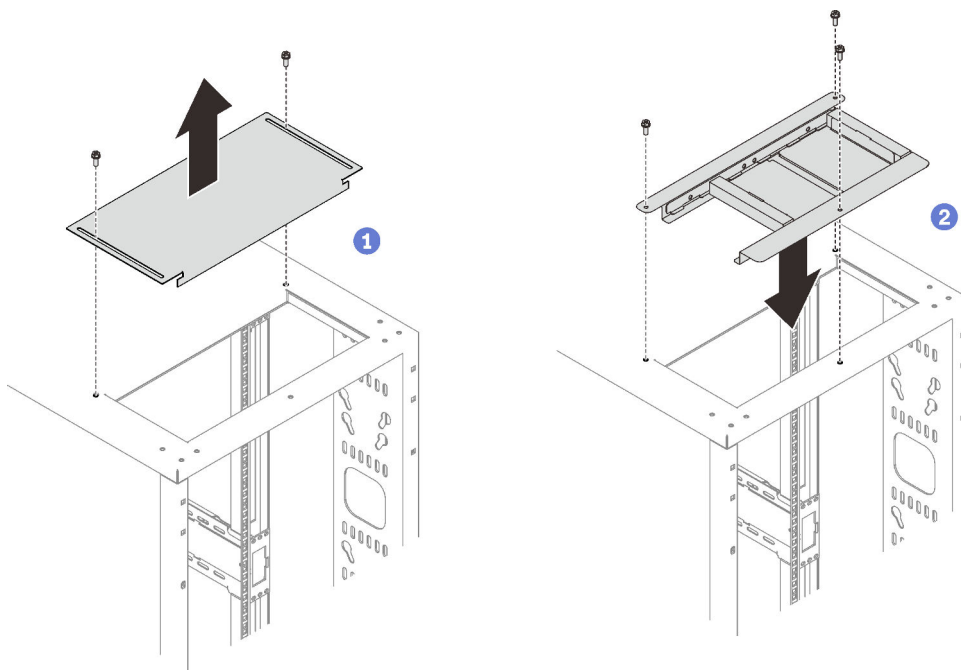
Figure 14. Installation de la grille d'aération supérieure
