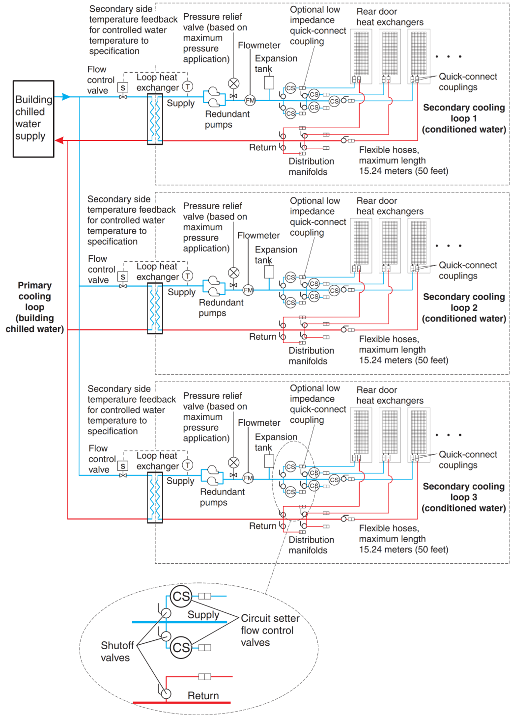
Figure 27. Circuits de refroidissement principal et secondaire
