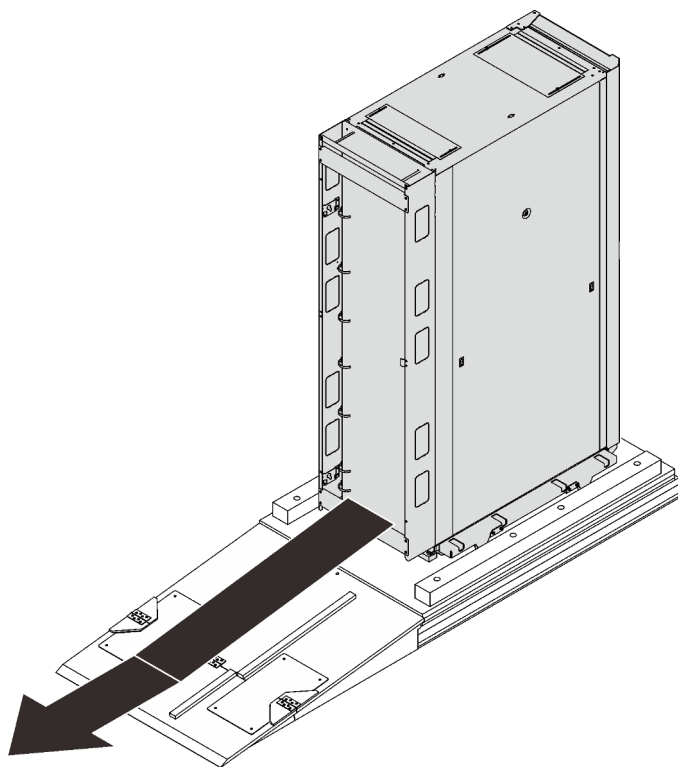
Figure 6. Déplacement de l'armoire depuis la palette
