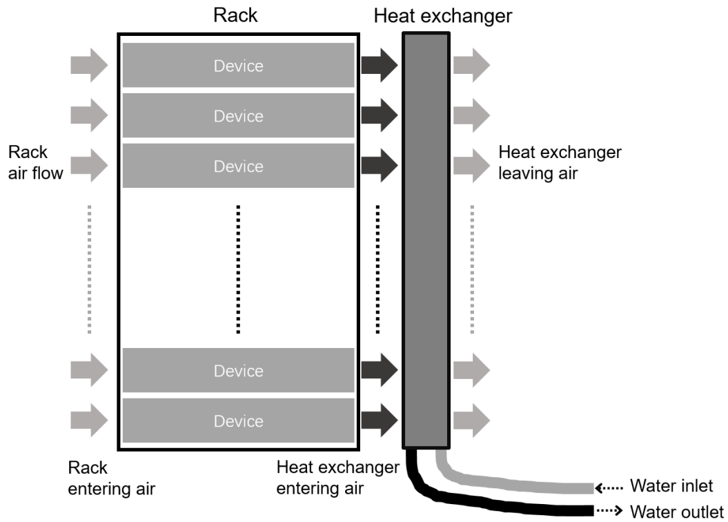
Figure 2. Schéma du débit d'air de l'armoire et du débit d'eau de l'échangeur de chaleur
