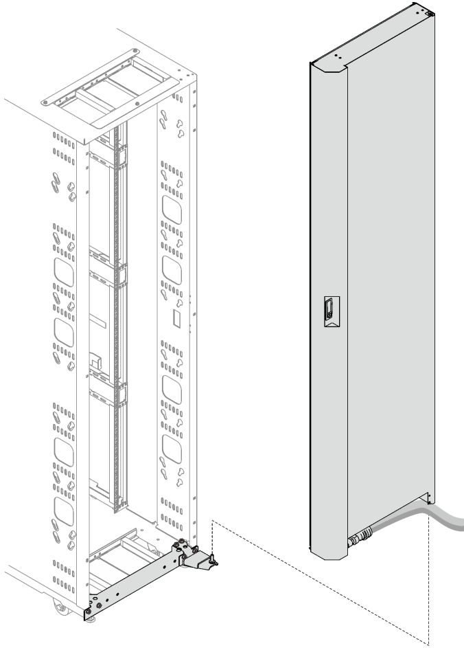
Figure 25. Installation de l'échangeur de chaleur dans l'armoire
