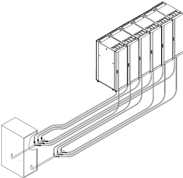
Figure 31. Collecteur central classique (dans un emplacement central pour plusieurs circuits d'eau)
