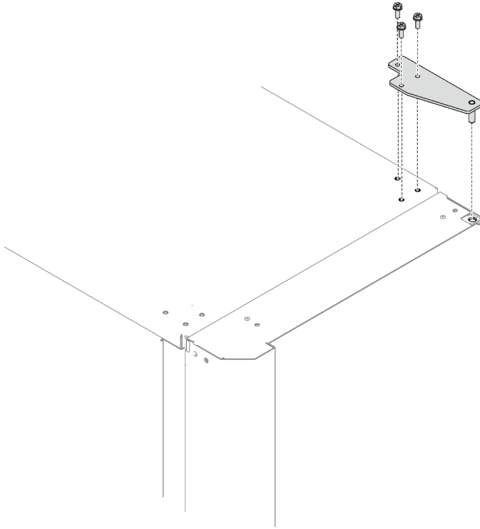
Figure 63. Installation de la charnière supérieure
