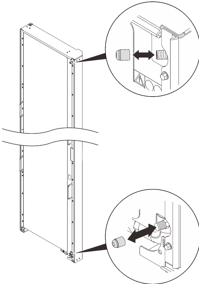
Figure 52. Installation des bouchons de valve
