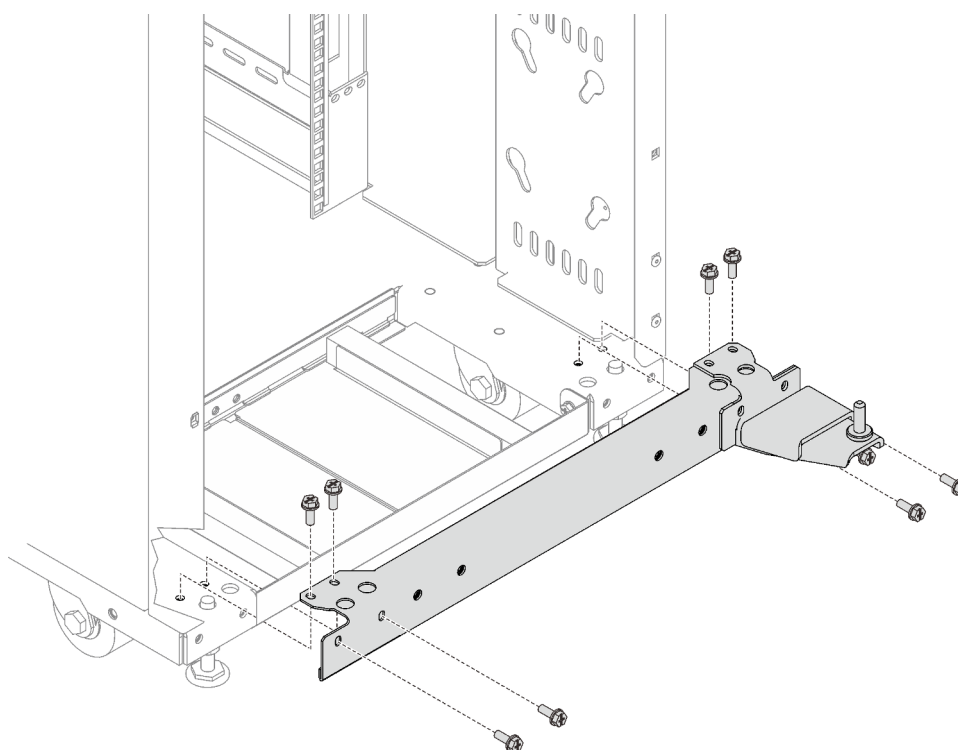
Figure 17. Installation du bloc charnière inférieur
