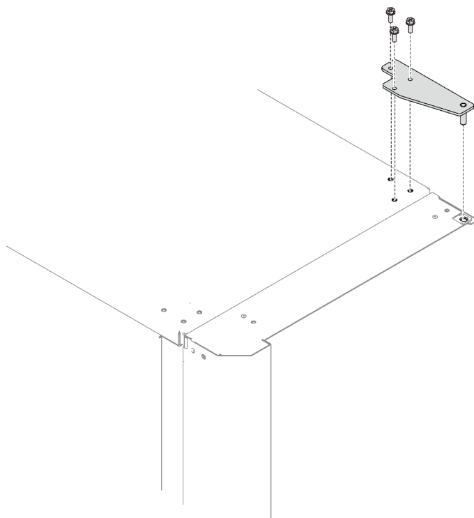
Figure 26. Installation de la charnière supérieure
