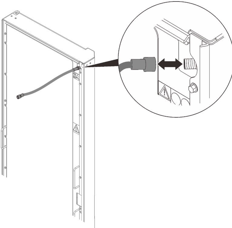
Figure 50. Retrait de la rallonge de l'outil de purge d'air
