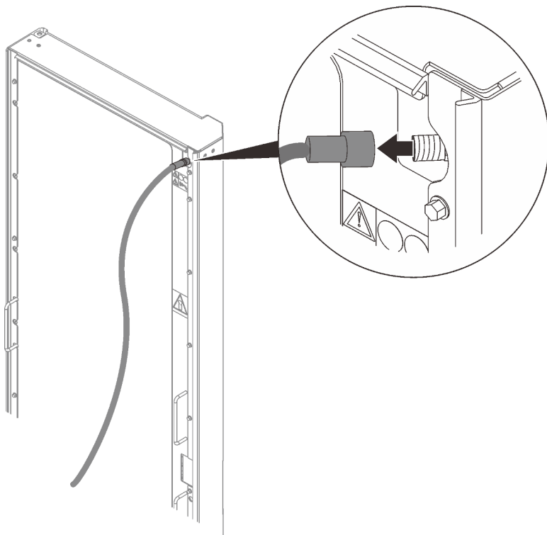
Figure 36. Retrait de l'outil de purge d'air
