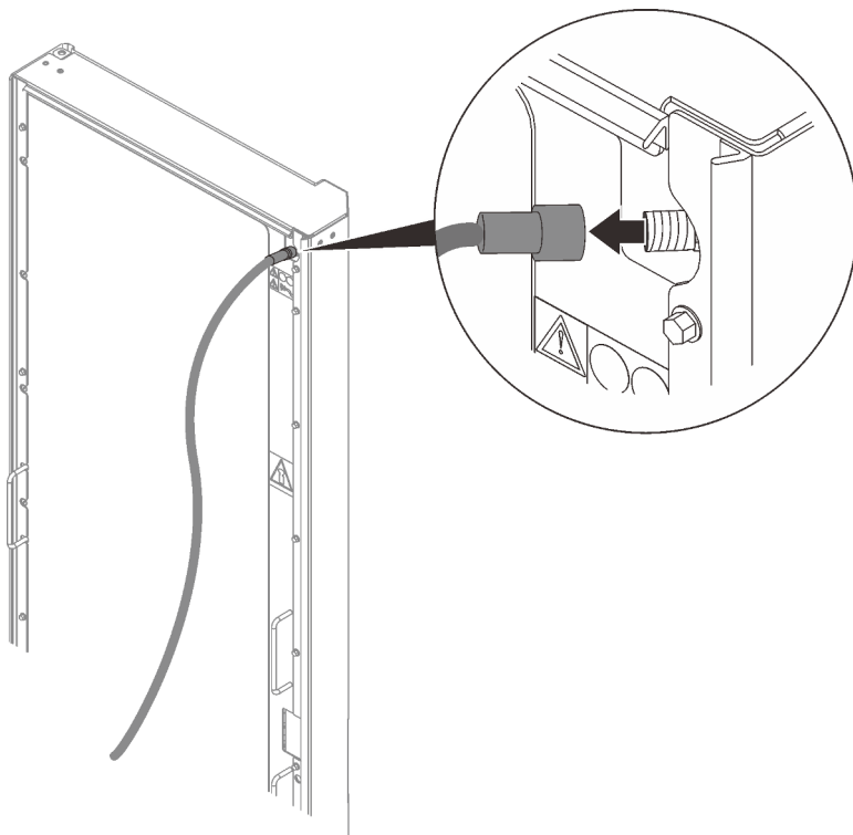
Figure 67. Retrait de l'outil de purge d'air
