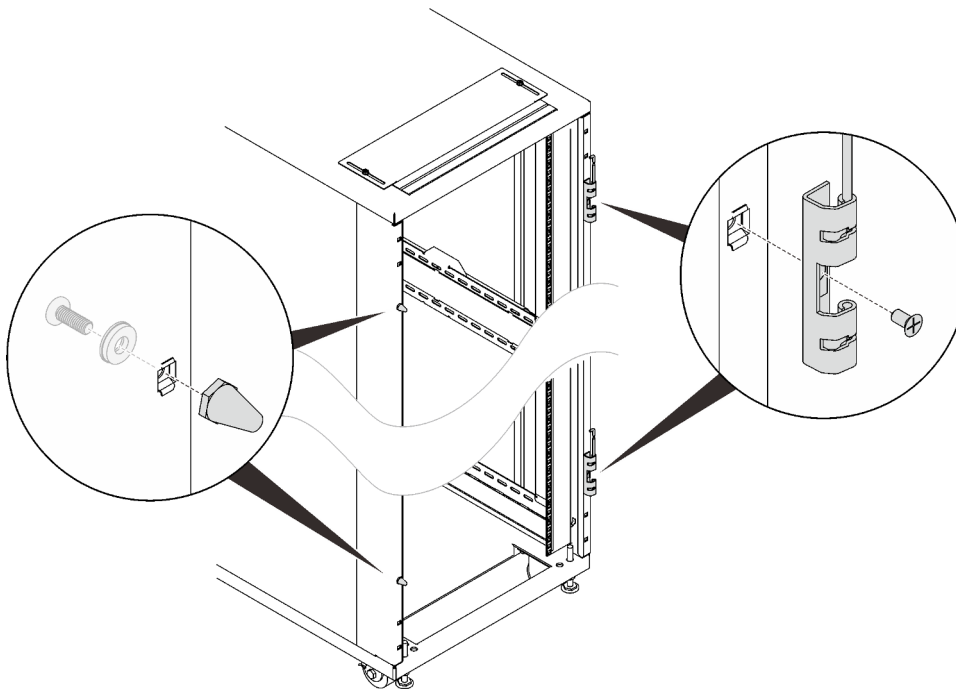
Figure 12. Retrait des charnières et des butées de porte
