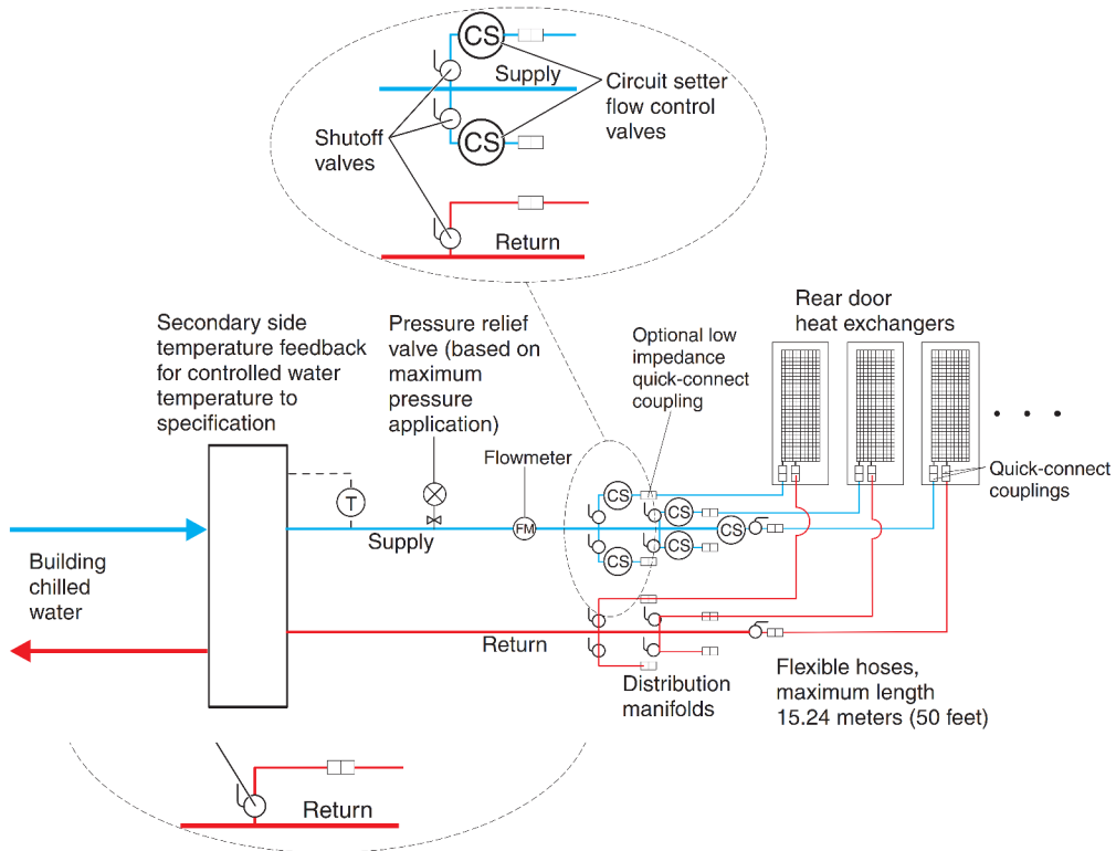
Figure 29. Unité de liquide de refroidissement utilisant des solutions du commerce prêtes à l'emploi
