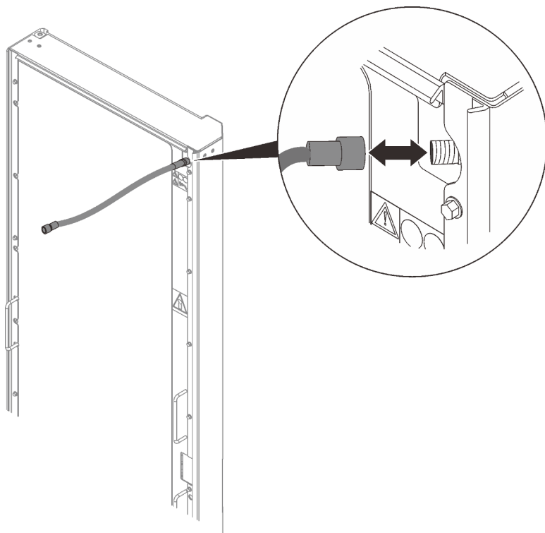
Figure 48. Insertion du tuyau d'extension de l'outil de purge d'air
