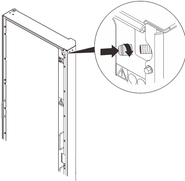
Figure 68. Installation du capuchon de la valve
