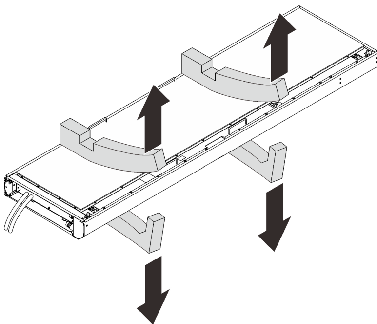
Figure 23. Retrait des matériaux d'emballage
