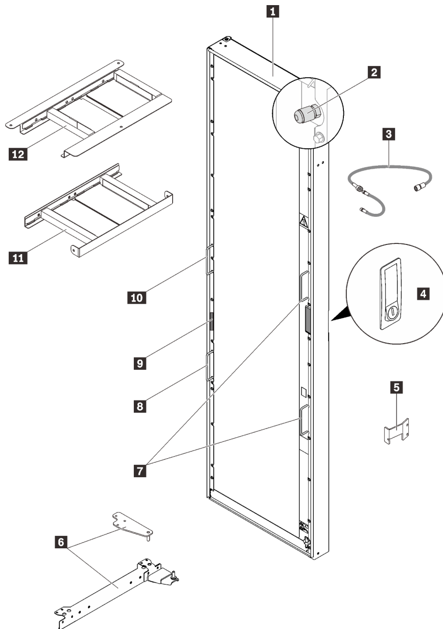
Figure 1. Composants du ThinkSystem Rear Door Heat eXchanger pour armoire 48U
