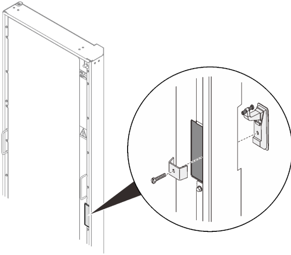
Figure 69. Remplacement du loquet de porte
