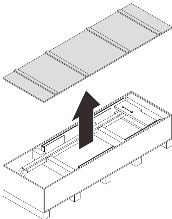
Figure 19. Retrait du couvercle de la boîte
