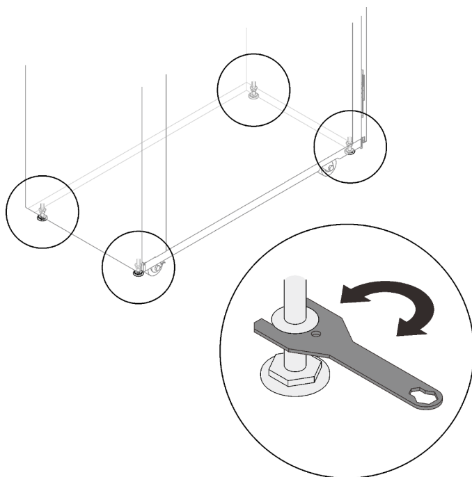
Figure 10. Abaissement des vérins de mise à niveau
