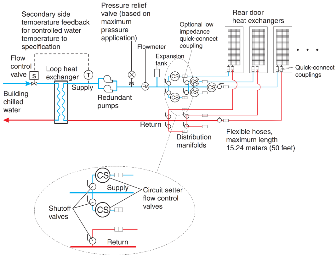
Figure 28. Unité de distribution de liquide de refroidissement avec une solution fabriquée pour des équipements
