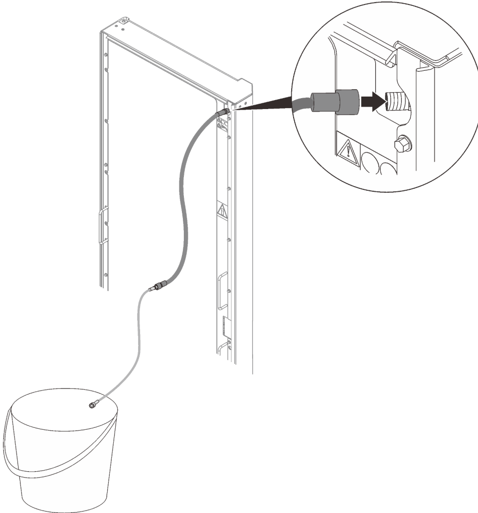
Figure 34. Installation de l'outil de purge d'air
