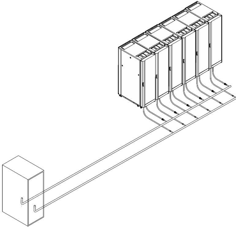
Figure 32. Collecteur étendu classique (le long des allées entre les armoires)
