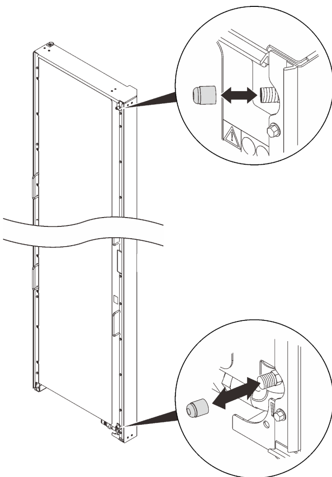
Figure 46. Retrait des bouchons de valve
