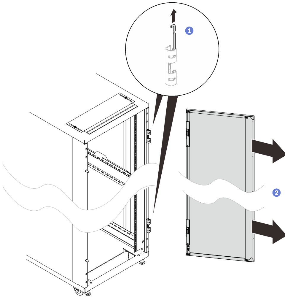
Figure 11. Retrait d'une porte
