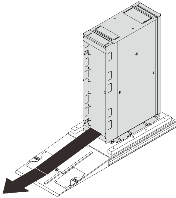
図11. 段ボールの取り外し
