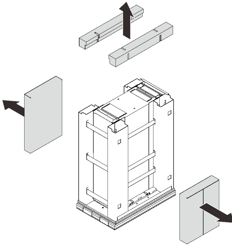
図4. トップ・バーと側面の段ボールの取り外し
