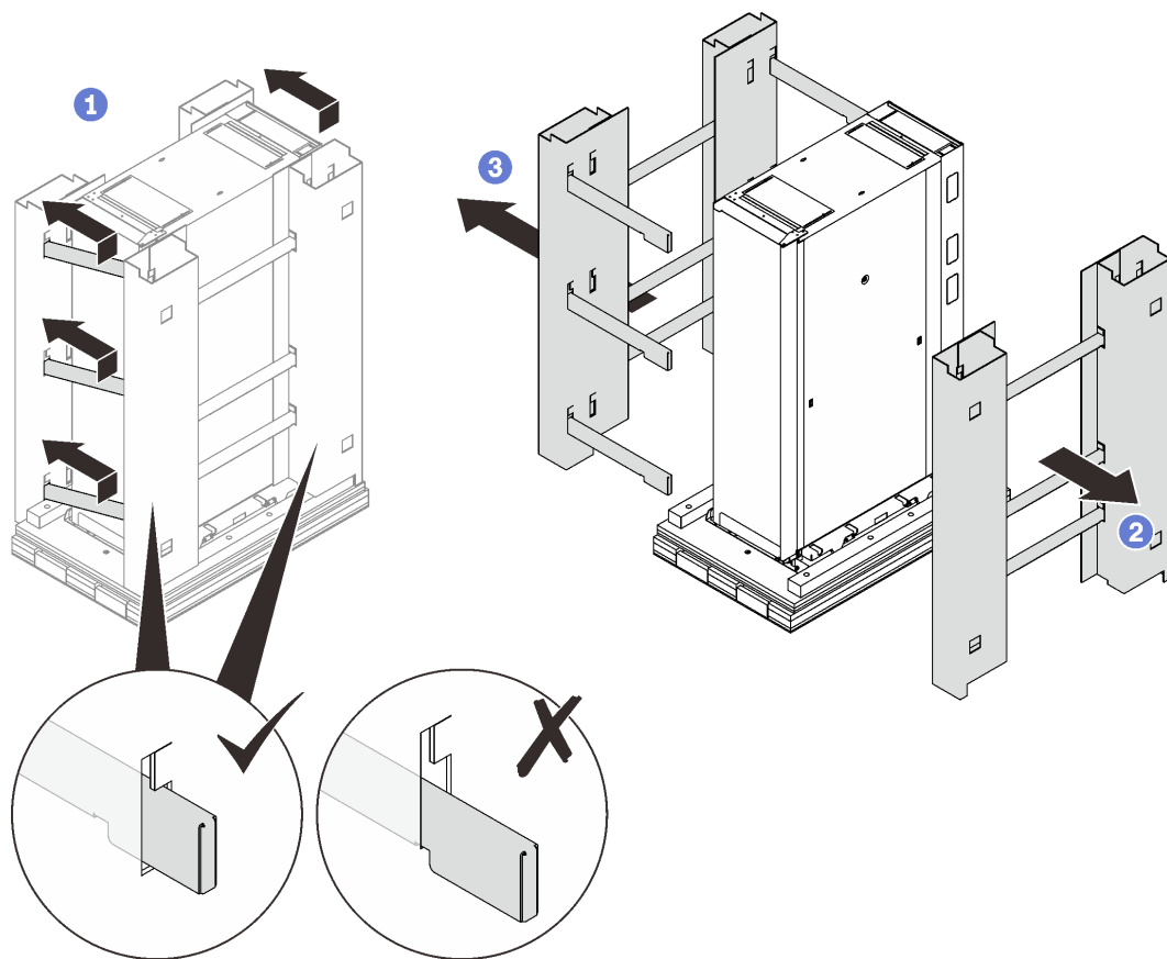
図5. サイド・フレームの取り外し
