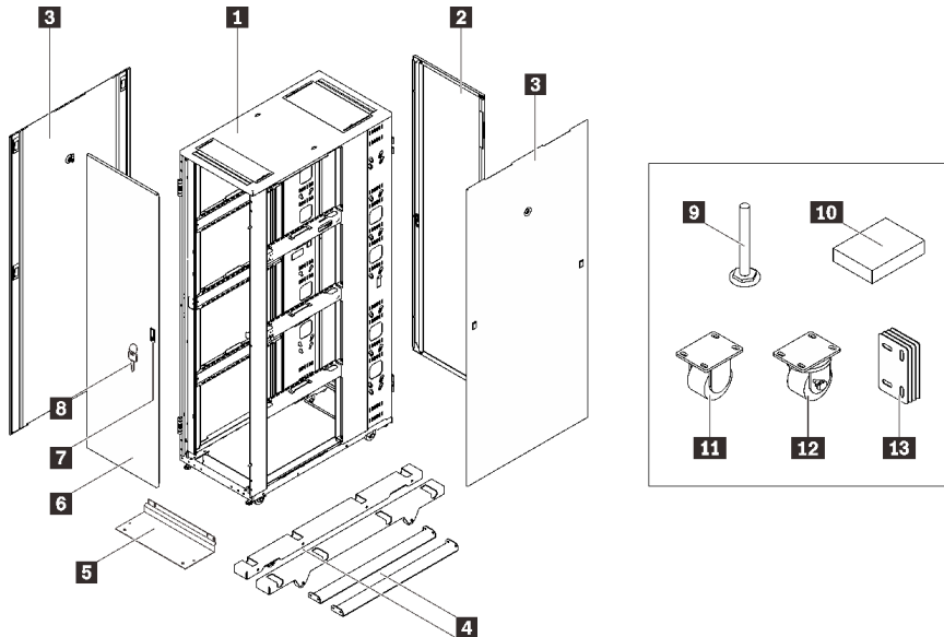
図12. 部品リスト
