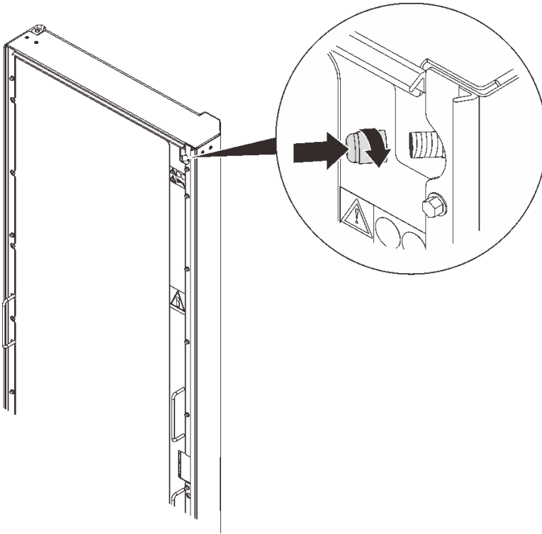
그림 97. 밸브 캡 설치
