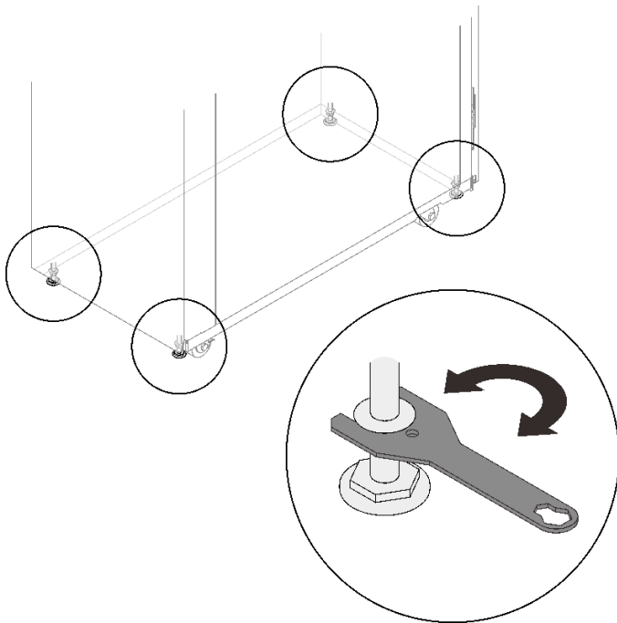
그림 40. 수평 조절 패드 내리기
