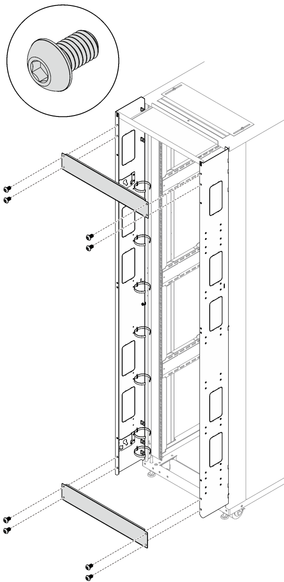
그림 37. 지지 브래킷 설치
