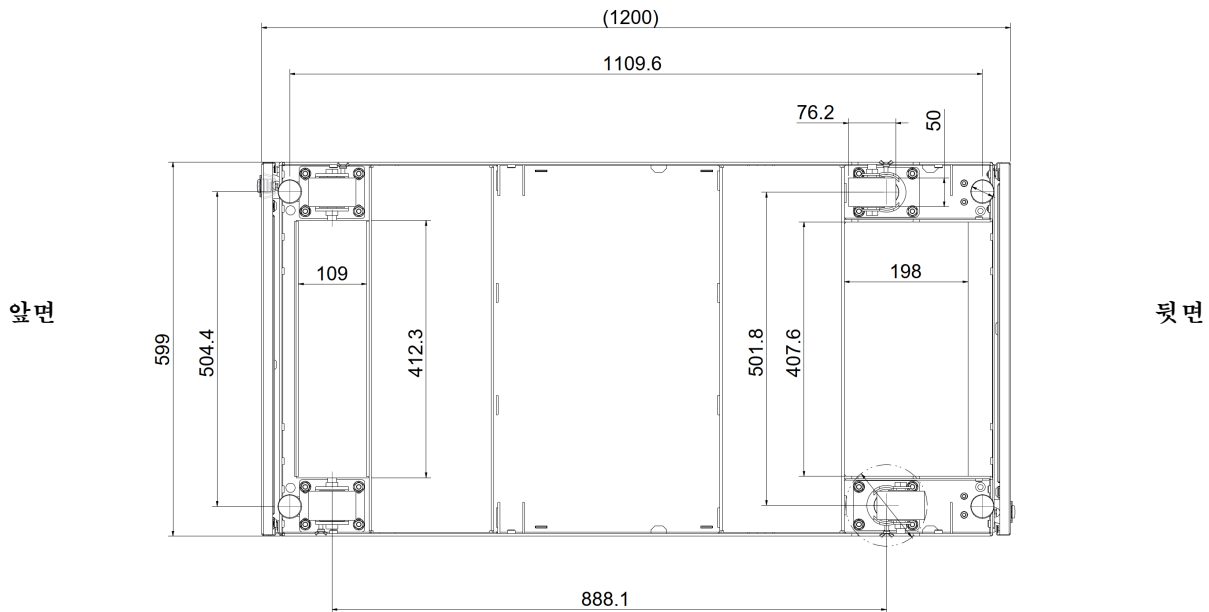
그림 15. 공간 계획(mm)
