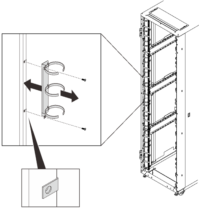
그림 179. 6U 앞면 케이블 관리 브래킷 제거
