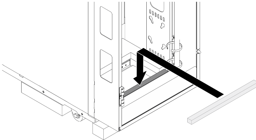
그림 51. 뒷면 폼 설치
