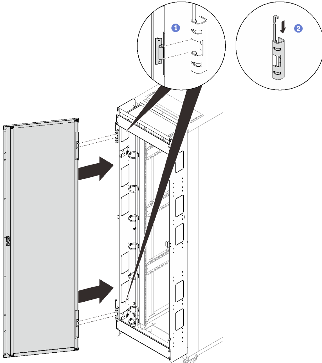
그림 39. 도어 설치
