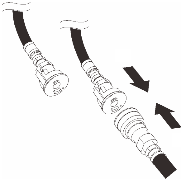
그림 95. 매니폴드 연결
