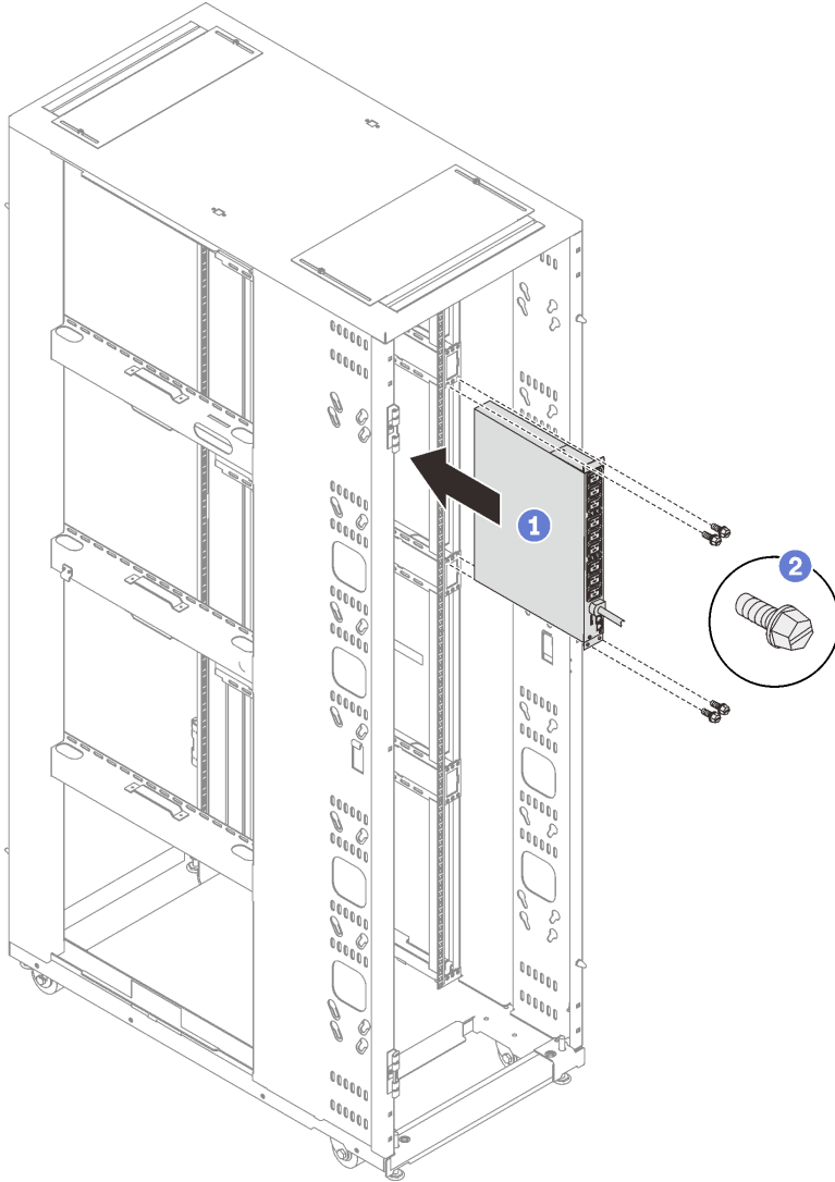
그림 100. 1U PDU 또는 콘솔 스위치 설치
