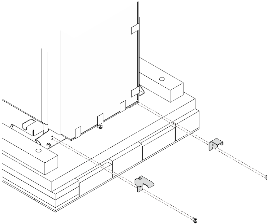
그림 65. 지지 브래킷 제거
