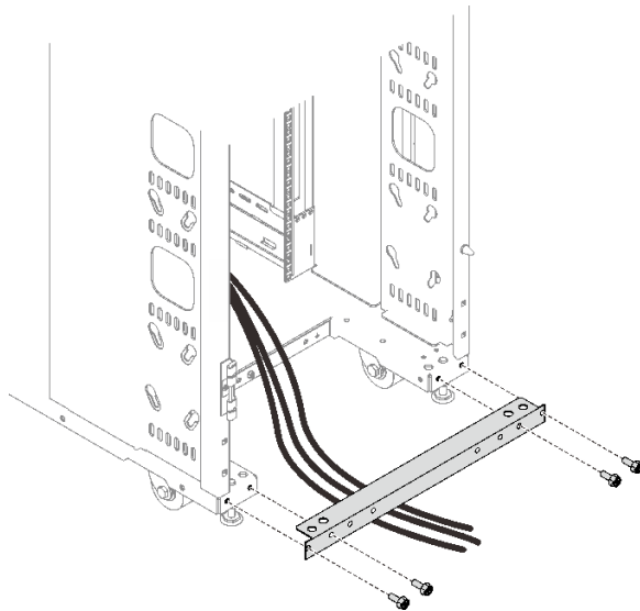
그림 75. 케이블 접근 바 제거
