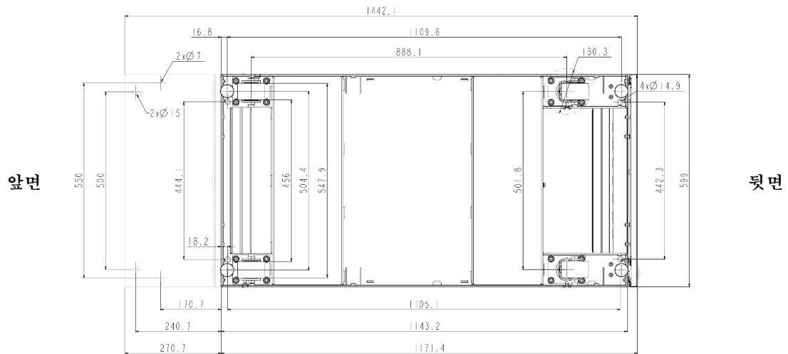
그림 29. 스테빌라이저가 설치된 랙 캐비닛
