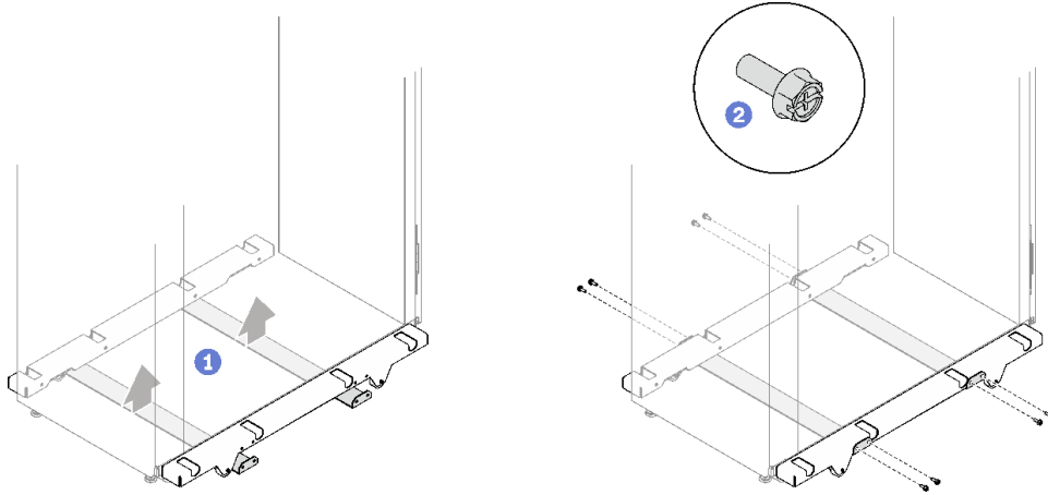
그림 176. 아웃리저 스테빌라이저 바 설치
