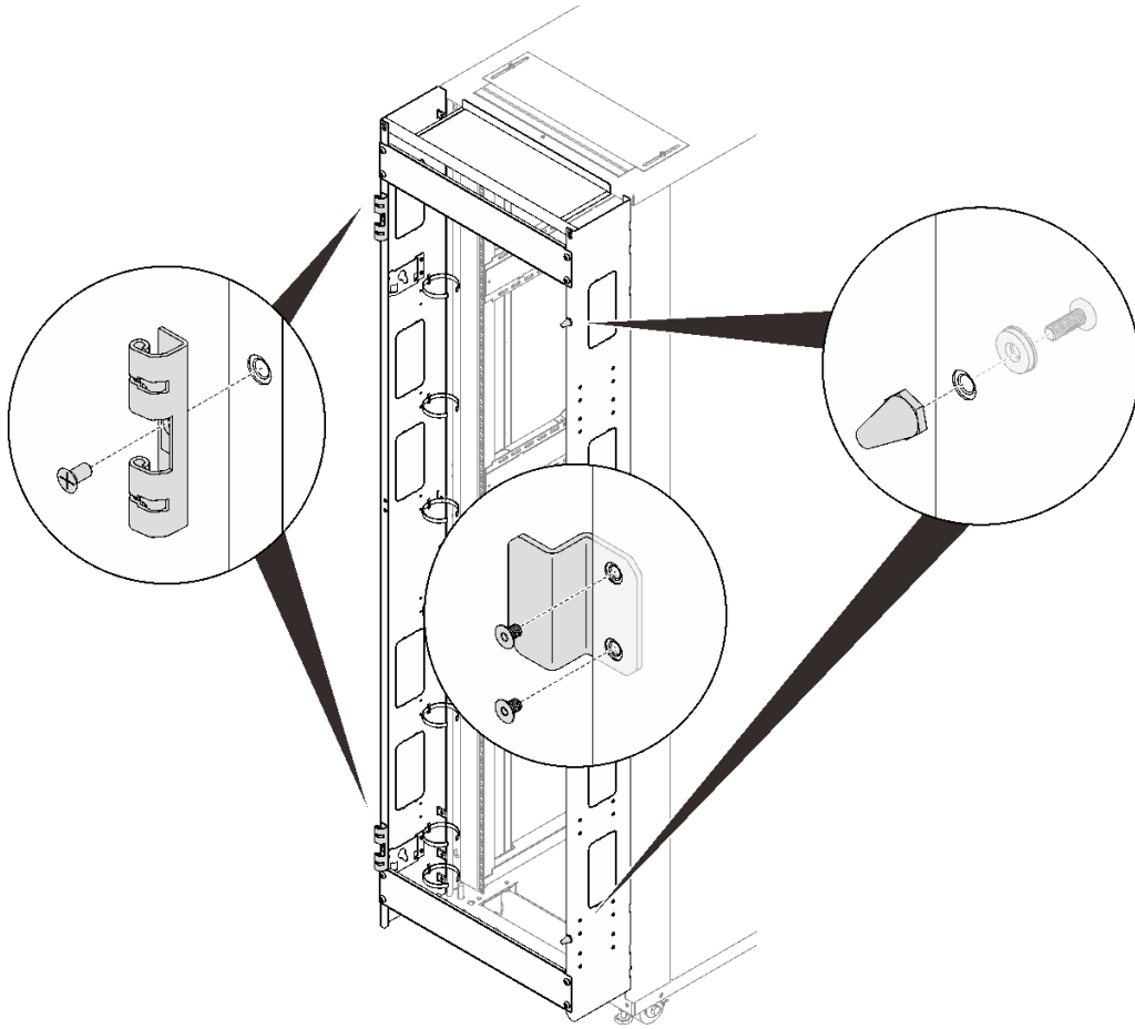
그림 156. 힌지, 도어스토퍼, 도어 래치 설치
