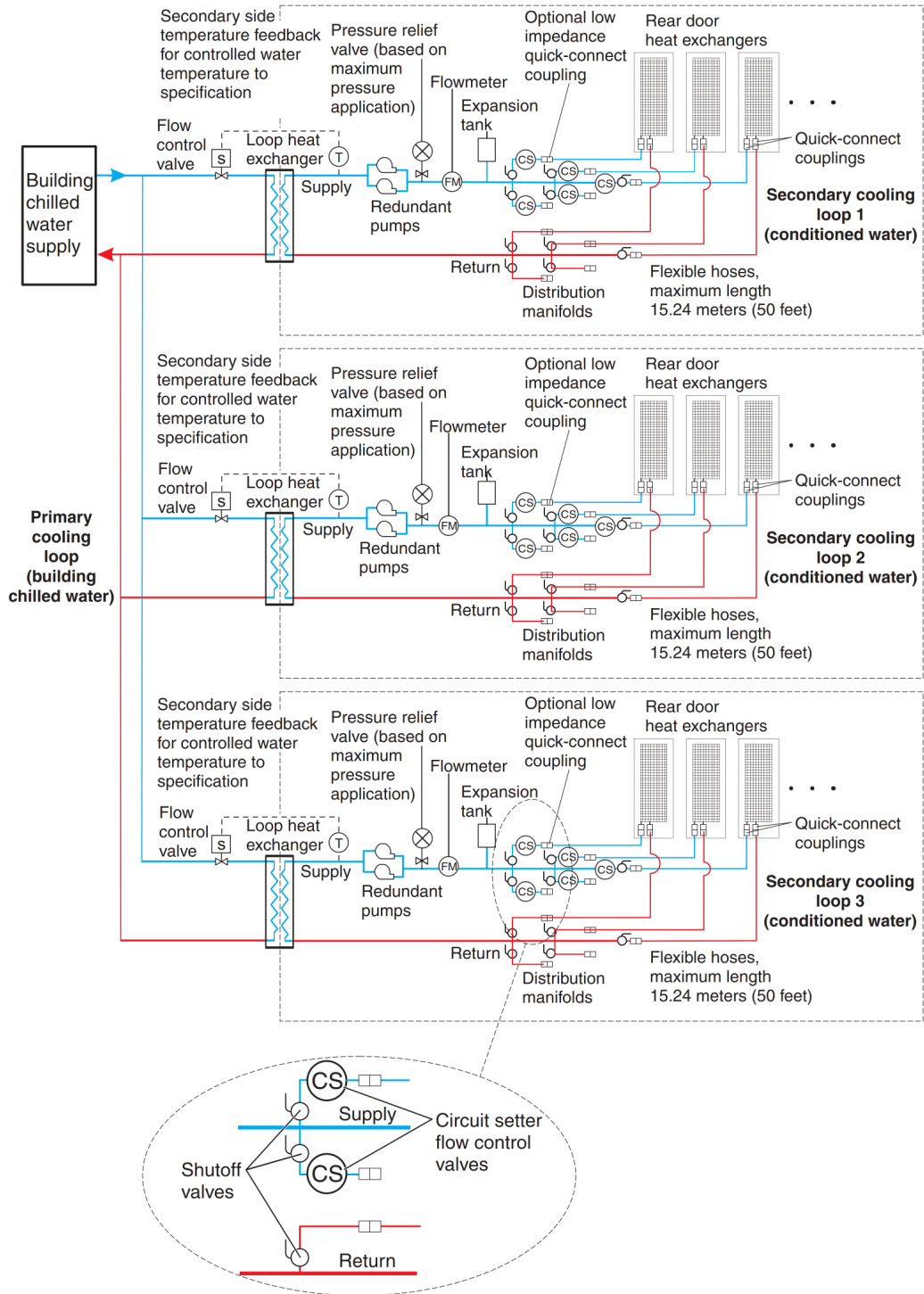
그림 87. 1차 및 2차 냉각 루프
