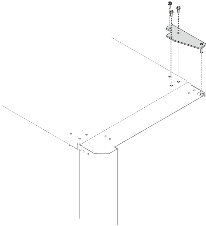
그림 86. 상단 힌지 설치
