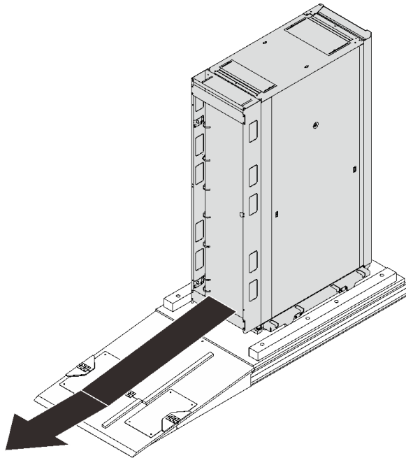
그림 26. 판지 제거
