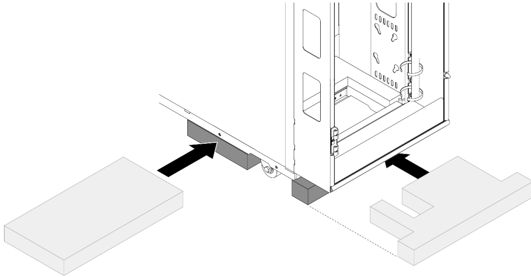
그림 52. 지면 폼 설치
