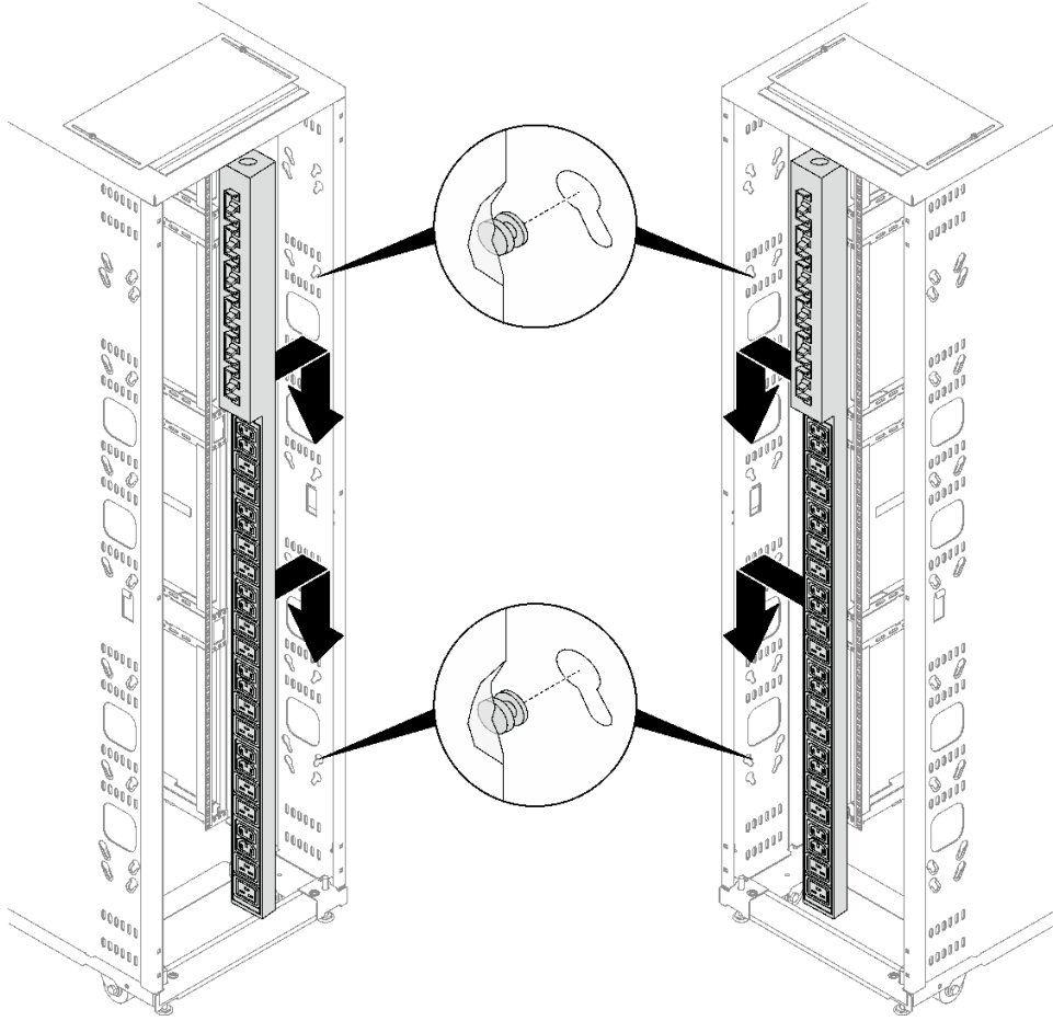
그림 98. 0U PDU 설치
