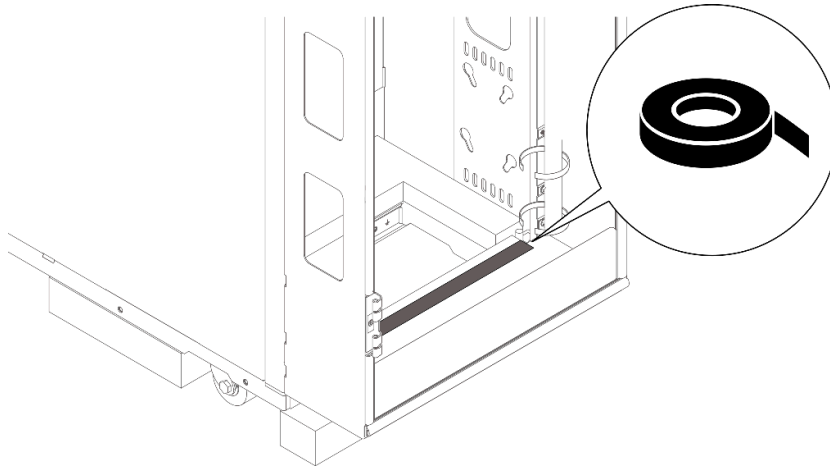
그림 49. 실링 폼 설치
