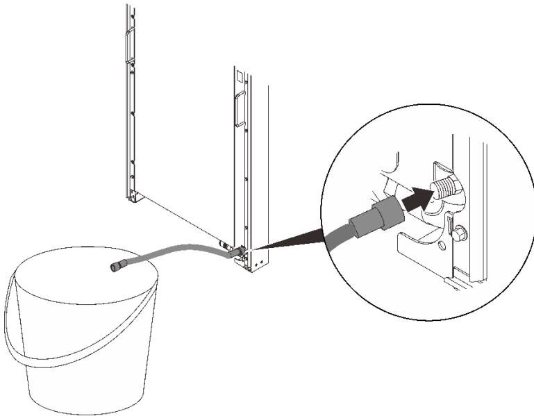
그림 130. 배수
