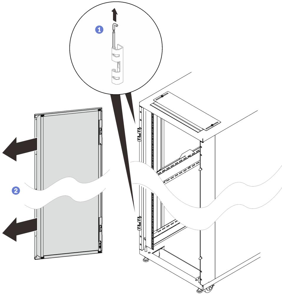
그림 31. 도어 제거
