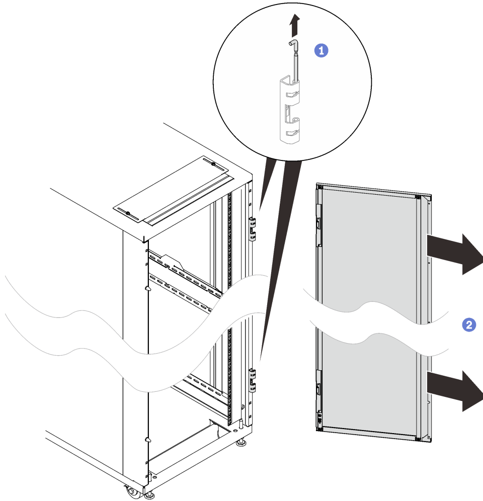
그림 71. 도어 제거
