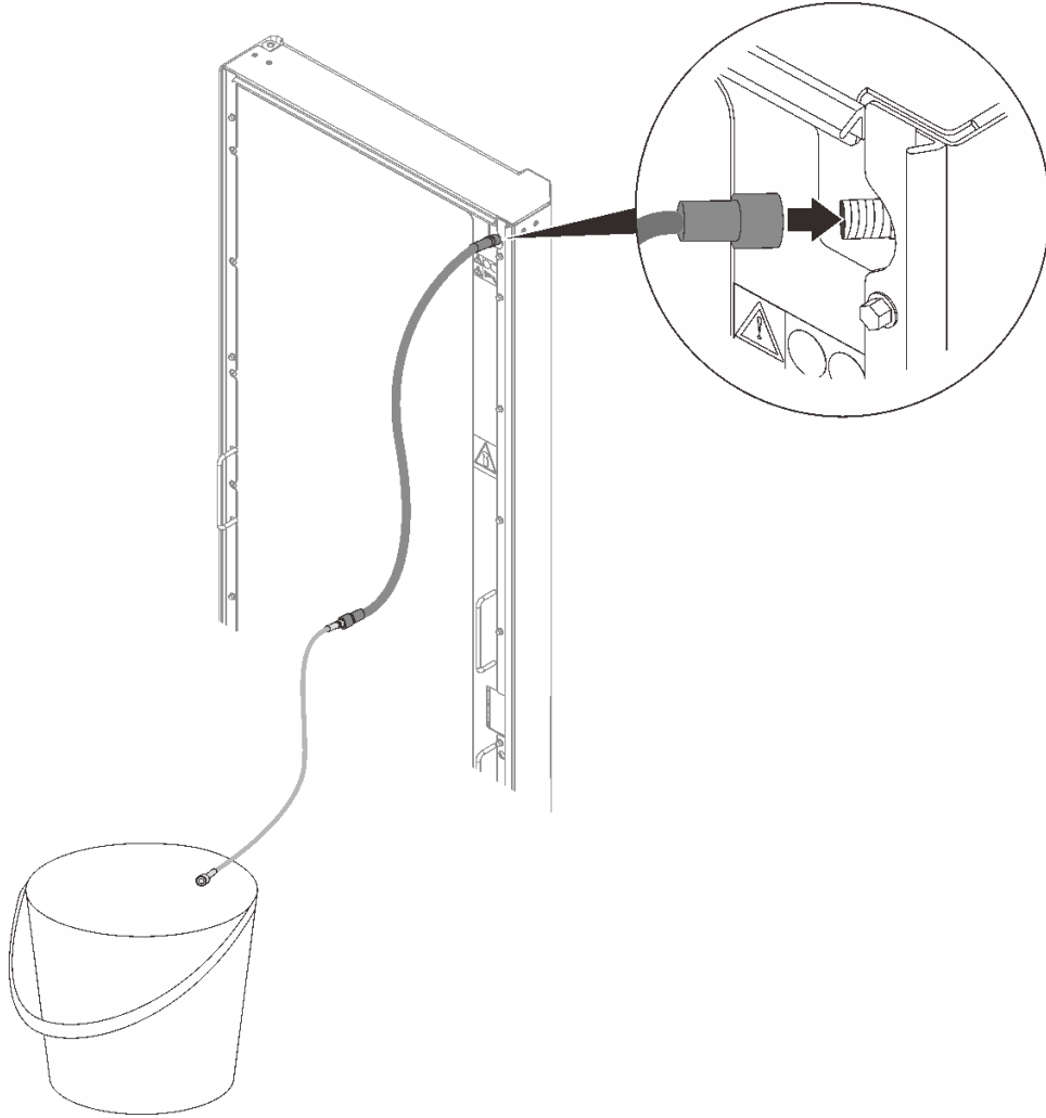
그림 146. 에어 퍼지 도구 설치
