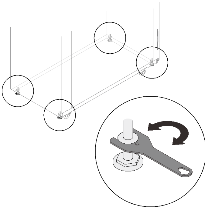
그림 23. 수평 조절 패드 올리기
