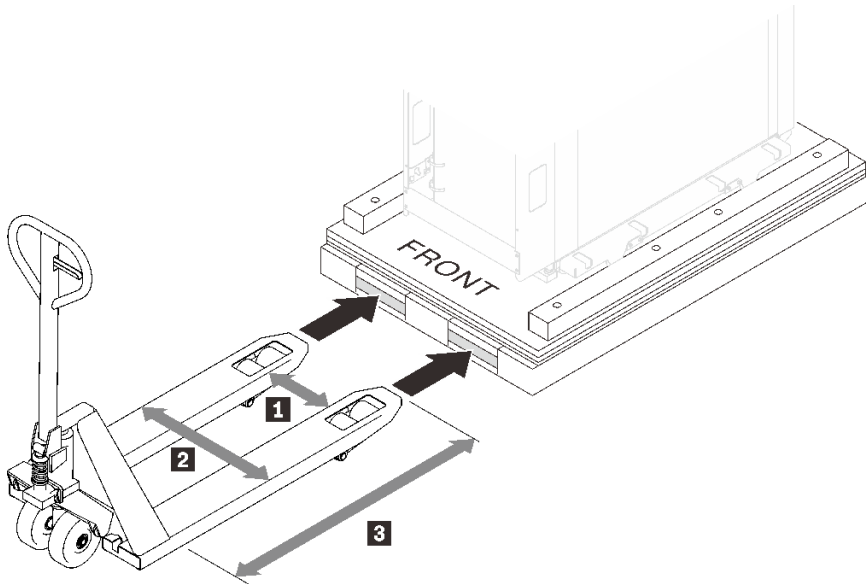
그림 16. 지게차
