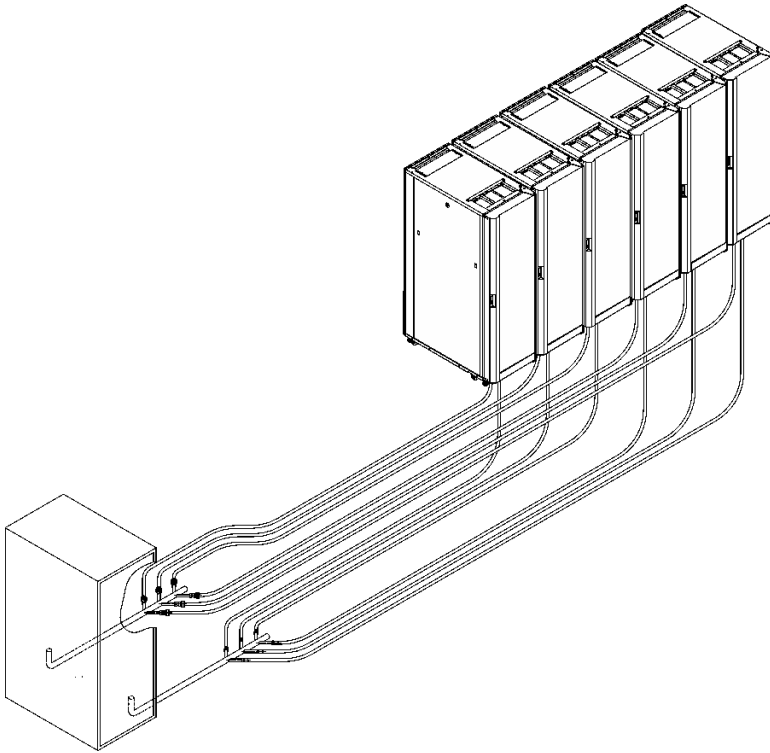
그림 91. 일반적인 중앙 매니폴드(다중 물 회로의 중앙 위치)
