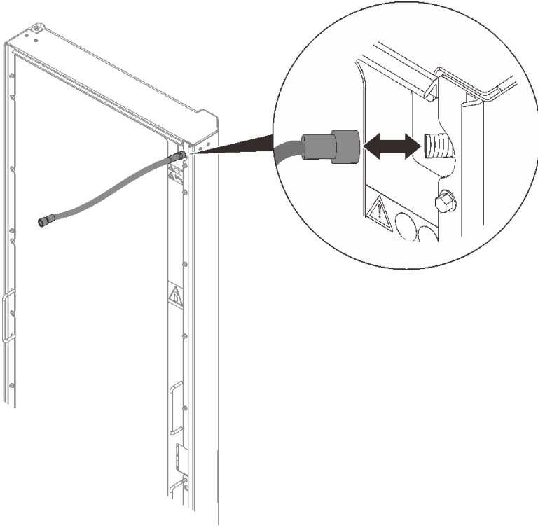
그림 131. 에어 퍼지 도구 연장 호스 제거
