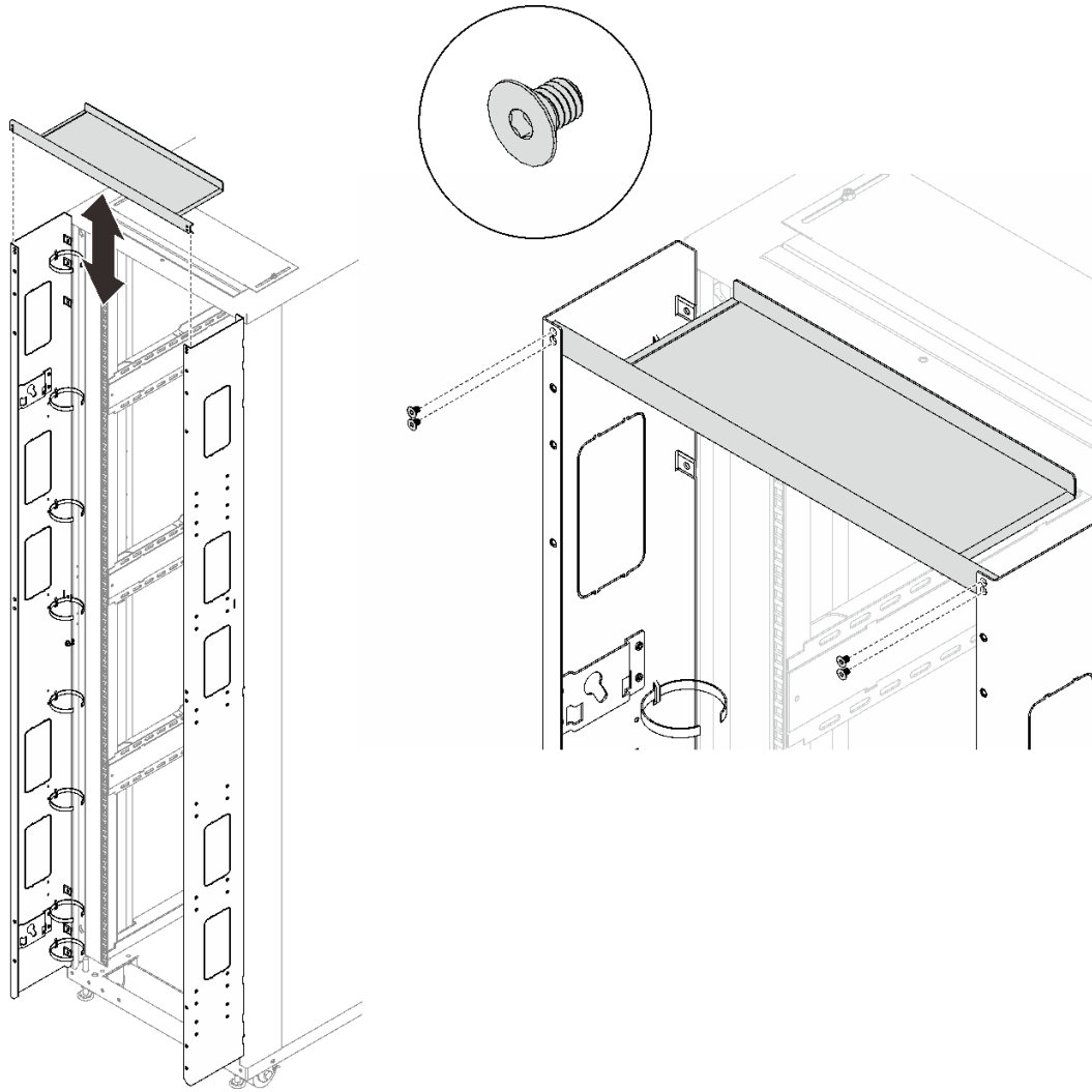
그림 160. 뒷면 덮개 제거
