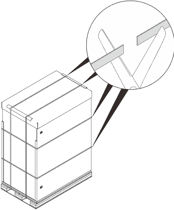
그림 17. 스트랩 자르기
