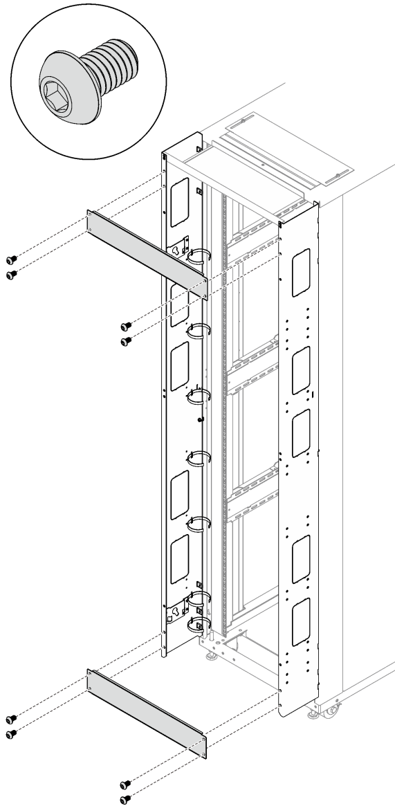
그림 155. 지지 브래킷 설치
