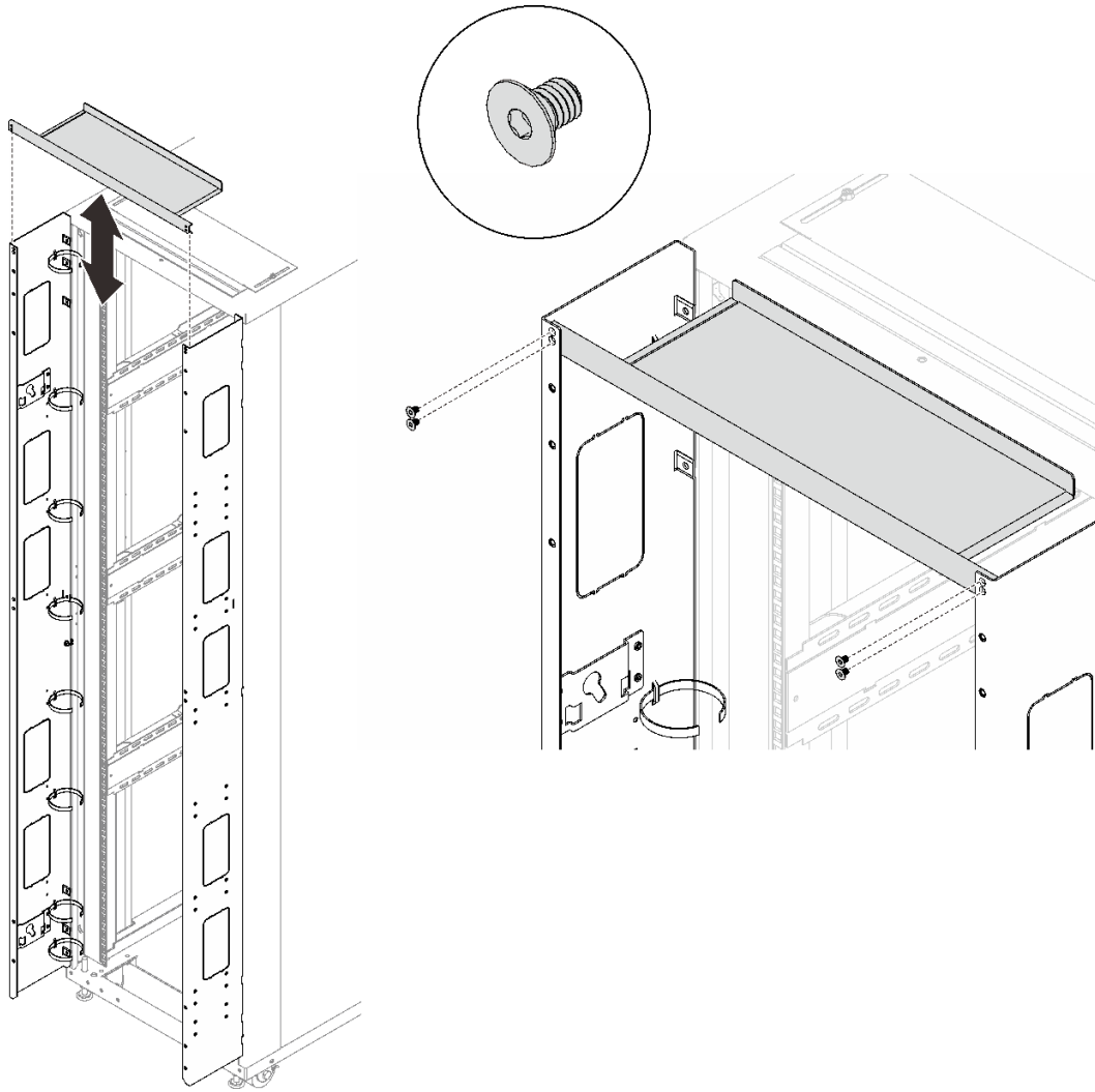
그림 36. 확장 윗면 덮개 설치
