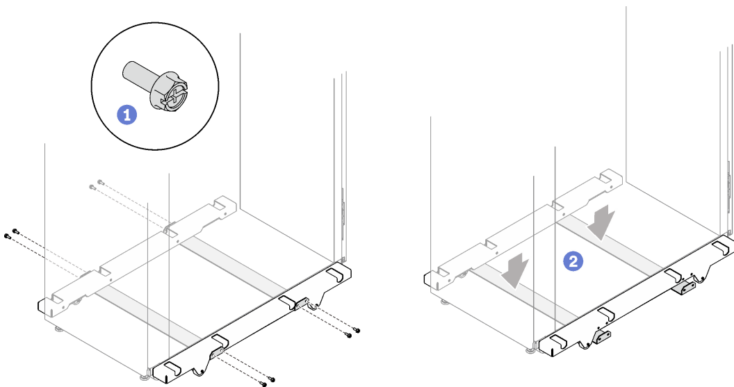
그림 172. 아웃리거 스테빌라이저 바 제거
