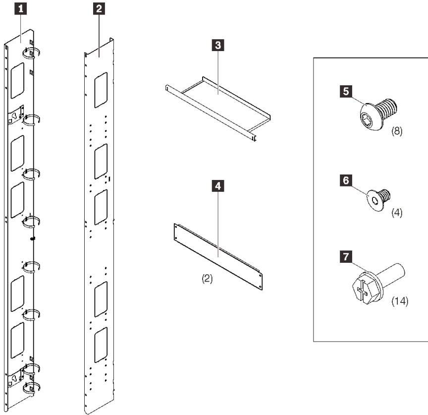
그림 6. 48U Standard Rack Extension Kit
