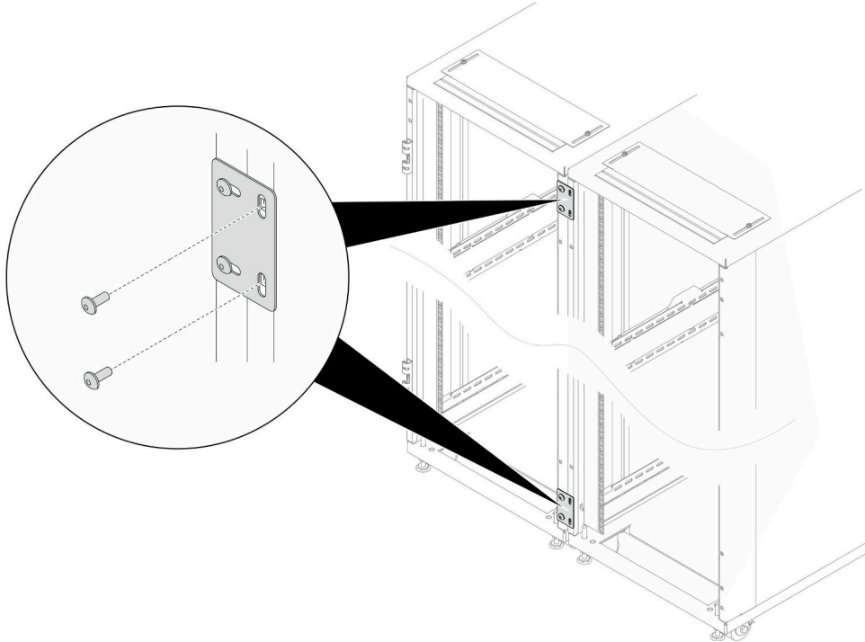
그림 47. 확장 설치 준비를 위해 나사 제거
