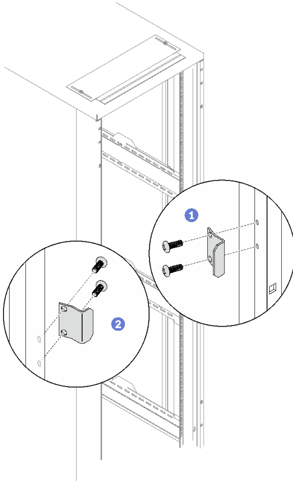
그림 119. 도어 래치 전환
