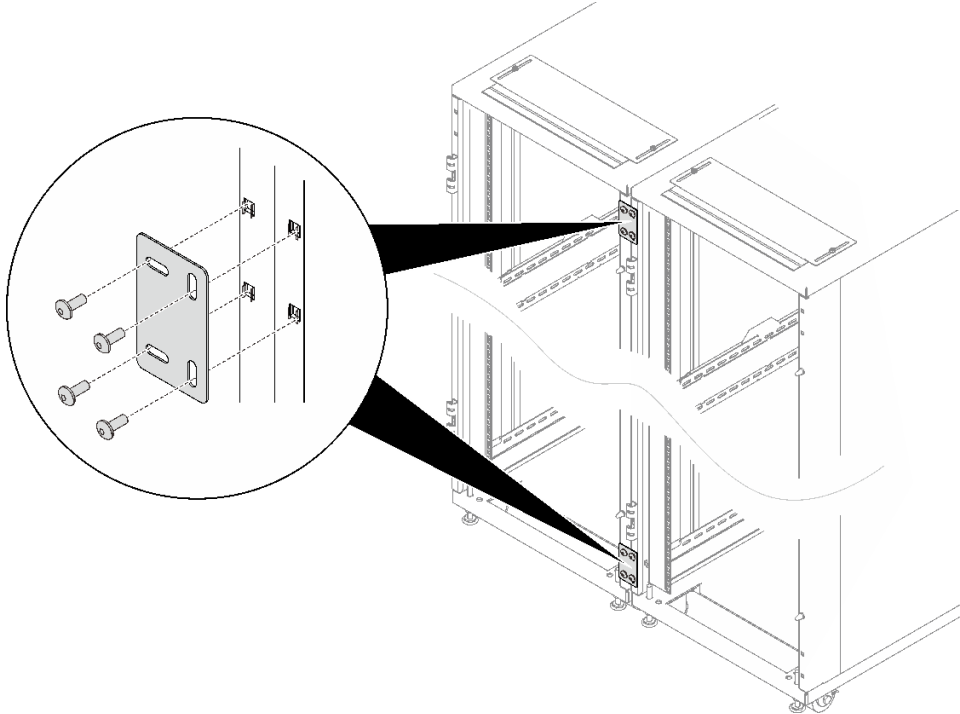
그림 46. 부착 브래킷 설치
