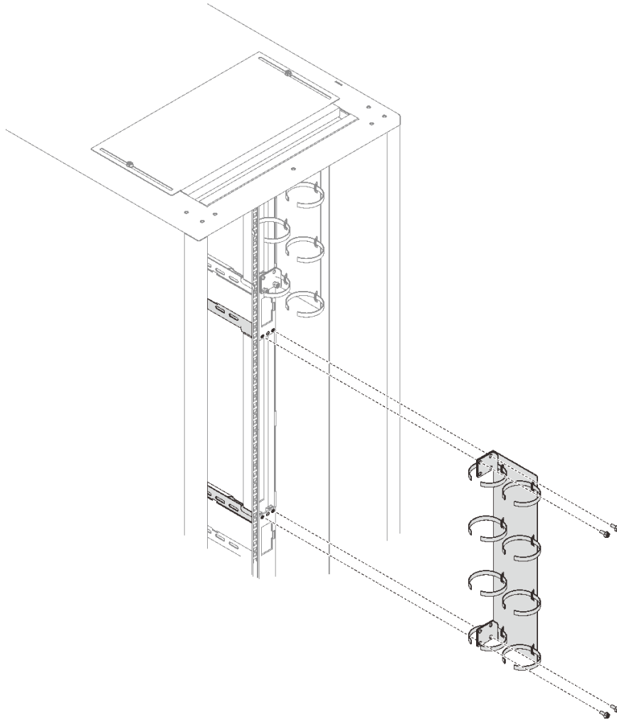
그림 180. 뒷면 케이블 관리 브래킷 제거
