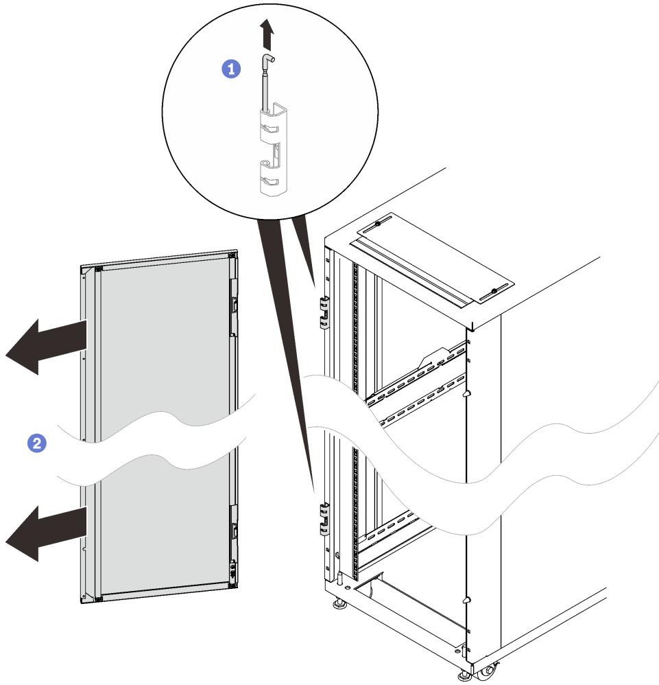
그림 43. 도어 제거
