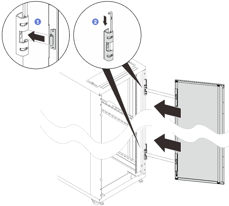
그림 116. 도어 설치
