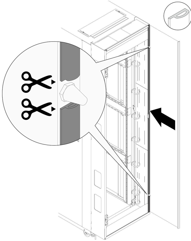
그림 56. 랙 오른쪽에 확장 실링 폼 설치
