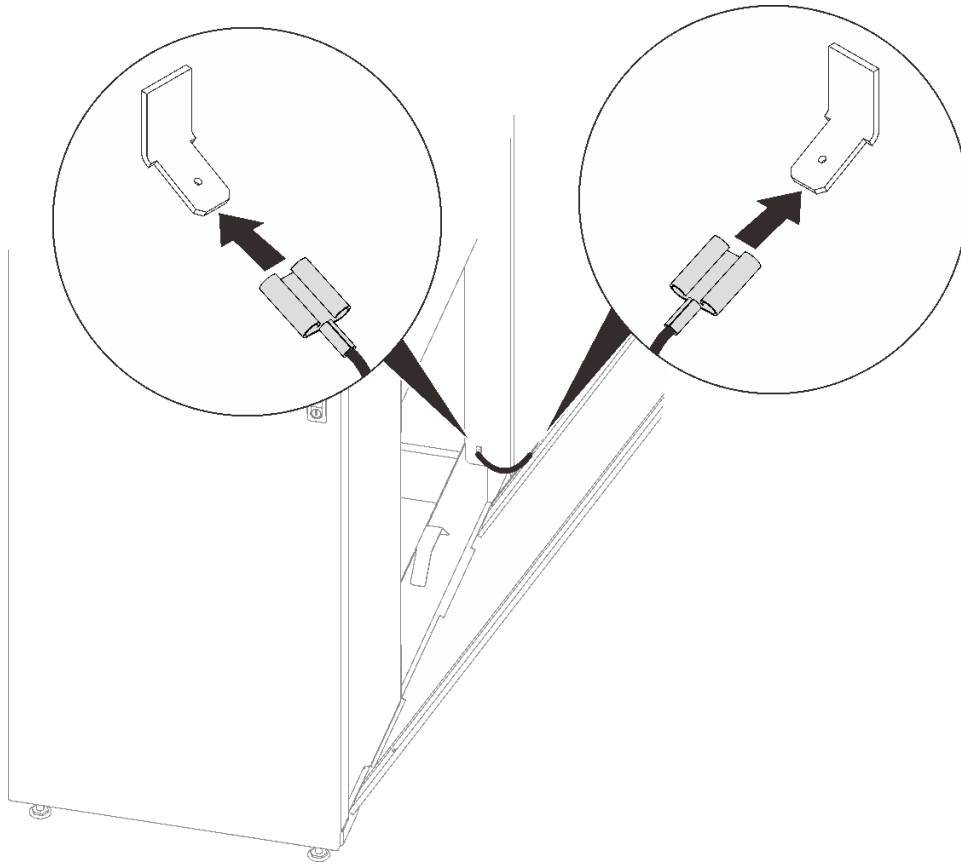
그림 63. 접지 점퍼 와이어 설치
