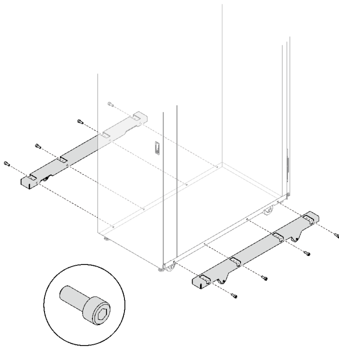
그림 175. 아웃리거 설치
