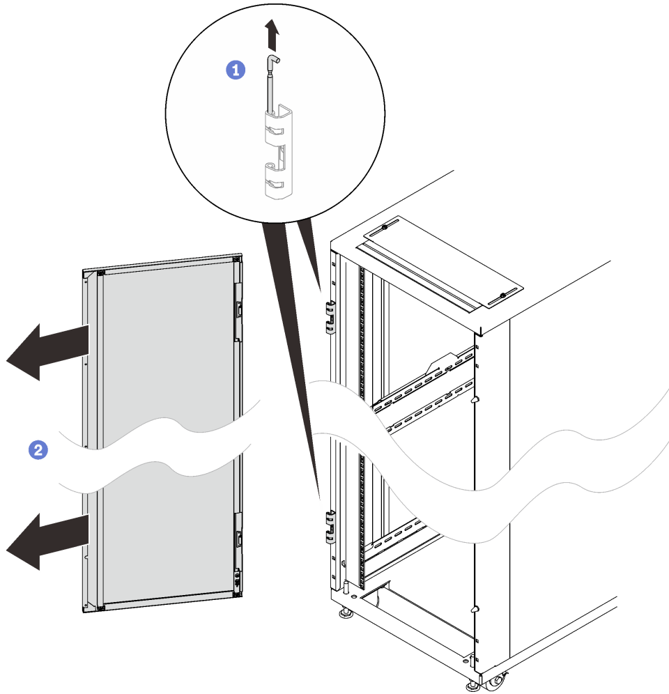
그림 117. 도어 제거
