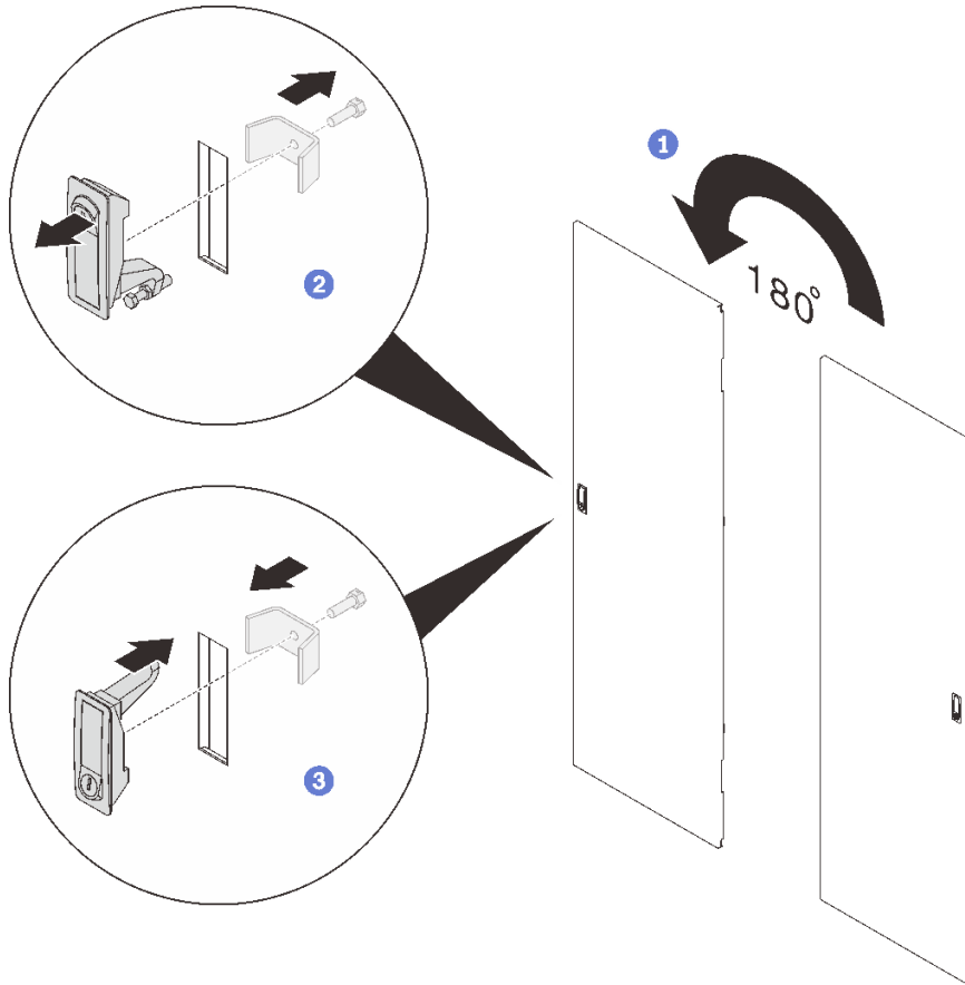
그림 122. 도어 핸들 전환
