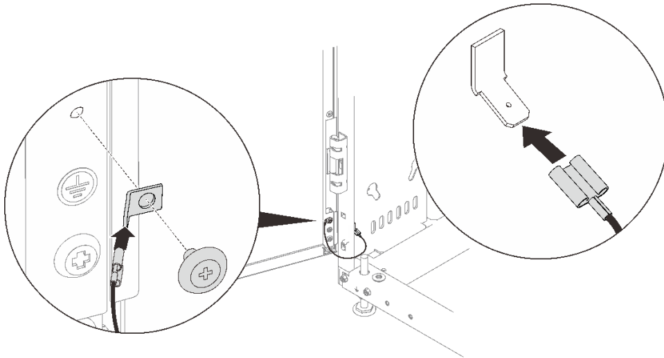
그림 61. 랙 접지 키트 설치
