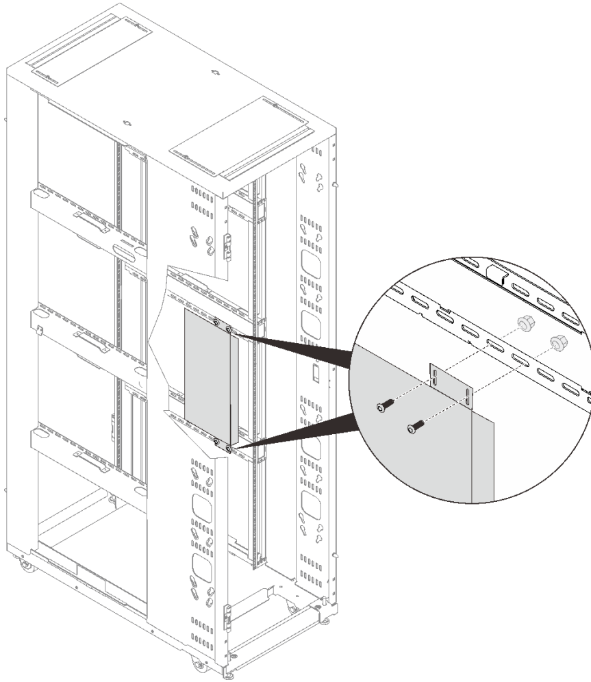
그림 168. 랙 측면에서 1U 장치 제거
