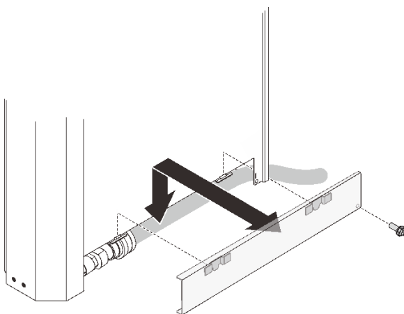
그림 125. 외부 호스 접근 패널 제거
