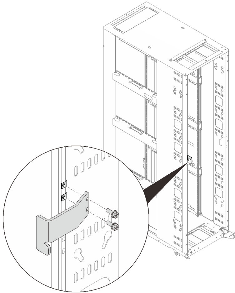
그림 78. 래치 플레이트 설치
