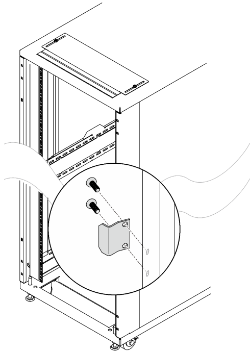
그림 162. 도어 래치 설치
