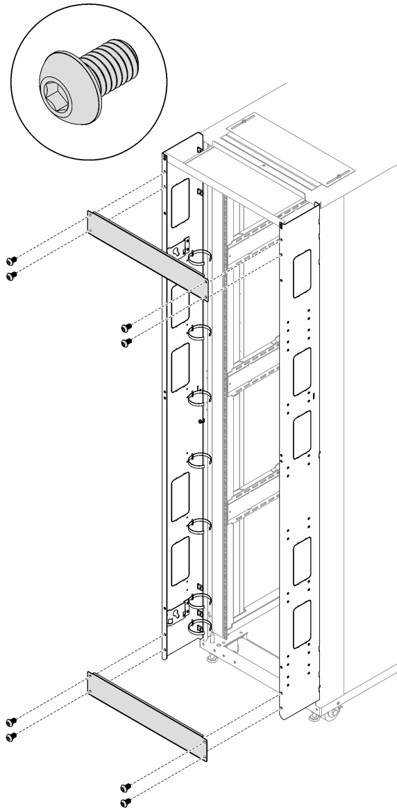
그림 159. 지지 브래킷 제거
