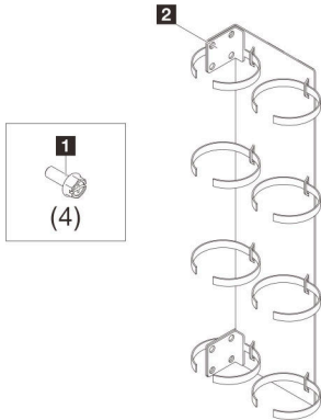
그림 10. 뒷면 케이블 관리 브래킷 구성 요소
