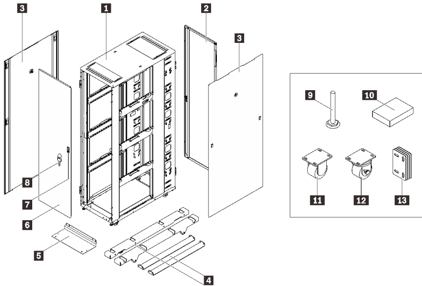
그림 2. 부품 목록
