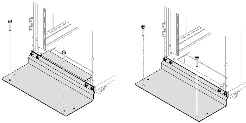
그림 28. 바닥에 스테빌라이저 고정
