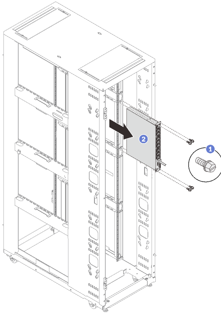
그림 170. 1U PDU 또는 콘솔 스위치 제거
