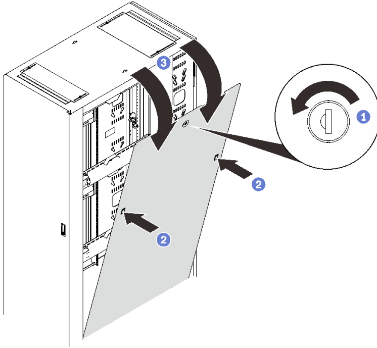
그림 44. 측면 덮개 제거
