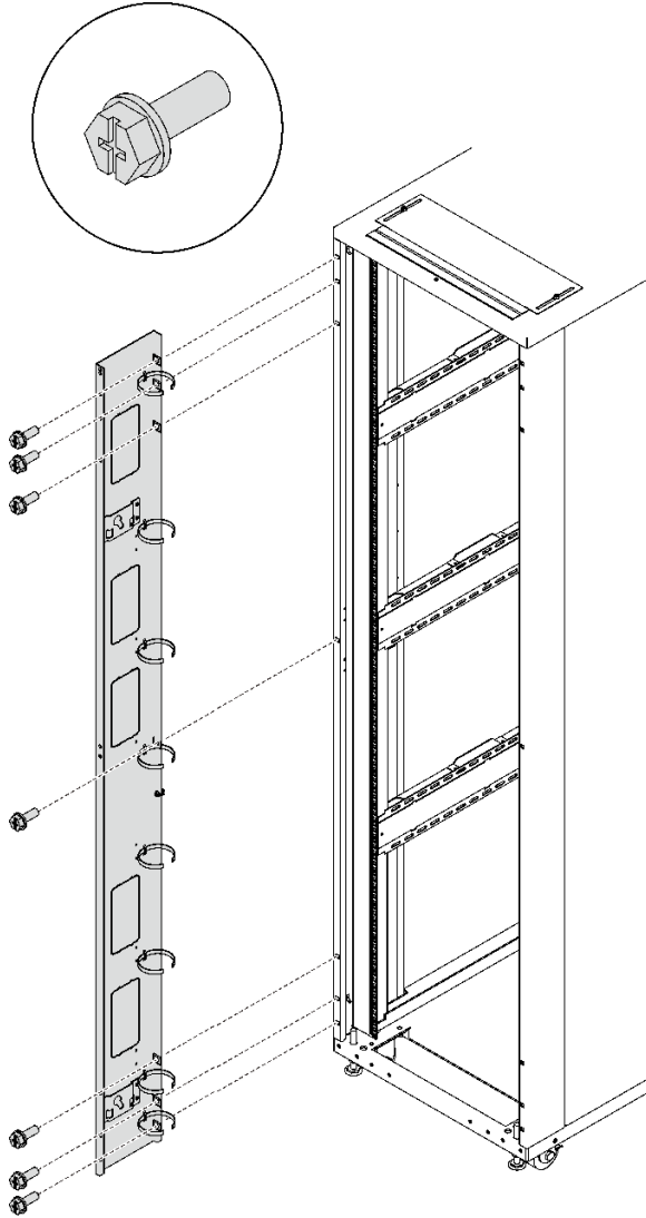
그림 161. 확장 패널 제거
