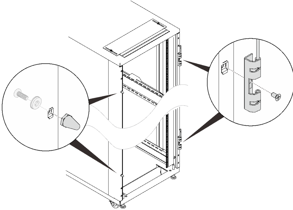
그림 72. 도어 힌지 및 도어스토퍼 제거
