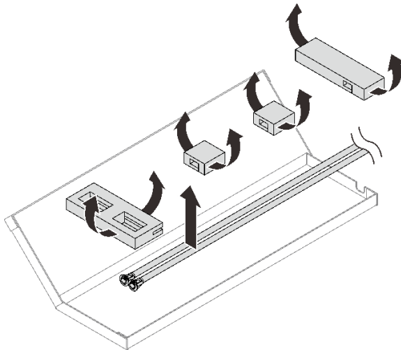
그림 69. 매니폴드 포장 개봉
