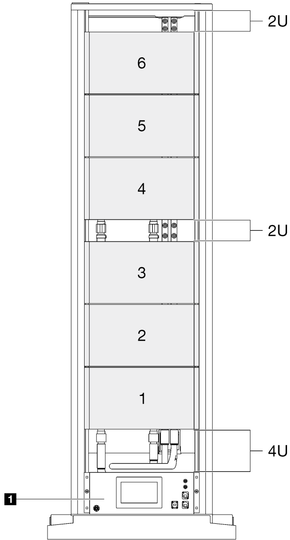
그림 4. 인렛 냉각수 분배 레이아웃 - 앞면
