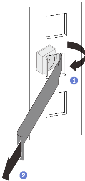
그림 60. 케이지 너트 설치
