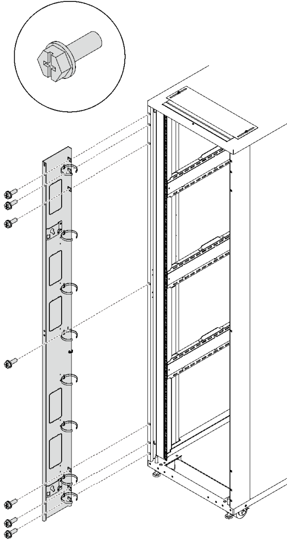
그림 34. 확장 패널 설치
