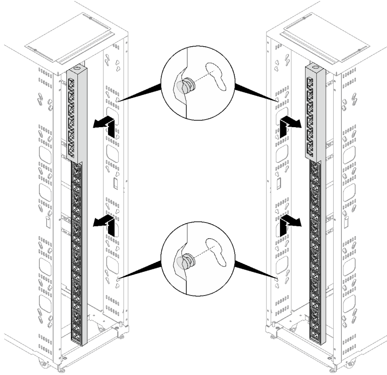
그림 166. 0U PDU 제거
