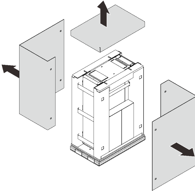
그림 18. 판지 제거
