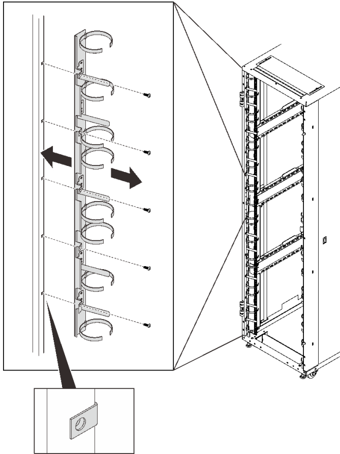
그림 178. 21U 앞면 케이블 관리 브래킷 제거
