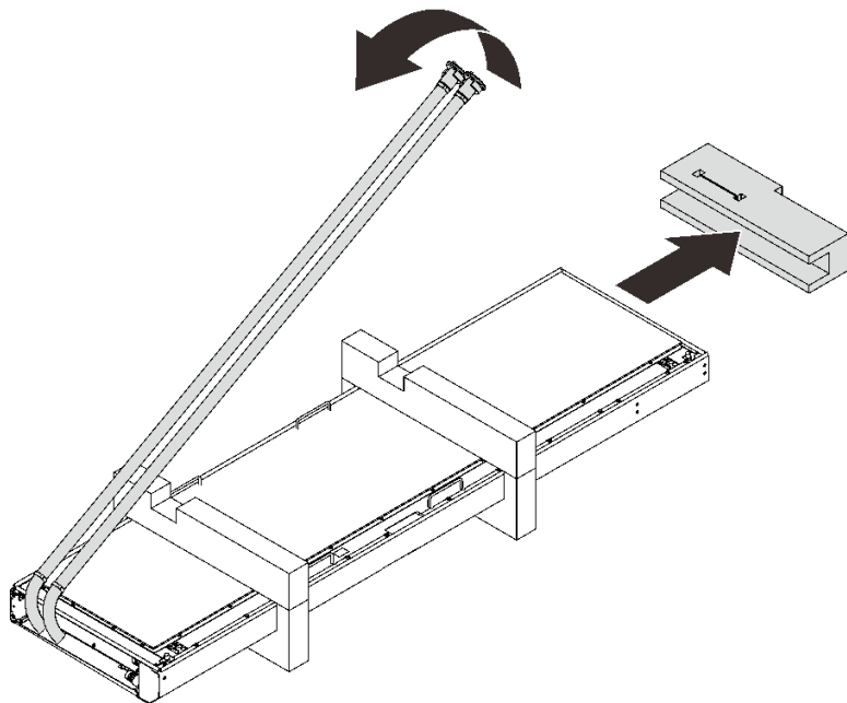
그림 140. 고정재 제거
