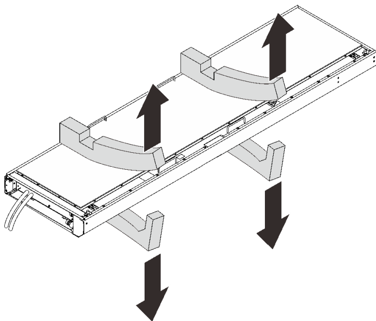
그림 141. 포장재 제거
