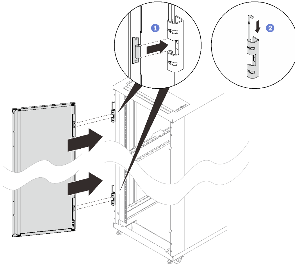
그림 164. 도어 설치
