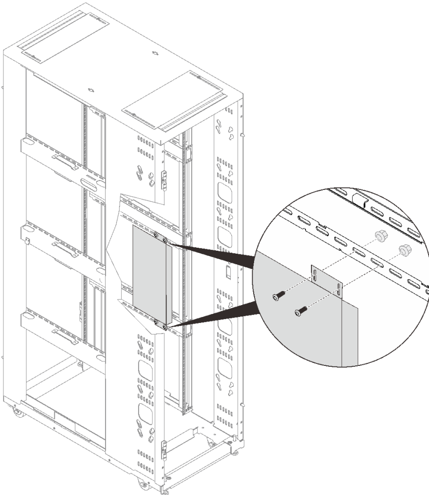
그림 167. 랙 측면에 1U 장치 설치
