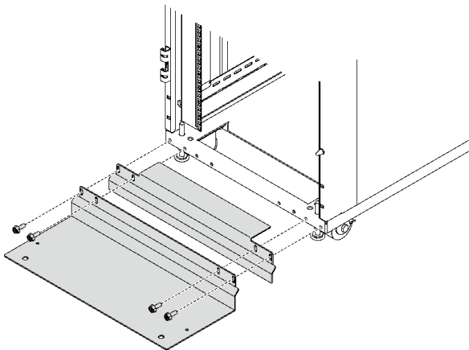
그림 27. 앞면 스테빌라이저 및 재순환 방지 플레이트 설치
