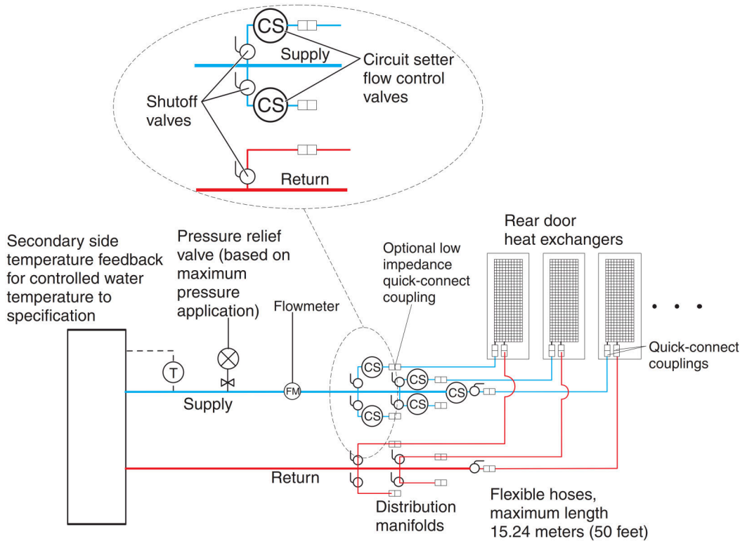
그림 90. 규격형 공급업체 솔루션을 사용하는 냉각수 분배 장치
