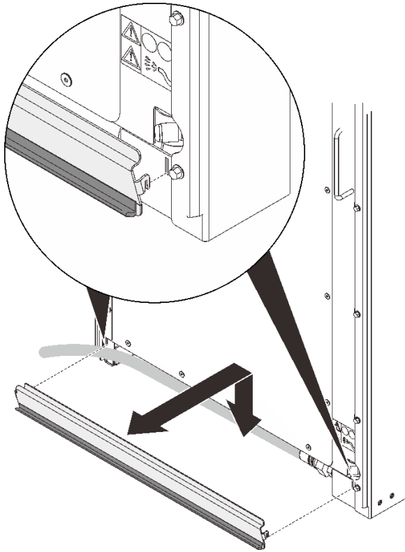
그림 124. 내부 호스 접근 패널 제거
