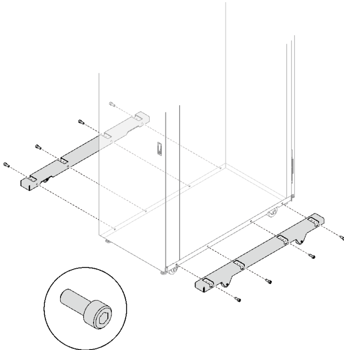
그림 42. 아웃리거 제거
