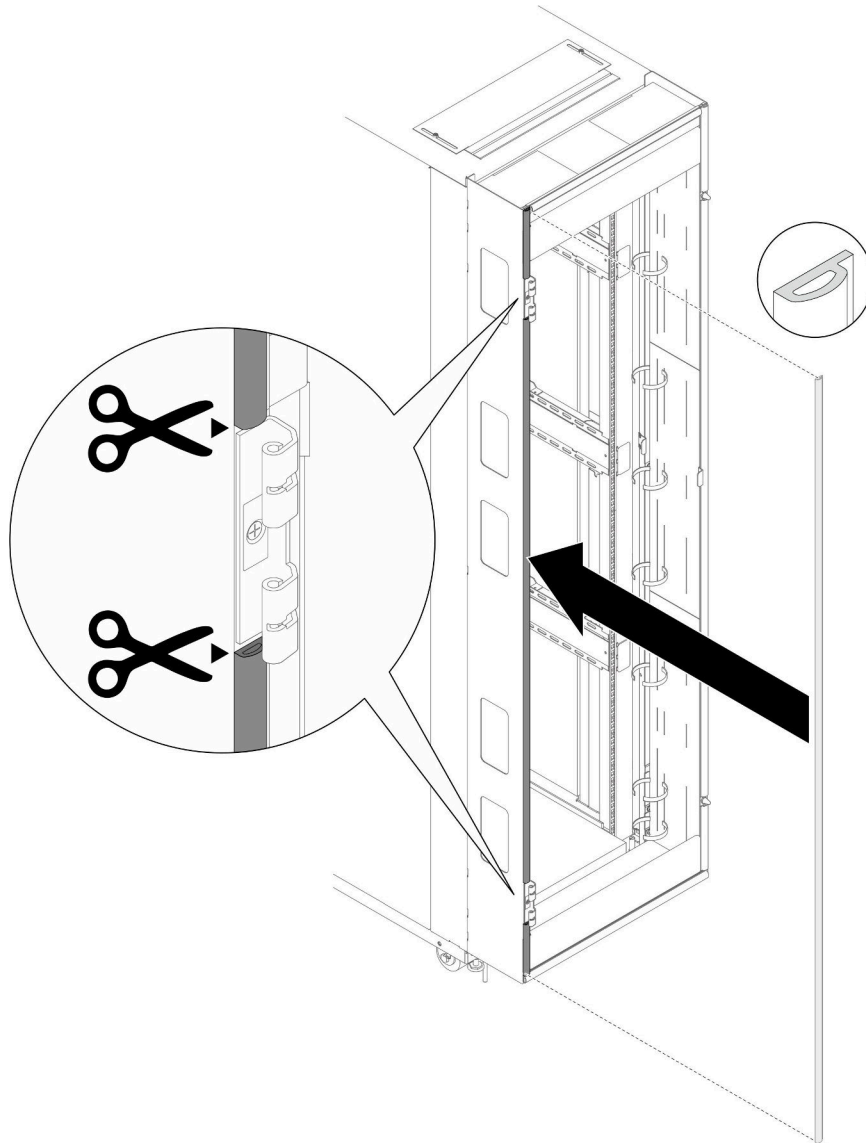
그림 55. 랙 왼쪽에 확장 실링 폼 설치
