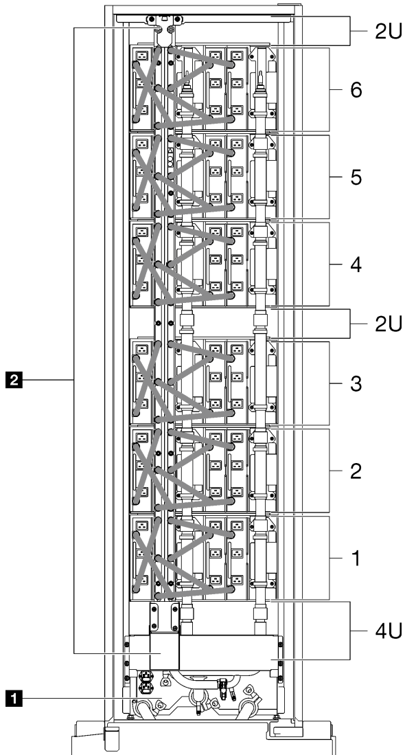
그림 5. 인력 냉각수 분배 레이아웃 - 뒷면
