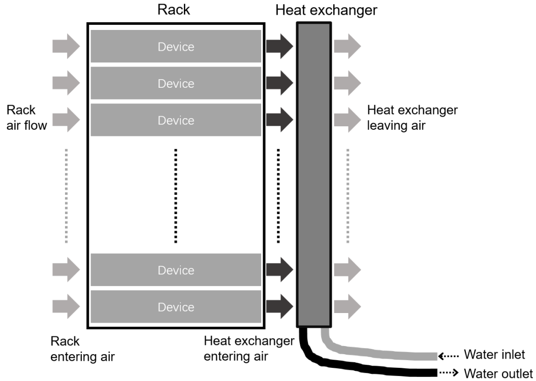
그림 12. 랙 공기 흐름 및 열교환기 물 흐름 도해
