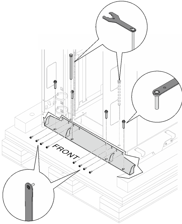
그림 21. 앞면 운송 브래킷 제거
