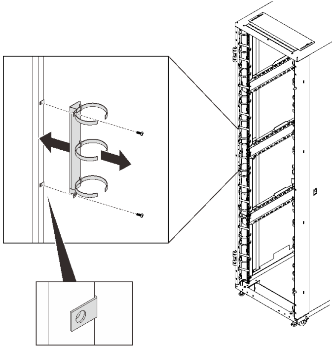
그림 182. 6U 앞면 케이블 관리 브래킷 설치
