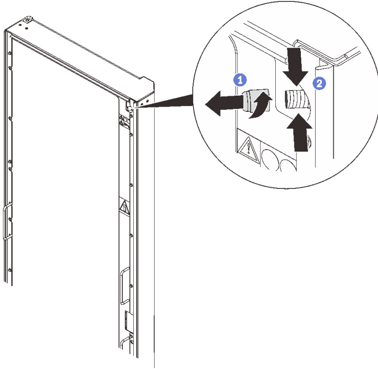
그림 145. 질소 퍼지
