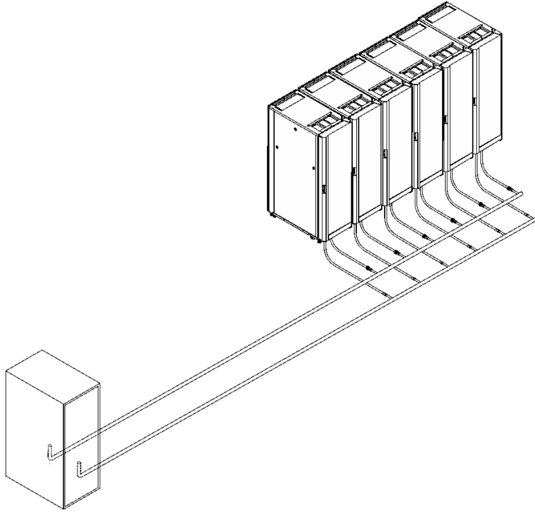
그림 92. 일반적인 확장 매니폴드(랙 사이 통로를 따라)
