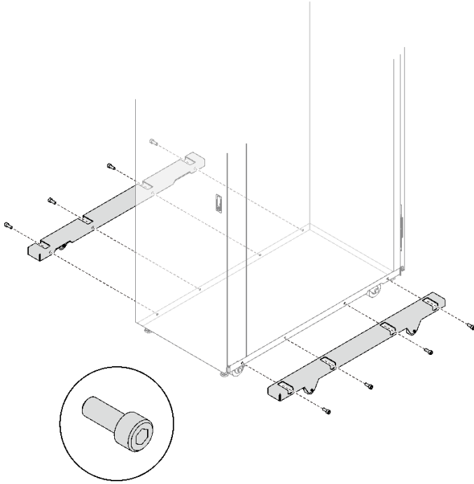
그림 173. 아웃리거 제거
