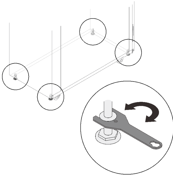
그림 174. 수평 조절 패드 내리기
