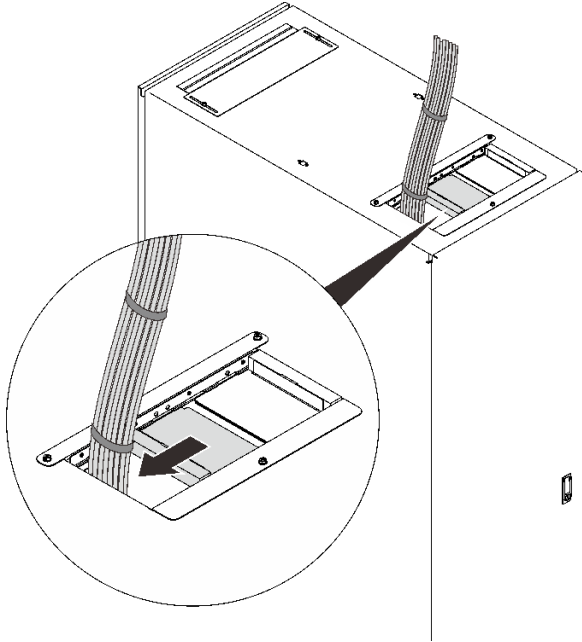
그림 107. 상부 공기 조절 장치로 케이블 관리
