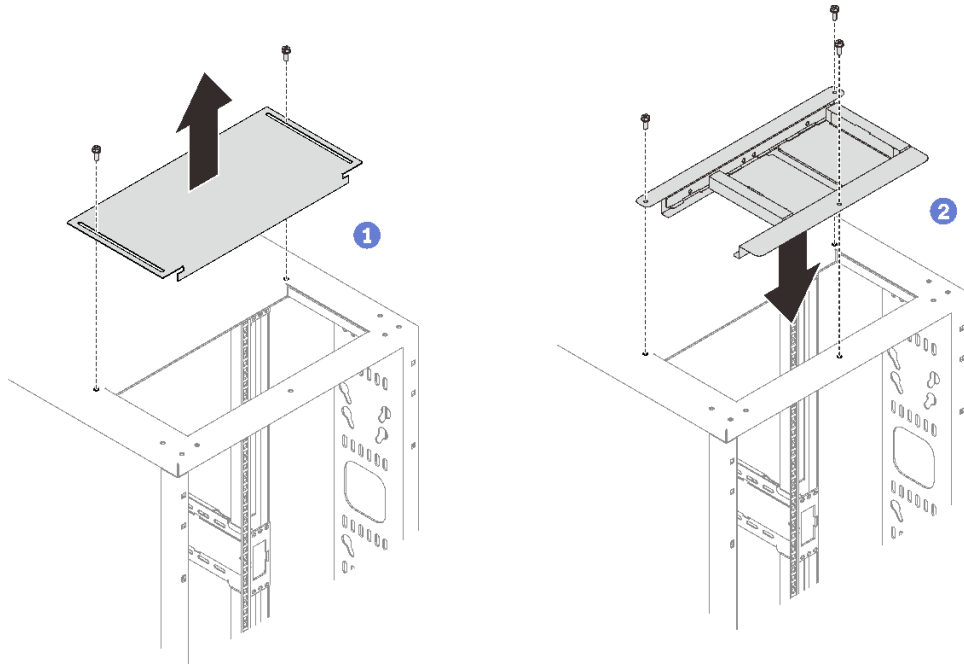
그림 74. 상부 공기 조절 장치 설치
