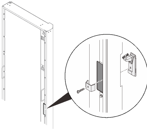
그림 150. 도어 래치 교체
