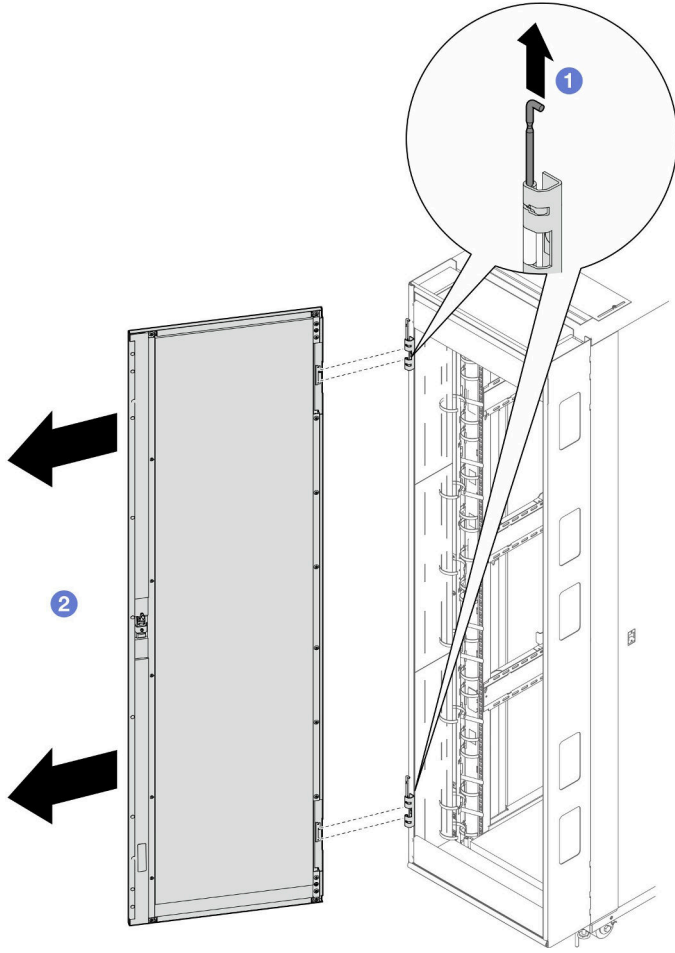
그림 54. 도어 제거
