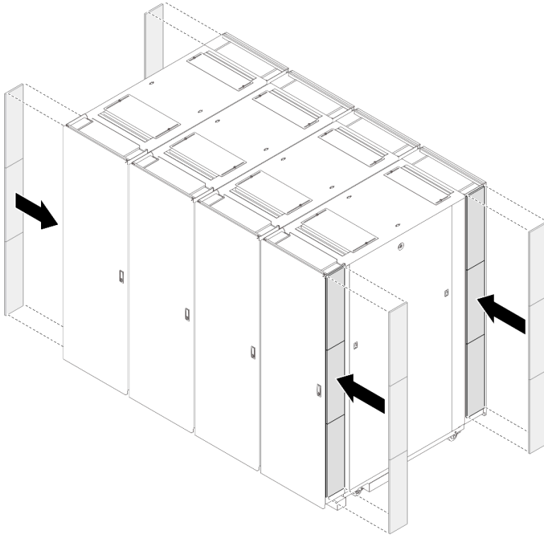
그림 53. 확장 품 설치
