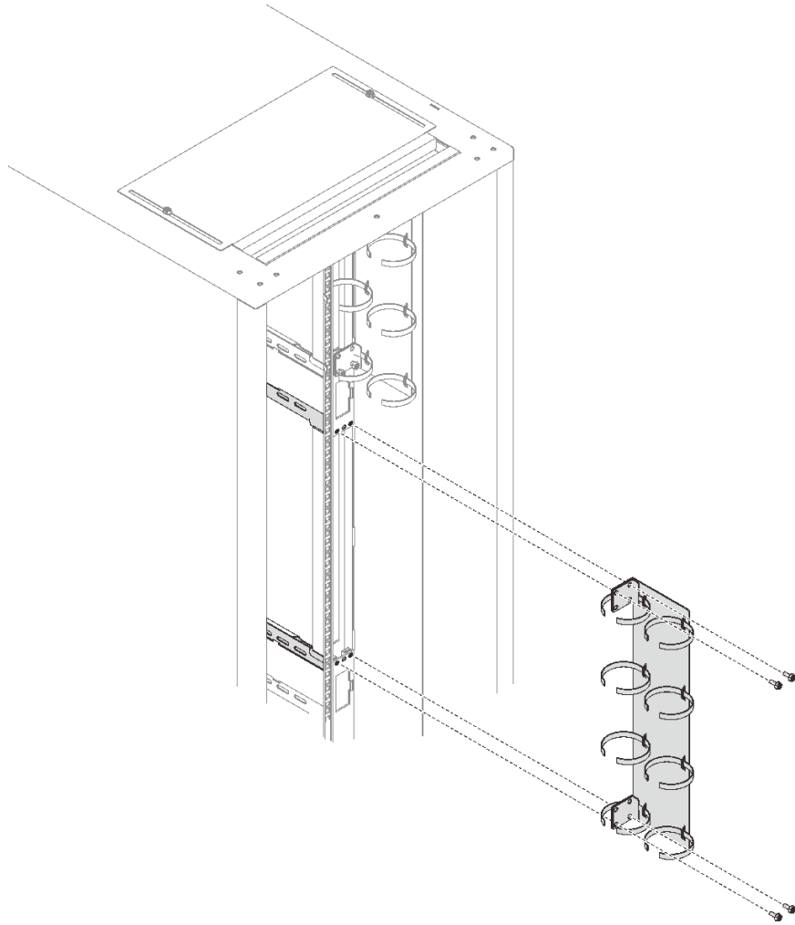
그림 183. 뒷면 케이블 관리 브래킷 설치
