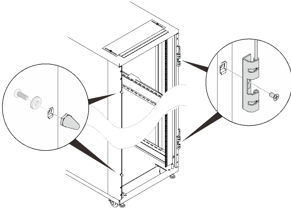
그림 121. 힌지 및 도어스토퍼 설치
