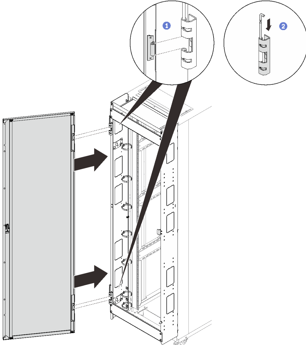
그림 157. 도어 설치
