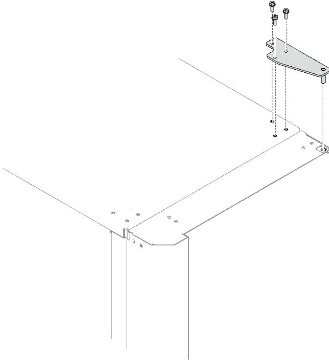
그림 134. 상단 힌지 제거
