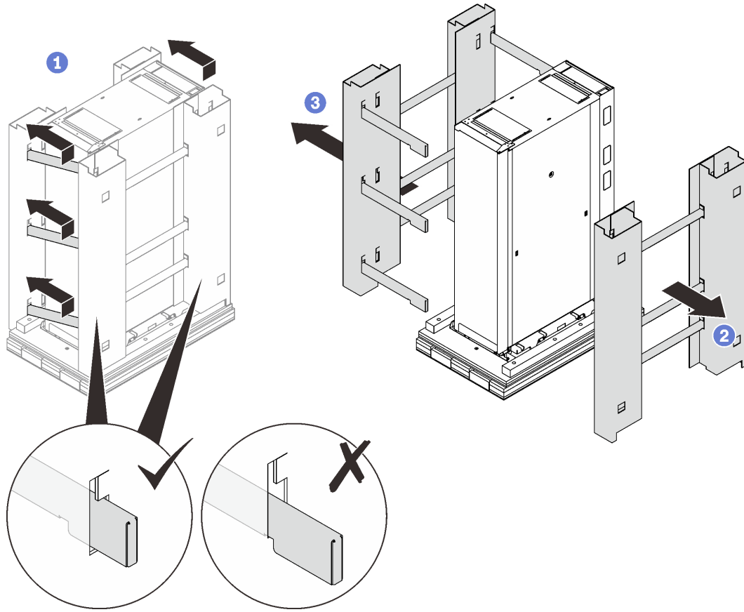
그림 20. 측면 프레임 제거
