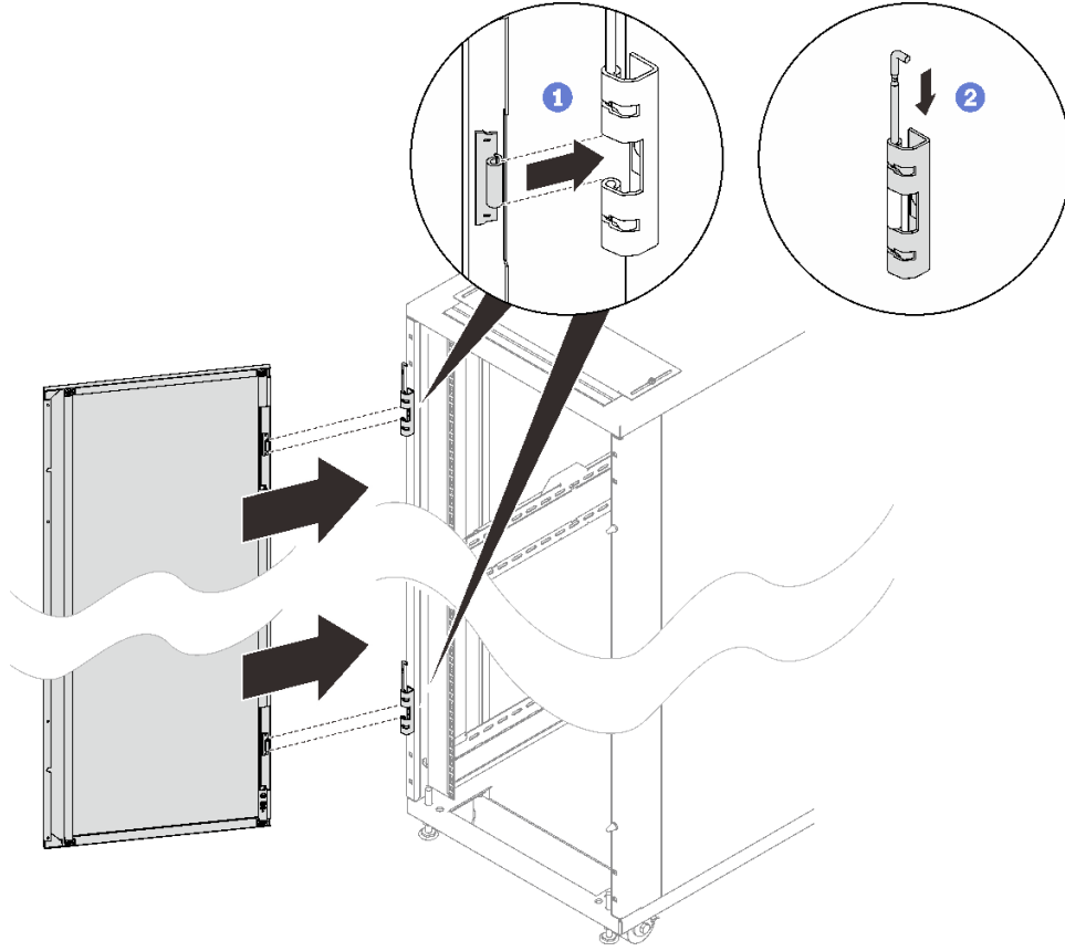
그림 48. 도어 설치
