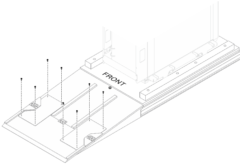
그림 24. 경사로에 플레이트 2개 고정
