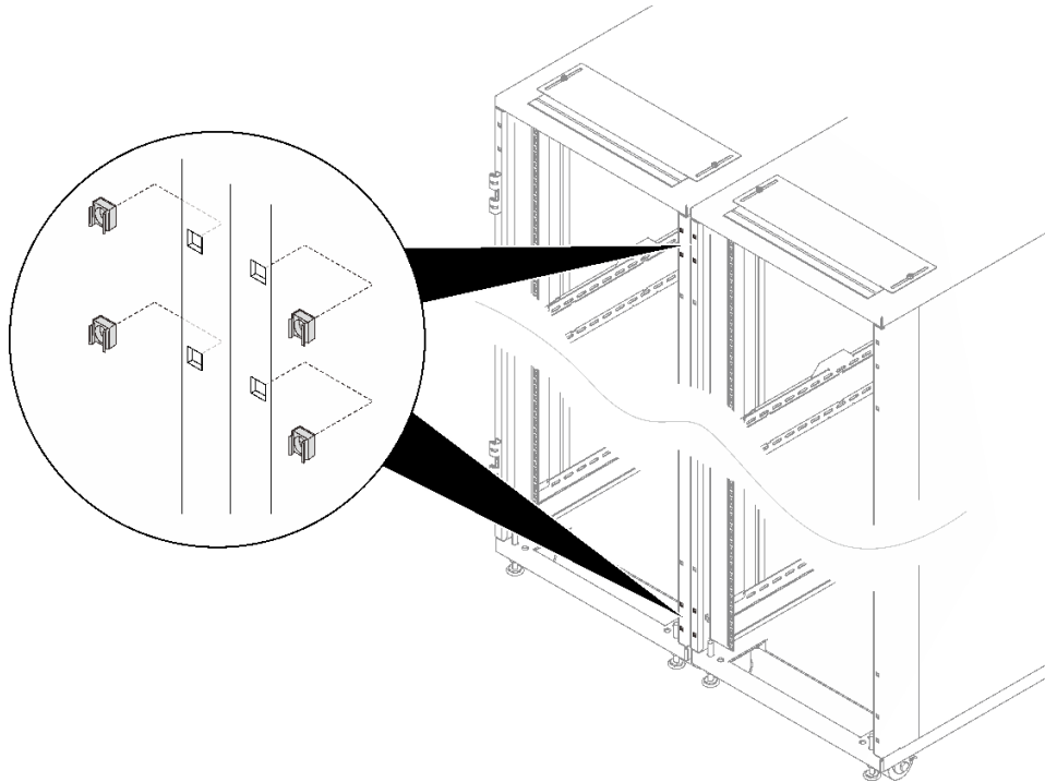
그림 45. 케이지 너트 설치
