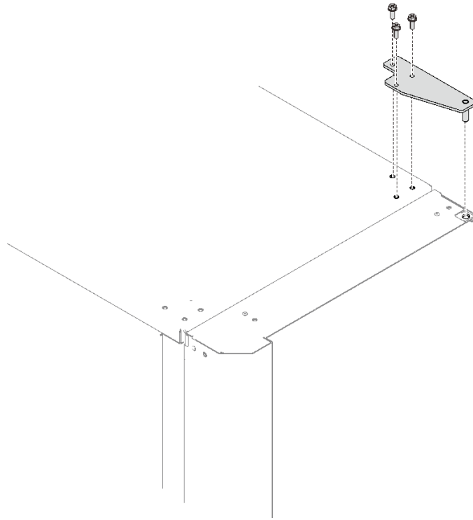
그림 144. 상단 힌지 설치
