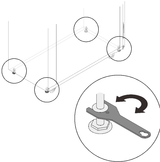
그림 177. 수평 조절 패드 줄이기
