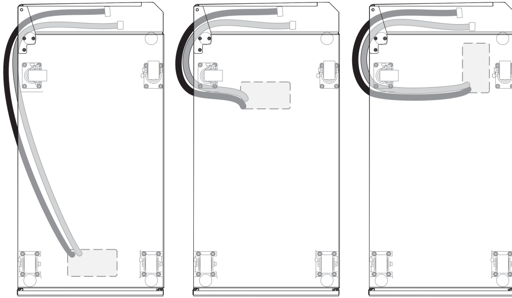
그림 109. 이중 바닥 환경에서 개별 랙의 호스 배선 및 고정(위에서 내려다본 모습)
