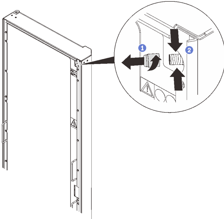
그림 93. 질소 퍼지
