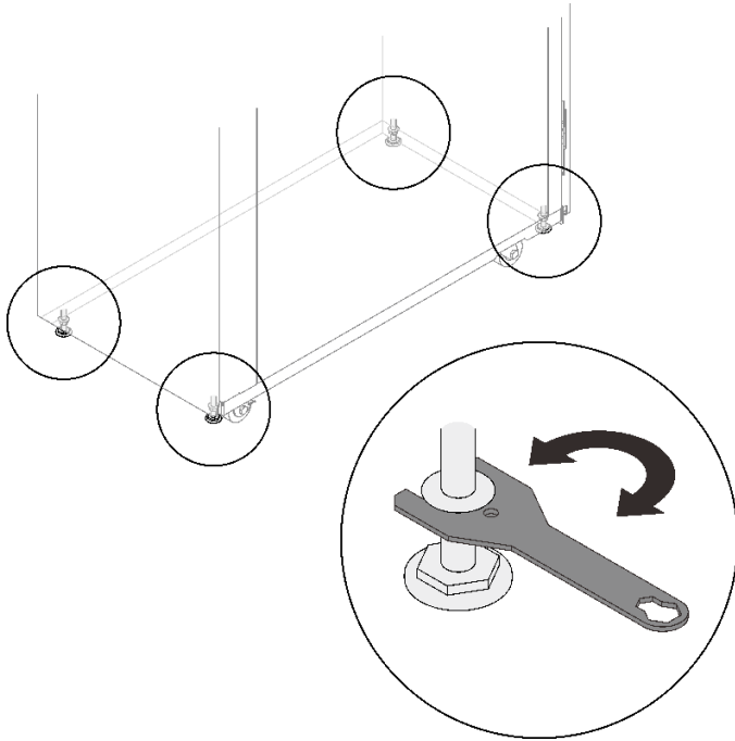
그림 171. 수평 조절 패드 내리기
