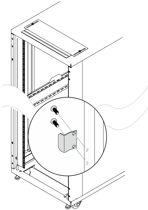
그림 33. 도어 래치 제거
