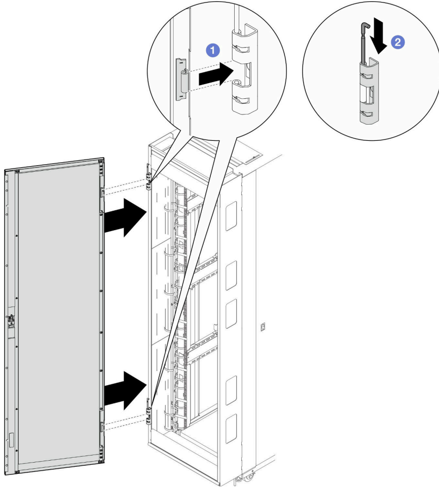
그림 58. 도어 설치
