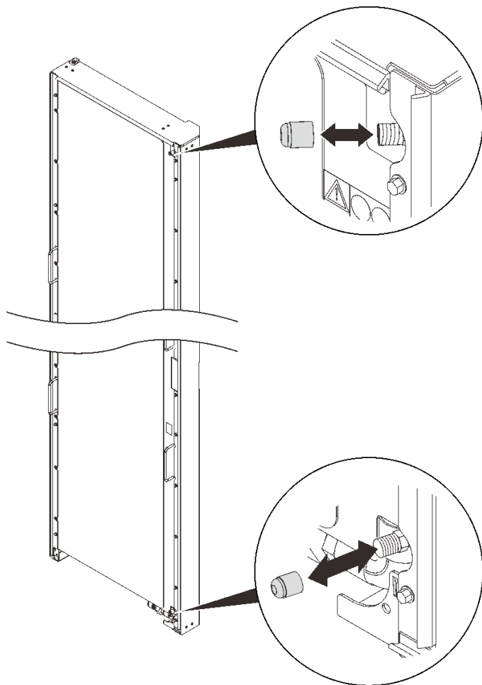
그림 133. 밸브 캡 설치
