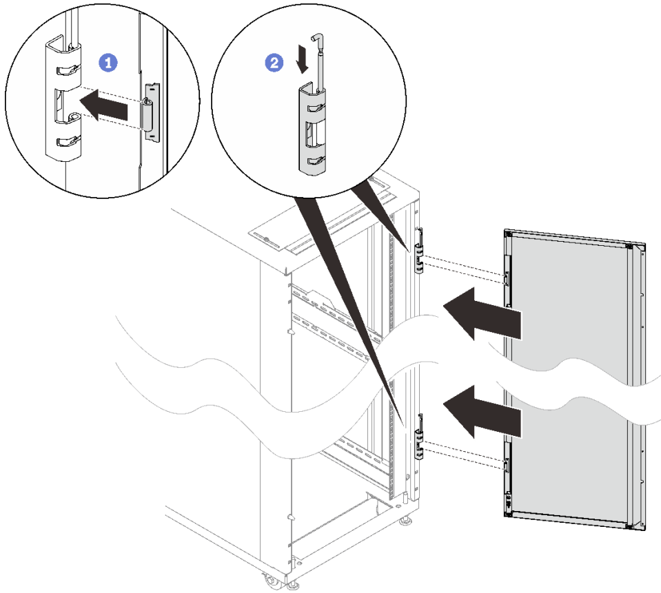
그림 123. 도어 설치
