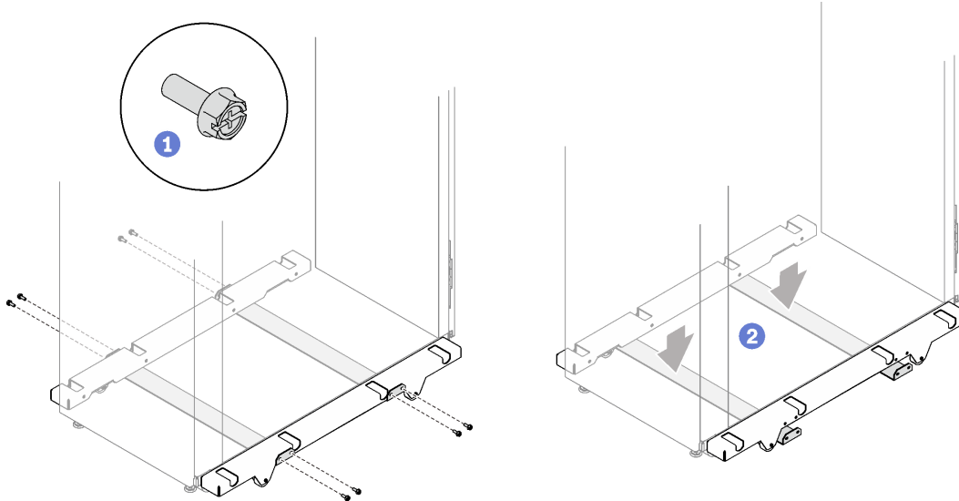
그림 41. 아웃리거 스테빌라이저 바 제거
