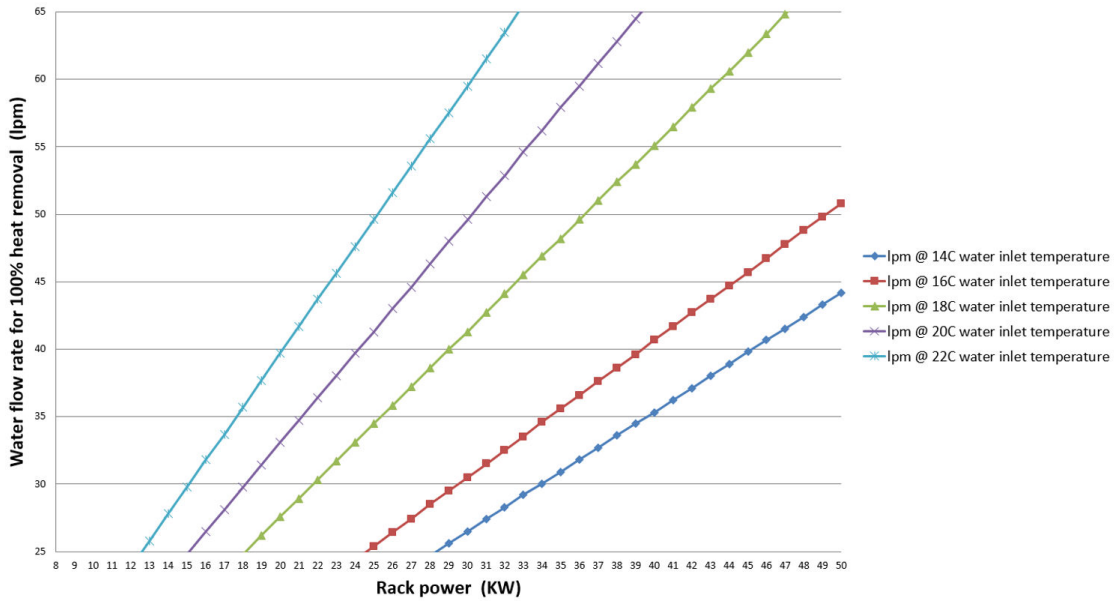
그림 13. 열교환기의 일반적인 성능, 3840SCFM 랙 공기 흐름, 25° C 랙 유입 온도
