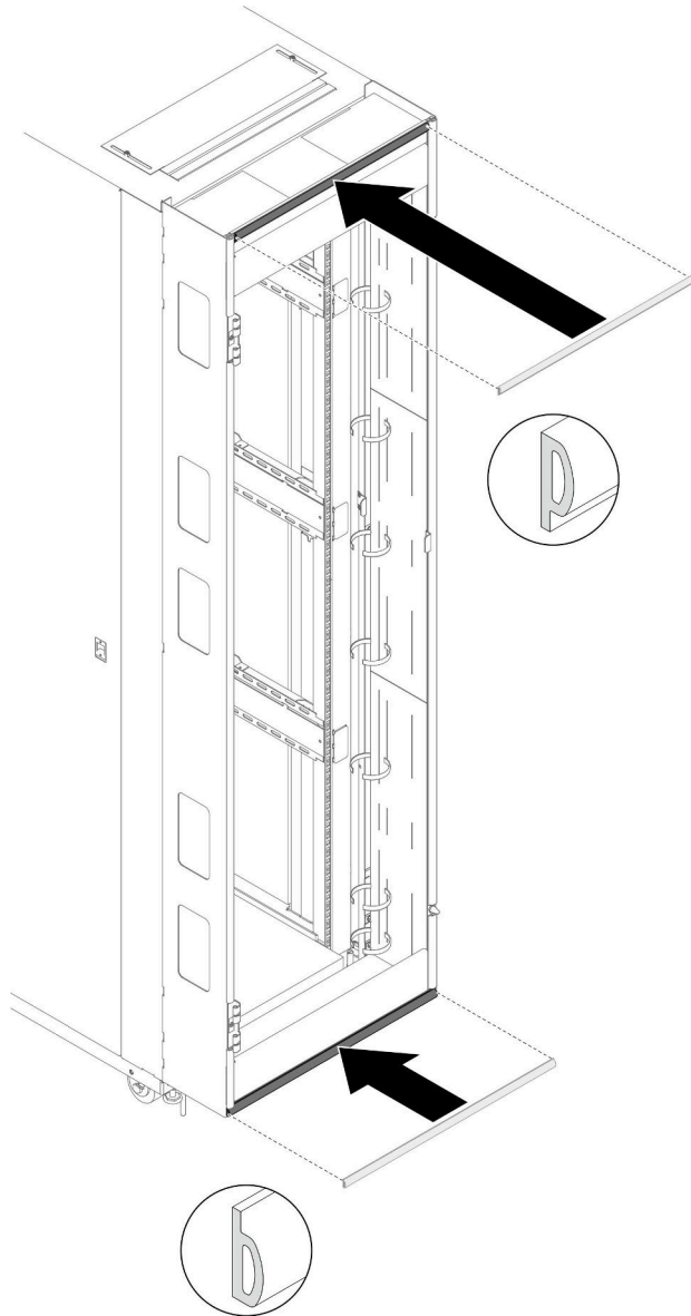
그림 57. 확장 윗면 덮개 및 밑면 덮개에 확장 실링 폼 설치
