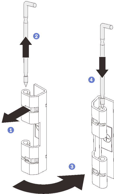
그림 120. 힌지 방향 전환
