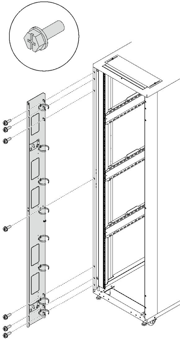
그림 152. 확장 패널 설치
