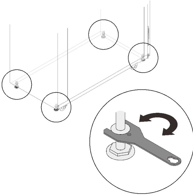
그림 70. 수평 조절 패드 내리기
