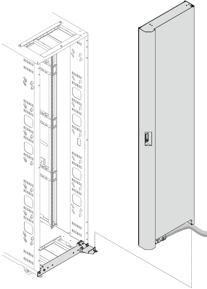
그림 143. 랙 캐비닛에 열교환기 설치
