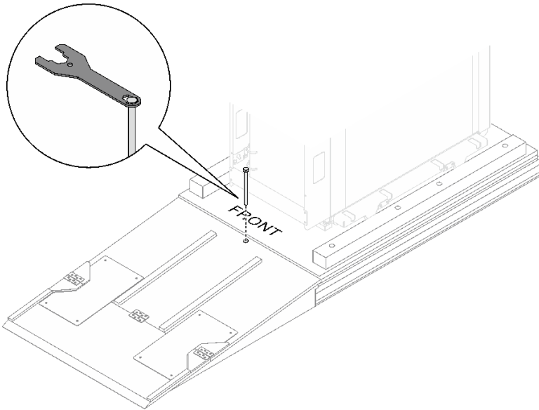
그림 25. 팔레트에 경사로 고정
