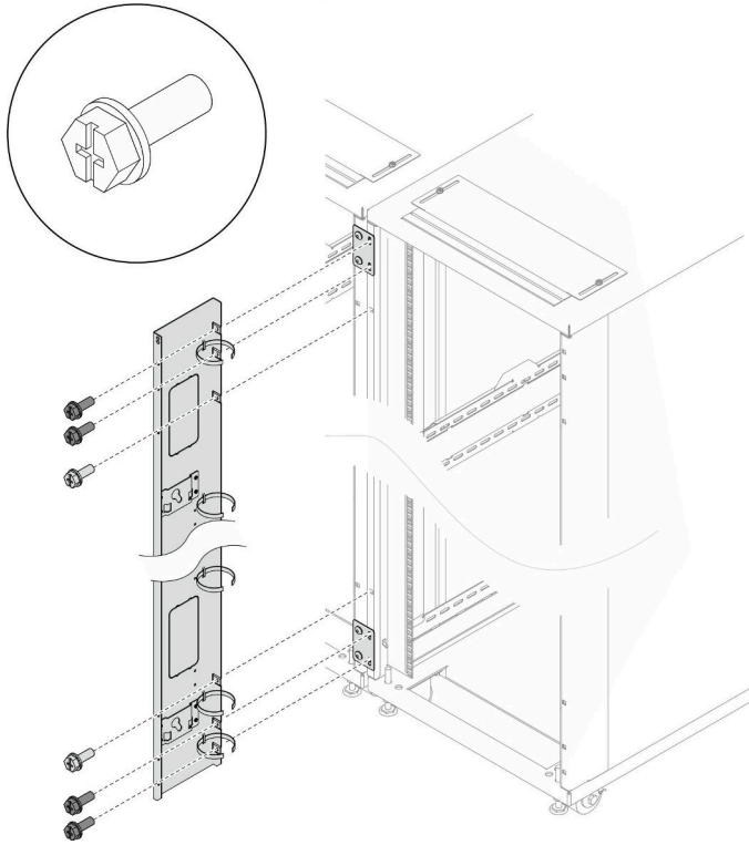
그림 153. 확장 패널 설치(베이 키트 포함)
