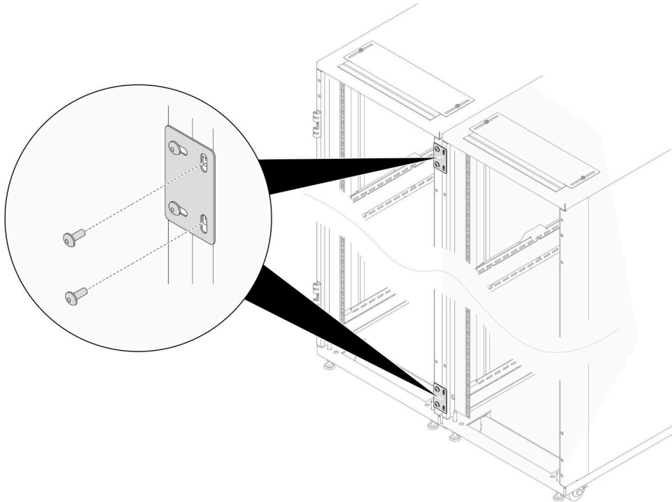
그림 30. 확장 설치 준비를 위해 나사 제거
