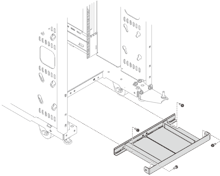
그림 76. 하부 공기 조절 장치 설치
