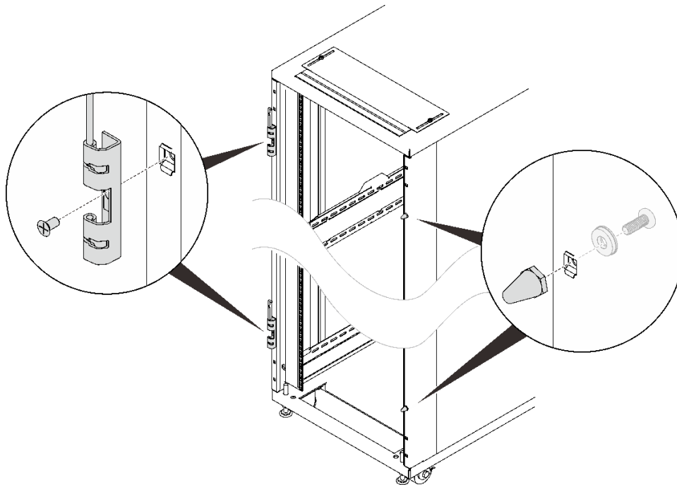
그림 163. 힌지 및 도어스토퍼 설치
