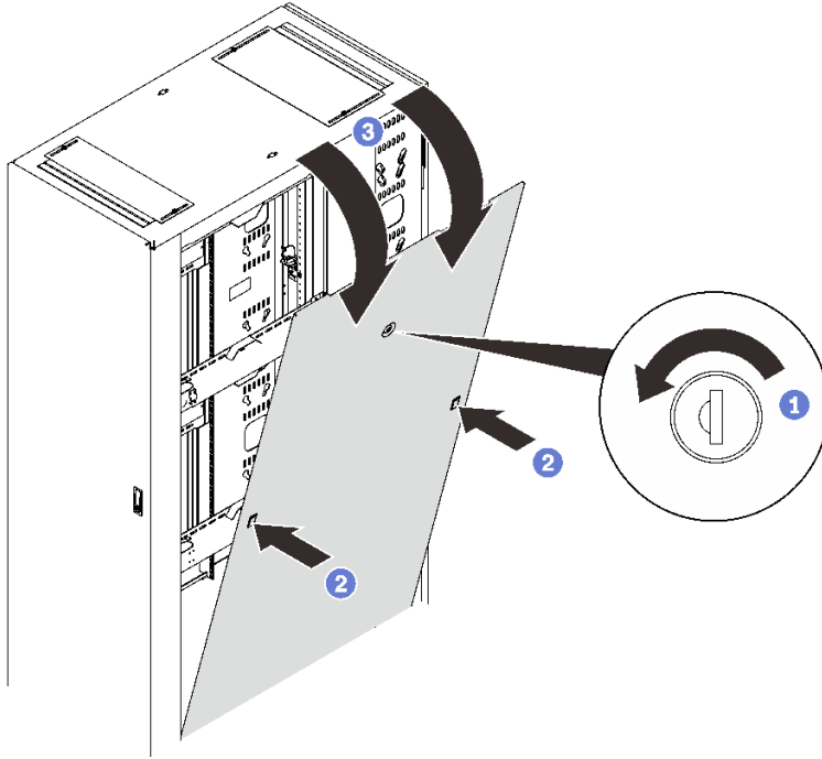
그림 62. 측면 덮개 제거
