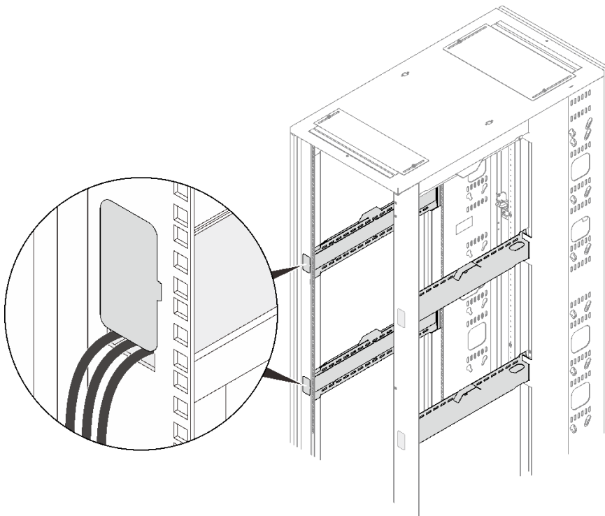
그림 101. 앞-뒤 케이블 채널
