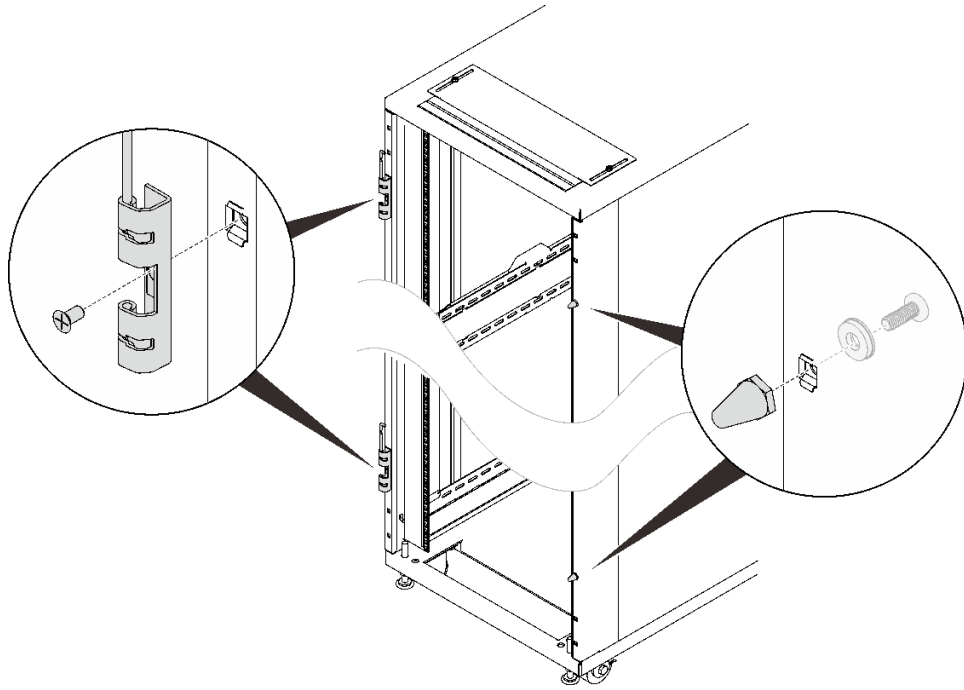
그림 118. 힌지 및 도어스토퍼 제거
