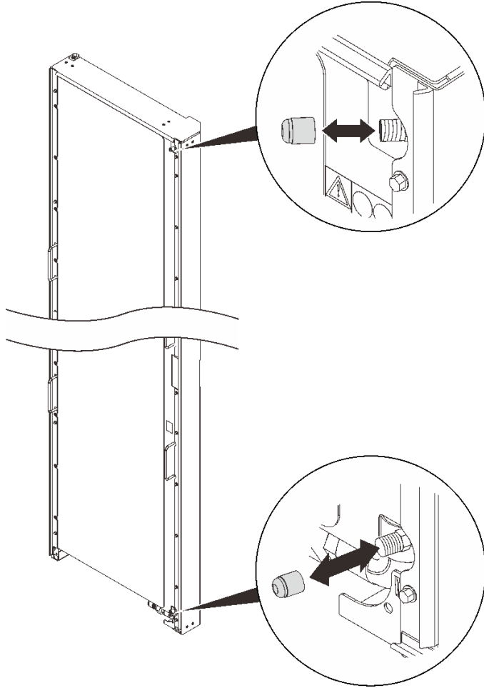
그림 127. 밸브 캡 제거
