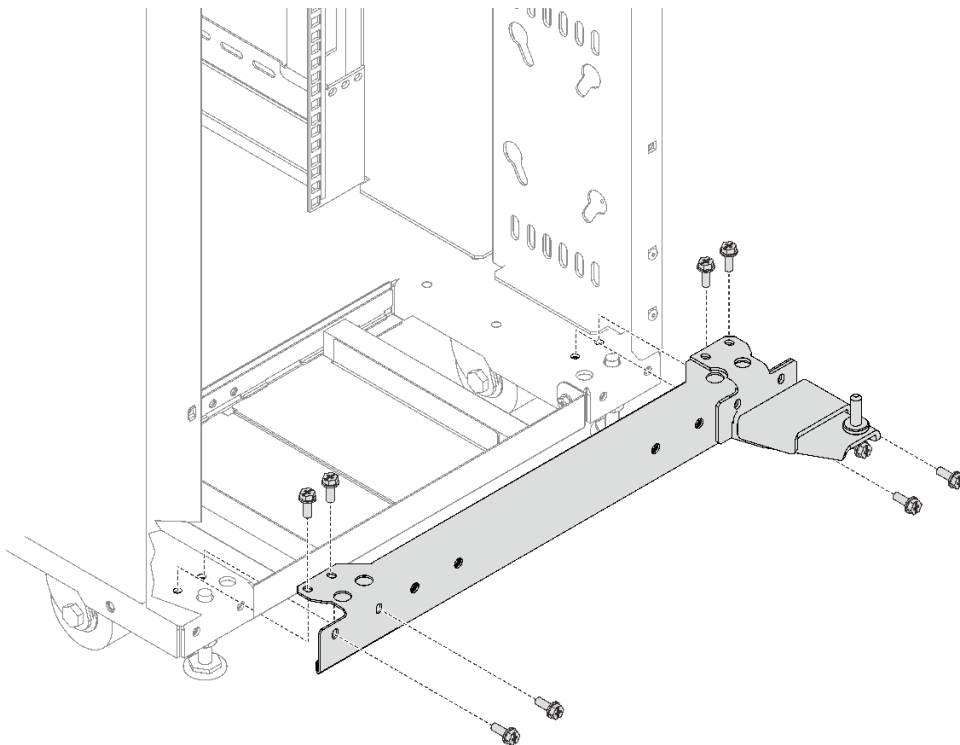
그림 77. 하단 힌지 어셈블리 설치
