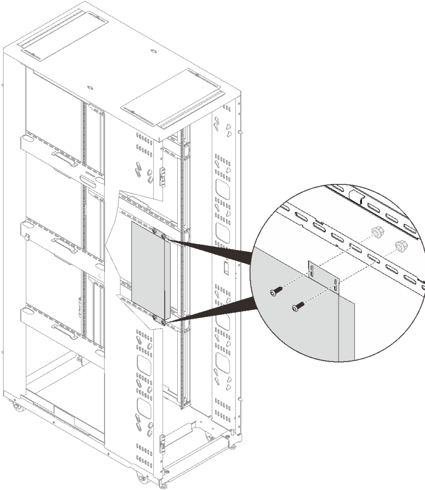
그림 99. 랙 측면에 1U 장치 설치
