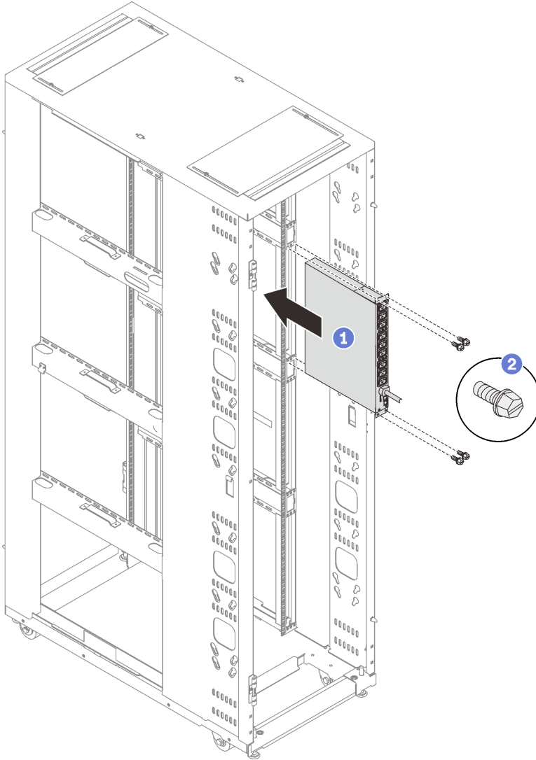
그림 169. 1U PDU 또는 콘솔 스위치 설치
