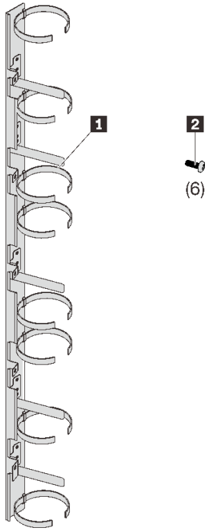
그림 8. 21U 앞면 케이블 관리 브래킷 구성 요소
