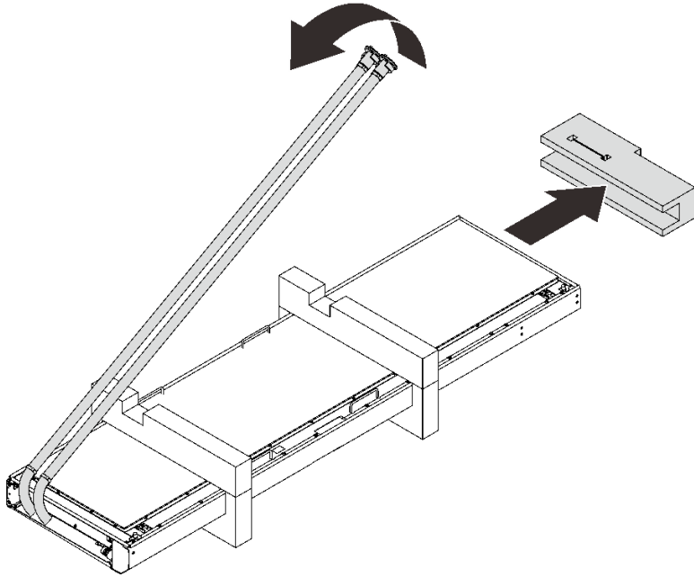
그림 82. 고정재 제거
