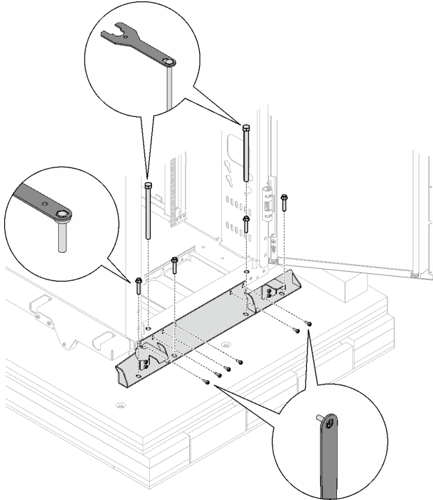
그림 22. 뒷면 운송 브래킷 제거
