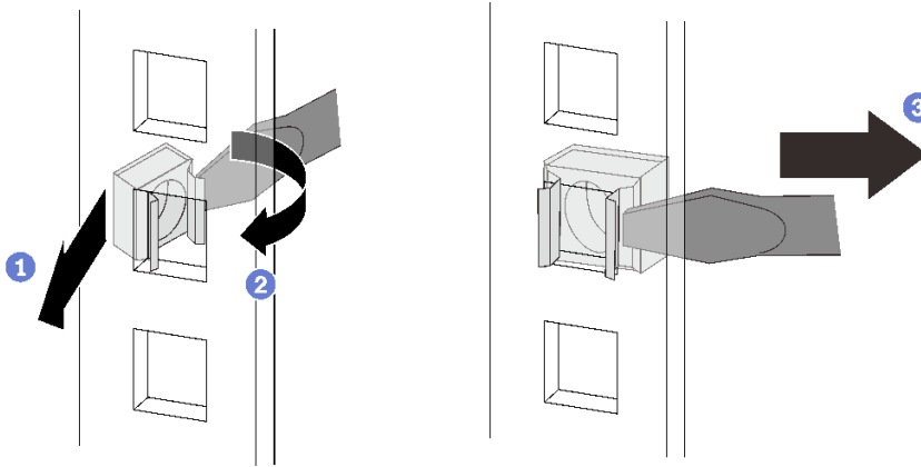
그림 59. 케이지 너트 설치
