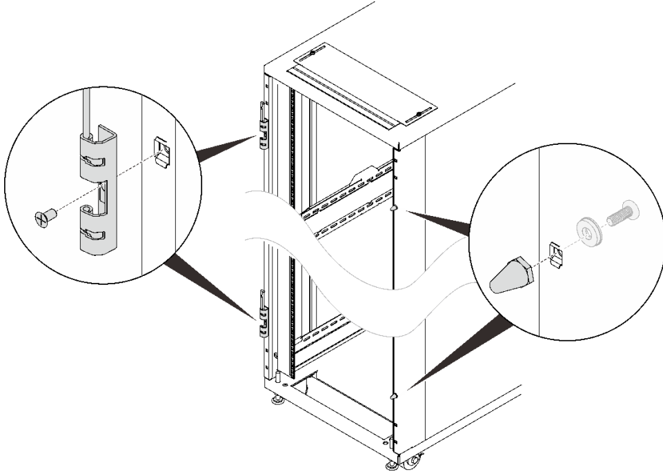
그림 32. 도어 힌지 및 도어스토퍼 제거
