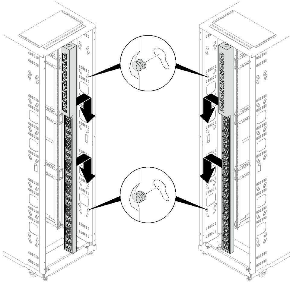
그림 165. 0U PDU 설치
