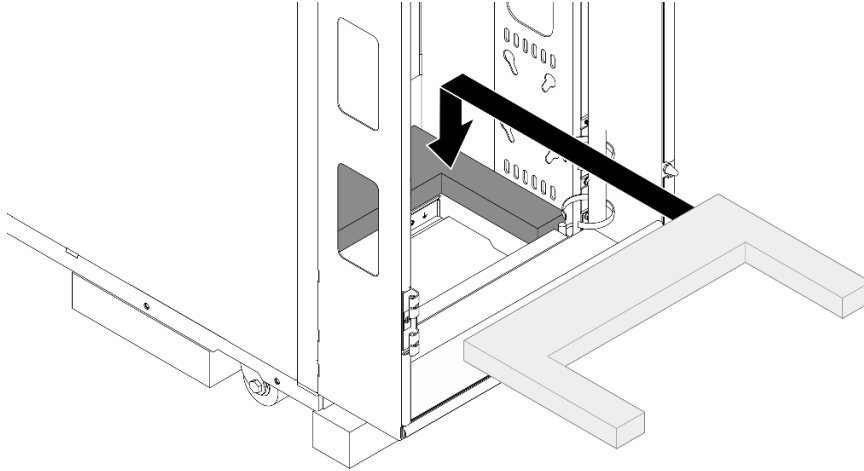
그림 50. 뒷면 폼 설치
