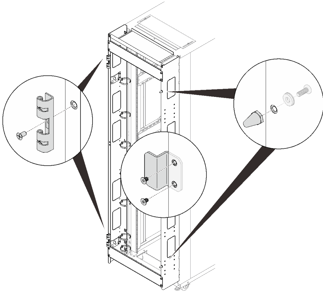
그림 38. 힌지, 도어스토퍼, 도어 래치 설치
