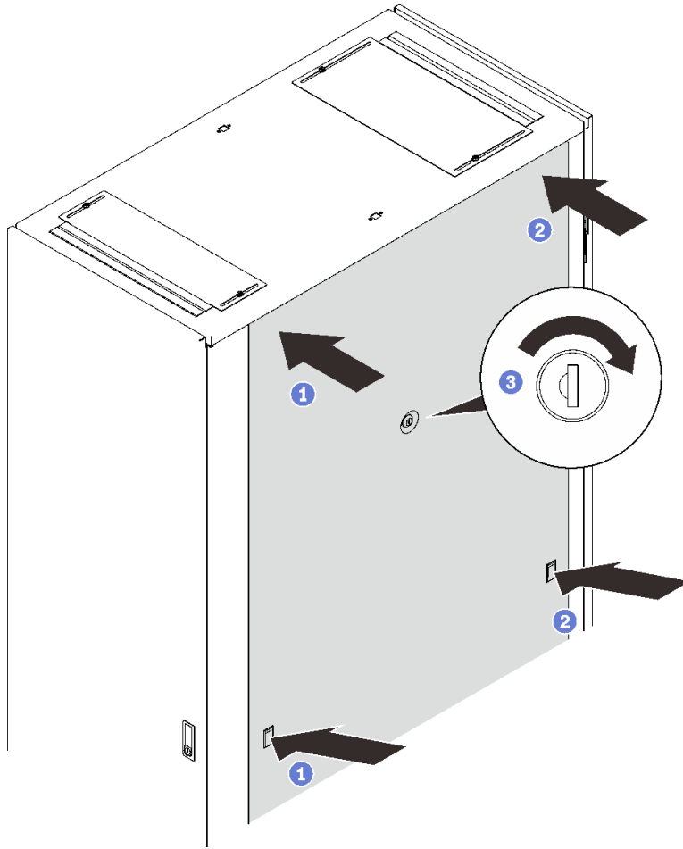
그림 114. 측면 덮개 고정
