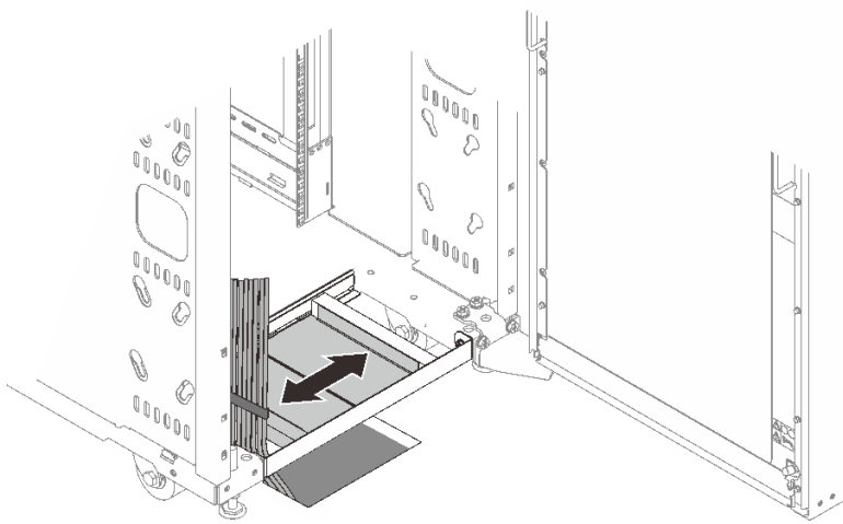
그림 108. 하부 공기 조절 장치로 케이블 관리
