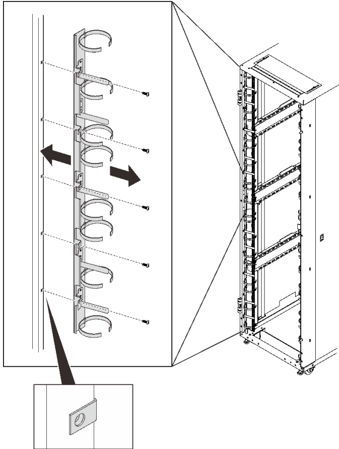
그림 181. 21U 케이블 스트랩 모듈 설치
