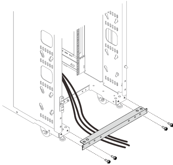
รูปภาพ 15. การถอดแถบการเข้าถึงสาย
