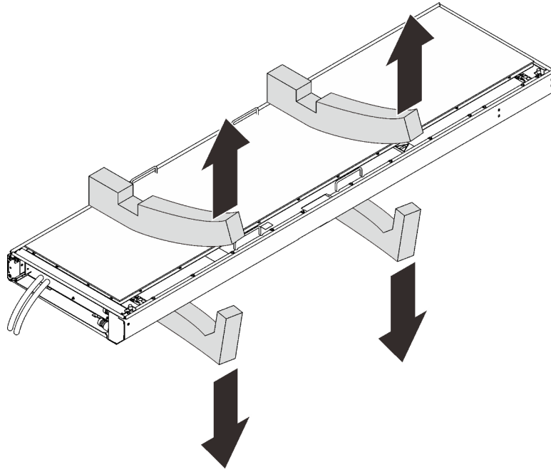
รูปภาพ 60. การถอดตัวสลับความร้อน
