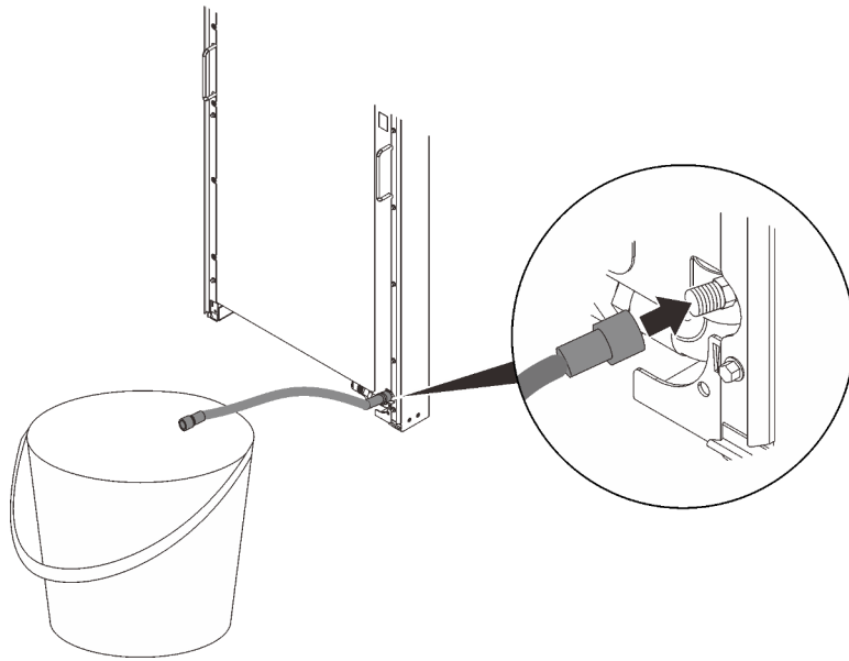
รูปภาพ 49. การระบายน้ำ
