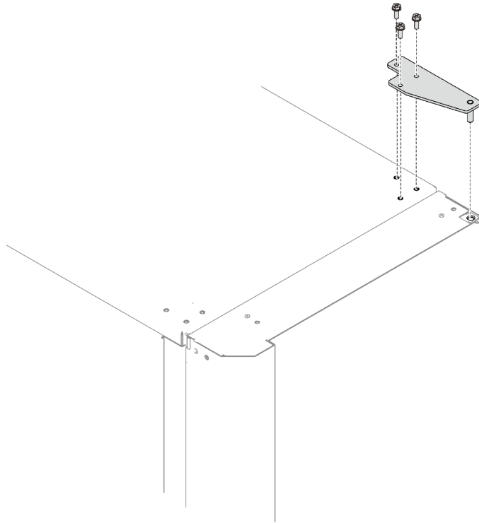
รูปภาพ 53. การถอดบานพับด้านบน
