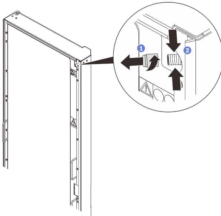
รูปภาพ 64. การไล่ไนโตรเจน
