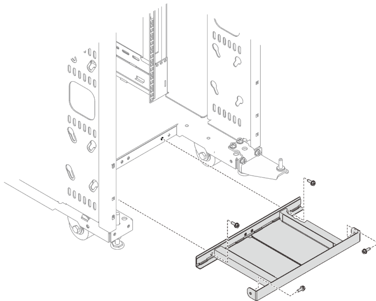
รูปภาพ 16. การติดตั้งแผ่นกั้นลมด้านล่าง
