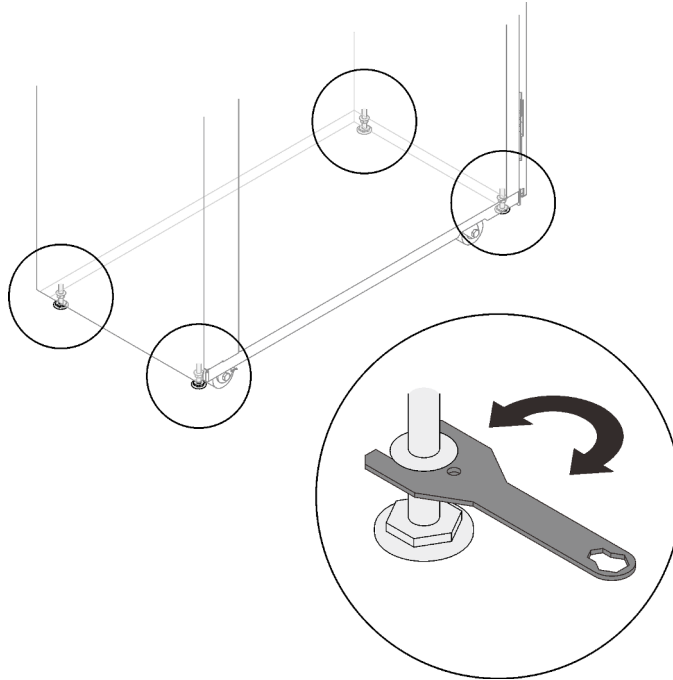
รูปภาพ 10. การลดแผ่นปรับระดับ
