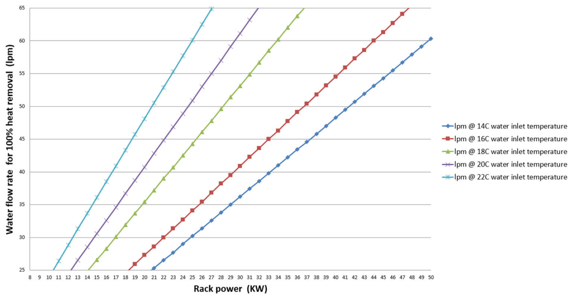
รูปภาพ 4. ประสิทธิภาพทั่วไปของตัวแลกเปลี่ยนความร้อน, การไหลของอากาศในแร็ค 4800SCFM อุณหภูมิเข้าสู่อากาศ 25°C
