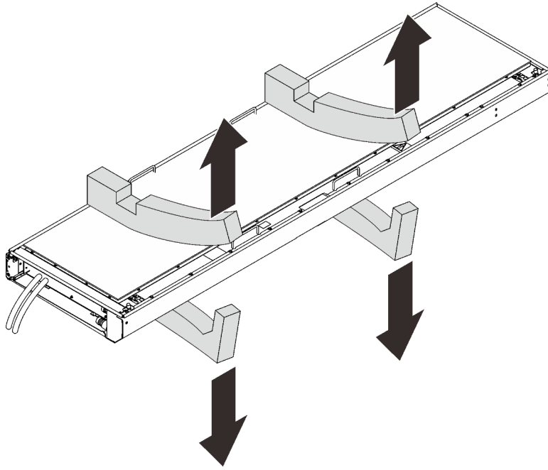
รูปภาพ 23. การถอดตัวสลับความร้อน
