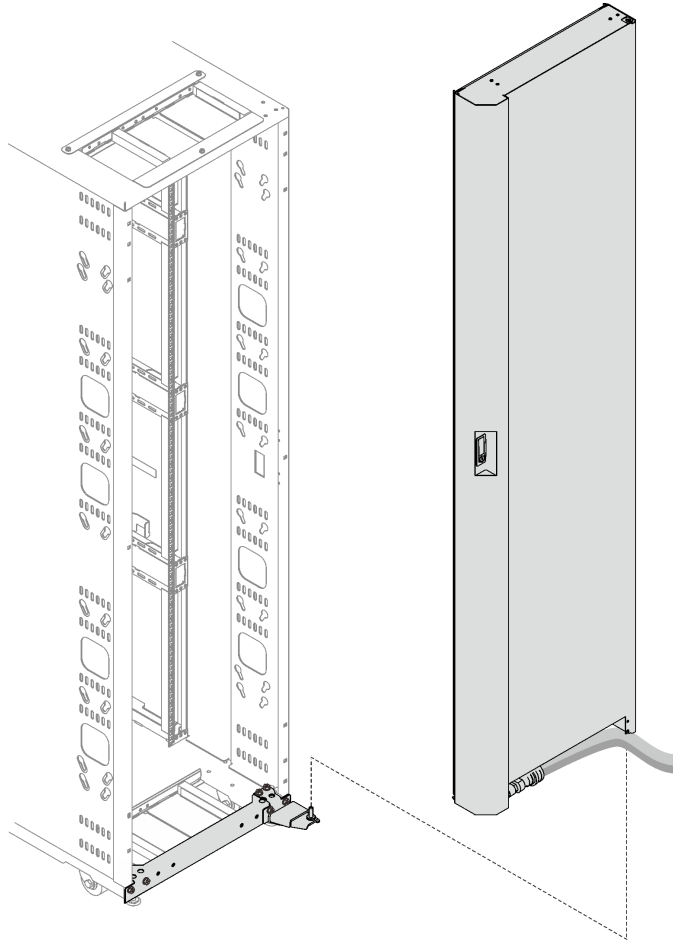
รูปภาพ 55. การถอดตัวแลกเปลี่ยนความร้อนออกจากตู้แร็ค
