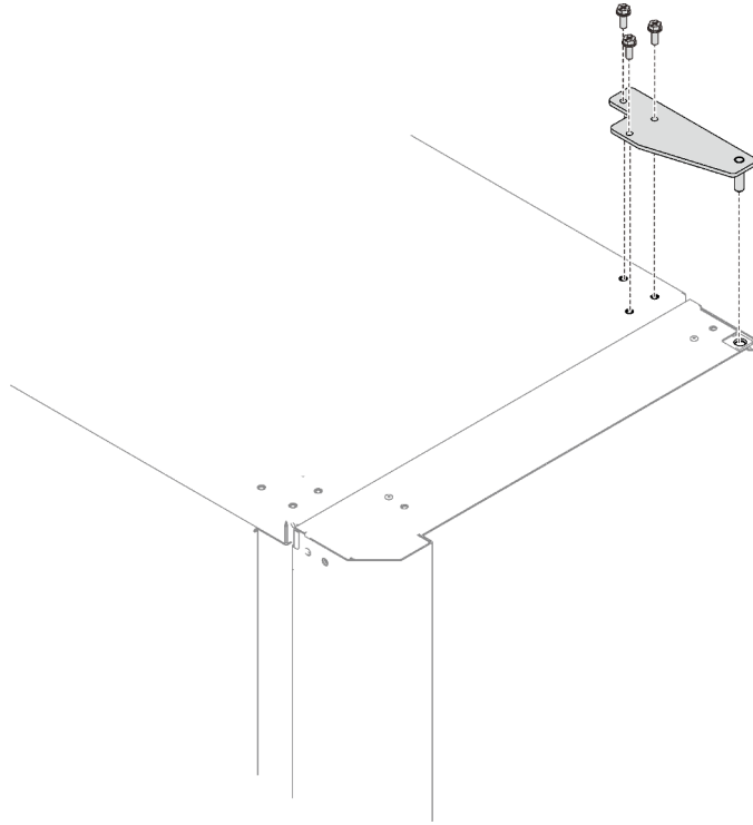
รูปภาพ 26. การติดตั้งบานพับด้านบน
