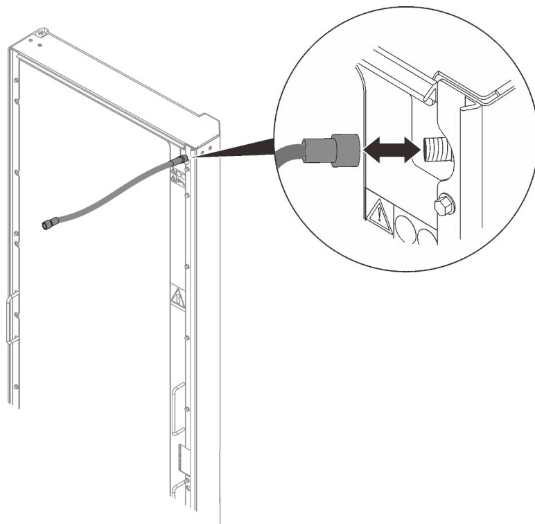
รูปภาพ 50. การถอดท่อต่อเครื่องมือไล่อากาศ
