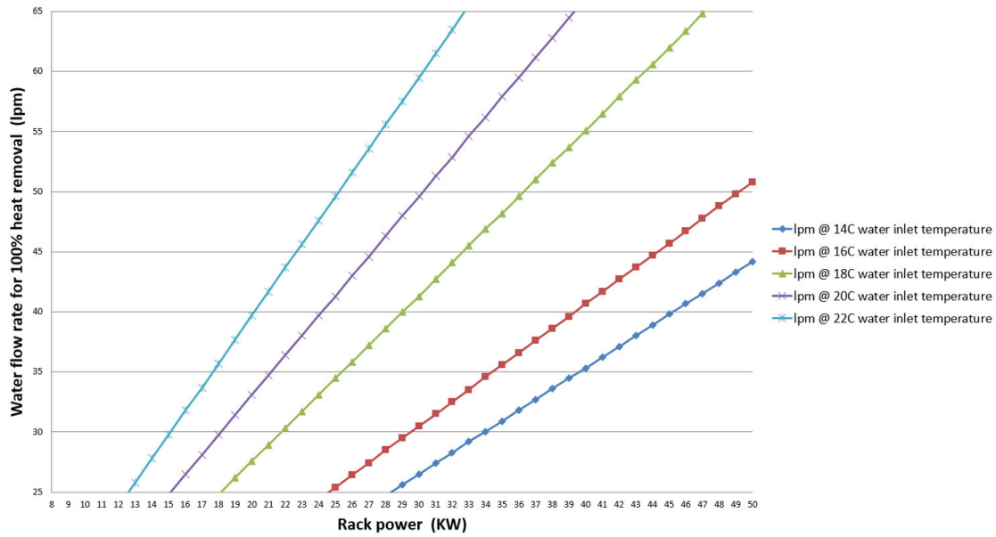
รูปภาพ 3. ประสิทธิภาพทั่วไปของตัวแลกเปลี่ยนความร้อน, การไหลของอากาศในแร็ค 3840SCFM อุณหภูมิเข้าสู่อากาศ 25°C
