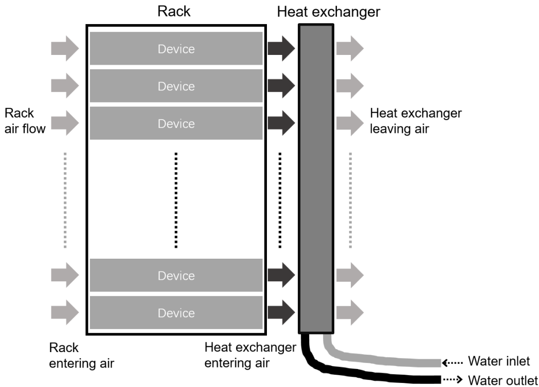
รูปภาพ 2. แผนผังการไหลของอากาศในแร็คและการไหลของน้ำในตัวแลกเปลี่ยนความร้อน
