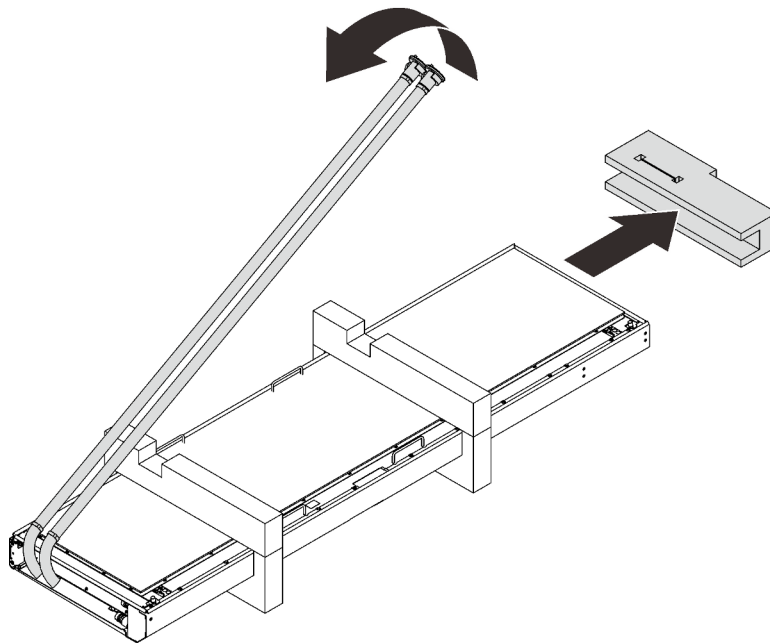
รูปภาพ 59. การถอดตัวสตูยึด
