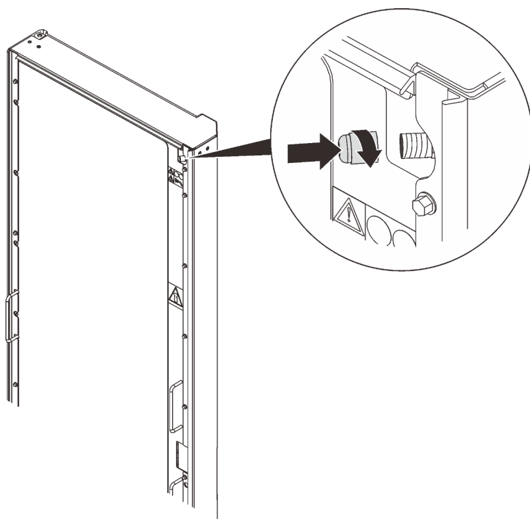
รูปภาพ 37. การติดตั้งฝวาลัว
