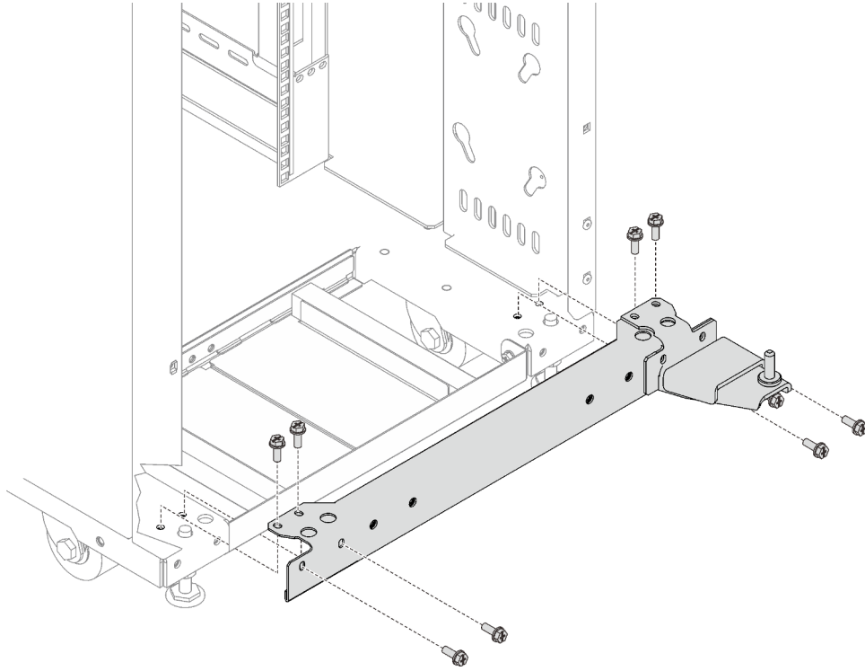
รูปภาพ 17. การติดตั้งส่วนประกอบบานพับด้านล่าง
