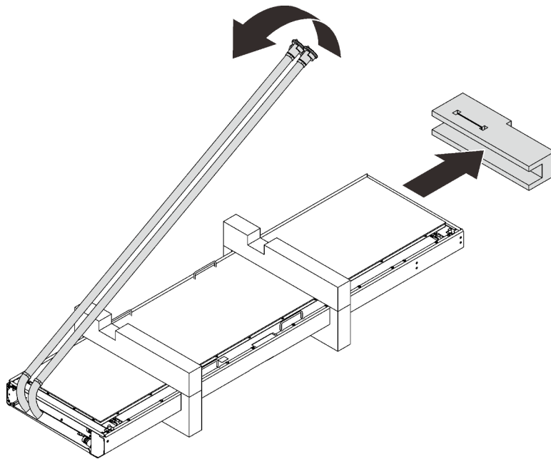
รูปภาพ 22. การถอดตัวสตูยึด
