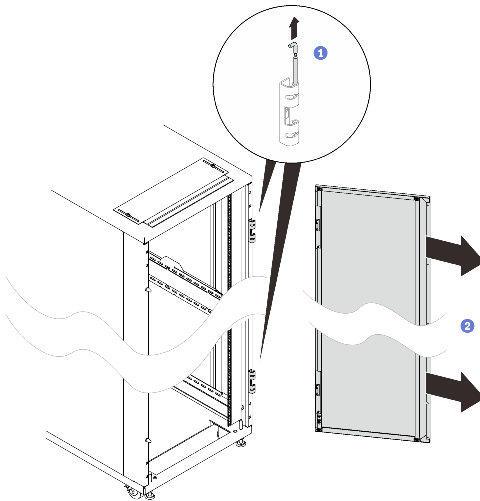
รูปภาพ 11. การถอดประตู
