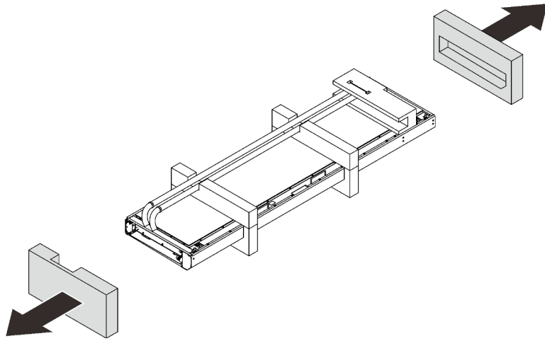
รูปภาพ 21. การถอดตัวสตูบรจุกัณฑ์
