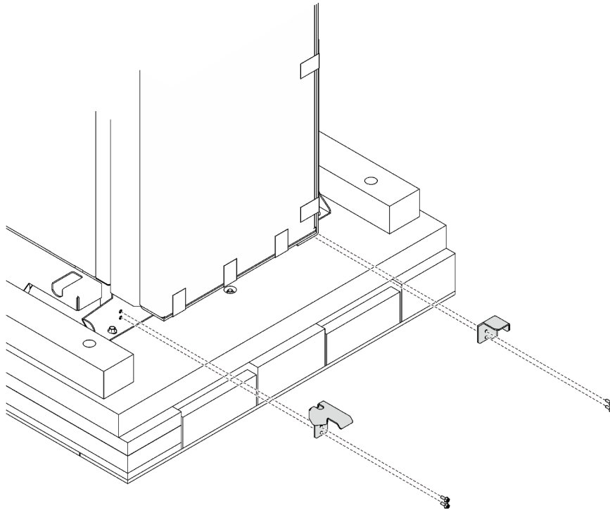
รูปภาพ 5. การถอดโครงยึดที่รองรับ
