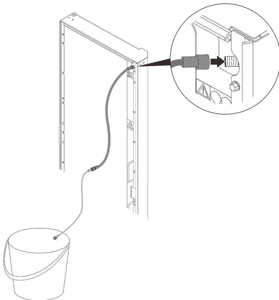
รูปภาพ 65. การติดตั้งเครื่องมือไล่อากาศ
