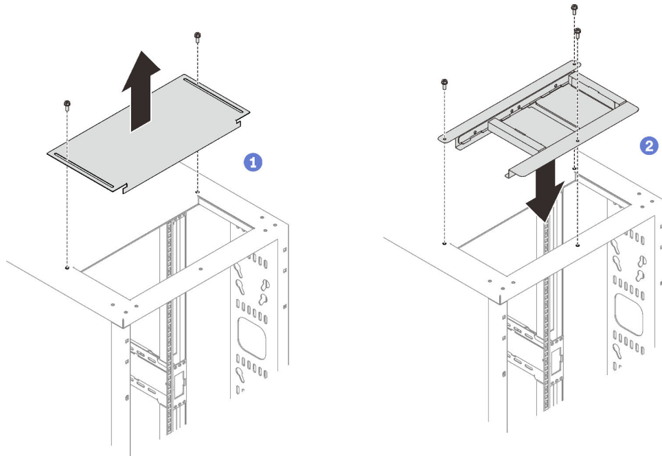
รูปภาพ 14. การติดตั้งแผ่นกันลมด้านบน
