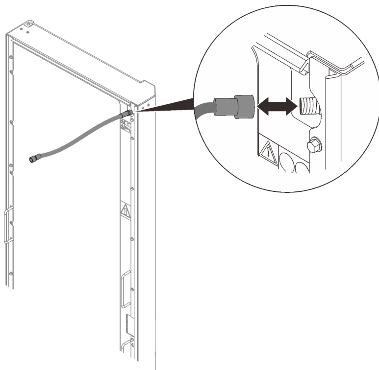
รูปภาพ 48. การใส่ท่อต่อเครื่องมือไล่อากาศ
