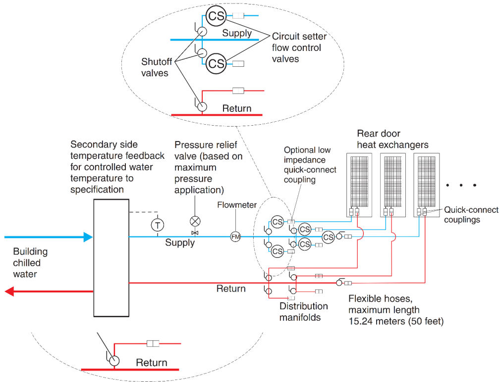
รูปภาพ 29. หน่วยจ่ายสารระบายความร้อนที่ใช้โซลูชันซีพพลายเออร์ที่มีจำหน่ายทั่วไป
