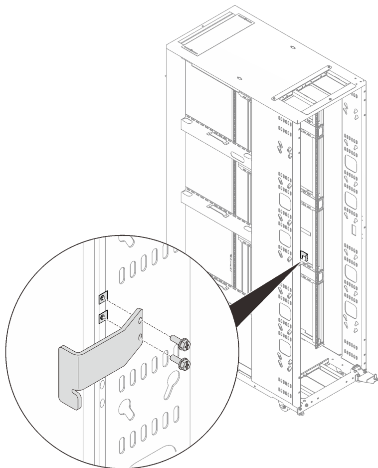
รูปภาพ 18. การติดตั้งแผ่นสลัก
