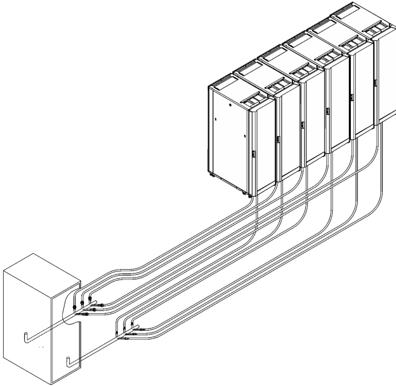
รูปภาพ 31. ท่อร่วมกลางทั่วไป (ในตำแหน่งศูนย์กลางสำหรับวงจรน้ำหลายวงจร)
