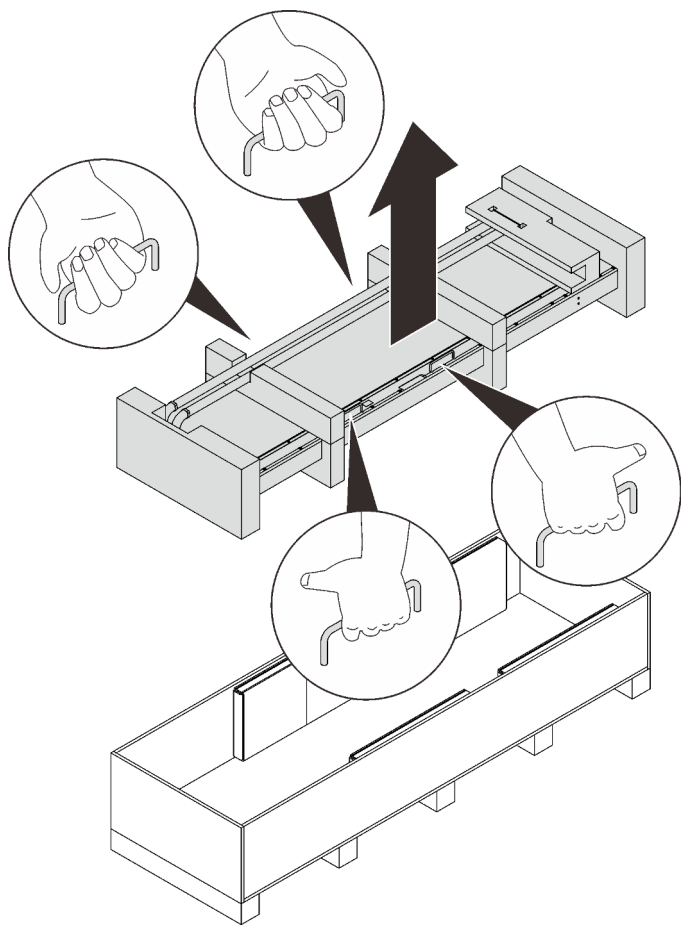
รูปภาพ 57. การถอดตัวแลกเปลี่ยนความร้อน
