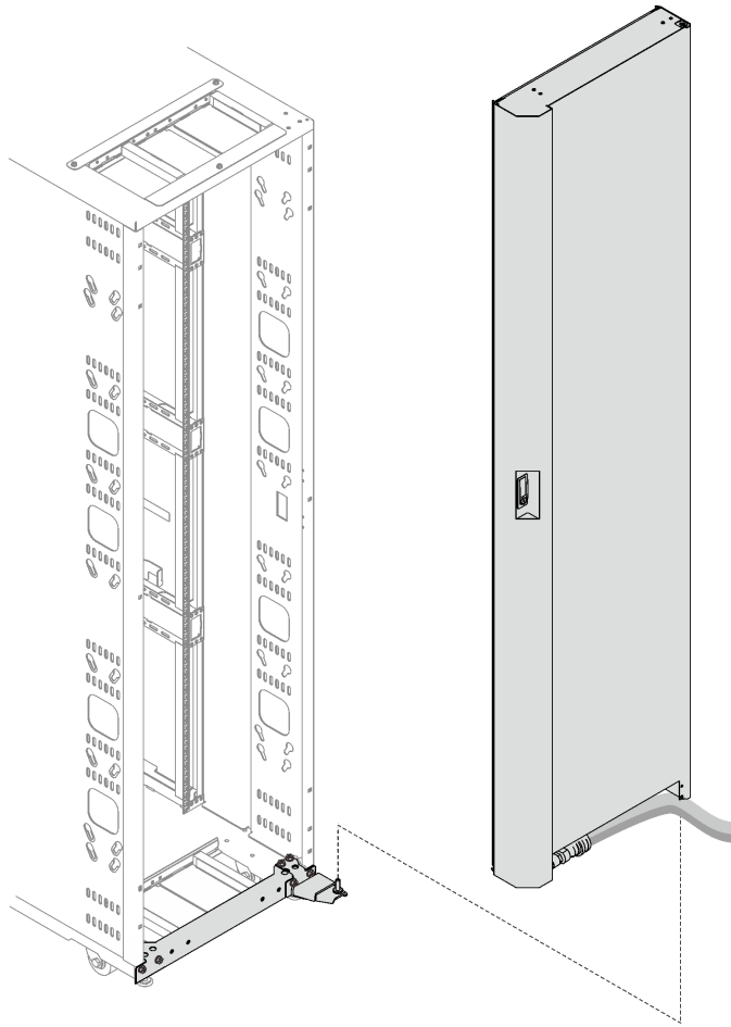
รูปภาพ 62. การติดตั้งตัวแลกเปลี่ยนความร้อนเข้ากับตู้แร็ค
