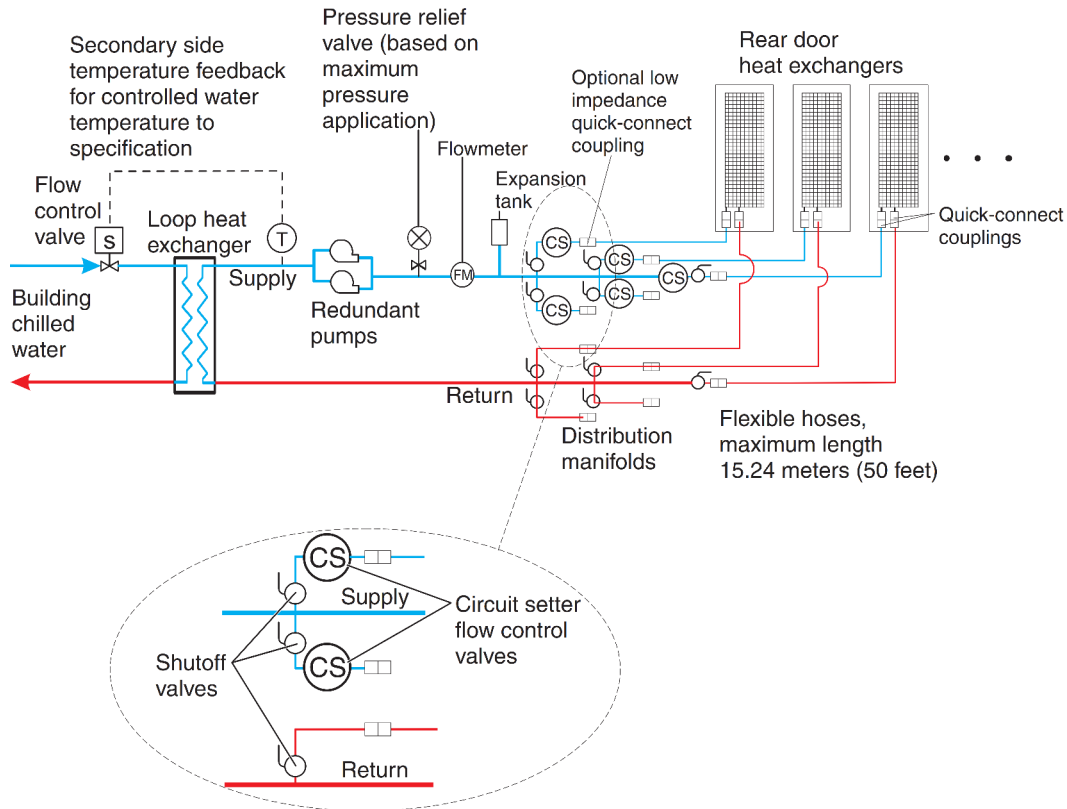
รูปภาพ 28. หน่วยจ่ายสารระบายความร้อนพร้อมโซลูชันสิ่งอำนวยความสะดวกประดิษฐ์
