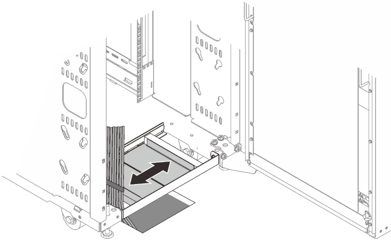
รูปภาพ 39. การจัดสายที่มีแผ่นกั้นลมด้านล่าง
