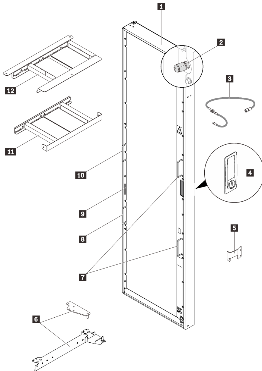
รูปภาพ 1. ส่วนประกอบ ThinkSystem Rear Door Heat eXchanger สำหรับแร็ค 48U
