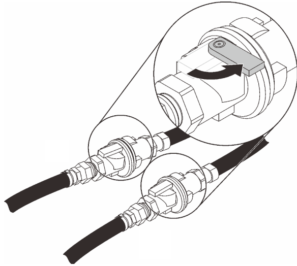
รูปภาพ 45. การเปิดบอลวาล์ว Eaton
