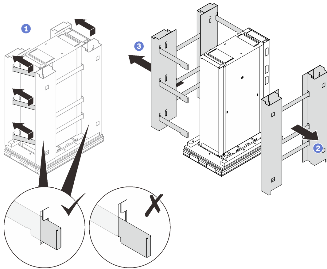
รูปภาพ 5. การถอดโครงด้านข้าง
