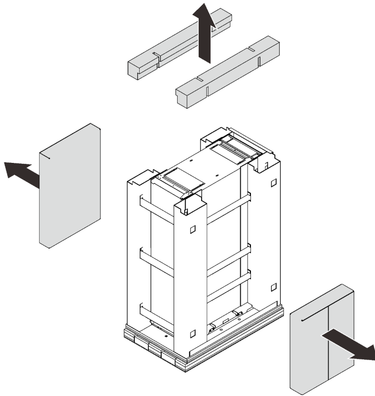
รูปภาพ 4. การถอดแถบด้านบนและกระดาดข้างด้านข้างออก
