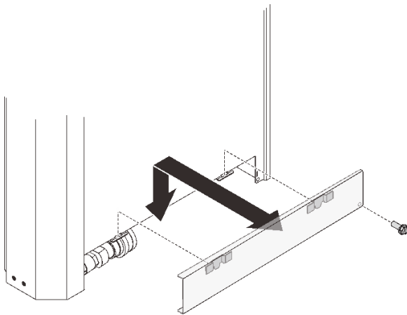
图 61. 卸下外侧软管走线面板
