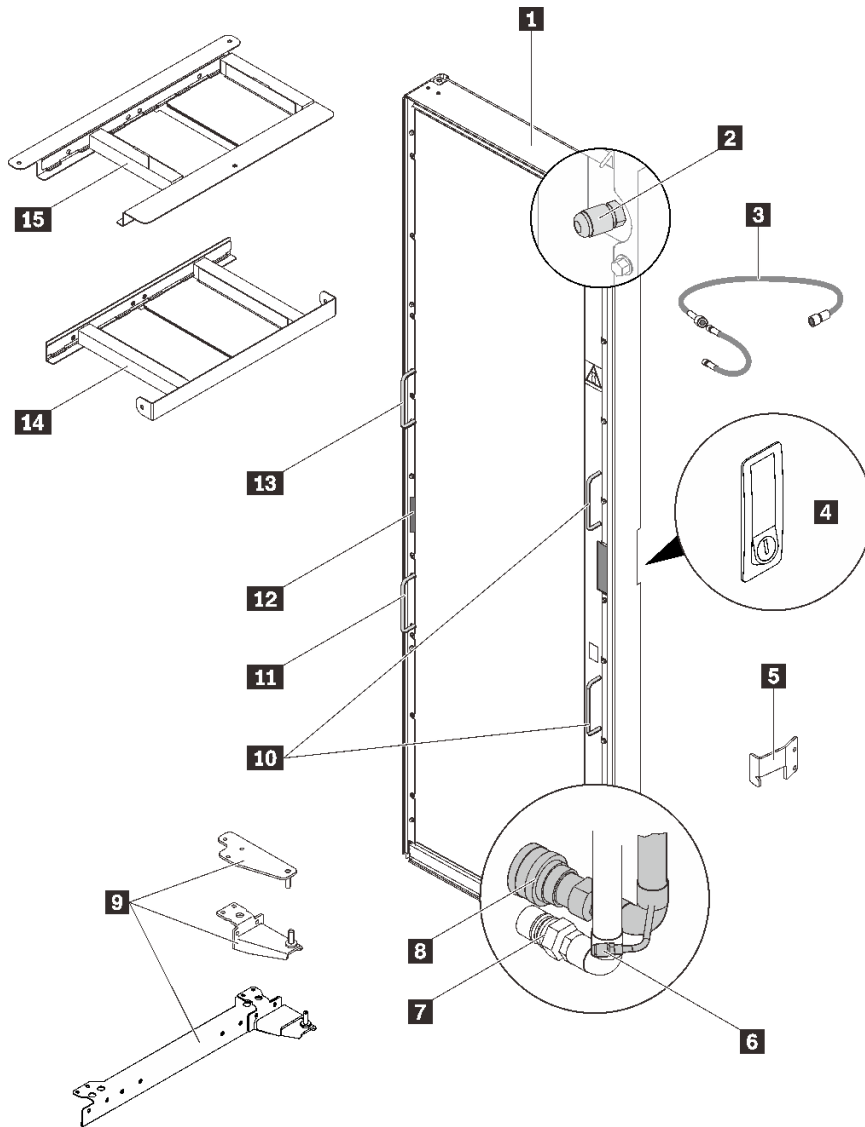
图 1. ThinkSystem Rear Door Heat eXchanger V2 组件
