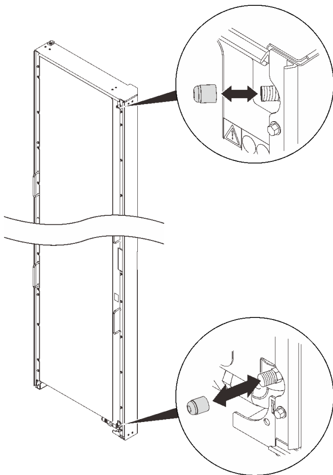
图 49. 安装阀盖
