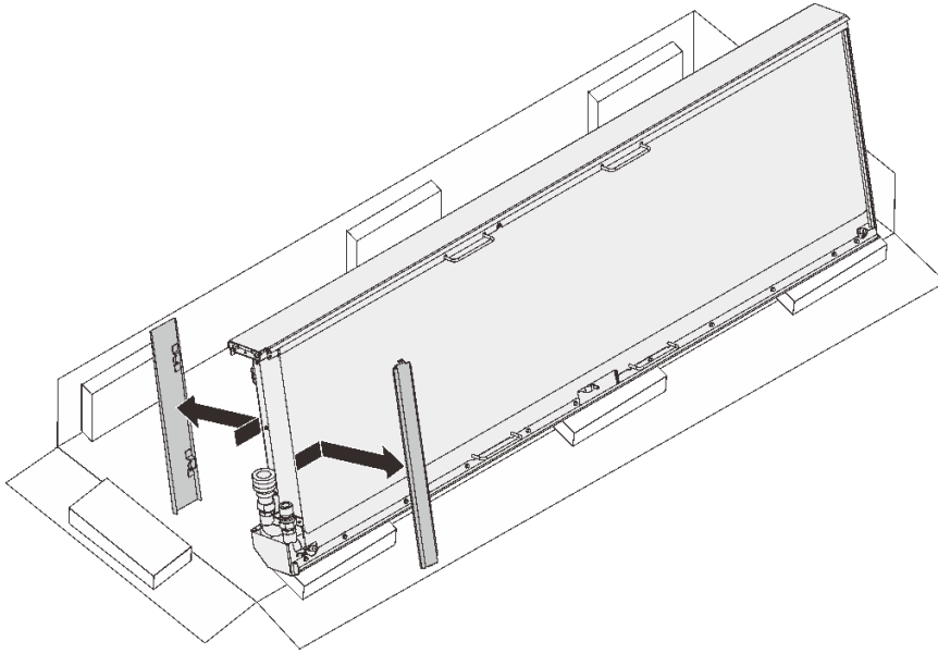
图 16. 卸下软管走线面板
