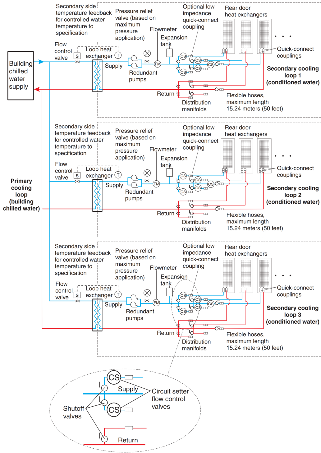
图 20. 初级冷却回路和二级冷却回路
