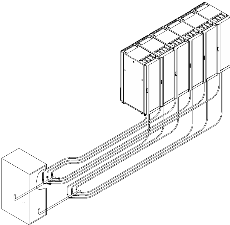
图 24. 典型的中央歧管（位于多个水回路的中心位置）
