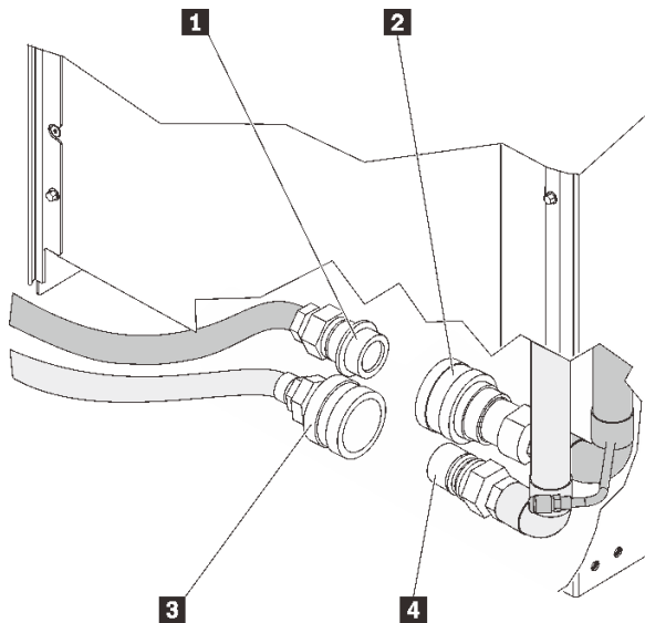
图 29. 供给软管和回流软管以及歧管接头
