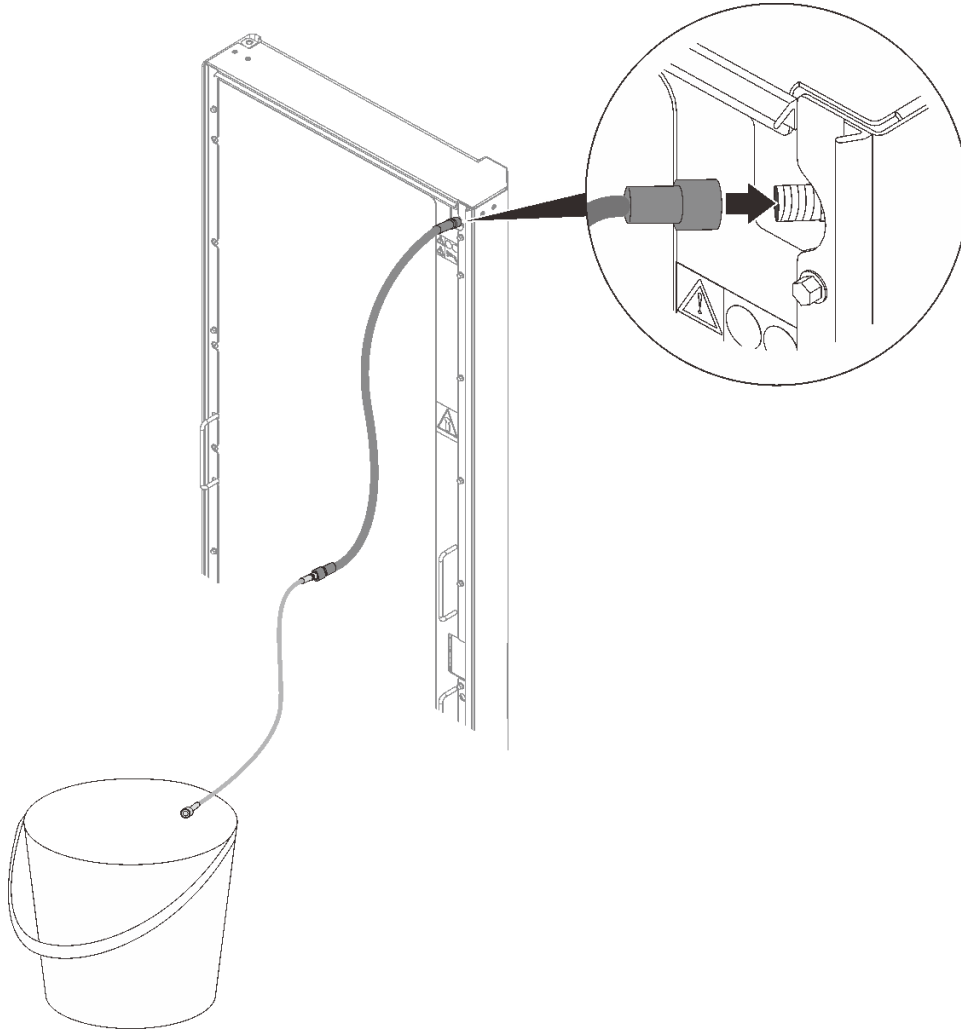
图 30. 安装空气吹扫工具
