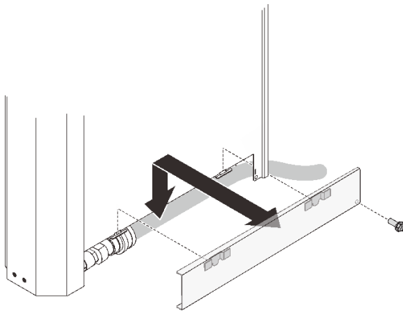
图 68. 安装外侧软管走线面板
