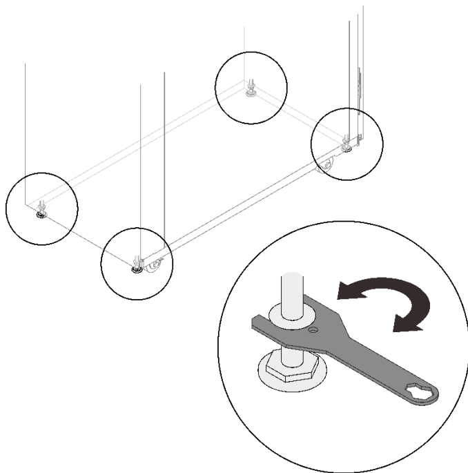
图 6. 降低调平垫片
