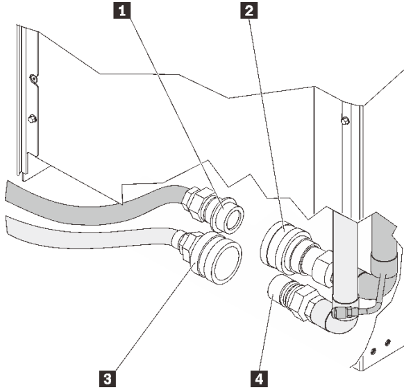
图 42. 供给软管和回流软管以及歧管接头
