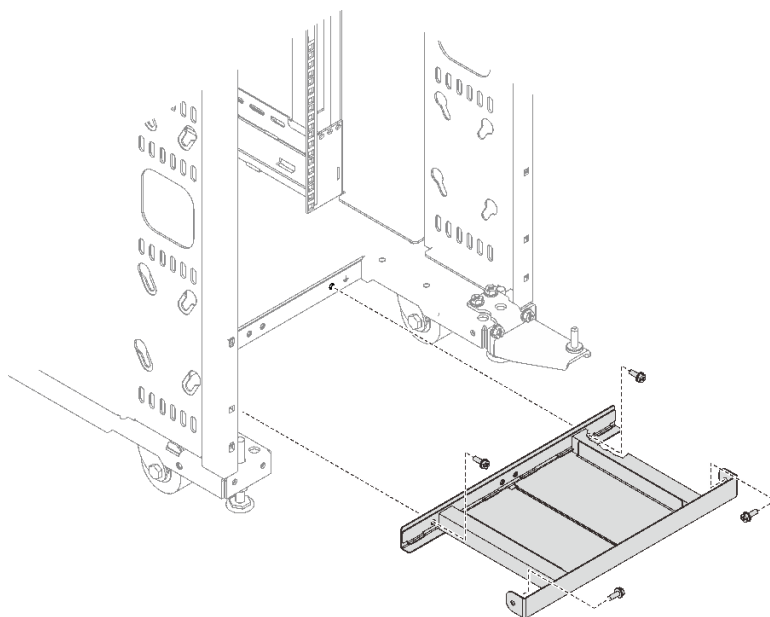
图 13. 安装下方导风罩
