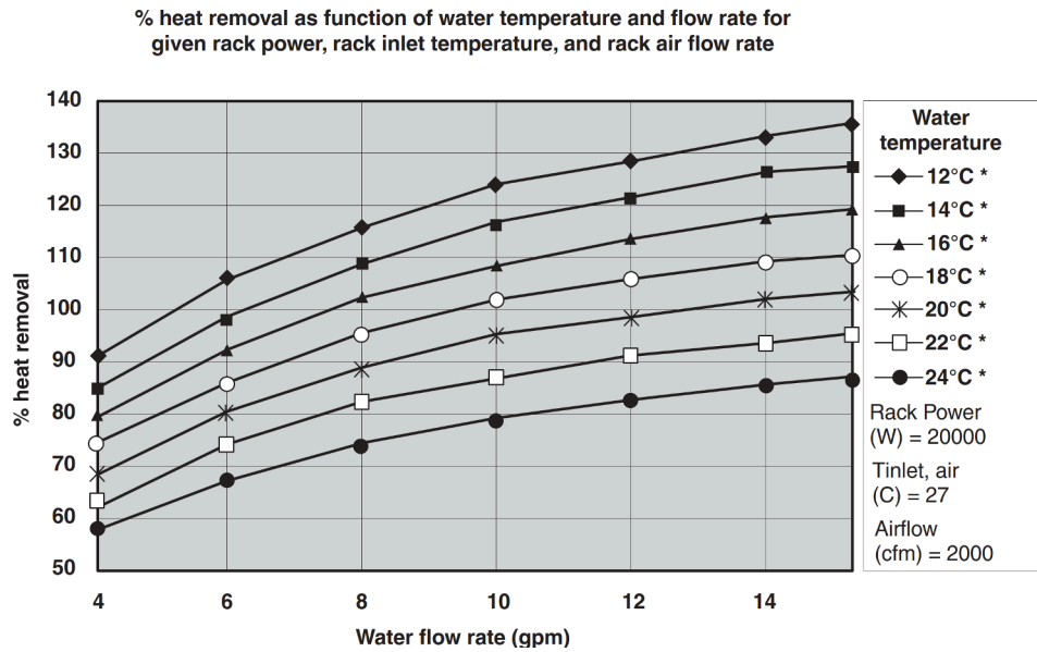
图 3. 热负荷为 20 kW 时，热交换器的典型性能
