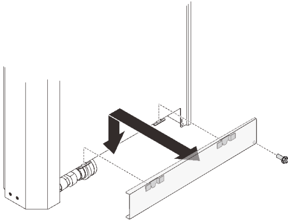
图 27. 卸下外侧软管走线面板
