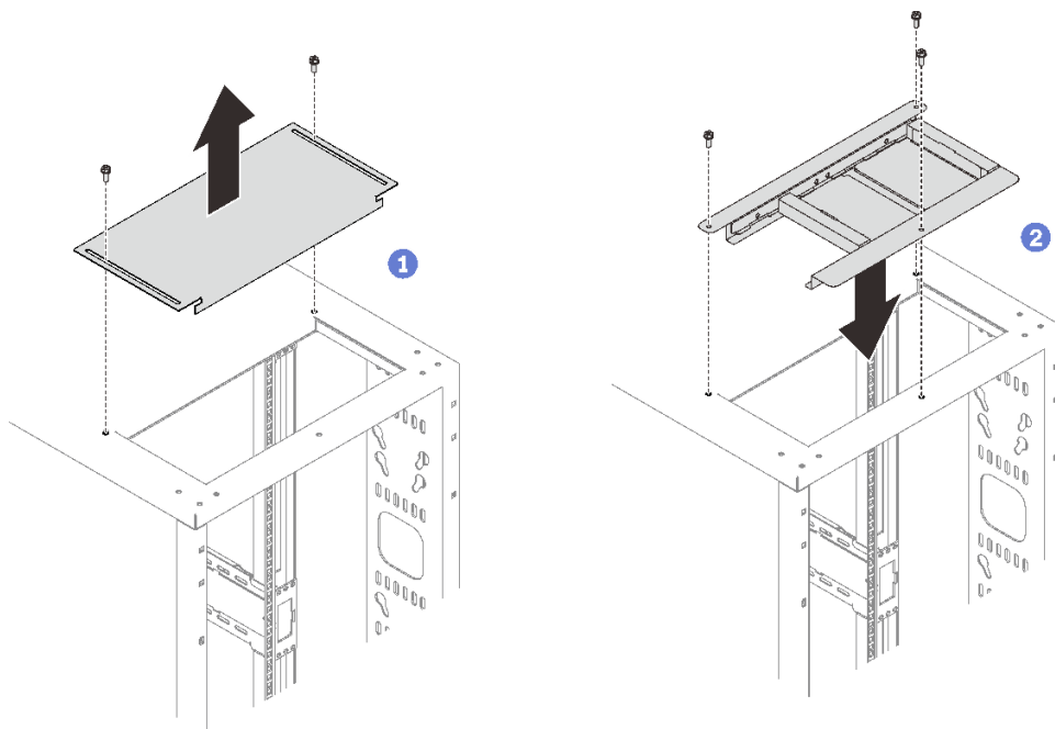
图 11. 安装上方导风罩
