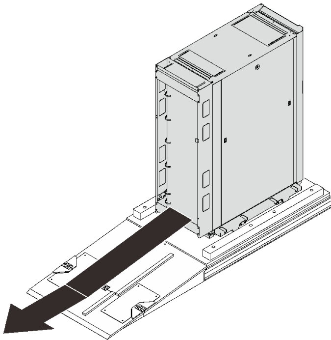
图 5. 将机架机柜从托板上移下
