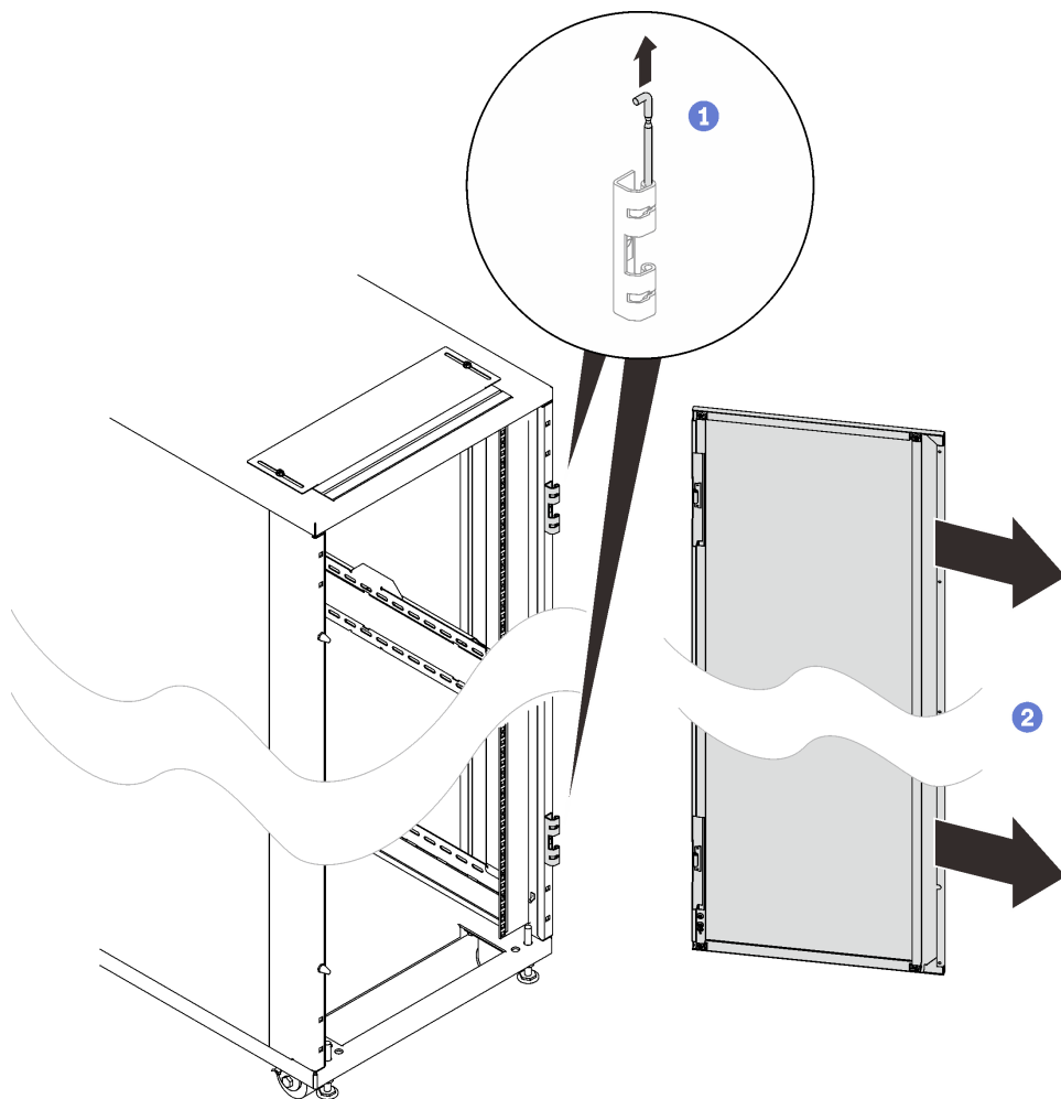
图 7. 卸下柜门
