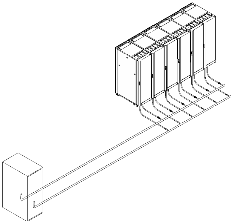
图 25. 典型的延长歧管（沿机架之间的通道）
