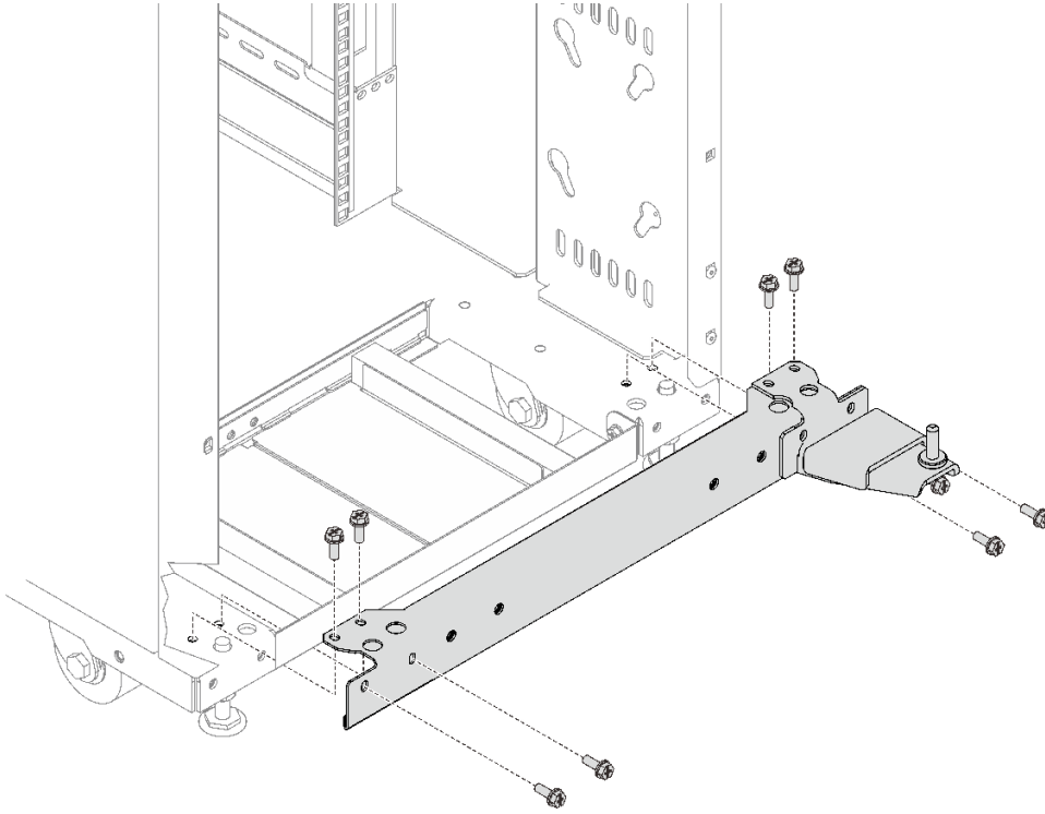
图 14. 安装底部铰链组合件
