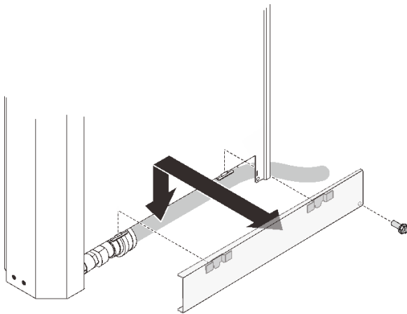
图 34. 安装外侧软管走线面板
