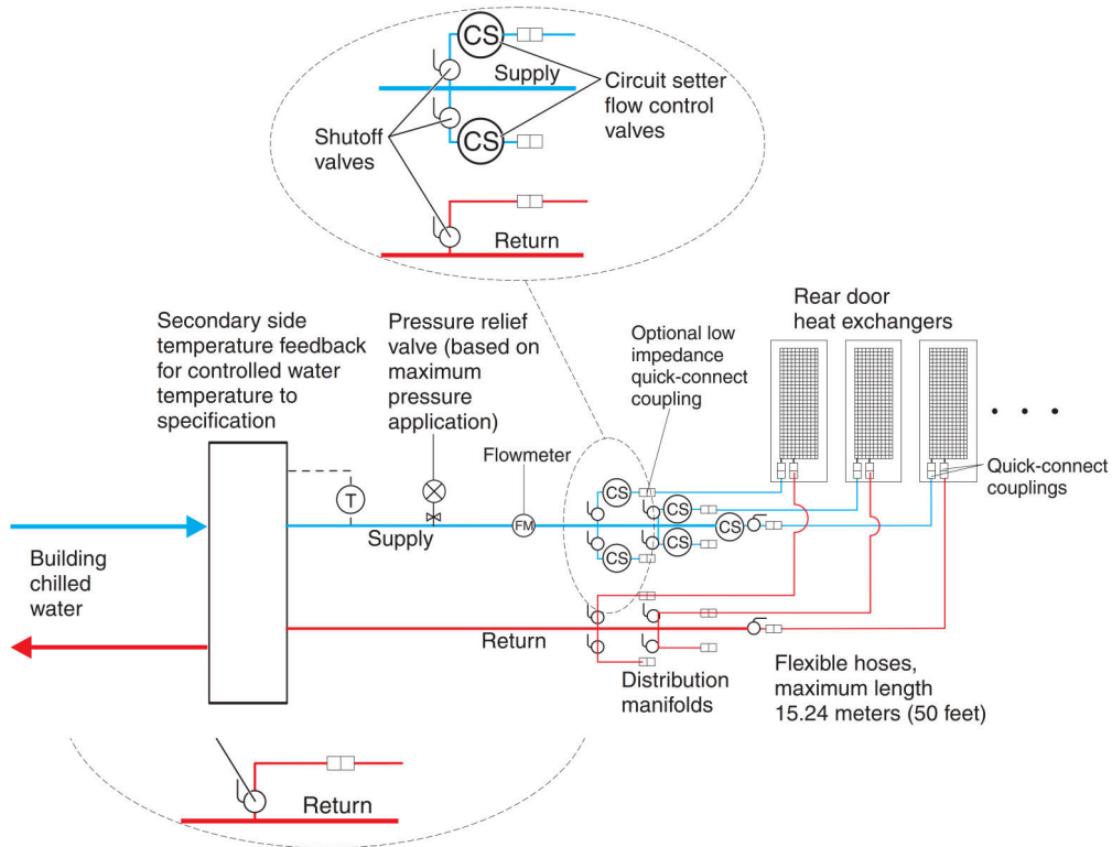
图 22. 使用现成供应商解决方案的冷却液分配单元
