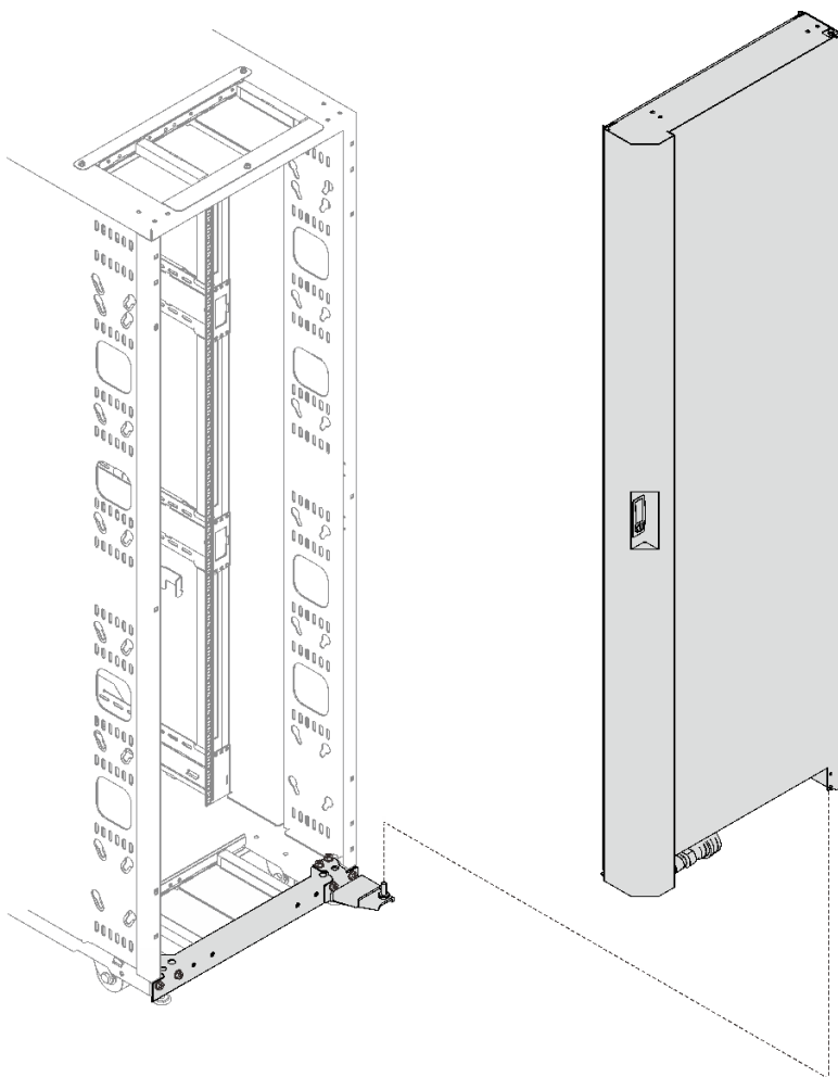
图 18. 将热交换器安装到机架机柜上
