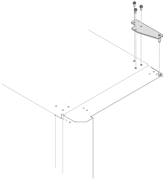
图 19. 安装顶部铰链
