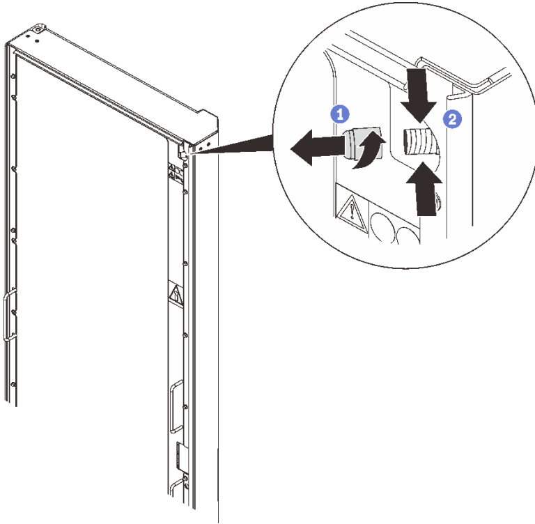
图 62. 吹扫氮气
