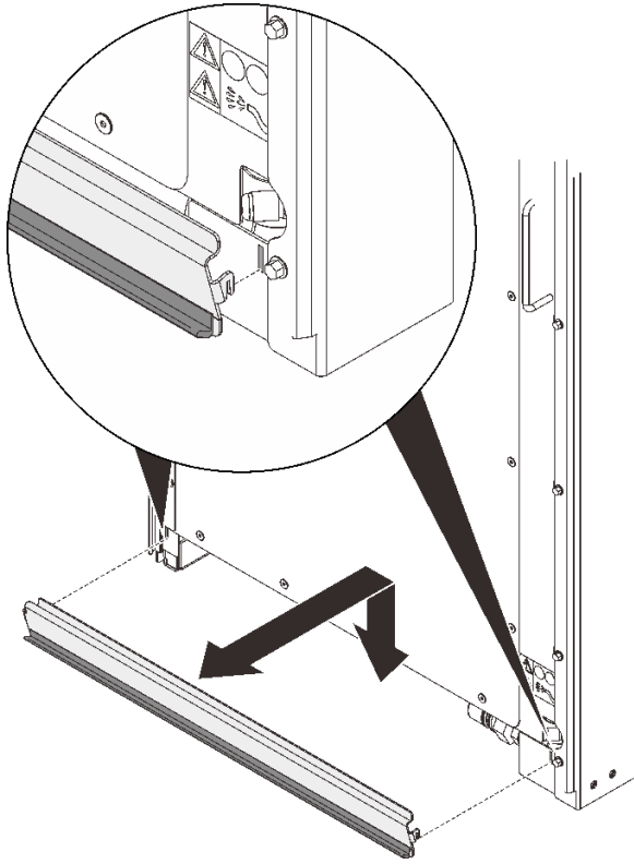
图 60. 卸下内侧软管走线面板
