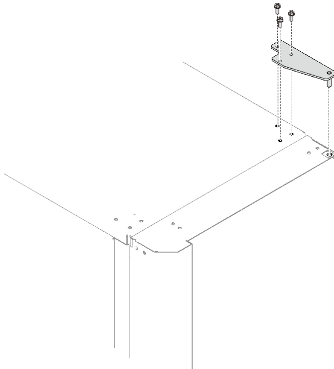
图 50. 卸下顶部铰链
