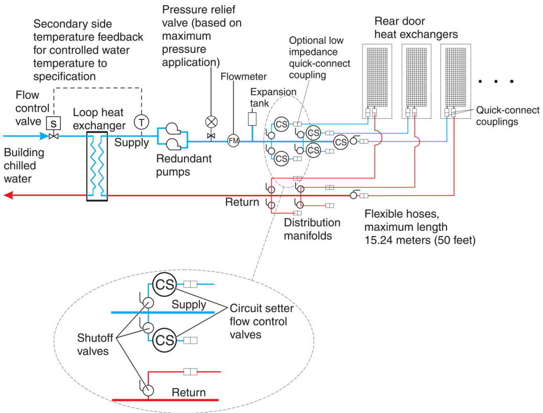
图 21. 采用定制设施解决方案的冷却液分配单元
