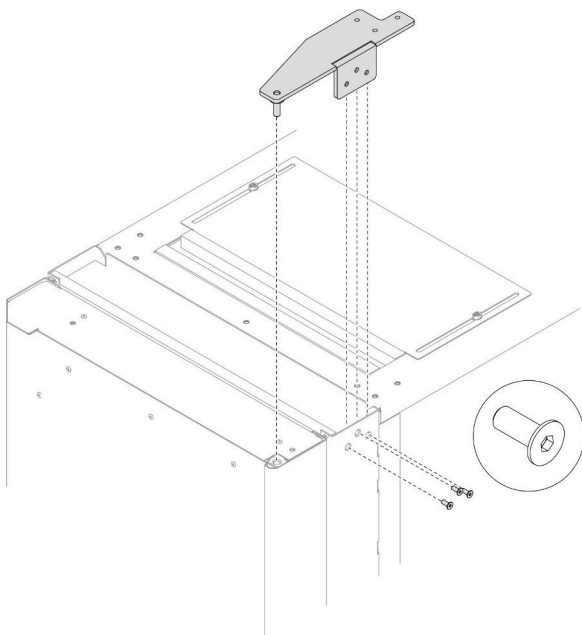
图 59. 安装顶部铰链
