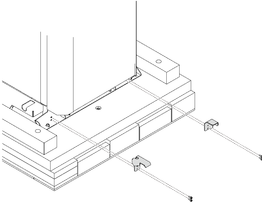
图 4. 卸下支撑架
