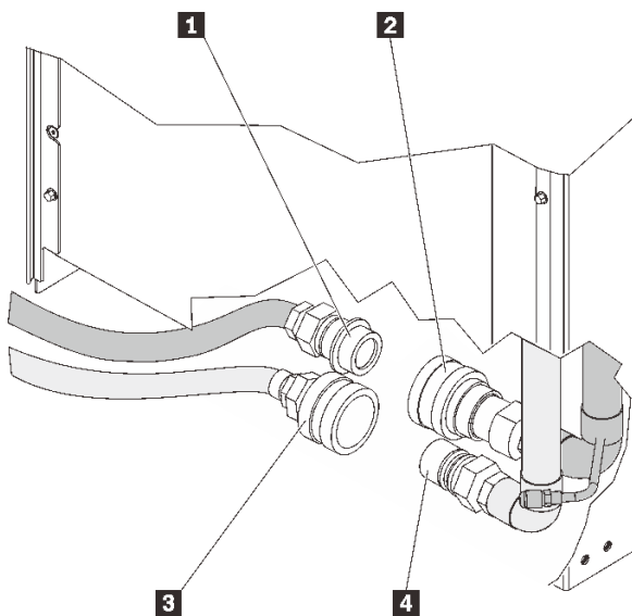
图 63. 供给软管和回流软管以及歧管接头
