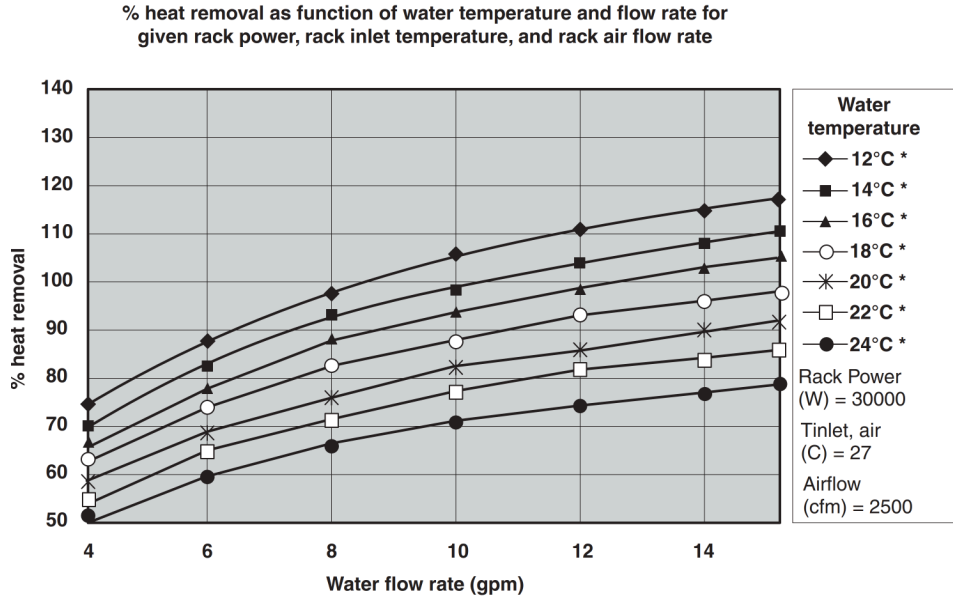
图 2. 热负荷为 30 kW 时，热交换器的典型性能
