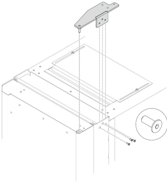
图 51. 卸下顶部铰链
