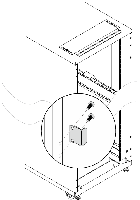
图 9. 卸下门闩
