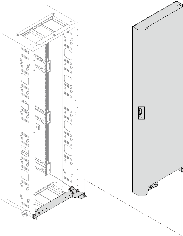
图 57. 将热交换器安装到机架机柜上
