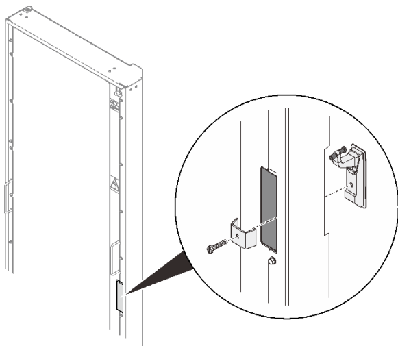
图 69. 更换门闩
