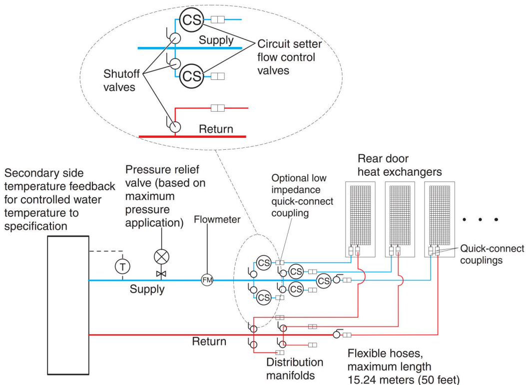
图 23. 使用现成供应商解决方案的冷却液分配单元
