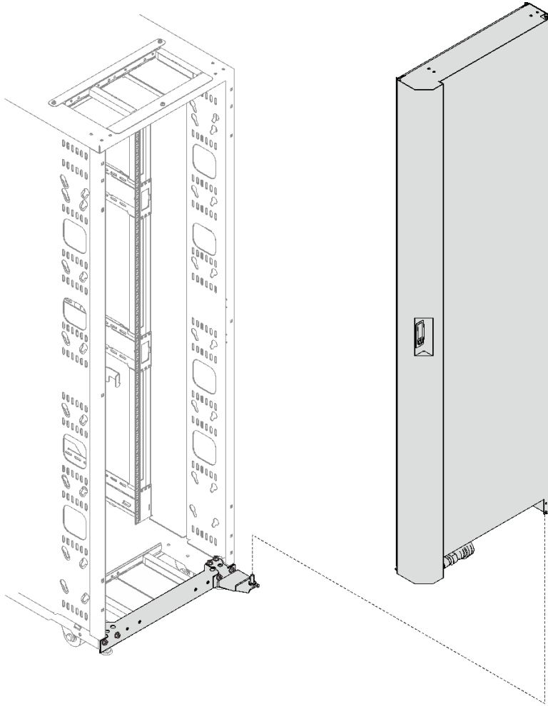
图 53. 从机架机柜中卸下热交换器
