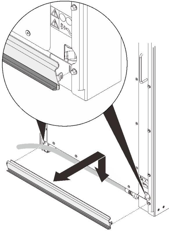
图 67. 安装内侧软管走线面板
