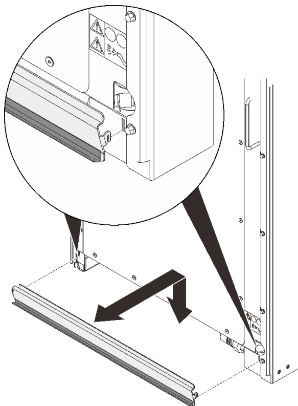
图 26. 卸下内侧软管走线面板
