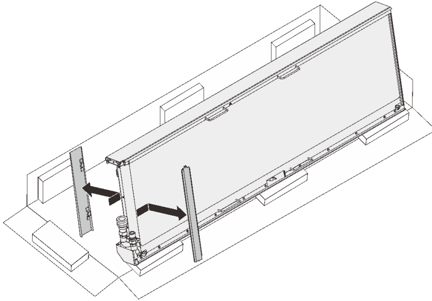
图 55. 卸下软管走线面板
