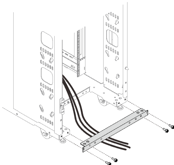
图 12. 卸下走线排
