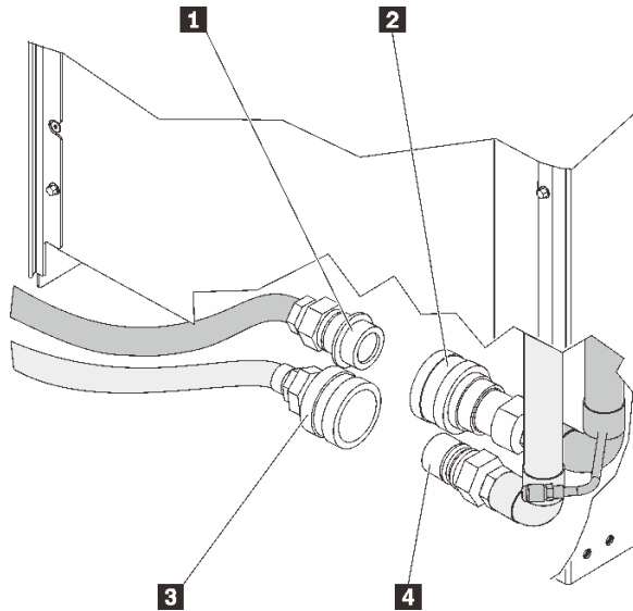
圖例 63. 供應和回流軟管以及歧管接頭
