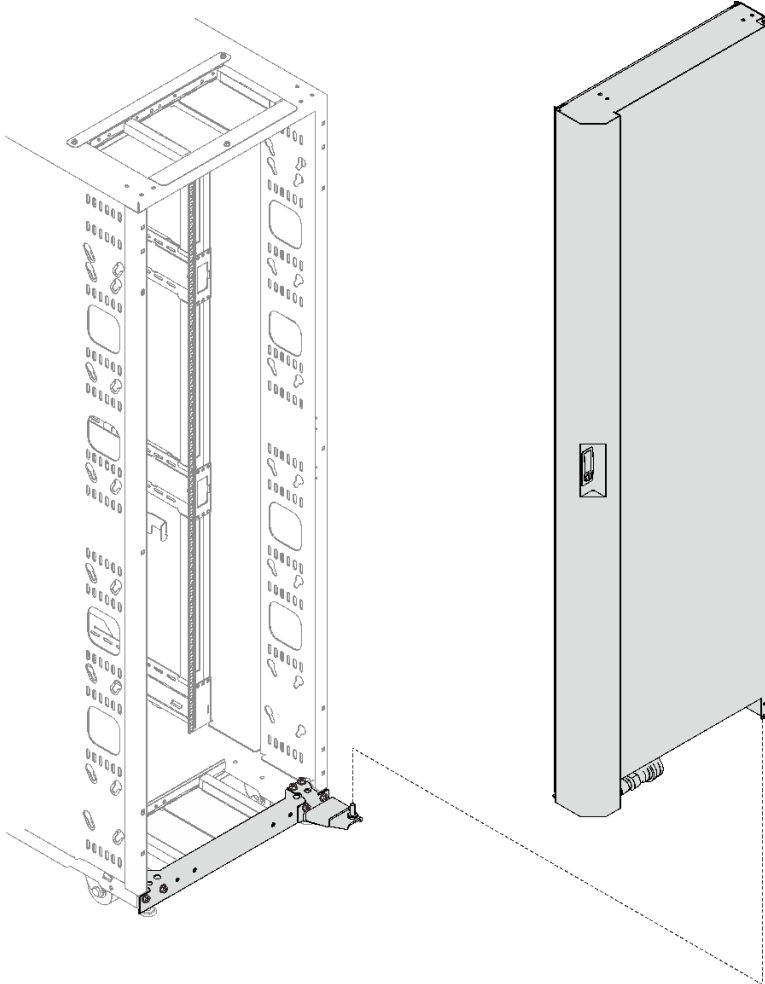
圖例 53. 從機櫃卸下熱交換器
