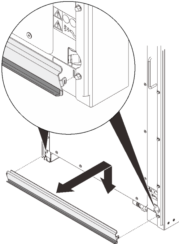
圖例 60. 卸下內部軟管檢修面板
