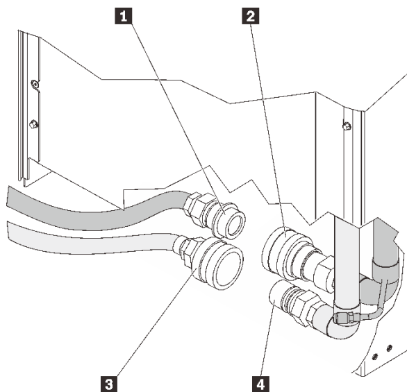
圖例 42. 供應和回流軟管以及歧管接頭
