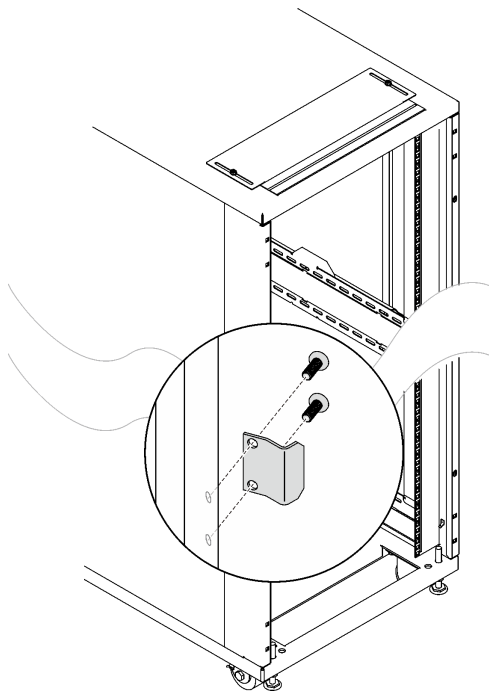
圖例 9. 卸下門門
