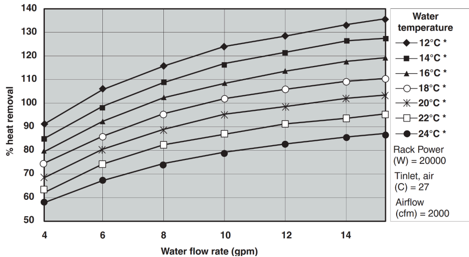
圖例 3. 熱交換器的典型效能，20 kW 熱負荷
