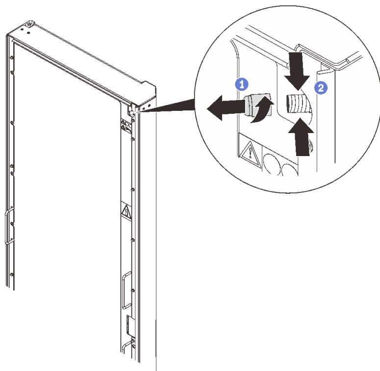
圖例 62. 吹掃氮氣
