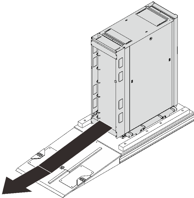
圖例 5. 將機櫃從托板上移開
