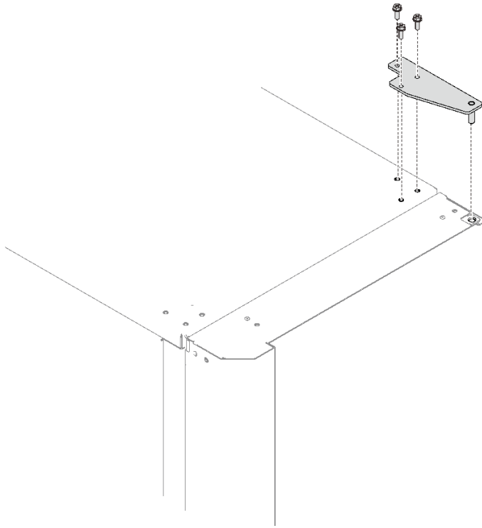
圖例 58. 安裝頂部鉸鏈
