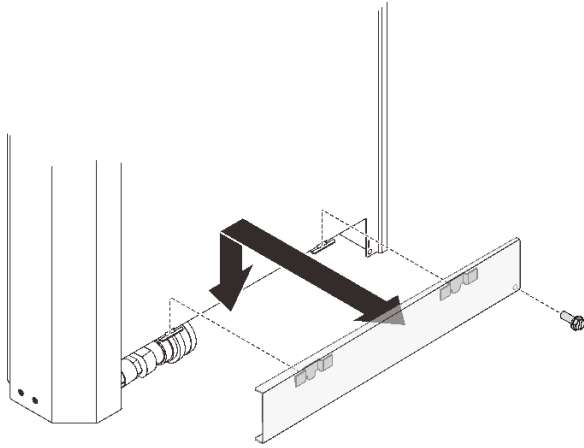
圖例 27. 卸下外軟管檢修面板
