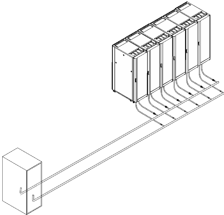
圖例 25. 典型的擴展歧管 (沿著機架之間的通道)
