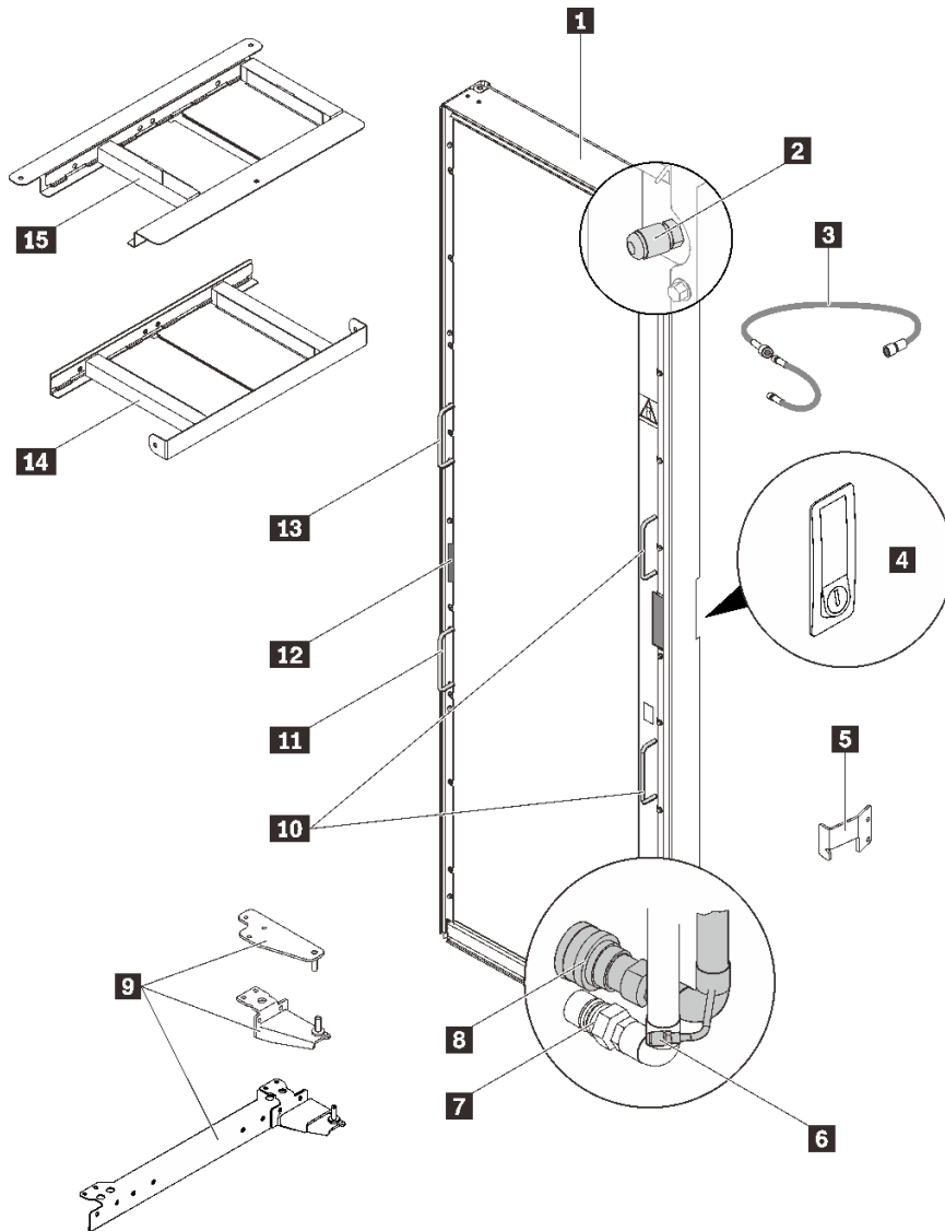
圖例 1. ThinkSystem Rear Door Heat eXchanger V2 元件
