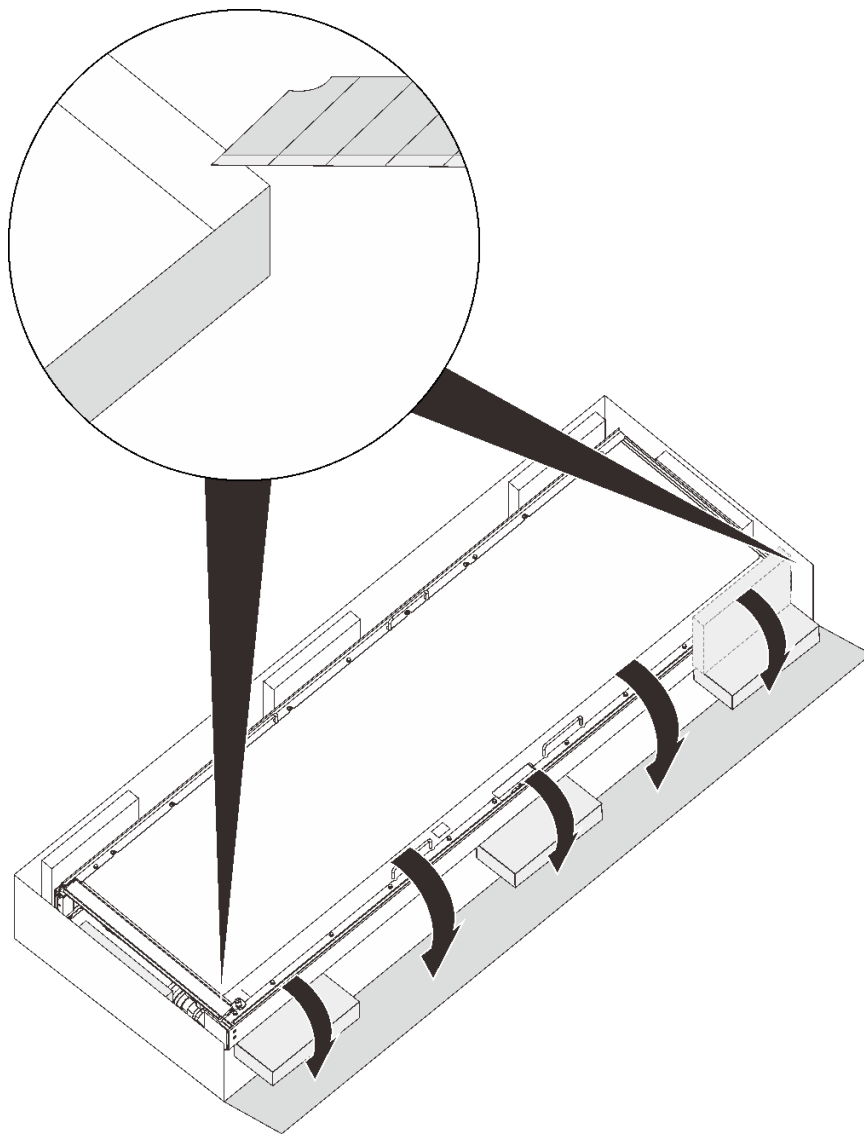
圖例 54. 拆開熱交換器的包裝
