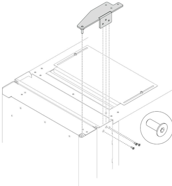
圖例 59. 安裝頂部鉸鏈
