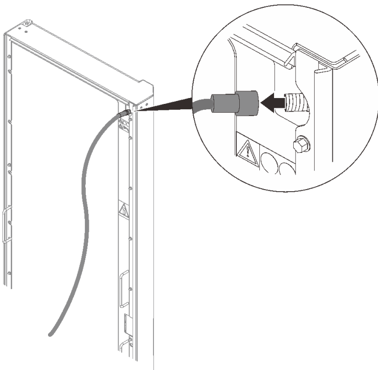
圖例 65. 卸下空氣吹掃工具
