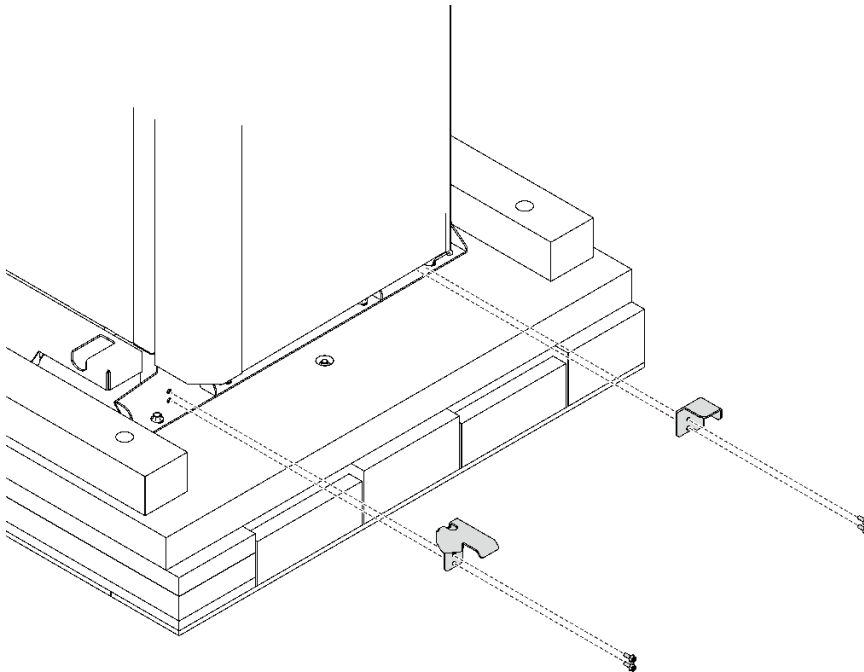
圖例 4. 卸下支撐托架
