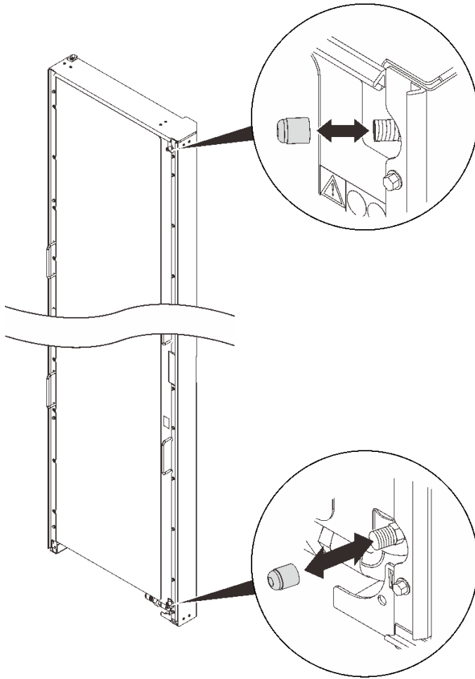
圖例 49. 安裝閘蓋
