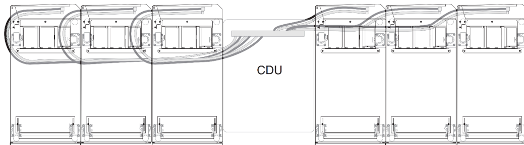
圖例 39. 在高架地板和非架起地板環境中佈線和固定軟管 (由上往下看)
