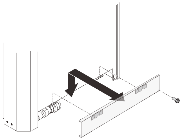
圖例 61. 卸下外軟管檢修面板
