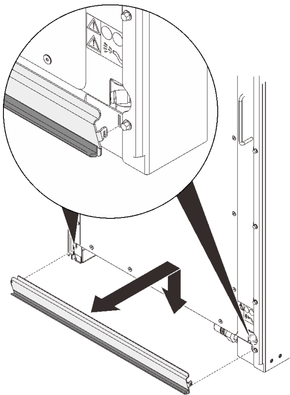
圖例 26. 卸下內部軟管檢修面板
