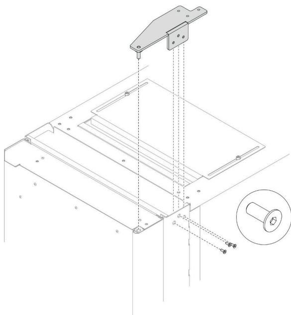
圖例 51. 卸下頂部鉸鏈
