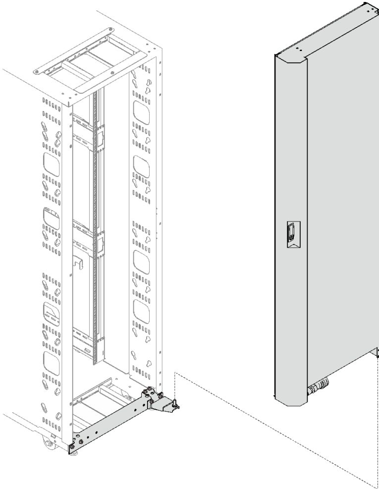
圖例 57. 將熱交換器安裝到機櫃
