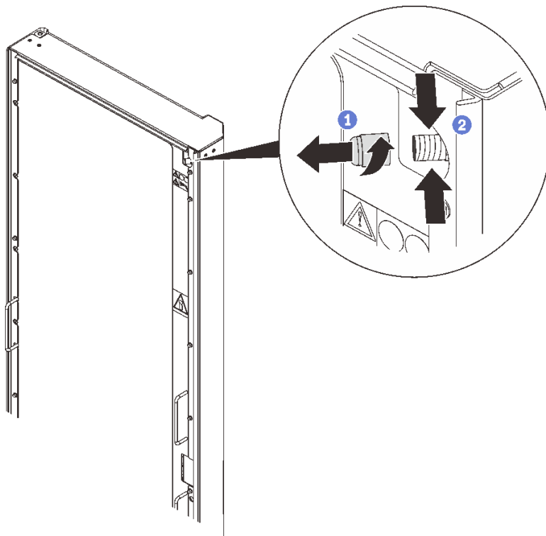
圖例 28. 吹掃氮氣
