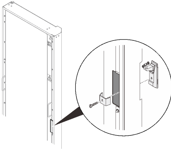
圖例 69. 更換門門
