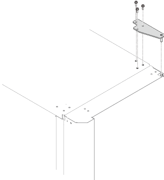
圖例 50. 卸下頂部鉸鏈
