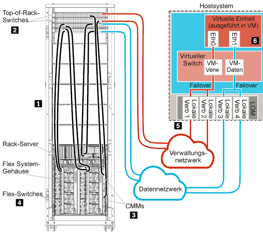
Abbildung 12. Beispiel: Topologie – Physisch getrenntes Daten- und Verwaltungsnetzwerk für eine virtuelle Einheit
