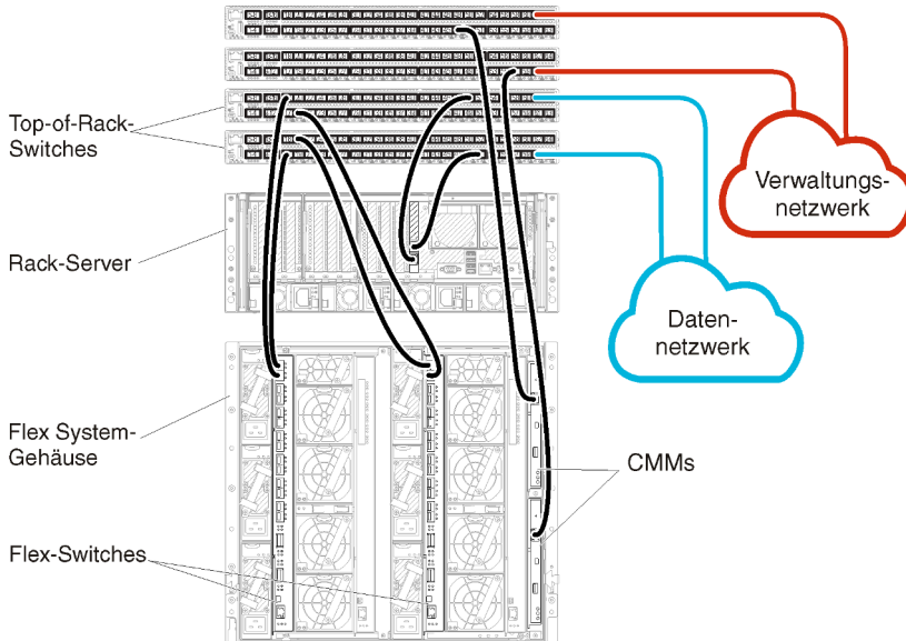
Abbildung 15. Beispiel: Verkabelung für physikalisch getrennte Daten- und Verwaltungsnetzwerke
