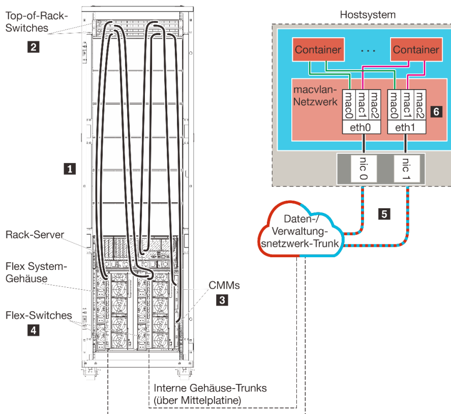
Abbildung 18. Beispiel: Topologie – Virtuell getrenntes Daten- und Verwaltungsnetzwerk für Container
