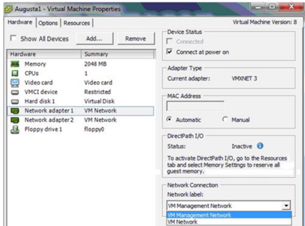
Abbildung 24. Konfiguration von Netzwerkadaptern
