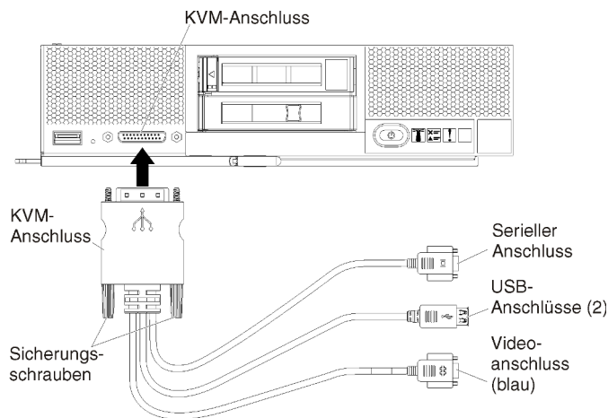
Abbildung 22. Konsolenverteilerkabel und Frontblende eines Servers
