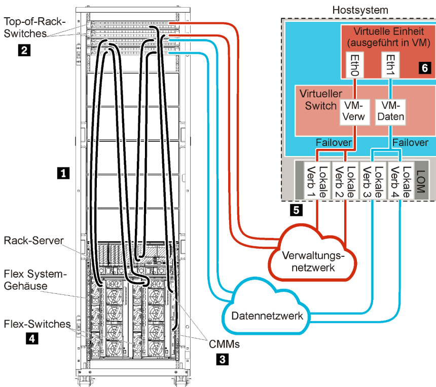
Abbildung 13. Beispiel: Topologie – Physisch getrenntes Daten- und Verwaltungsnetzwerk für eine virtuelle Einheit
