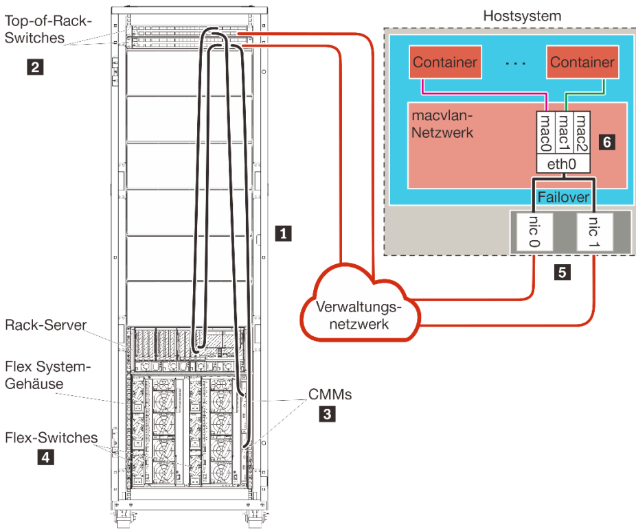
Abbildung 26. Beispiel: Topologie von Nur-Verwaltungsnetzwerken für Container
