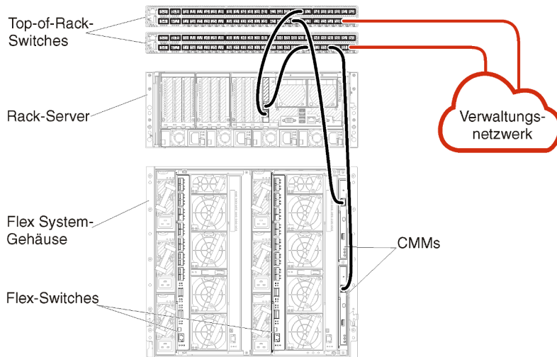
Abbildung 27. Beispiel: Verkabelung für Nur-Verwaltungsnetzwerke
