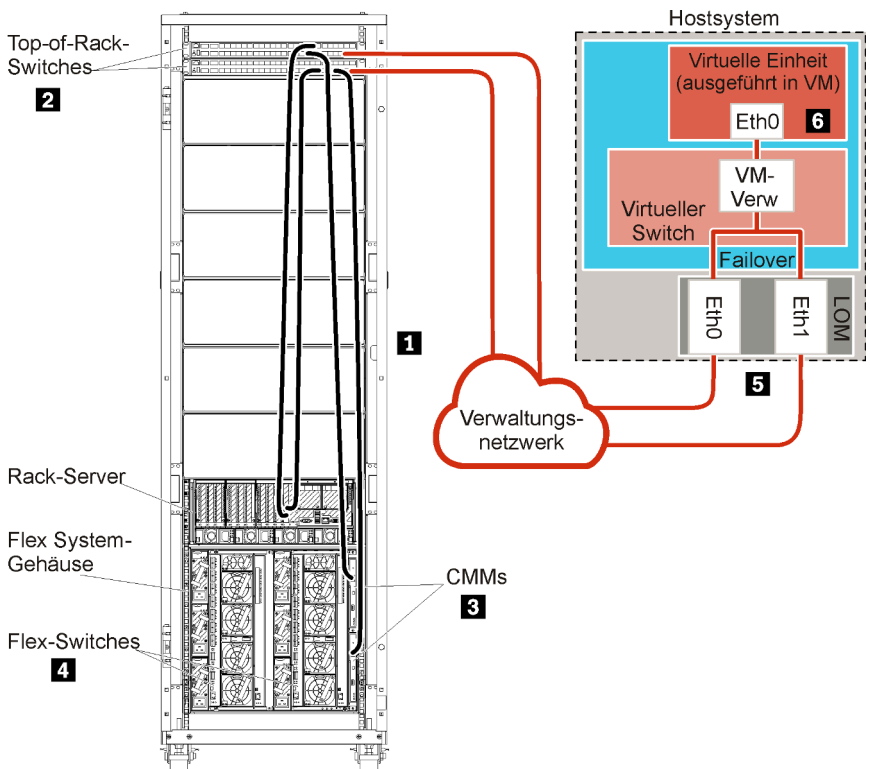
Abbildung 25. Beispiel: Topologie von Nur-Verwaltungsnetzwerken für eine virtuelle Einheit
