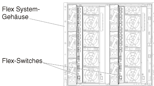
Abbildung 28. Flex-Switch-Positionen in einem Gehäuse
