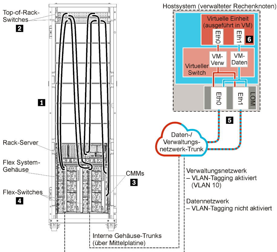
Abbildung 17. Beispiel: Topologie – Virtuell getrenntes Daten- und Verwaltetzwerk für eine virtuelle Einheit
