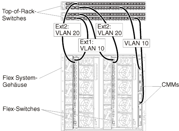
Abbildung 20. Beispiel: Konfiguration für Flex-Switches in logisch getrennten Daten- und Verwaltungsnetzwerken (Red Hat KVM) mit aktiviertem VLAN-Tagging in beiden Netzwerken
