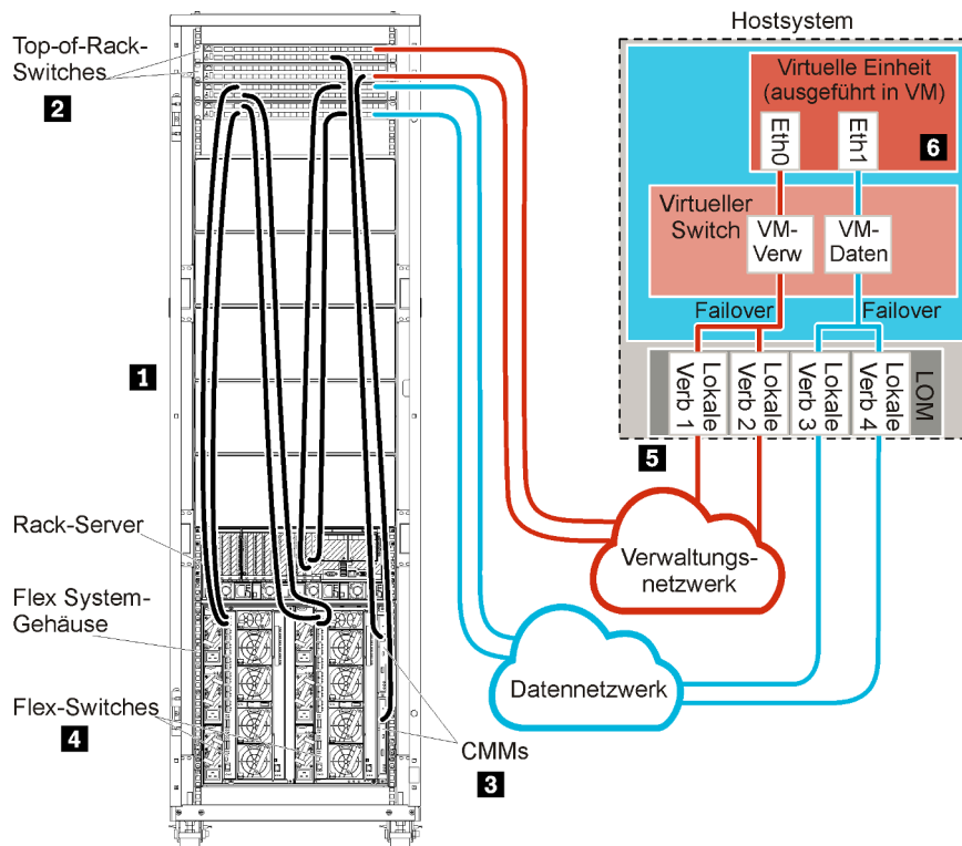
Abbildung 12. Beispiel: Topologie – Physisch getrenntes Daten- und Verwaltungsnetzwerk für eine virtuelle Einheit
