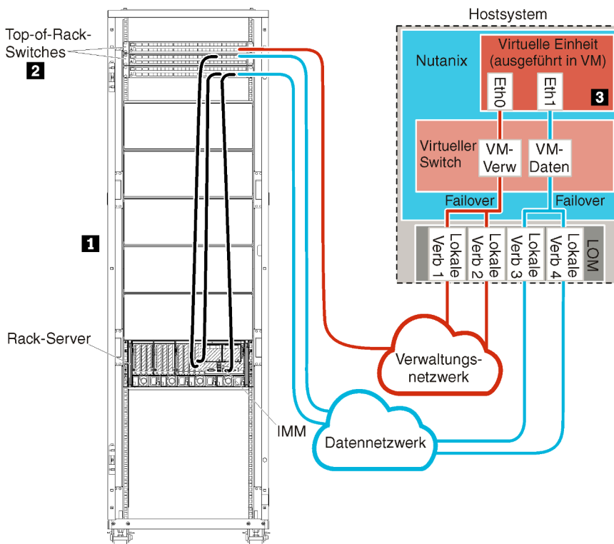
Abbildung 10. Beispiel: Netzwerktopologie – Physisch getrennte Daten- und Verwaltungsnetzwerke (Nutanix AHV)
