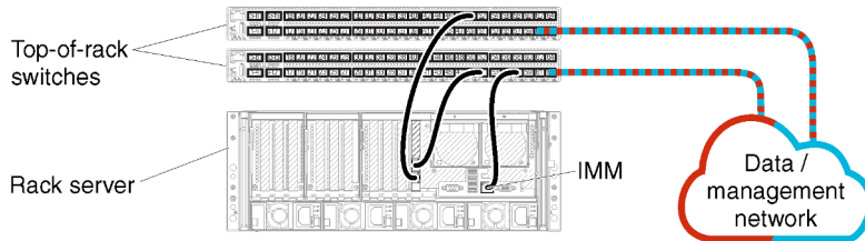
Abbildung 9. Beispiel: Verkabelung für Verwaltungsnetzwerke und Netzwerke mit einzelnen Daten
