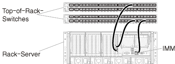
Abbildung 13. Beispiel: Verkabelung für logisch getrennte Daten- und Verwaltungsnetzwerke
