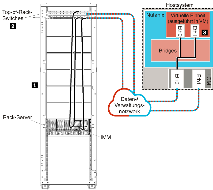
Abbildung 8. Beispiel: Topologie von Verwaltungsnetzwerken und Netzwerken mit einzelnen Daten (Nutanix AHV)
