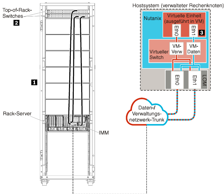
Abbildung 12. Beispiel: Netzwerktopologie – Logisch getrennte Daten- und Verwaltungsnetzwerke (Nutanix AHV)
