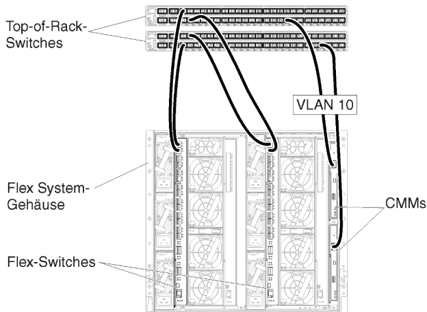
Abbildung 14. Beispiel: Konfiguration für Flex-Switches in logisch getrennten Daten- und Verwaltungsnetzwerken (KVM) mit aktiviertem VLAN-Tagging im Verwaltungsnetzwerk
