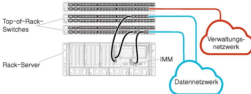
Abbildung 11. Beispiel: Verkabelung für physisch getrennte Daten- und Verwaltungsnetzwerke (VMware ESXi)
