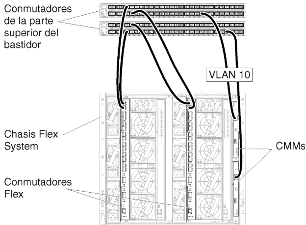
Figura 20. Ejemplo de configuración para Conmutadores Flex en redes de datos y gestión separadas virtualmente en las que el etiquetado VLAN está habilitado solo en la red de gestión
