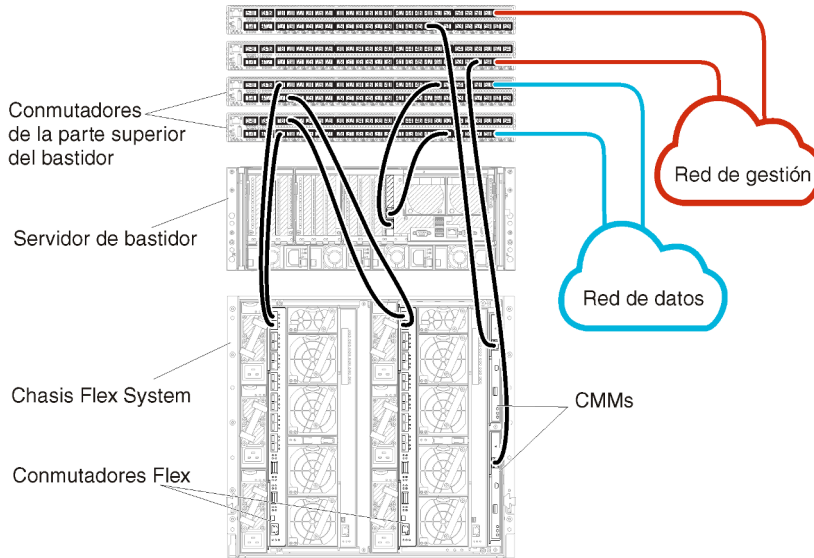
Figura 15. Ejemplo de cableado para redes de datos y de gestión separadas físicamente
