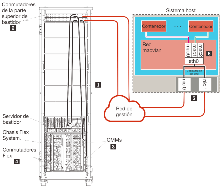
Figura 26. Ejemplo de topología de red de solo gestión para contenedores
