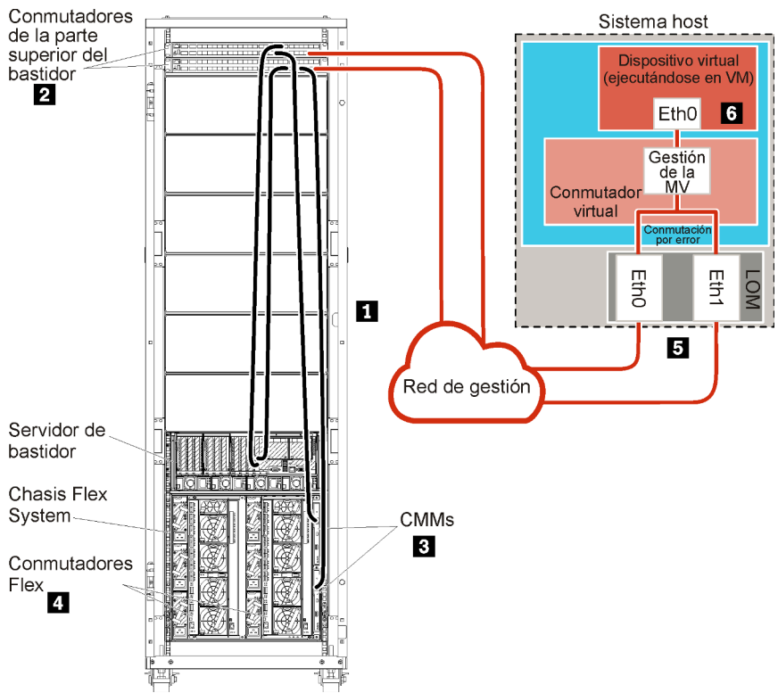
Figura 25. Ejemplo de topología de red de solo gestión para un dispositivo virtual
