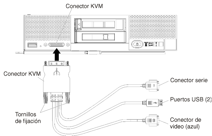
Figura 22. Cable multiconector de la consola y marco biselado frontal de un servidor
