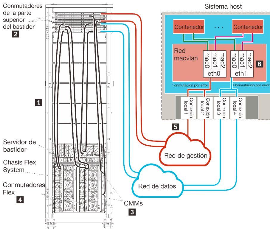
Figura 14. Ejemplo de datos separados físicamente y topología de red de administración para contenedores
