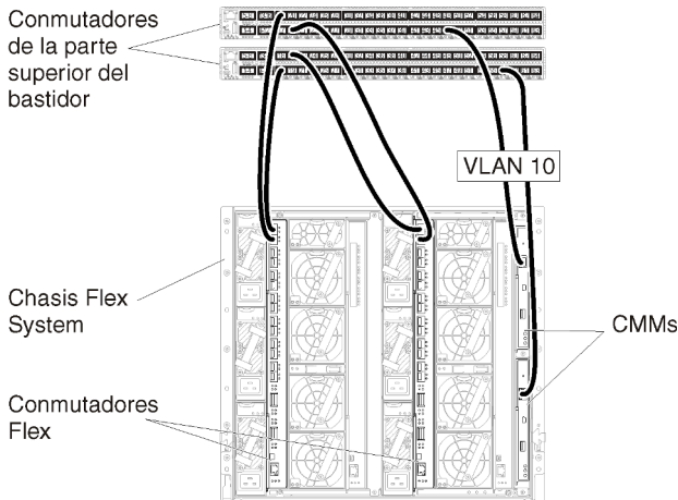
Figura 21. Ejemplo de configuración para Conmutadores Flex en redes de datos y gestión separadas virtualmente (VMware ESXi) en las que el etiquetado VLAN está habilitado solo en la red de gestión
