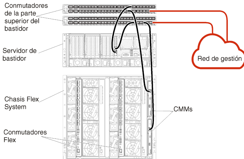
Figura 27. Ejemplo de cableado para una red de solo gestión
