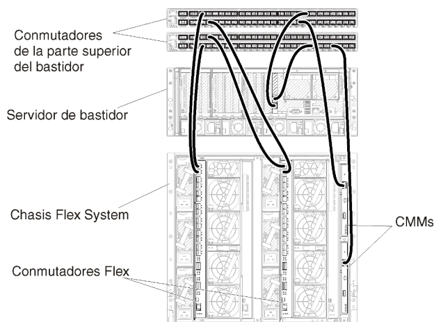
Figura 19. Ejemplo de cableado para redes de datos y de gestión separadas virtualmente
