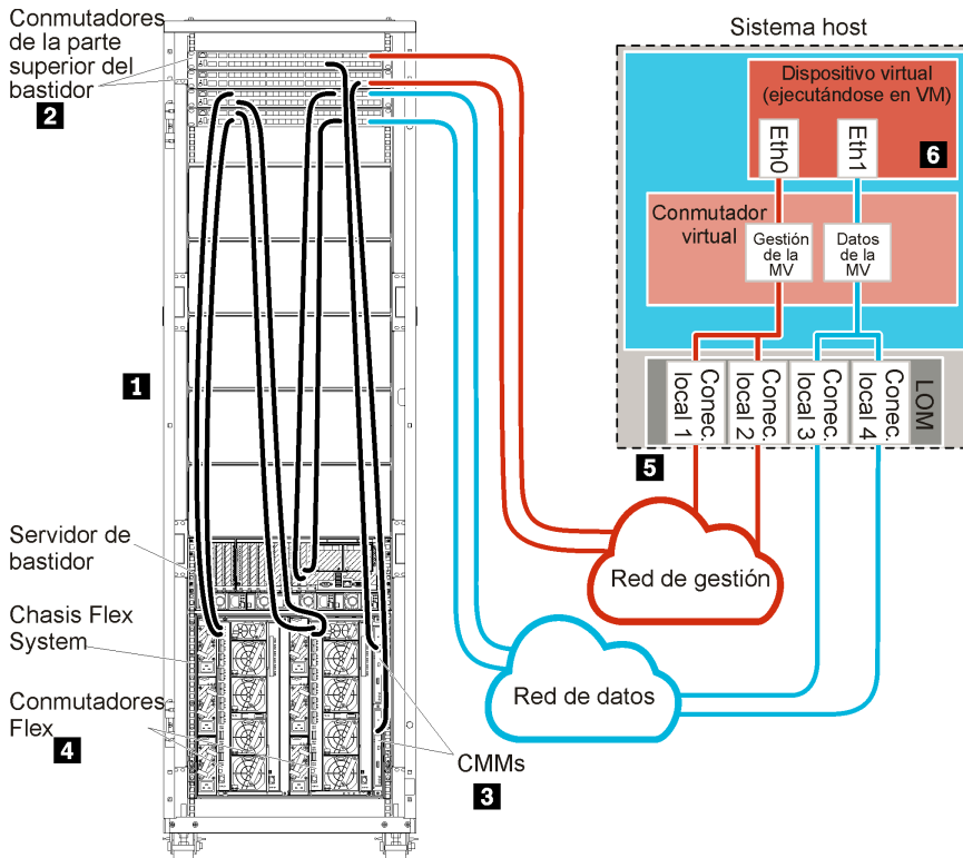
Figura 13. Ejemplo de datos separados físicamente y topología de red de administración para un dispositivo virtual
