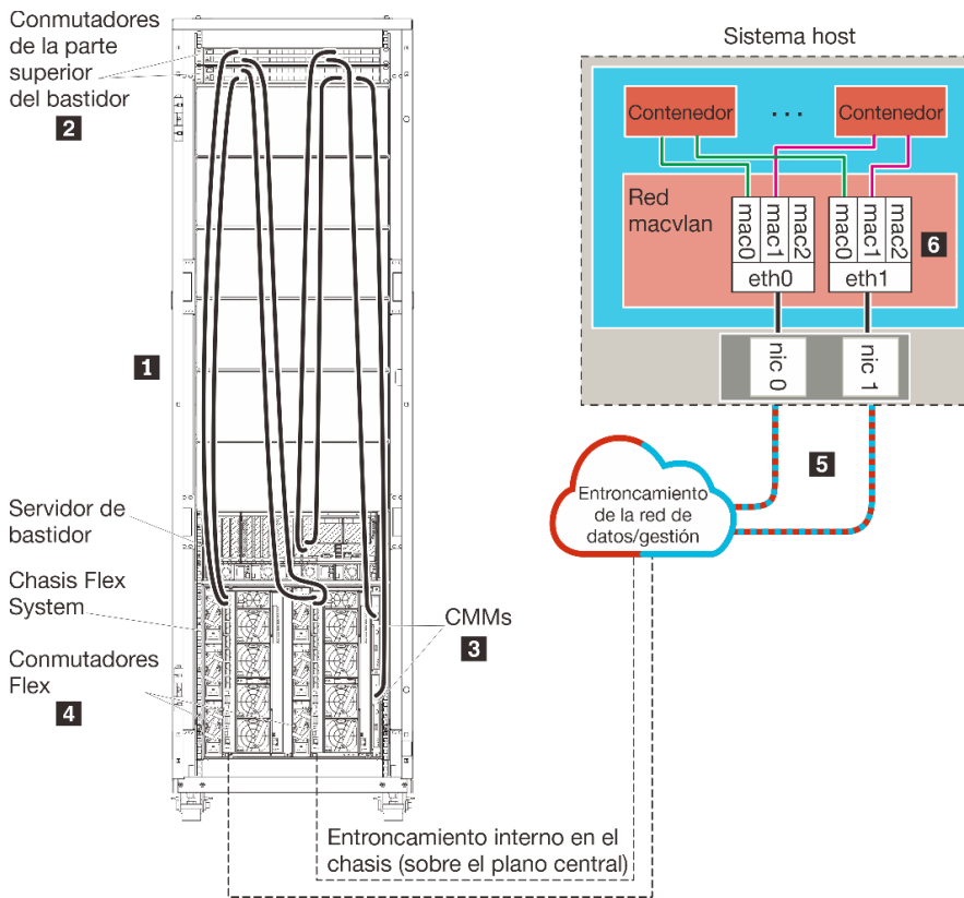
Figura 18. Ejemplo de datos separados virtualmente y topología de red de administración para contenedores
