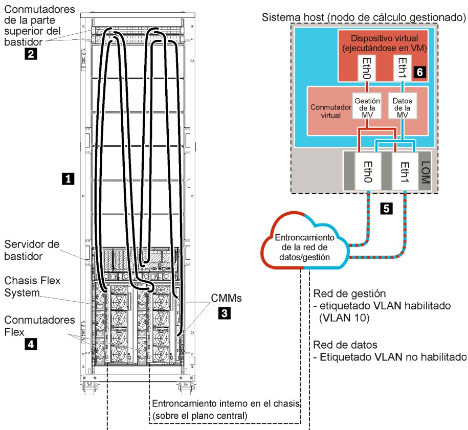
Figura 17. Ejemplo de datos separados virtualmente y topología de red de administración para un dispositivo virtual
