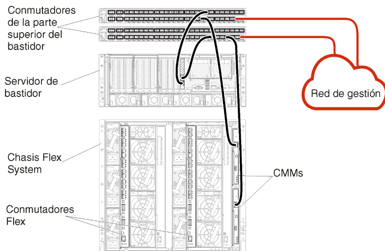
Figura 25. Ejemplo de cableado para una red de solo gestión
