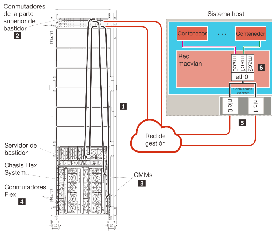
Figura 24. Ejemplo de topología de red de solo gestión para contenedores
