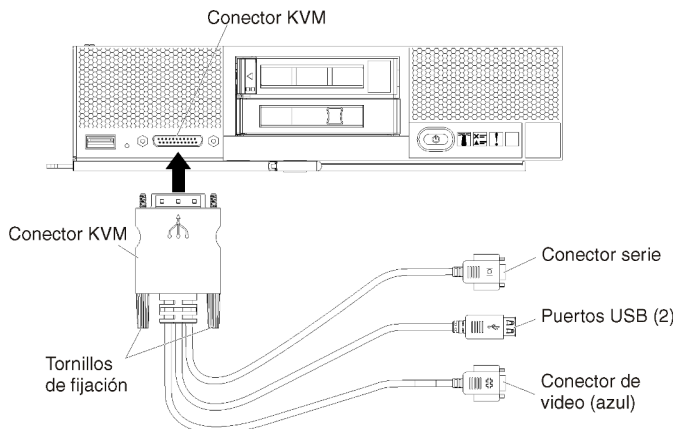
Figura 21. Cable multiconector de la consola y marco biselado frontal de un servidor
