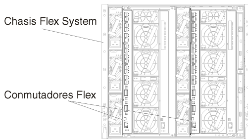
Figura 26. Ubicaciones de los Conmutador Flex en un chasis
