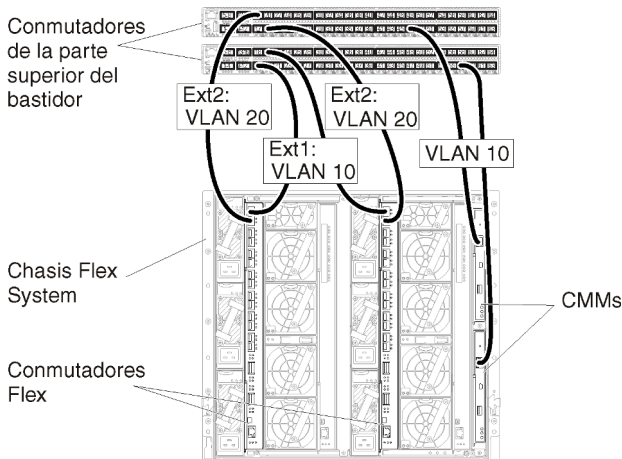
Figura 20. Ejemplo de configuración de Conmutadores Flex en redes de datos y de gestión virtualmente separadas (VMware ESXi) en la que el etiquetado de la VLAN está habilitado en ambas redes
