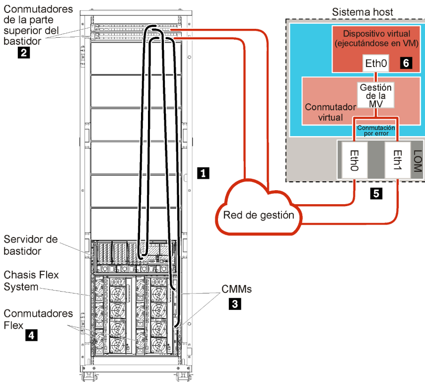
Figura 23. Ejemplo de topología de red de solo gestión para un dispositivo virtual
