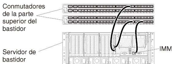
Figura 13. Ejemplo de cableado para redes de datos y de gestión separadas virtualmente
