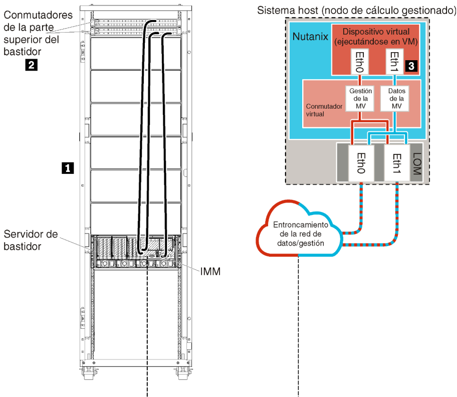
Figura 12. Topología de red de ejemplo: redes de datos y de gestión separadas virtualmente (Nutanix AHV)
