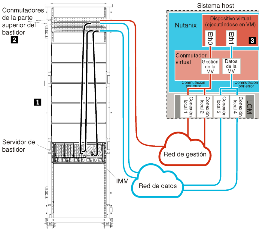
Figura 10. Topología de red de ejemplo: redes de datos y de gestión separadas físicamente (Nutanix AHV)
