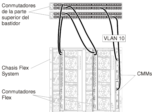
Figura 14. Ejemplo de configuración para Conmutadores Flex en redes de datos y gestión separadas virtualmente (KVM) en las que el etiquetado VLAN está habilitado solo en la red de gestión
