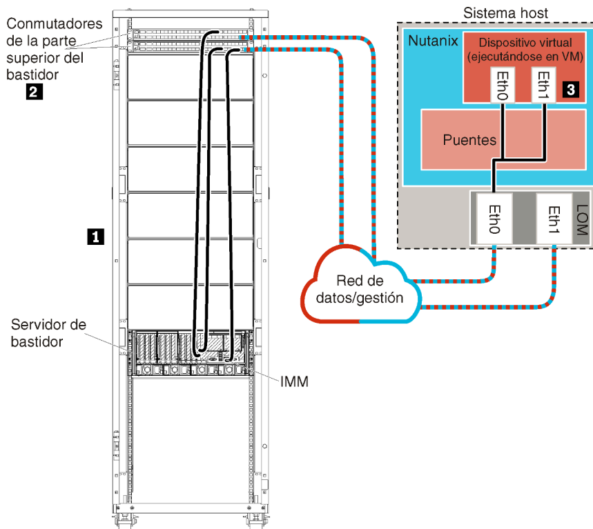
Figura 8. Ejemplo de topología de una red de datos únicos y de gestión (Nutanix AHV)
