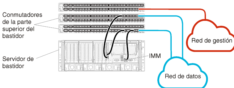
Figura 11. Ejemplo de cableado para redes de datos y de gestión separadas físicamente (VMware ESXi)
