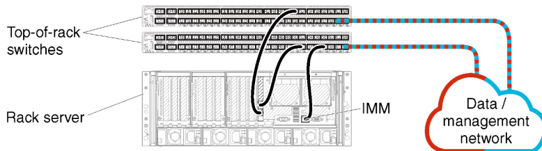
Figura 9. Ejemplo de cableado para una sola red de datos y gestión
