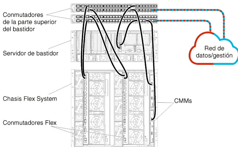
Figura 10. Ejemplo de cableado para una sola red de datos y gestión
