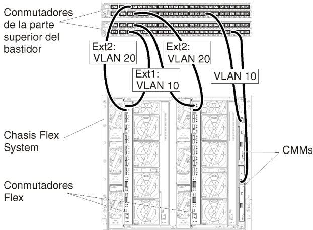
Figura 20. Ejemplo de configuración de Conmutadores Flex en redes de datos y de gestión virtualmente separadas (Red Hat KVM) donde el etiquetado de la VLAN está habilitado en ambas redes
