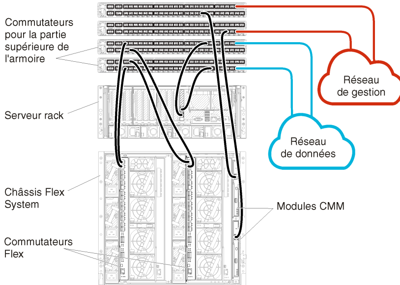
Figure 14. Exemple de câblage pour les réseaux de gestion et de données séparés physiquement
