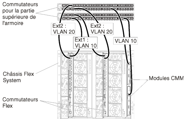
Figure 20. Exemple de configuration pour Commutateurs Flex sur des réseaux de données séparées virtuellement et de gestion (Red Hat KVM) dans lesquels le marquage VLAN est activé sur les deux réseaux
