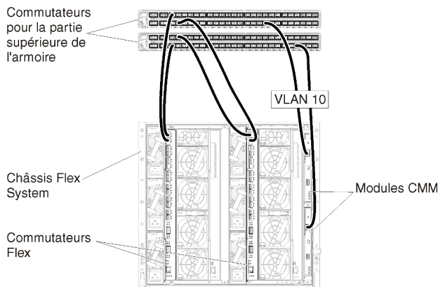
Figure 19. Exemple de configuration pour Commutateurs Flex sur des réseaux de données séparés virtuellement et de gestion (VMware ESXi) dans lesquels le marquage VLAN est activé sur le réseau de gestion.
