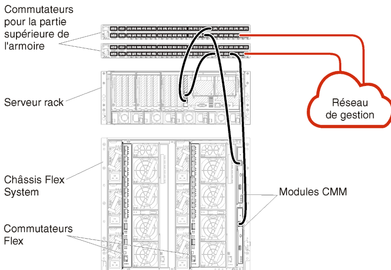
Figure 27. Exemple de câblage pour un réseau de gestion uniquement
