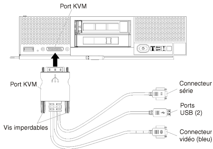
Figure 22. Câble d'interface de console et panneau frontal d'un serveur
