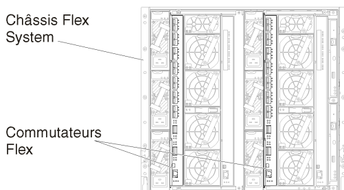
Figure 28. Emplacements Commutateur Flex dans un châssis
