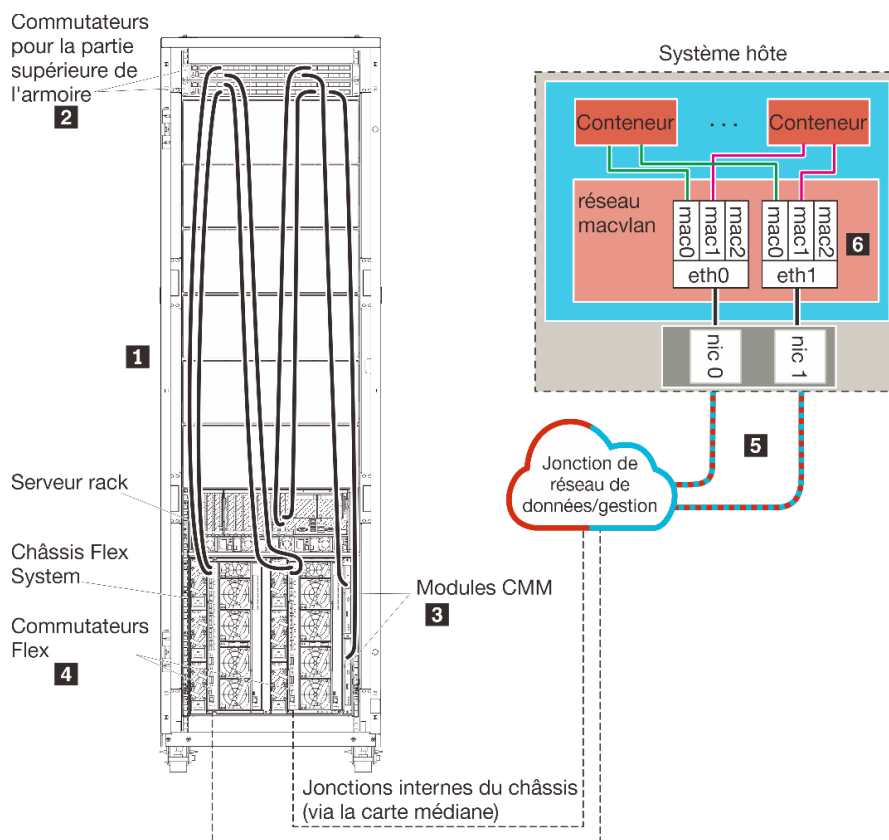
Figure 18. Exemple de données séparées virtuellement et de topologie du réseau de gestion pour les conteneurs
