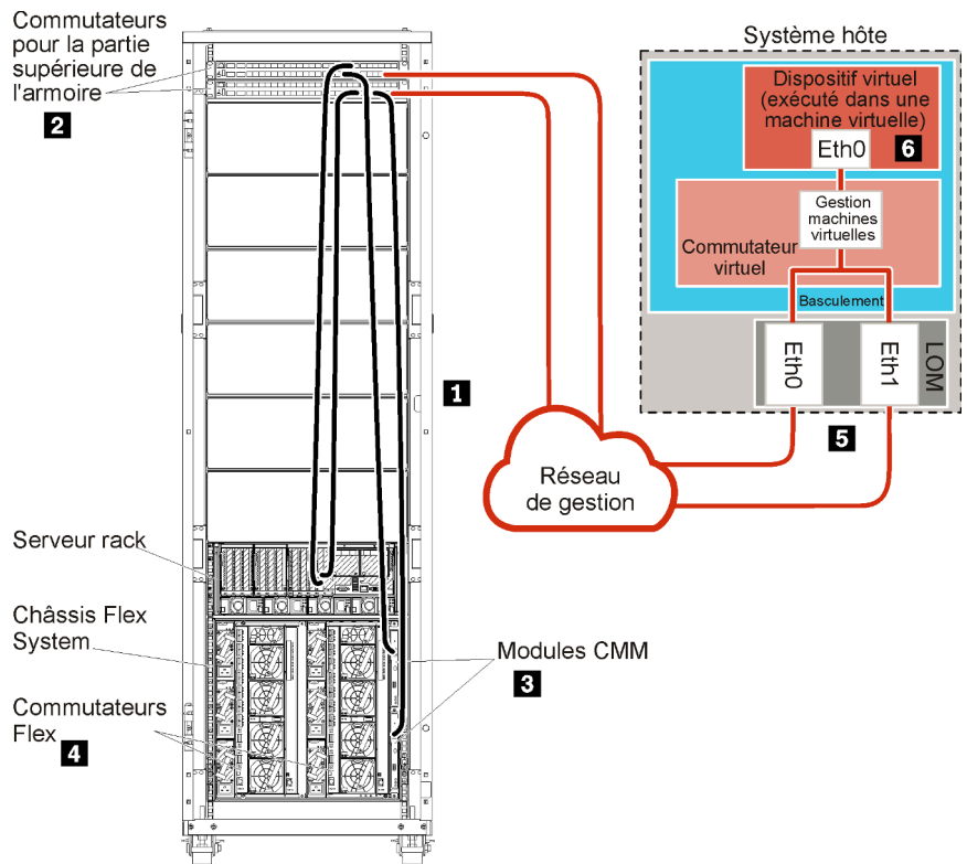
Figure 25. Exemple de topologie du réseau de gestion uniquement pour un dispositif virtuel
