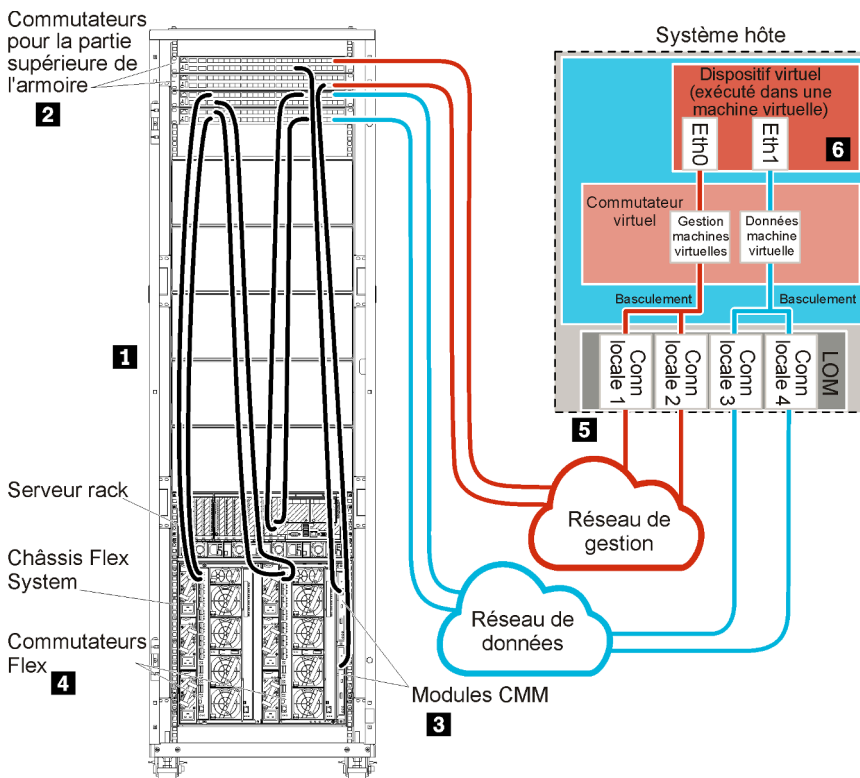
Figure 13. Exemple de données séparées physiquement et de topologie du réseau de gestion pour un dispositif virtuel
