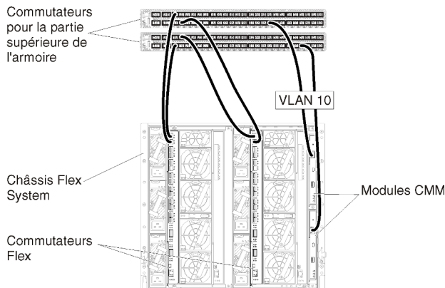
Figure 21. Exemple de configuration pour Commutateurs Flex sur des réseaux de données séparés virtuellement et de gestion (VMware ESXi) dans lesquels le marquage VLAN est activé sur le réseau de gestion.
