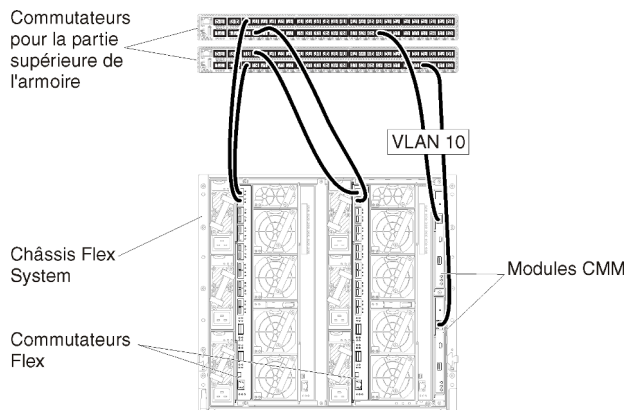
Figure 20. Exemple de configuration pour Commutateurs Flex sur des réseaux de données séparés virtuellement et de gestion (VMware ESXi) dans lesquels le marquage VLAN est activé sur le réseau de gestion.
