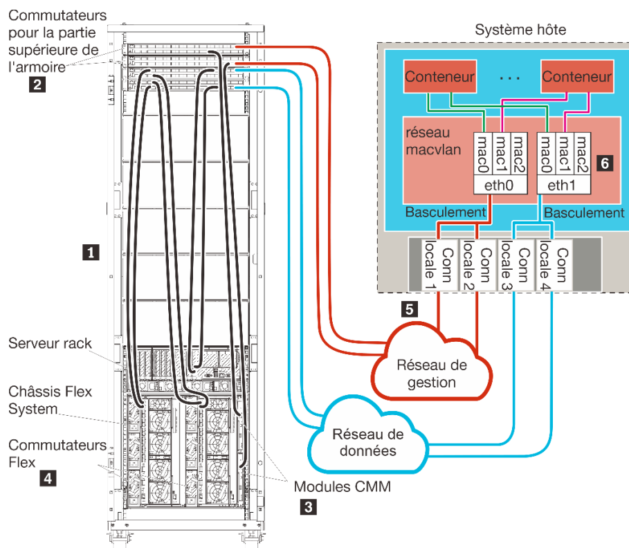
Figure 14. Exemple de données séparées physiquement et de topologie du réseau de gestion pour les conteneurs
