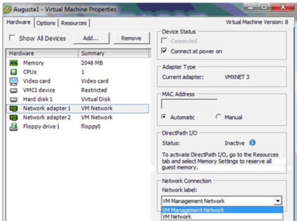
Figure 24. Configuration de la carte réseau
