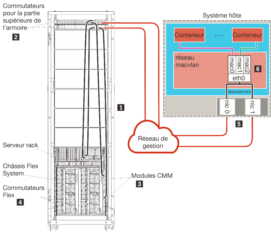
Figure 26. Exemple de topologie du réseau de gestion uniquement pour les conteneurs
