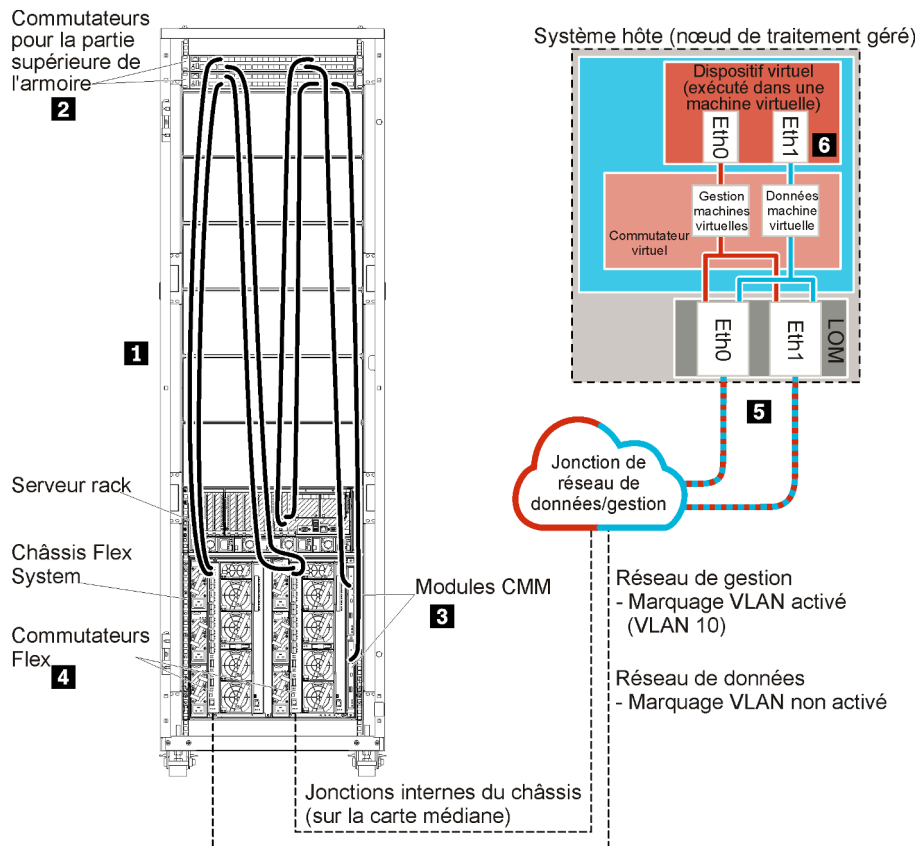
Figure 17. Exemple de données séparées virtuellement et de topologie du réseau de gestion pour un dispositif virtuel
