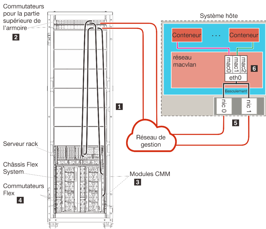
Figure 24. Exemple de topologie du réseau de gestion uniquement pour les conteneurs
