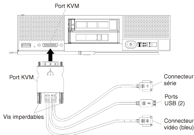
Figure 21. Câble d'interface de console et panneau frontal d'un serveur
