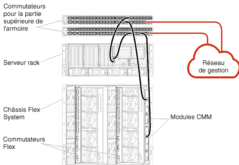
Figure 25. Exemple de câblage pour un réseau de gestion uniquement
