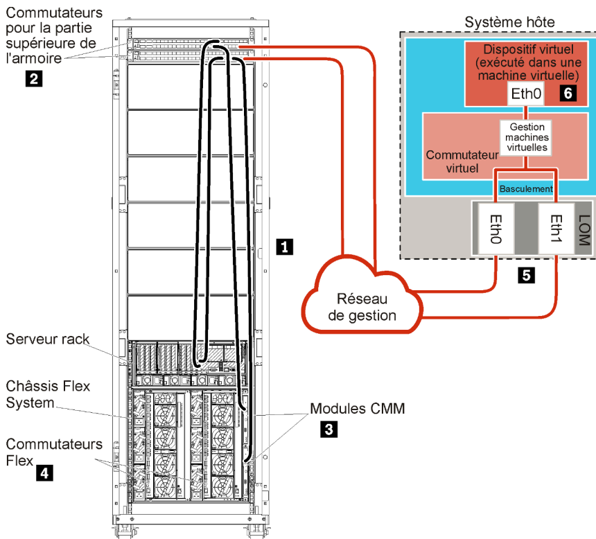
Figure 23. Exemple de topologie du réseau de gestion uniquement pour un dispositif virtuel
