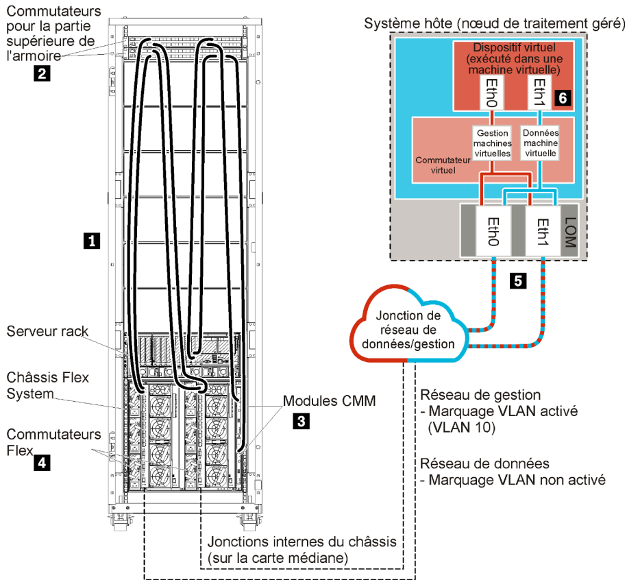
Figure 16. Exemple de données séparées virtuellement et de topologie du réseau de gestion pour un dispositif virtuel
