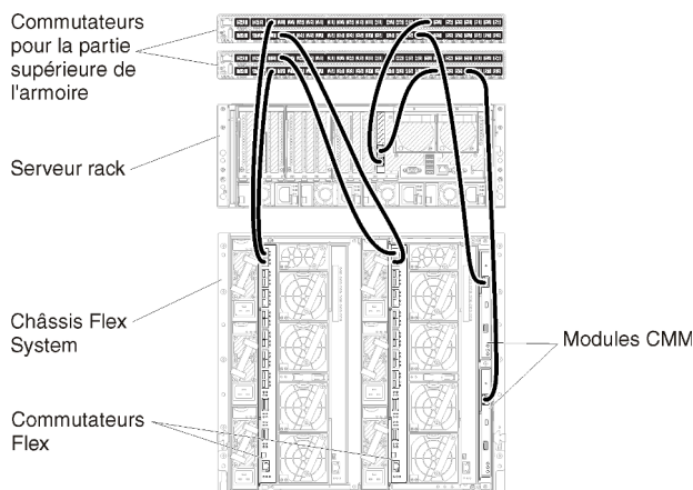
Figure 18. Exemple de câblage pour les réseaux de données séparés virtuellement et de gestion
