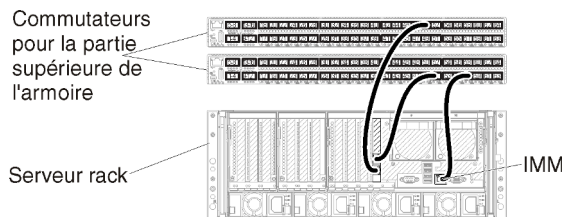
Figure 13. Exemple de câblage pour les réseaux de données séparés virtuellement et de gestion
