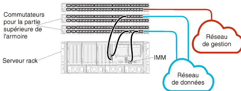
Figure 11. Exemple de câblage pour les réseaux de gestion et de données séparés physiquement (VMware ESXi)
