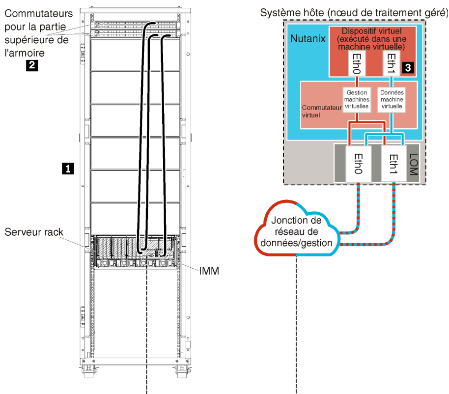
Figure 12. Exemple de topologie de réseau - Réseau de données séparées virtuellement et de gestion (Nutanix AHV)
