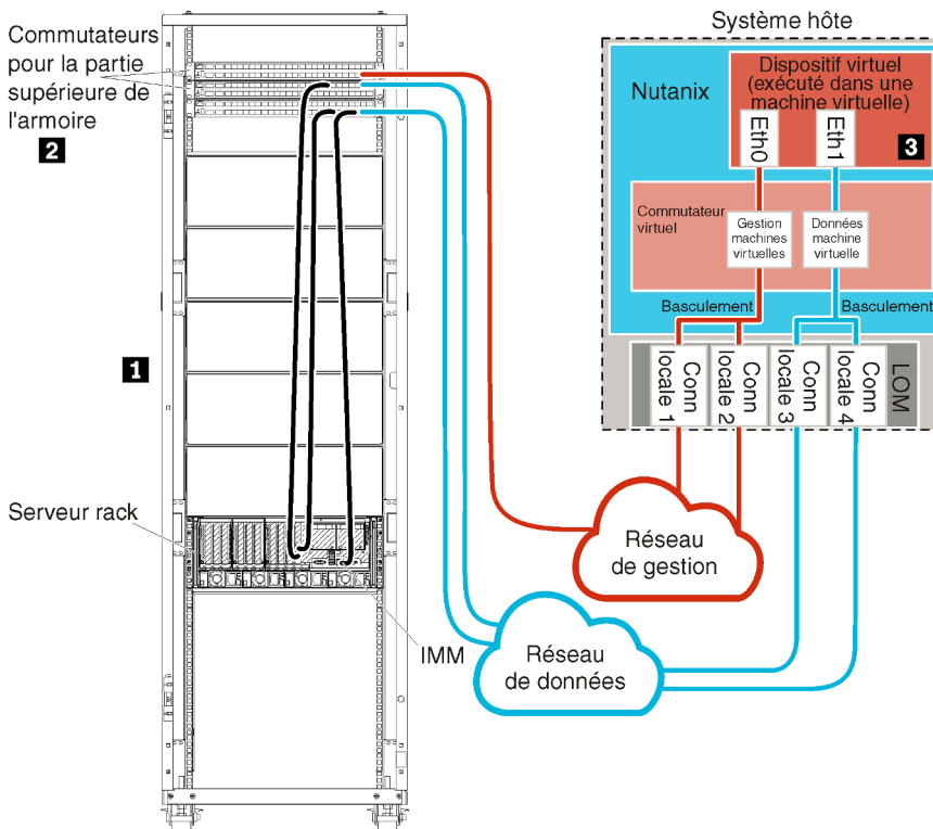
Figure 10. Exemple de topologie de réseau - Données séparées physiquement et réseau de gestion (Nutanix AHV)
