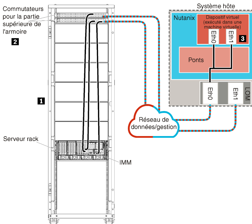
Figure 8. Exemple de topologie du réseau de donnée unique et de gestion (Nutanix AHV)
