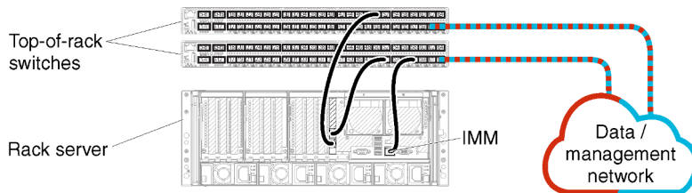
Figure 9. Exemple de câblage pour un réseau de donnée unique et de gestion
