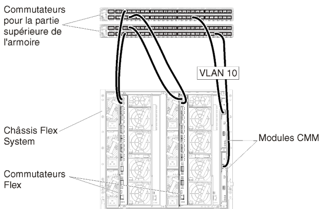
Figure 14. Exemple de configuration pour Commutateurs Flex sur des réseaux de données séparées virtuellement et de gestion (KVM) dans lesquels le marquage VLAN est activé sur le réseau de gestion.
