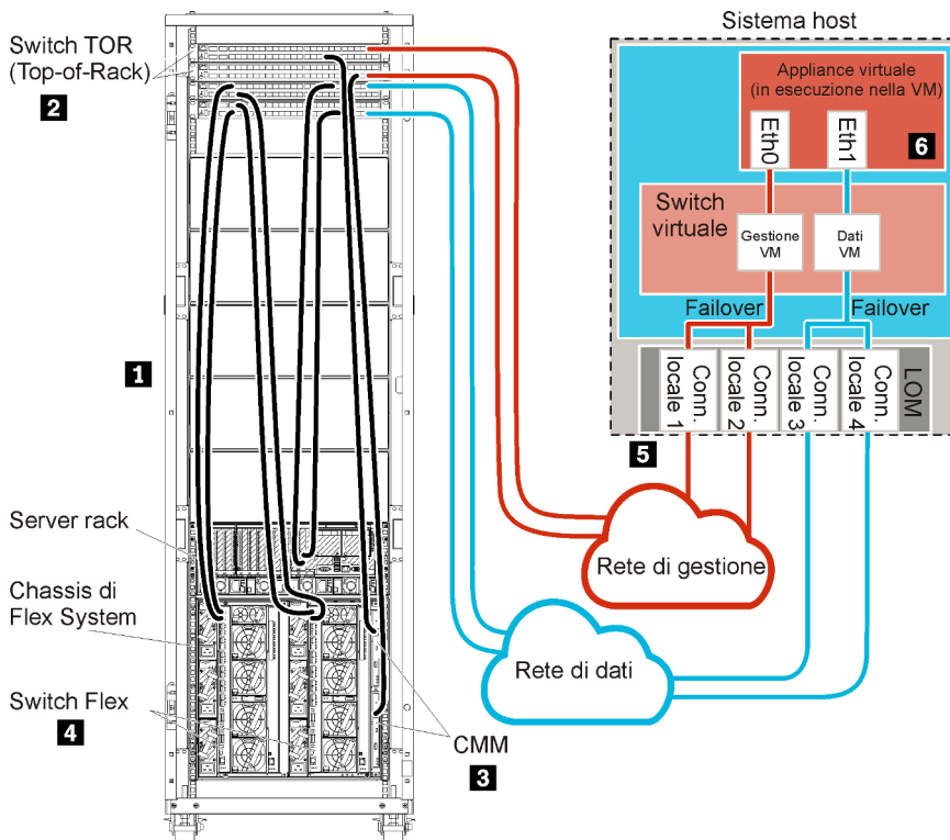
Figura 12. Esempio di topologia della rete di gestione e di dati separate fisicamente per un'appliance virtuale
