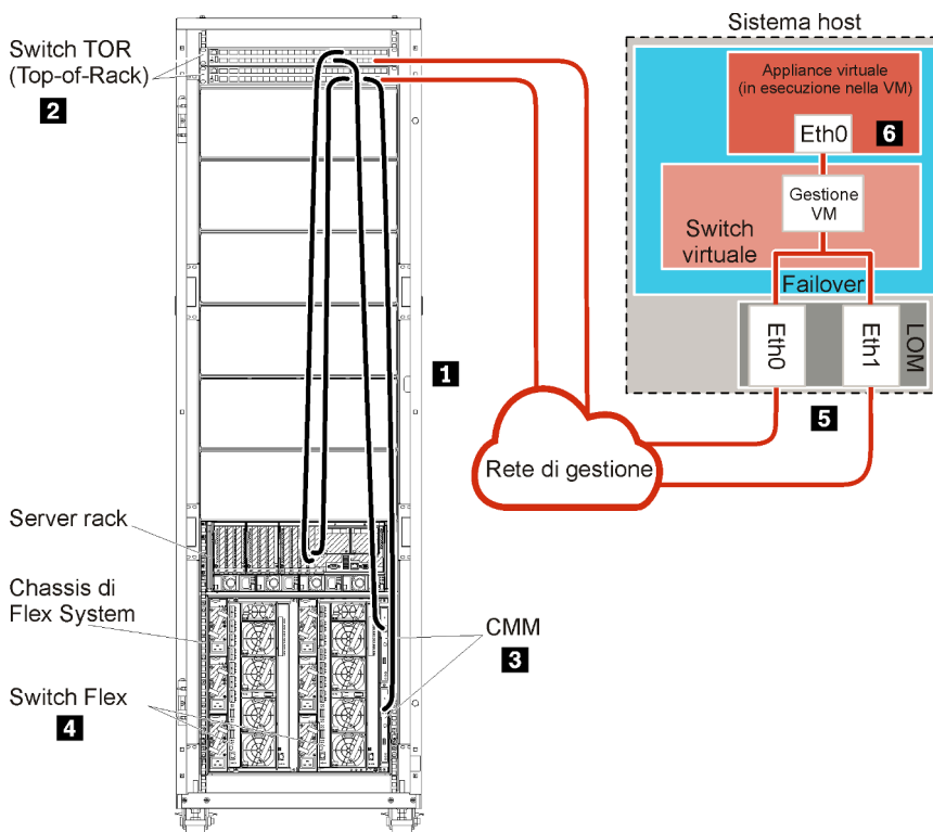
Figura 21. Esempio di topologia di rete di sola gestione per un'appliance virtuale
