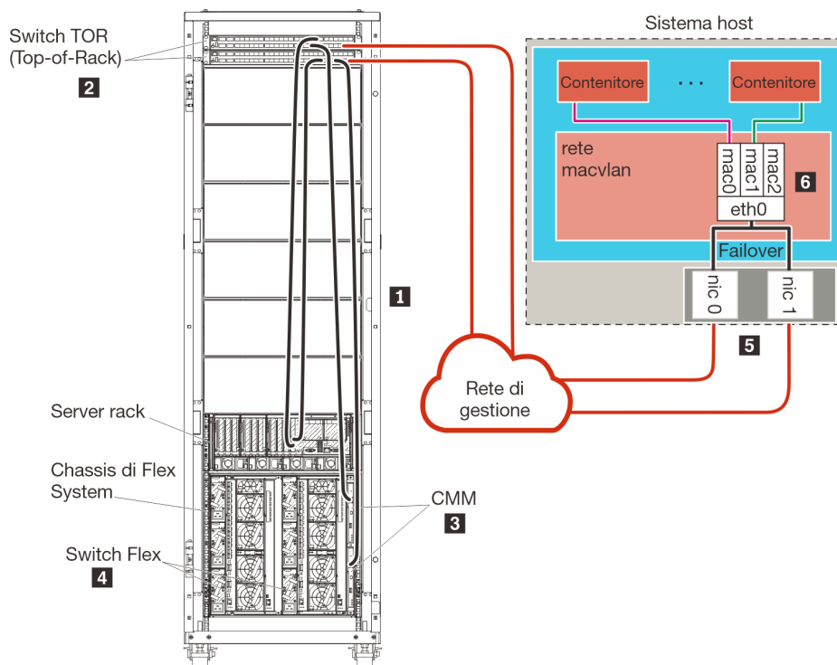
Figura 22. Esempio di topologia della rete di sola gestione per i contenitori
