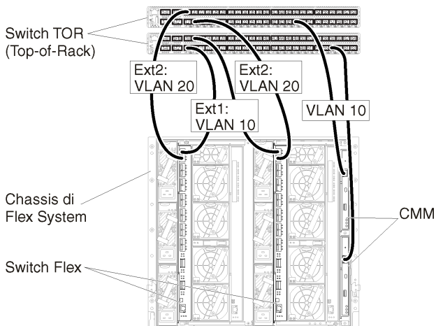
Figura 20. Configurazione di esempio per Switch Flex in reti virtualmente separate di dati e gestione (Red Hat KVM) in cui l'etichettatura VLAN è abilitata in entrambe le reti
