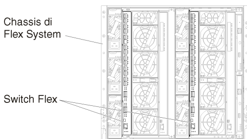
Figura 15. Posizioni degli Switch Flex in uno chassis
