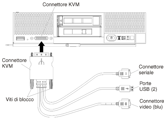
Figura 22. Cavo di ripartizione della console e mascherina anteriore di un server
