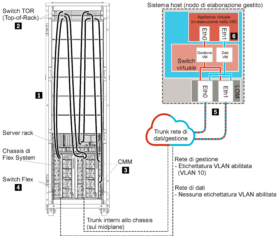
Figura 17. Esempio di topologia della rete di gestione e di dati separati virtualmente per un'appliance virtuale
