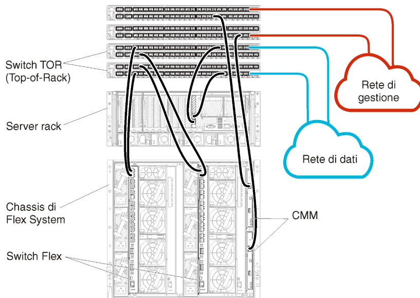
Figura 15. Esempio di cablaggio per reti fisicamente separate di dati e gestione
