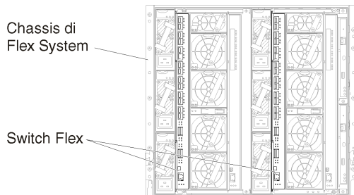
Figura 16. Posizioni degli Switch Flex in uno chassis
