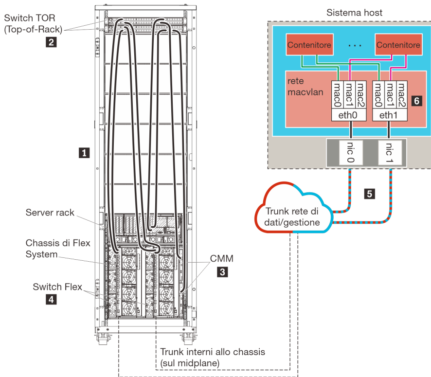
Figura 18. Esempio di topologia della rete di gestione e di dati separati virtualmente per i contenitori
