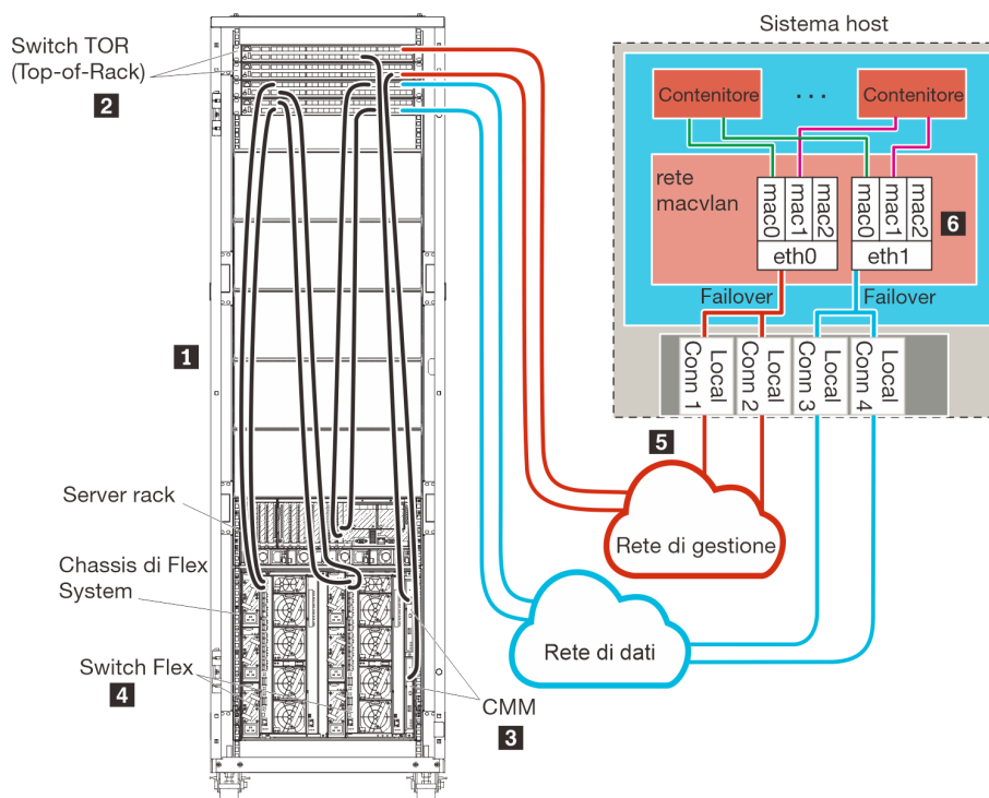
Figura 14. Esempio di topologia della rete di gestione e di dati separate fisicamente per i contenitori
