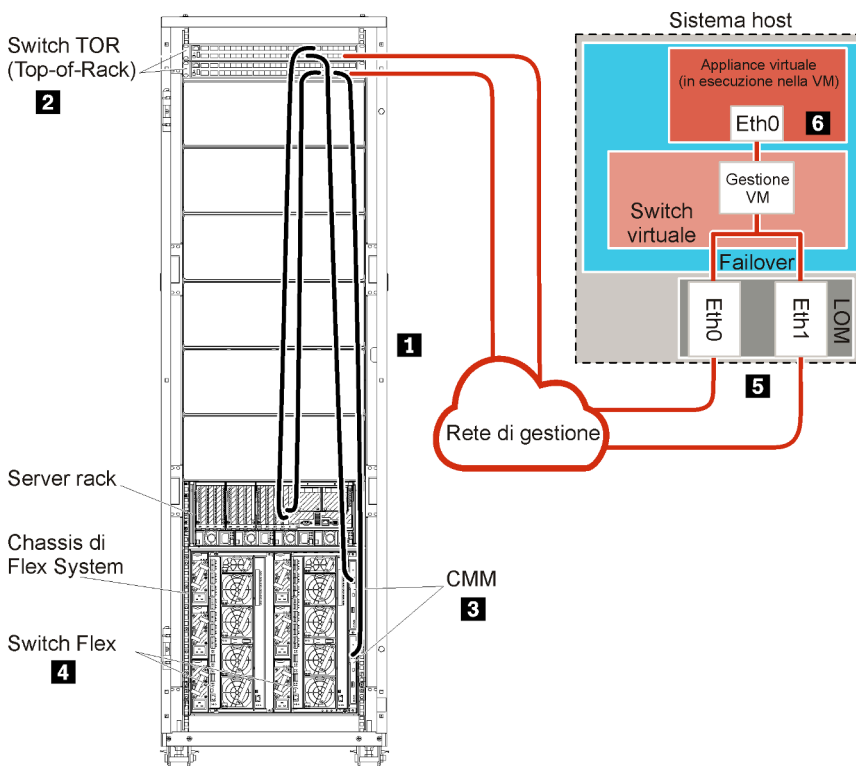
Figura 23. Esempio di topologia di rete di sola gestione per un'appliance virtuale
