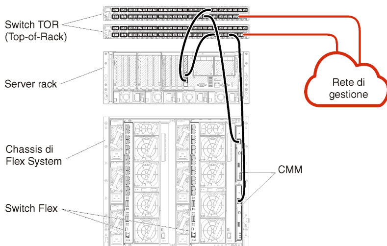
Figura 25. Esempio di cablaggio per una rete di sola gestione
