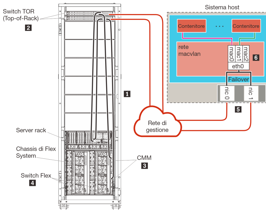
Figura 24. Esempio di topologia della rete di sola gestione per i contenitori
