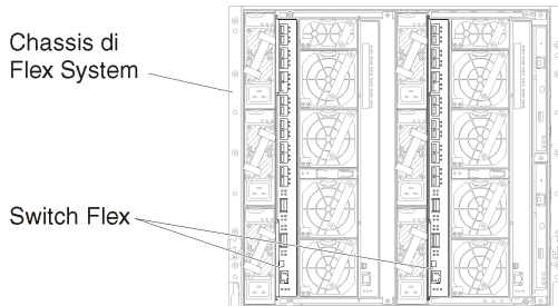
Figura 26. Posizioni degli Switch Flex in uno chassis
