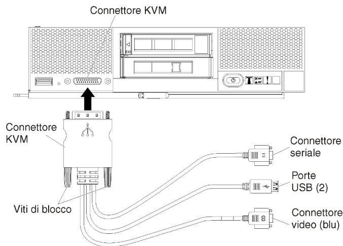
Figura 21. Cavo di ripartizione della console e mascherina anteriore di un server
