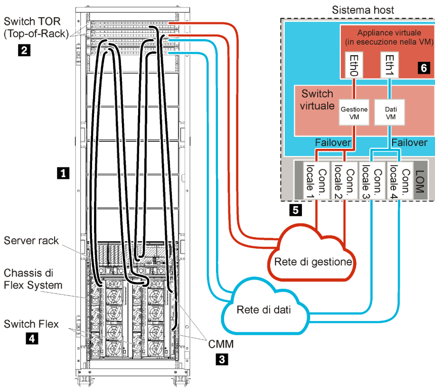
Figura 12. Esempio di topologia della rete di gestione e di dati separati fisicamente per un'appliance virtuale
