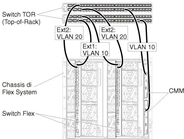
Figura 20. Configurazione di esempio per Switch Flex in reti virtualmente separate di dati e gestione (VMware ESXi) in cui l'etichettatura VLAN è abilitata in entrambe le reti
