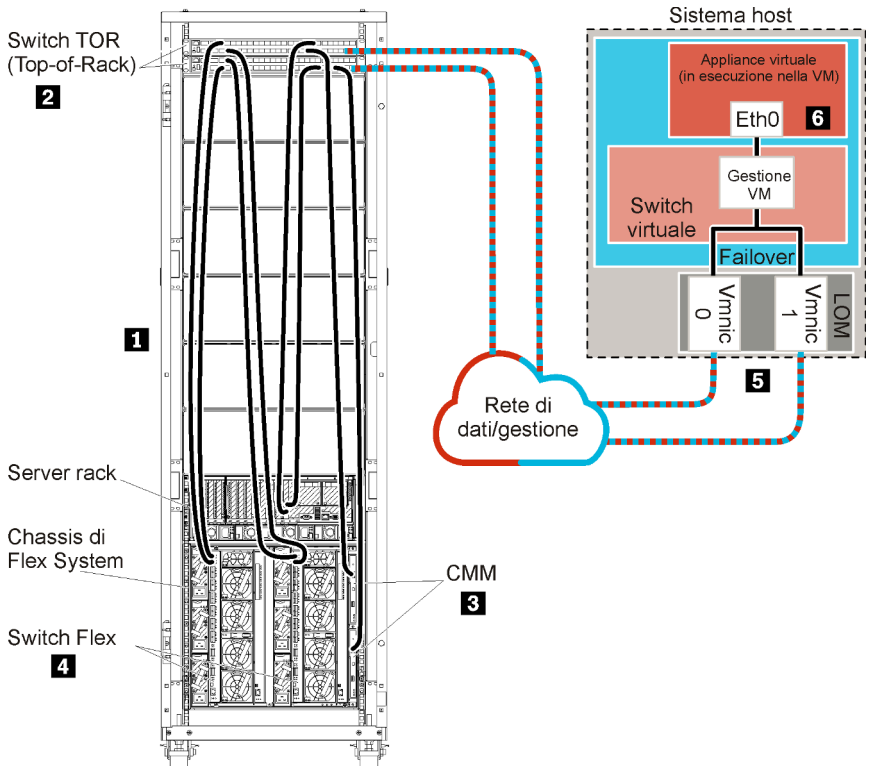
Figura 8. Esempio di topologia della rete di gestione e di dati Single per un'appliance virtuale
