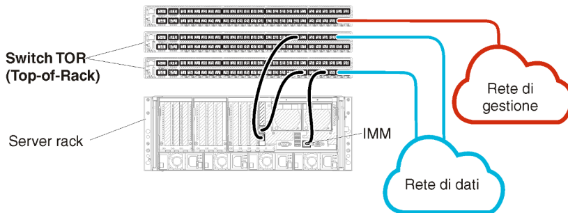
Figura 11. Esempio di cablaggio per reti fisicamente separate di dati e gestione (VMware ESXi)
