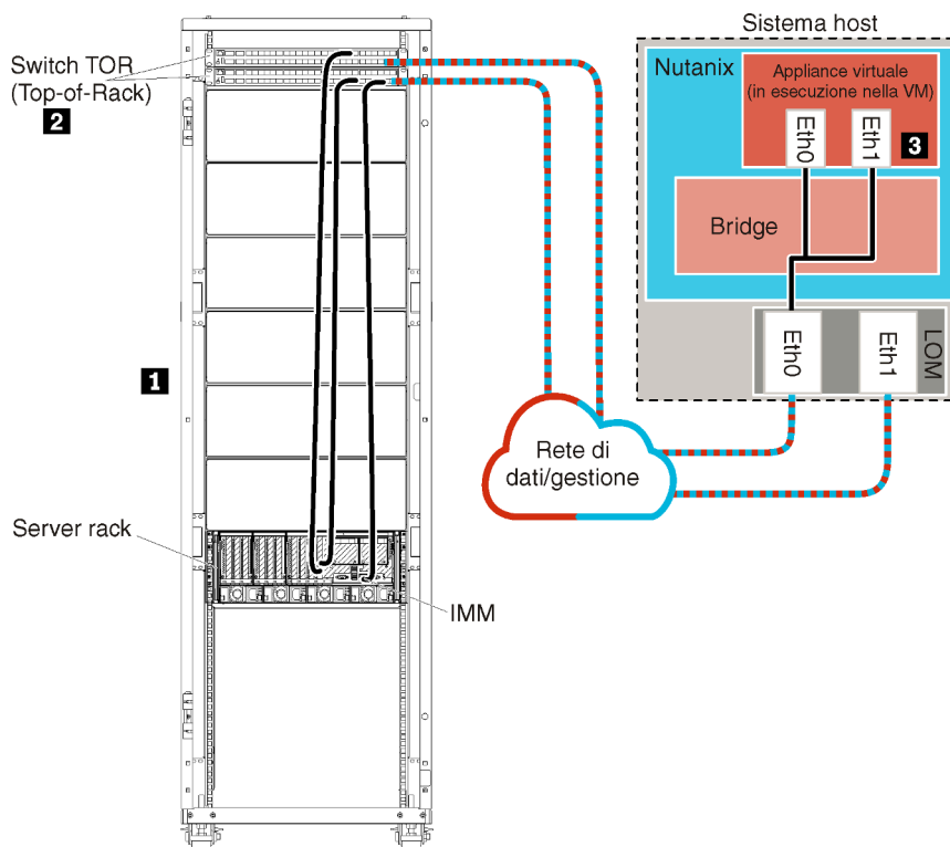
Figura 8. Esempio di topologia di rete singola di dati e gestione (Nutanix AHV)
