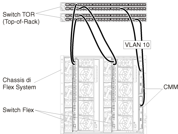
Figura 14. Configurazione di esempio per Switch Flex in reti virtualmente separate di dati e gestione (KVM) in cui l'etichettatura VLAN è abilitata nella rete di gestione
