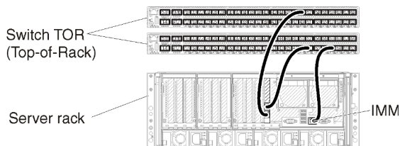
Figura 13. Esempio di cablaggio per reti virtualmente separate di dati e gestione
