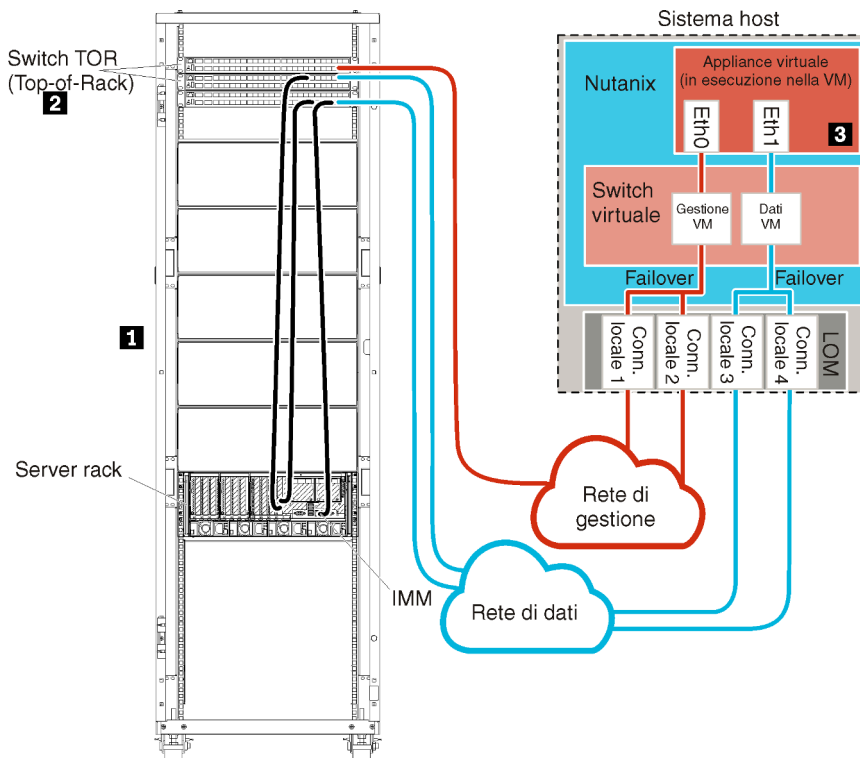
Figura 10. Esempio di topologia di rete - Rete fisicamente separata di dati e gestione (Nutanix AHV)
