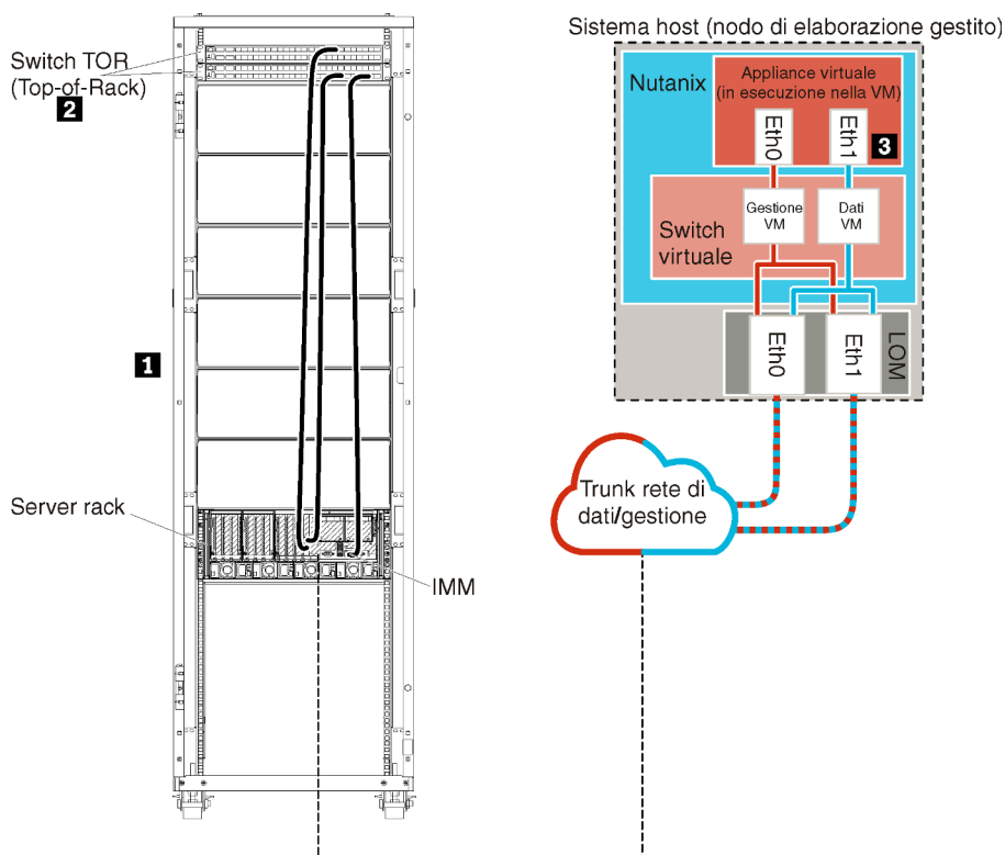
Figura 12. Esempio di topologia di rete - Rete virtualmente separata di dati e gestione (Nutanix AHV)
