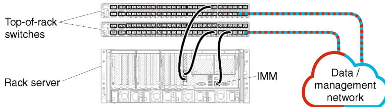
Figura 9. Esempio di cablaggio per una rete singola di dati e gestione
