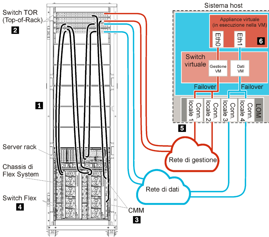
Figura 12. Esempio di topologia della rete di gestione e di dati separate fisicamente per un'appliance virtuale
