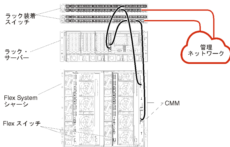
図 27. 管理専用ネットワークの配線の例
