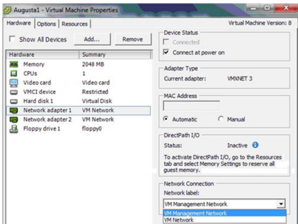
図 29. ネットワーク・アダプターの構成
