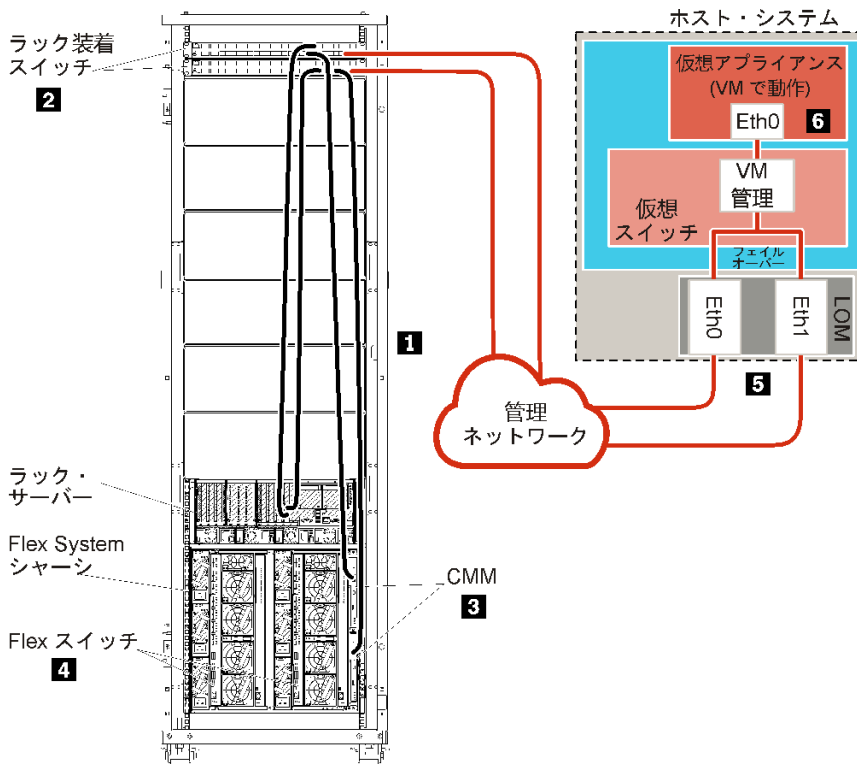
図 25. 仮想アプライアンスの管理専用ネットワーク・トポロジーの例
