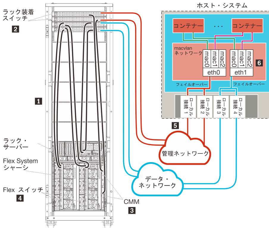
図 14. コンテナの物理的に分離したデータ/管理ネットワーク・トポロジーの例
