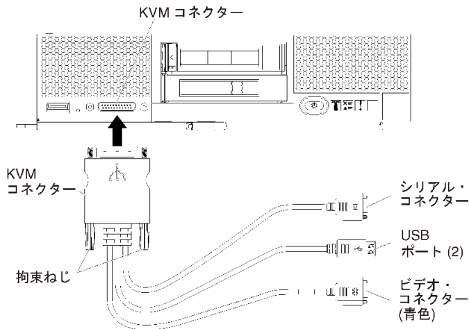
図 22. コンソールの分岐ケーブルとサーバーの前面ベゼル
