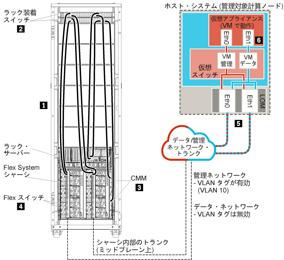
図 17. 仮想アプライアンスの仮想的に分離したデータ/管理ネットワーク・トポロジーの例
