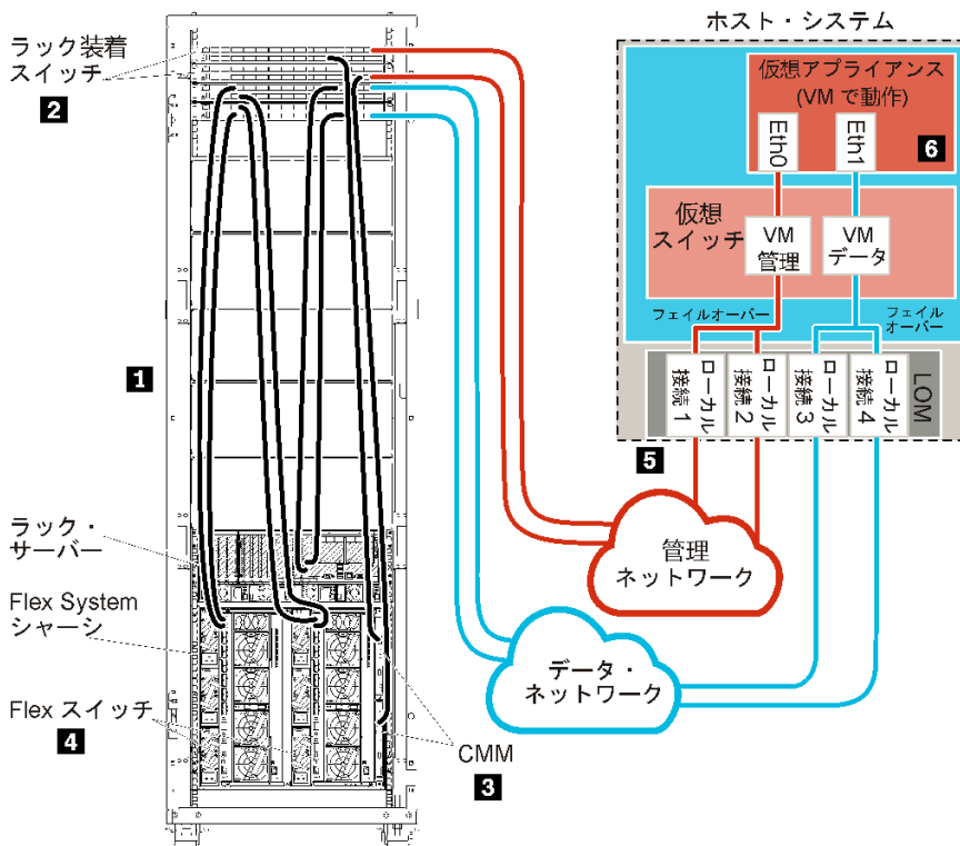
図 13. 仮想アプライアンスの物理的に分離したデータ/管理ネットワーク・トポロジーの例
