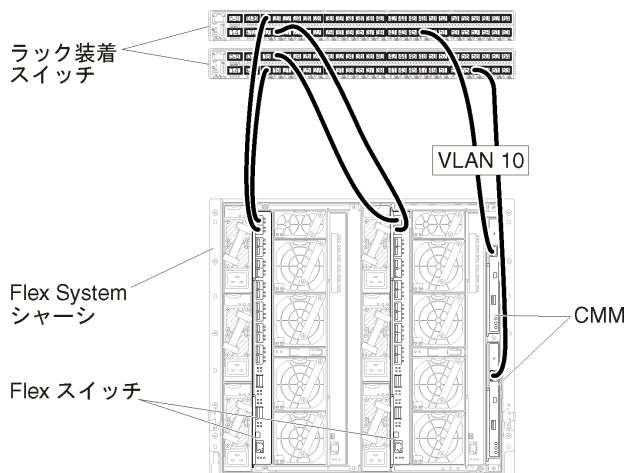
図 21. 管理ネットワークで VLAN タグ付けが有効になっている仮想的に分離したデータ/管理ネットワーク (VMware ESXi) での Flex スイッチの構成の例
