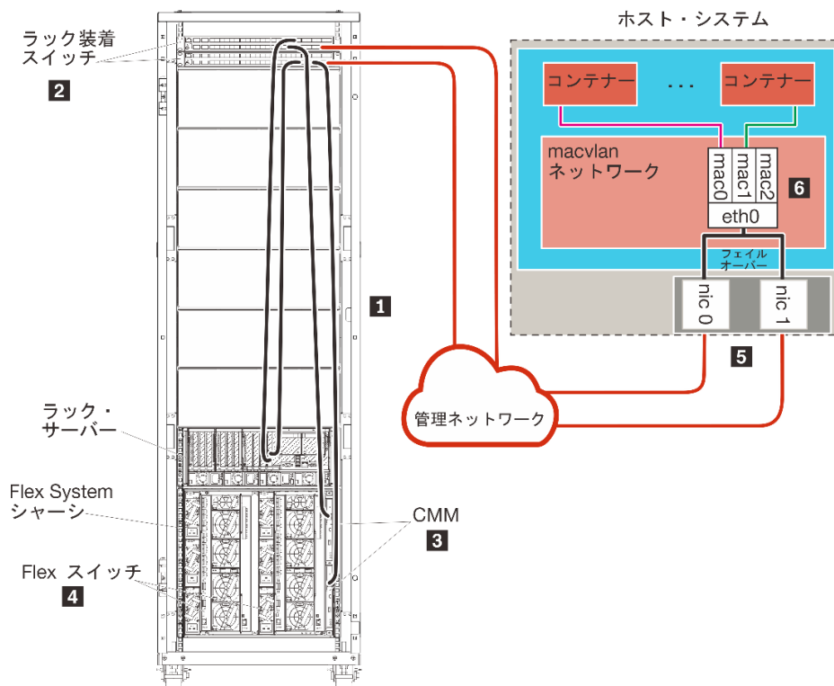
図 26. コンテナの管理専用ネットワーク・トポロジーの例
