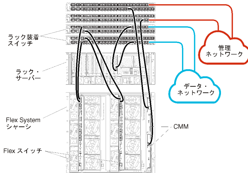
図 15. 物理的に分離したデータ/管理ネットワークの配線の例
