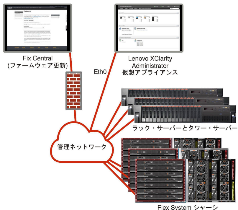
図 6. オペレーティング・システム・デプロイメントをサポートしない管理専用ネットワークの実装例
