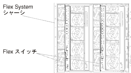
図 28. シャーシにおける Flex スイッチの場所
