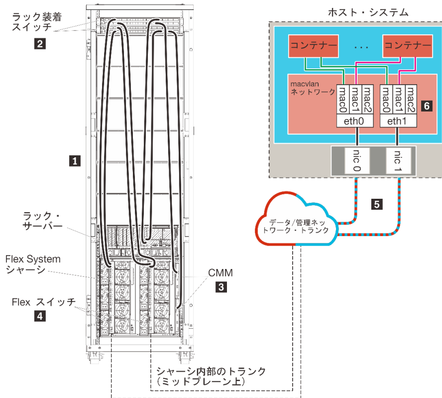
図 18. コンテナの仮想的に分離したデータ/管理ネットワーク・トポロジーの例
