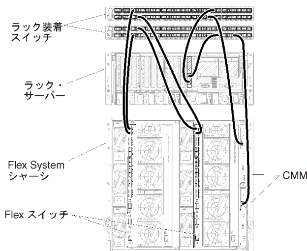
図 19. 仮想的に分離したデータ/管理ネットワークの配線の例
