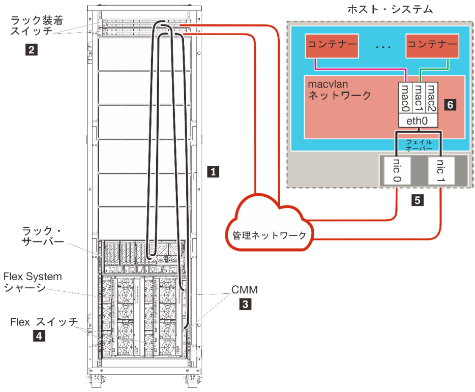
図 24. コンテナの管理専用ネットワーク・トポロジーの例
