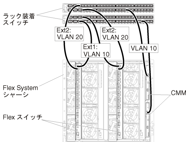
図 20. 両方のネットワークで VLAN タグ付けが有効になっている仮想的に分離したデータ/管理ネットワーク (VMware ESXi) での Flex スイッチの構成の例
