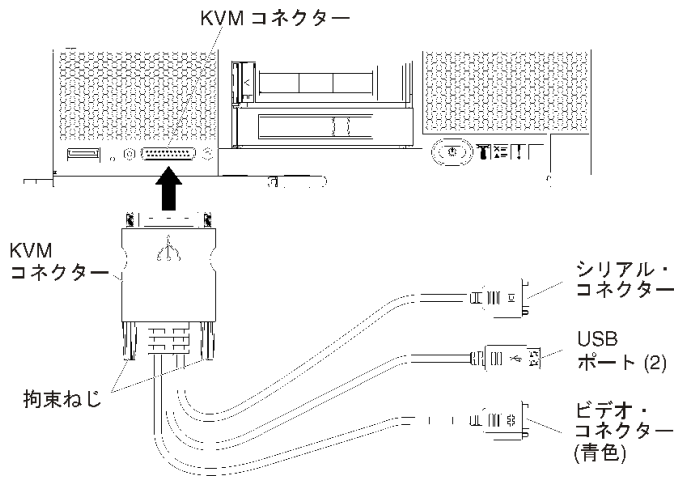
図 21. コンソールの分岐ケーブルとサーバーの前面ベゼル
