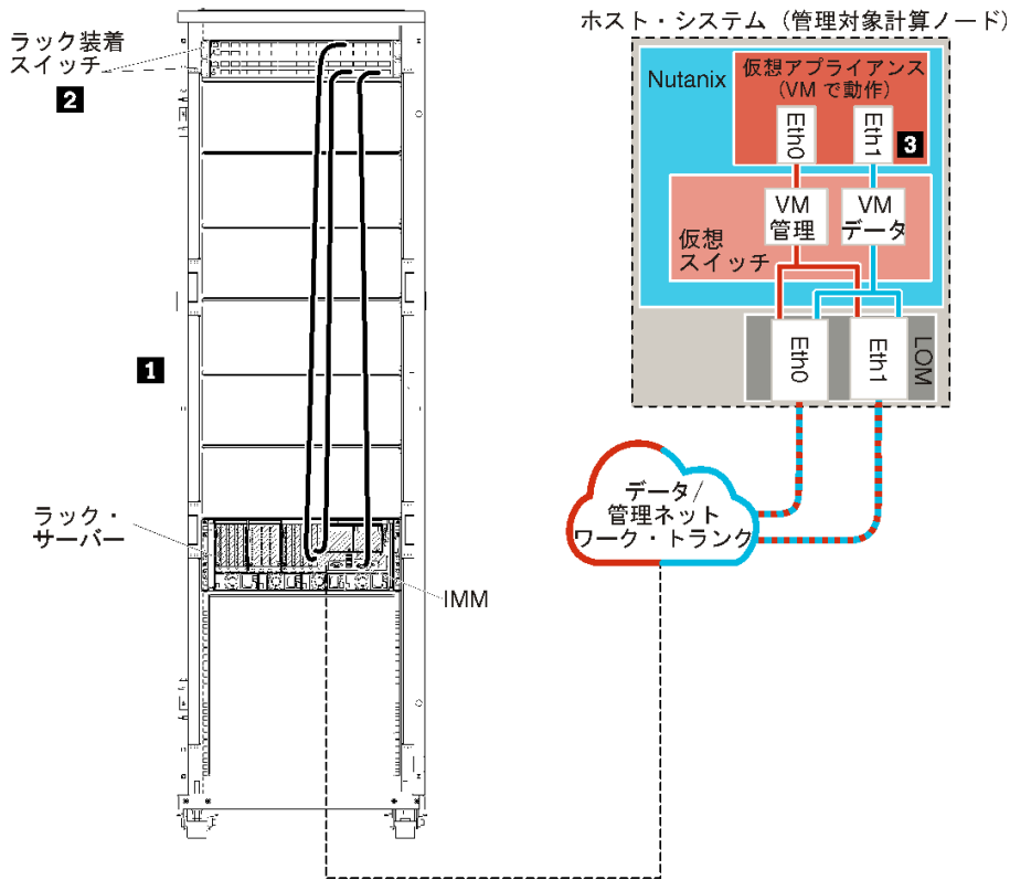
図 12. サンプル・ネットワーク・トポロジー - 仮想的に分離したデータ/管理ネットワーク (Nutanix AHV)
