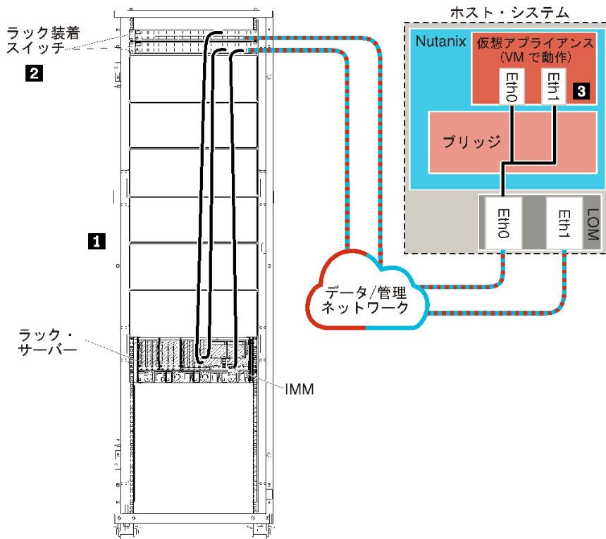
図8. 単一データ/管理ネットワーク・トポロジーのサンプル (Nutanix AHV)
