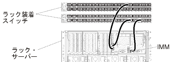
図 13. 仮想的に分離したデータ/管理ネットワークの配線の例
