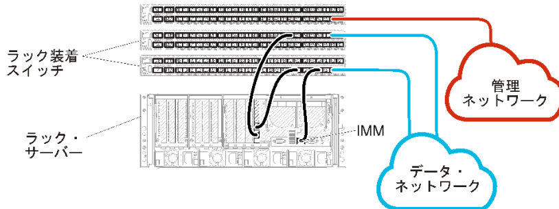
図 11. 物理的に分離したデータ/管理ネットワークの配線の例 (VMware ESXi)
