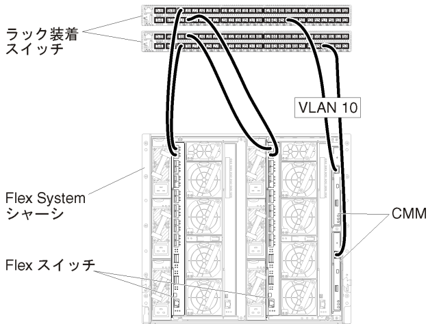
図 14. 管理ネットワークで VLAN タグ付けが有効になっている仮想的に分離したデータ/管理ネットワーク (KVM) での Flex スイッチ の構成の例
