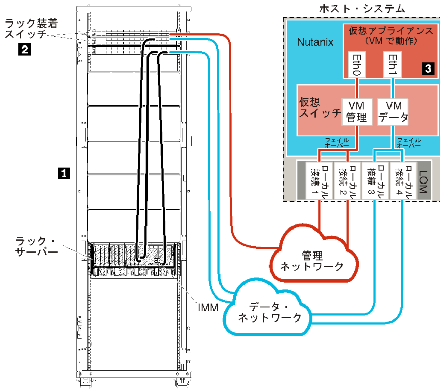
図 10. サンプル・ネットワーク・トポロジー - 物理的に分離したデータ/管理ネットワーク (Nutanix AHV)
