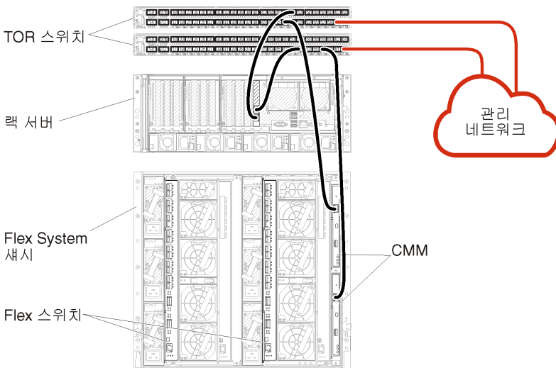
그림 23. 관리 전용 네트워크 케이블 연결 예
