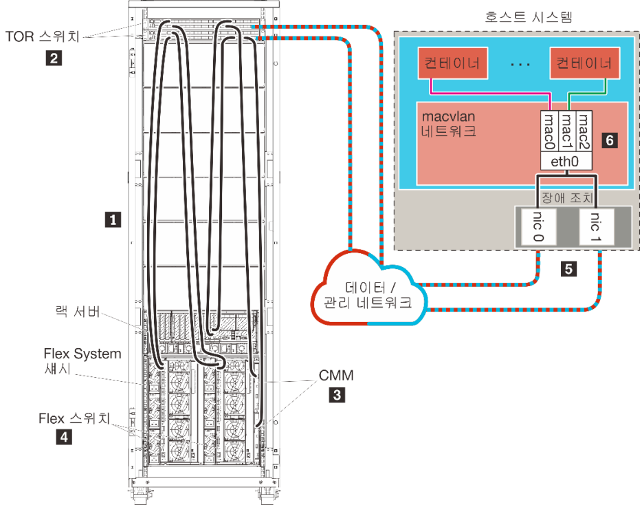
그림 9. 컨테이너의 단일 데이터 및 관리 네트워크 토폴로지 샘플
