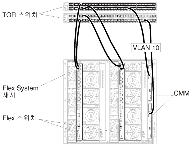
그림 20. 관리 네트워크에서 VLAN 태그 지정이 사용으로 설정된 가상으로 분리된 데이터 및 관리 네트워크의 Flex 스위치 구성 예
