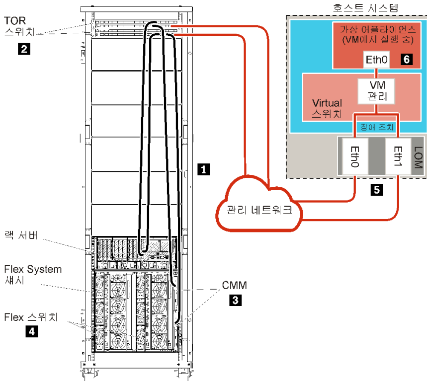
그림 25. 가상 어플라이언스의 샘플 관리 전용 네트워크 토폴로지
