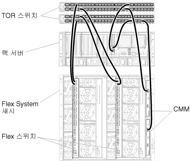
그림 19. 가상으로 분리된 데이터 및 관리 네트워크의 케이블 연결 예
