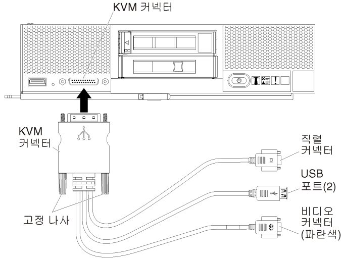
그림 22. 서버의 콘솔 연결 케이블과 앞면 배젤
