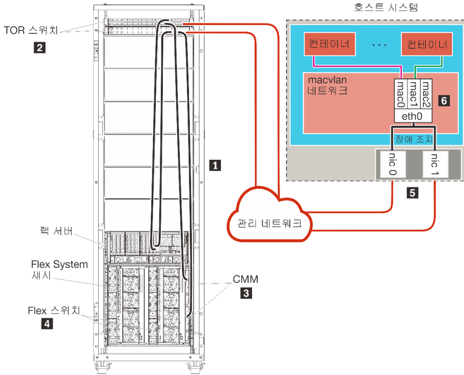
그림 26. 컨테이너의 샘플 관리 전용 네트워크 토폴로지
