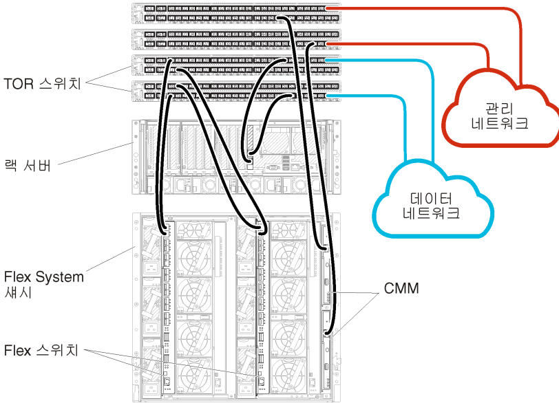
그림 15. 물리적으로 분리된 데이터 및 관리 네트워크의 케이블 연결 예
