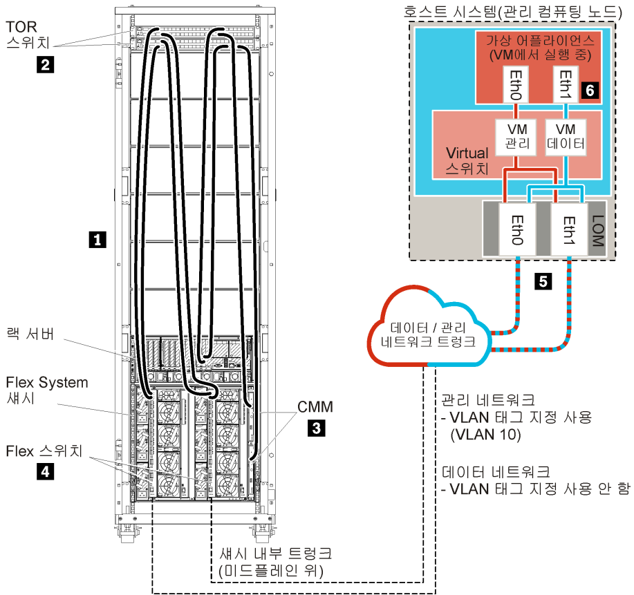
그림 17. 가상 어플라이언스의 가상으로 분리된 데이터 및 관리 네트워크 토폴로지 샘플
