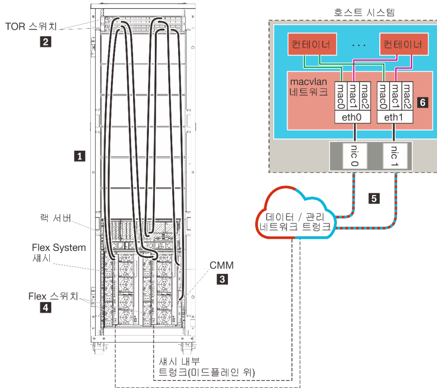
그림 18. 컨테이너의 가상으로 분리된 데이터 및 관리 네트워크 토폴로지 샘플
