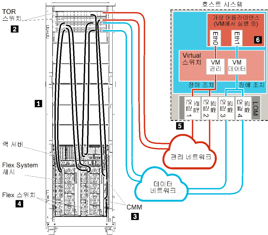
그림 13. 가상 어플라이언스의 물리적으로 분리된 데이터 및 관리 네트워크 토폴로지 샘플
