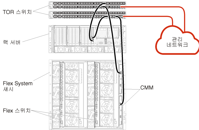
그림 27. 관리 전용 네트워크 케이블 연결 예
