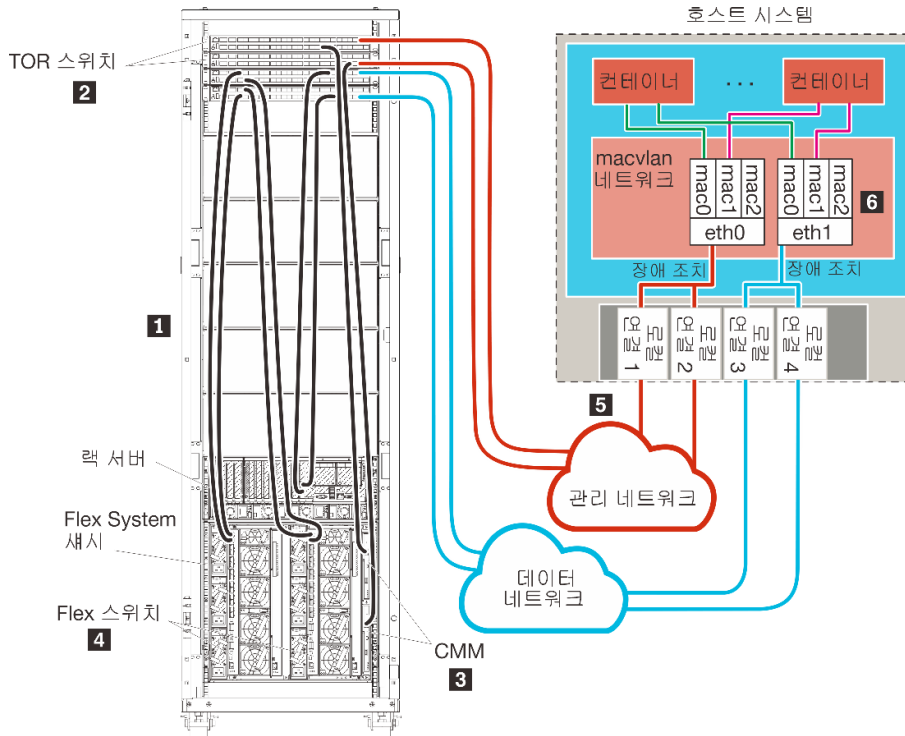
그림 14. 컨테이너의 물리적으로 분리된 데이터 및 관리 네트워크 토폴로지 샘플
