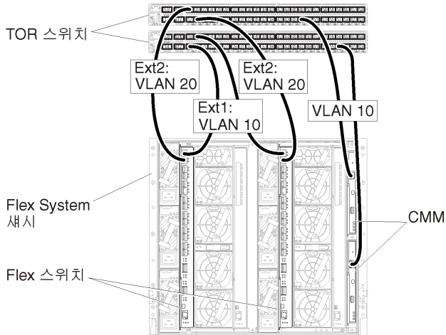
그림 20. 두 네트워크에서 VLAN 태그 지정이 사용으로 설정된 가상으로 분리된 데이터 및 관리 네트워크(VMware ESXi)의 Flex 스위치 구성 예
