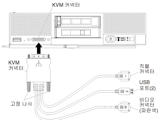
그림 21. 서버의 콘솔 연결 케이블과 앞면 배젤
