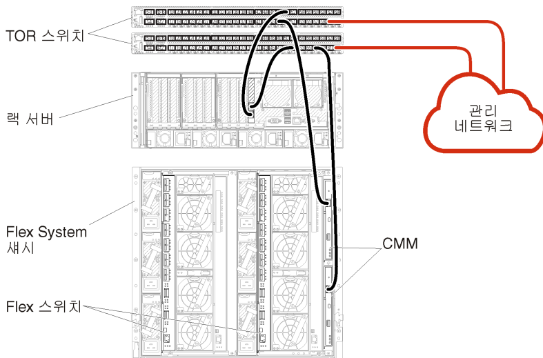
그림 25. 관리 전용 네트워크 케이블 연결 예
