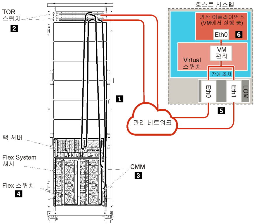
그림 23. 가상 어플라이언스의 샘플 관리 전용 네트워크 토폴로지
