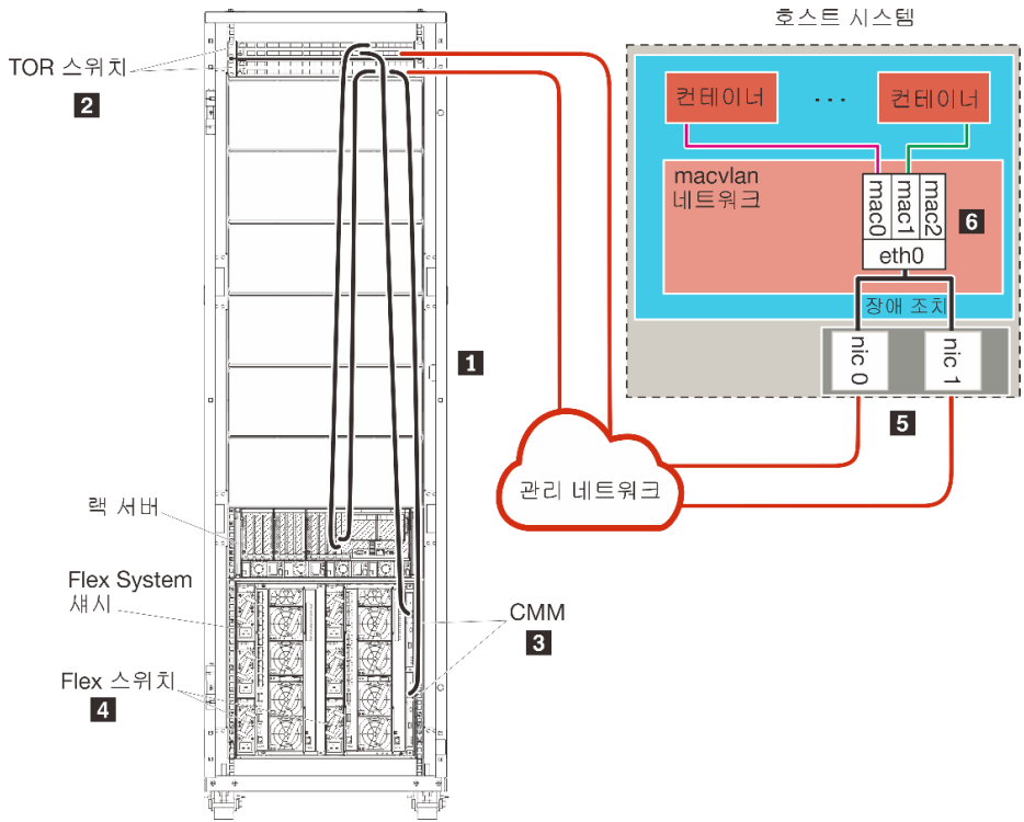
그림 24. 컨테이너의 샘플 관리 전용 네트워크 토폴로지
