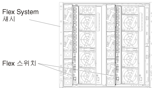
그림 26. 새시의 Flex 스위치 위치
