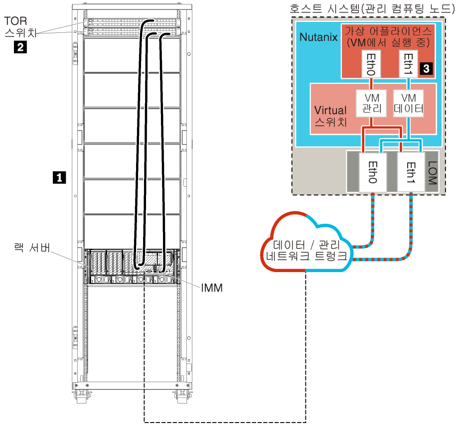
그림 12. 샘플 네트워크 토폴로지 - 가상으로 분리된 데이터 및 관리 네트워크(Nutanix AHV)
