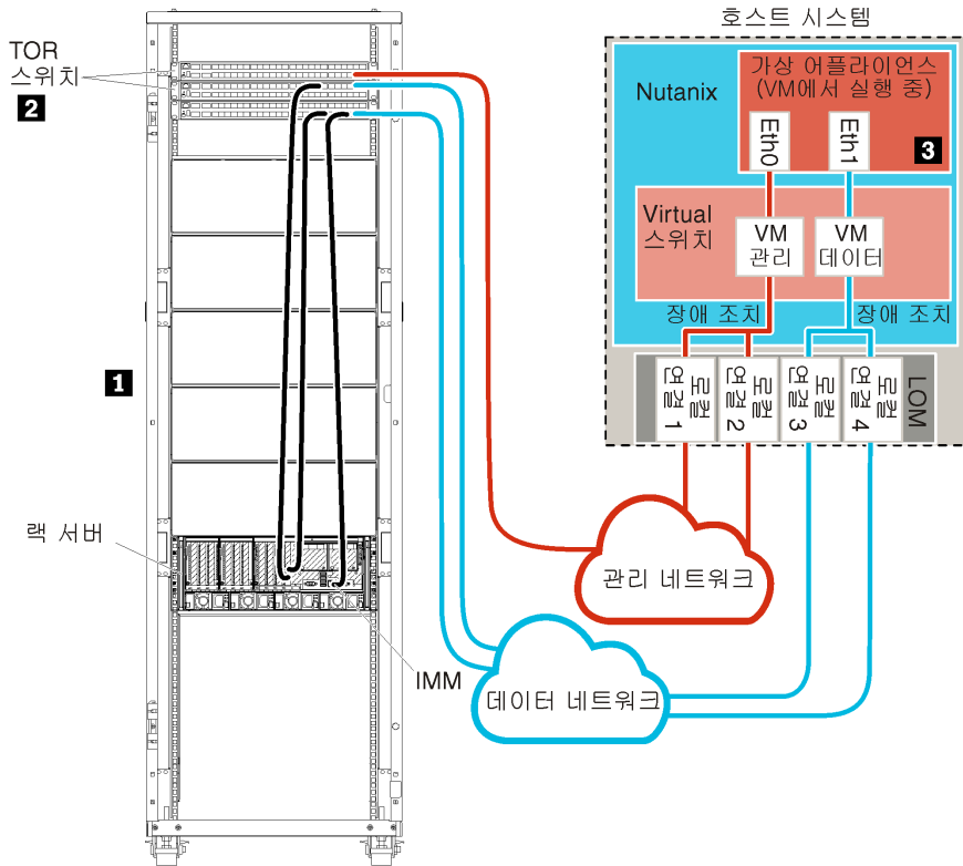
그림 10. 샘플 네트워크 토폴로지 - 물리적으로 분리된 데이터 및 관리 네트워크(Nutanix AHV)
