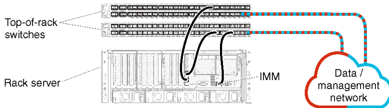
그림 9. 단일 데이터 및 관리 네트워크의 케이블 연결 예
