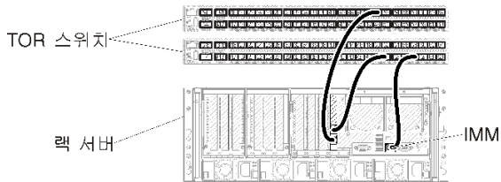
그림 13. 가상으로 분리된 데이터 및 관리 네트워크의 케이블 연결 예
