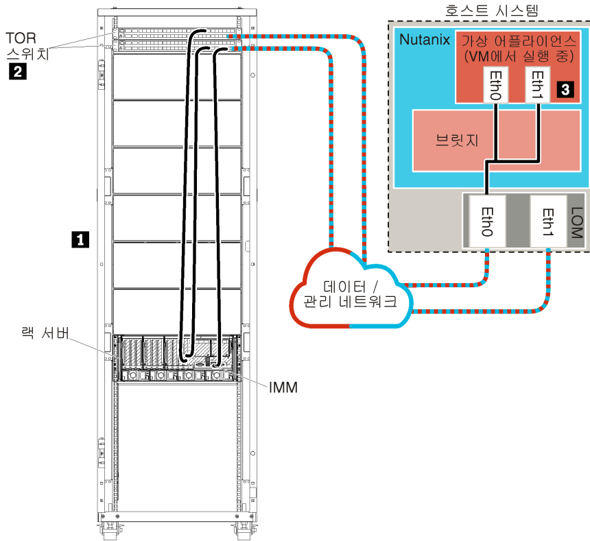
그림 8. 샘플 단일 데이터 및 관리 네트워크 토폴로지(Nutanix AHV)
