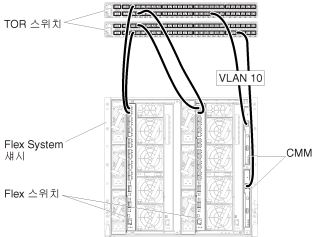
그림 14. 관리 네트워크에서 VLAN 태그 지정이 사용으로 설정된 가상으로 분리된 데이터 및 관리 네트워크(KVM)의 Flex 스위치 구성 예
