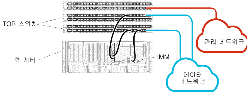
그림 11. 물리적으로 분리된 데이터 및 관리 네트워크의 케이블 연결 예 (VMware ESXi)
