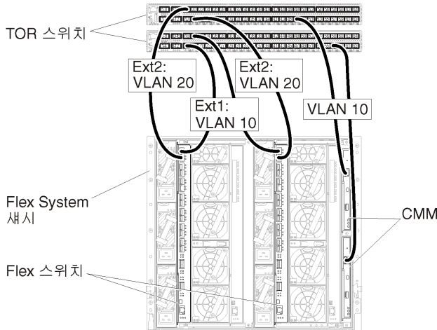
그림 20. 두 네트워크에서 VLAN 태그 지정이 사용으로 설정된 가상으로 분리된 데이터 및 관리 네트워크(Red Hat KVM)의 Flex 스위치 구성 예
