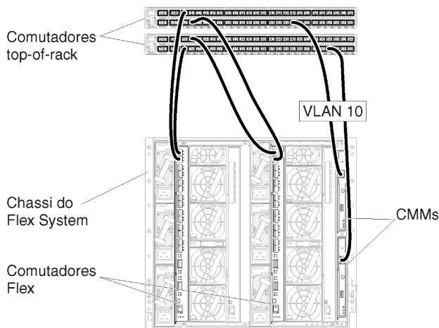
Figura 20. Configuração de exemplo do Comutadores Flex em redes de gerenciamento e dados separados virtualmente nas quais a marcação de VLAN está ativada na rede de gerenciamento
