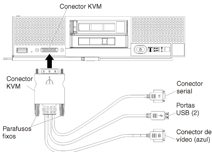
Figura 22. Cabo breakout do console e painel frontal de um servidor
