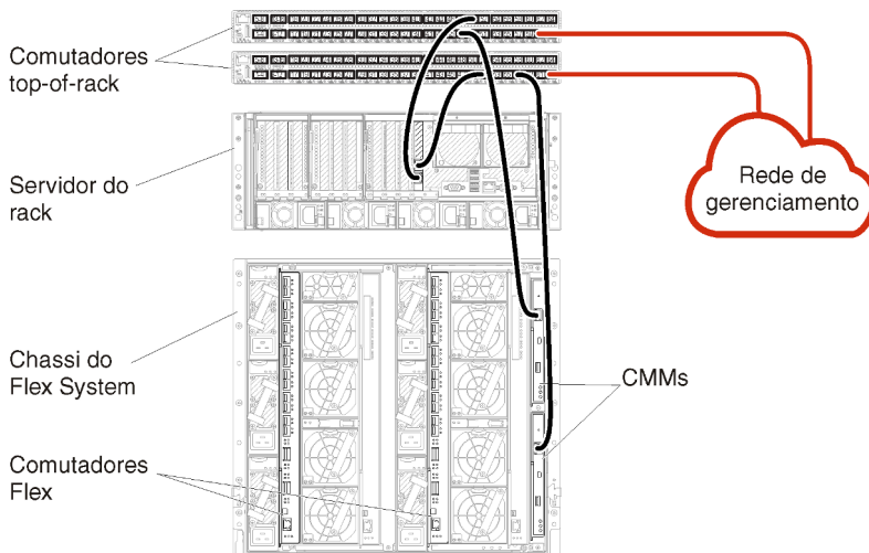
Figura 27. Exemplo de cabeamento para uma rede somente de gerenciamento
