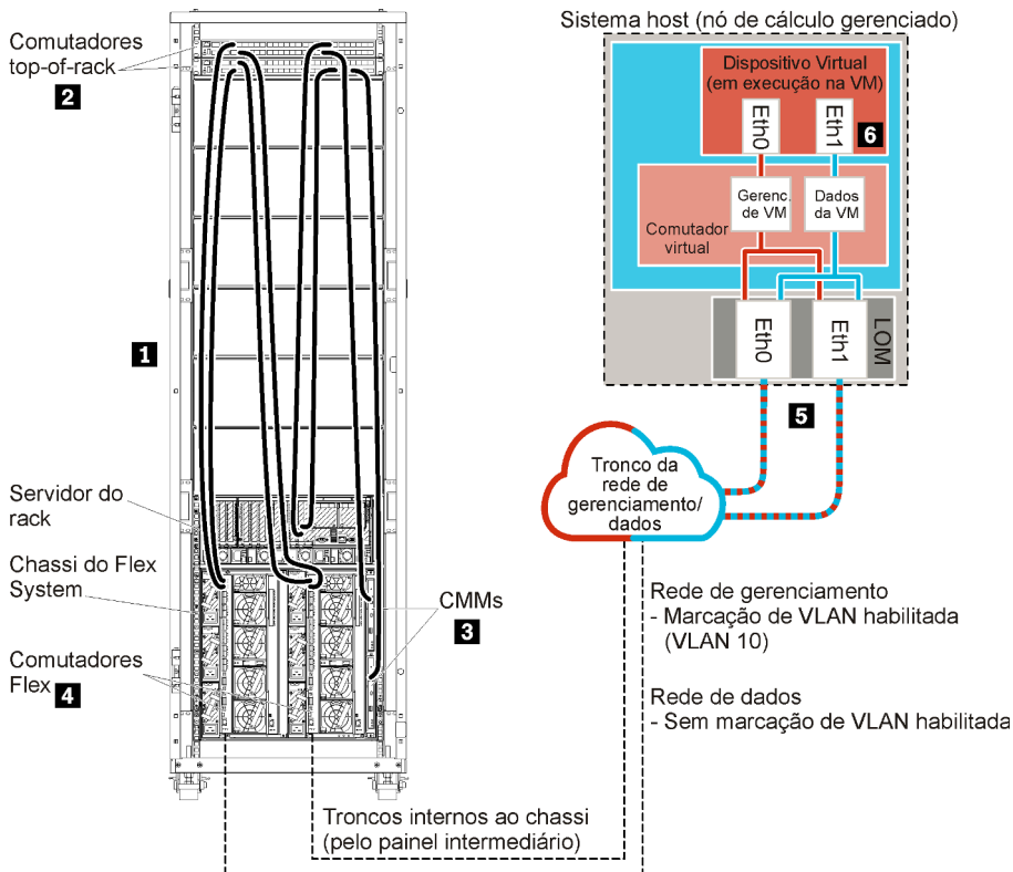
Figura 17. Exemplo de topologia de rede de gerenciamento e dados separados virtualmente para um dispositivo virtual
