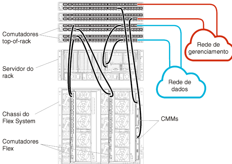
Figura 15. Exemplo de cabeamento de dados separados fisicamente e redes de gerenciamento
