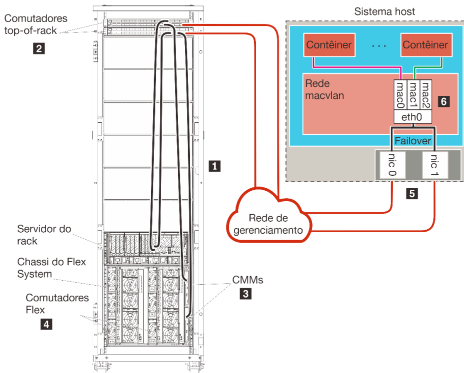
Figura 26. Exemplo de topologia de rede somente de gerenciamento para contêineres
