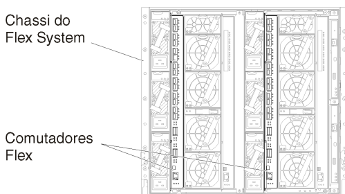
Figura 28. Locais de Comutador Flex em um chassi
