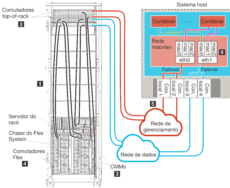
Figura 14. Exemplo de topologia de rede de gerenciamento e dados separados fisicamente para contêineres
