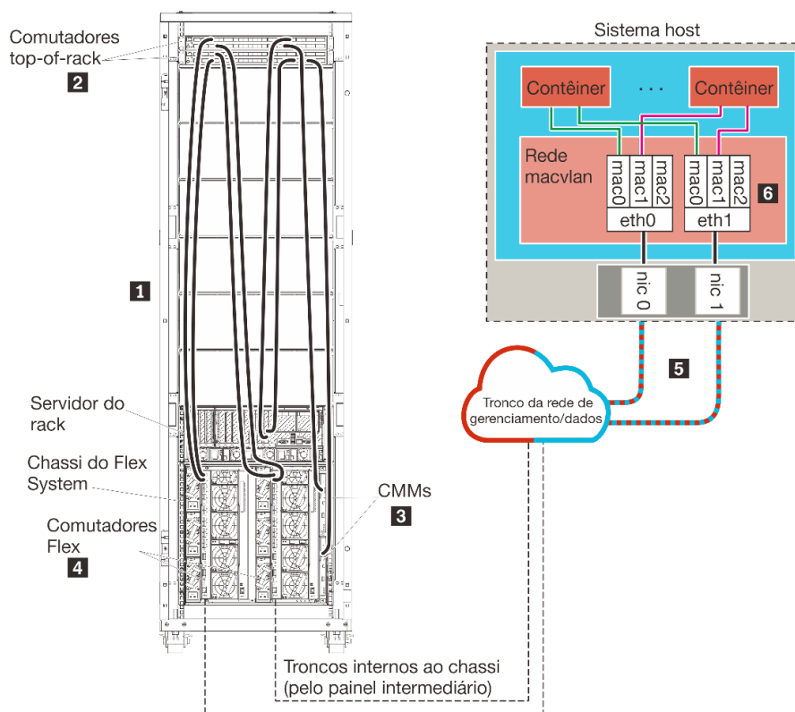
Figura 18. Exemplo de topologia de rede de gerenciamento e dados separados virtualmente para contêineres
