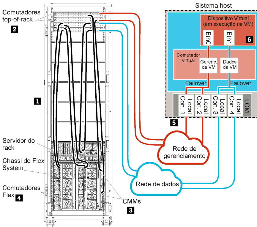
Figura 13. Exemplo de topologia de rede de gerenciamento e dados separados fisicamente para um dispositivo virtual
