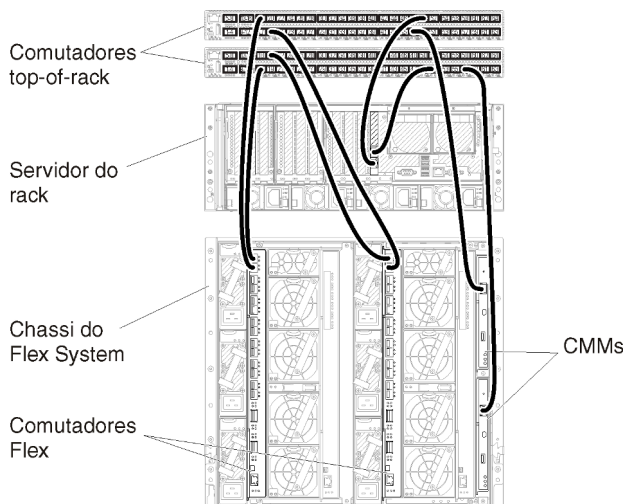
Figura 19. Exemplo de cabeamento de dados separados virtualmente e redes de gerenciamento
