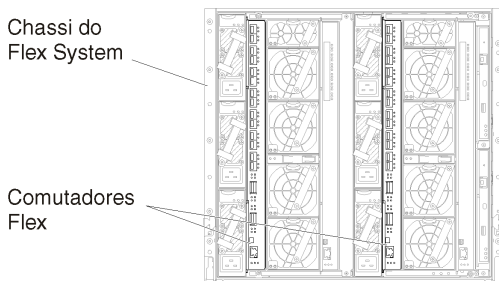
Figura 16. Locais de Comutador Flex em um chassi
