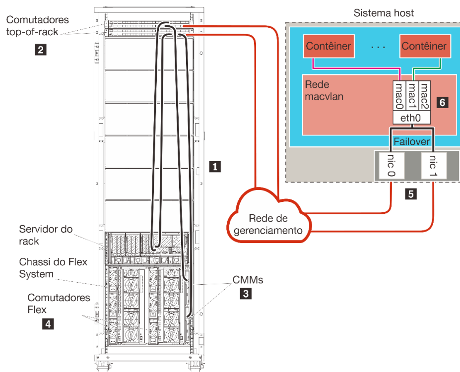
Figura 24. Exemplo de topologia de rede somente de gerenciamento para contêineres
