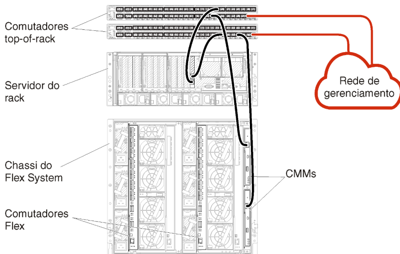
Figura 25. Exemplo de cabeamento para uma rede somente de gerenciamento
