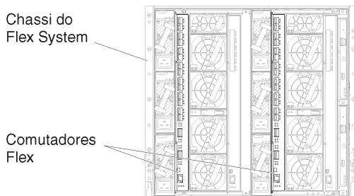
Figura 15. Locais de Comutador Flex em um chassi
