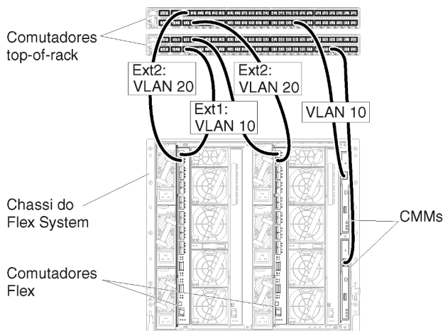
Figura 20. Configuração de exemplo do Comutadores Flex em redes de gerenciamento e dados separados virtualmente (VMware ESXi) nas quais a marcação de VLAN está ativada nas duas redes
