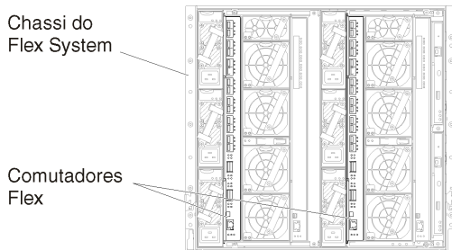
Figura 26. Locais de Comutador Flex em um chassi
