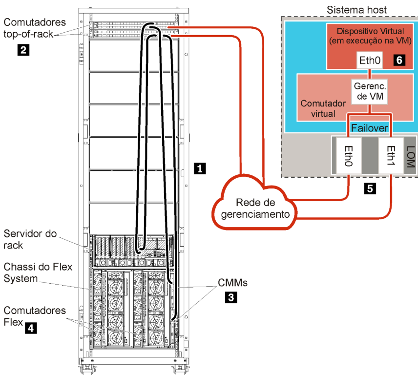
Figura 23. Exemplo de topologia de rede somente de gerenciamento para um dispositivo virtual
