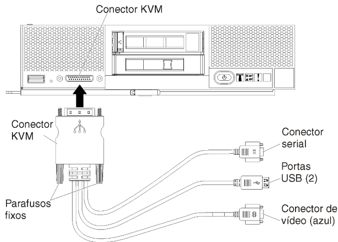
Figura 21. Cabo breakout do console e painel frontal de um servidor
