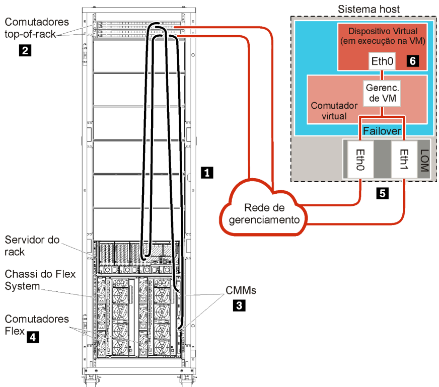
Figura 21. Exemplo de topologia de rede somente de gerenciamento para um dispositivo virtual
