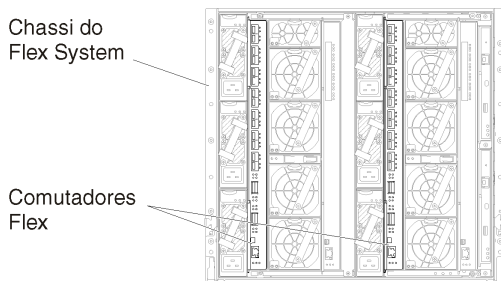
Figura 15. Locais de Comutador Flex em um chassi
