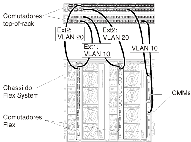
Figura 20. Configuração de exemplo do Comutadores Flex em redes de gerenciamento e dados separados virtualmente (Red Hat KVM) nas quais a marcação de VLAN está ativada nas duas redes
