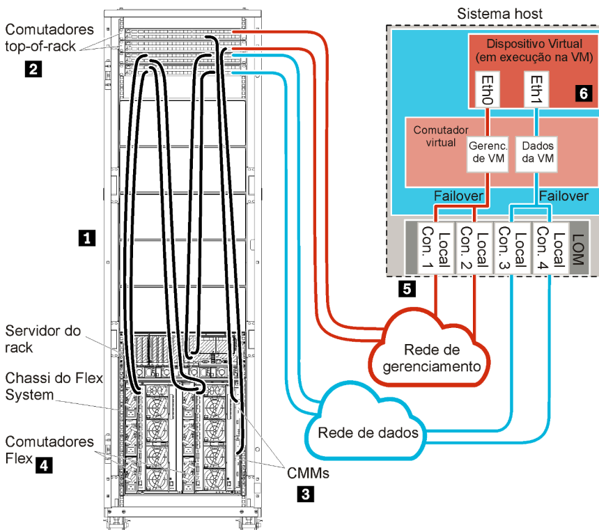
Figura 12. Exemplo de topologia de rede de gerenciamento e dados separados fisicamente para um dispositivo virtual
