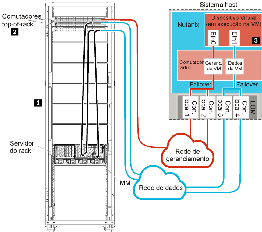
Figura 10. Topologia de rede de amostra - Dados separados fisicamente e rede de gerenciamento (Nutanix AHV)
