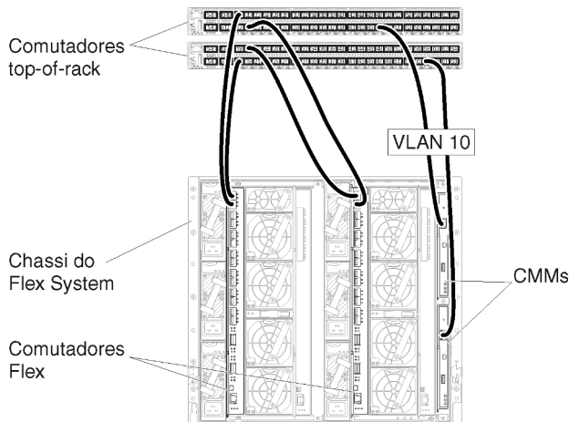
Figura 14. Configuração de exemplo do Comutadores Flex em redes de gerenciamento e dados separados virtualmente (KVM) nas quais a marcação de VLAN está ativada na rede de gerenciamento
