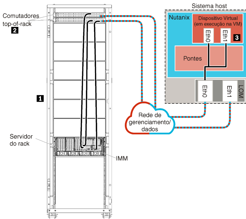
Figura 8. Dados únicos e topologia de rede de gerenciamento de amostra (Nutanix AHV)
