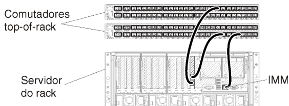
Figura 13. Exemplo de cabeamento de dados separados virtualmente e redes de gerenciamento
