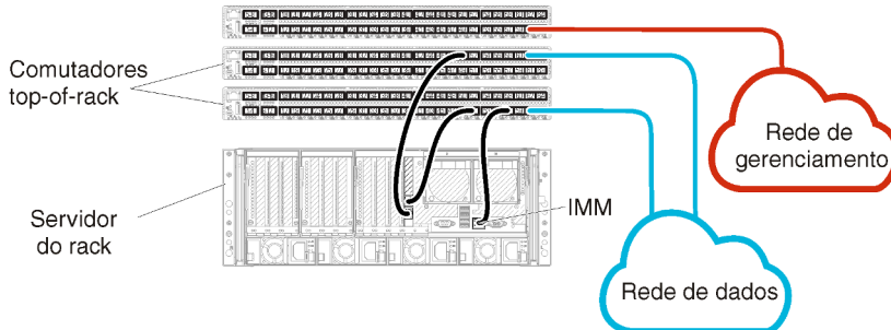
Figura 11. Exemplo de cabeamento de dados separados fisicamente e redes de gerenciamento (VMware ESXi)
