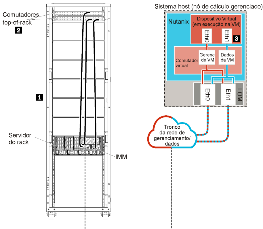
Figura 12. Topologia de rede de amostra - Dados separados virtualmente e rede de gerenciamento (Nutanix AHV)
