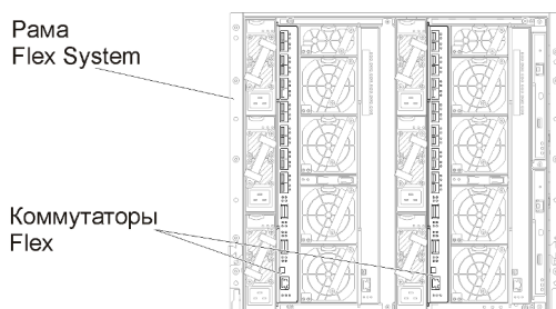
Рис. 28. Места установки Коммутатор Flex в раме
