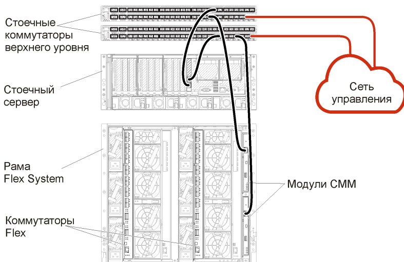
Рис. 27. Пример кабельных соединений для сети только для управления
