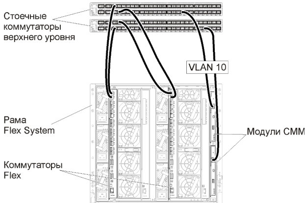
Рис. 21. Пример конфигурации для Коммутаторы Flex в виртуально разделенных сетях данных и управления (VMware ESXi), в которой добавление меток VLAN включено в сети управления
