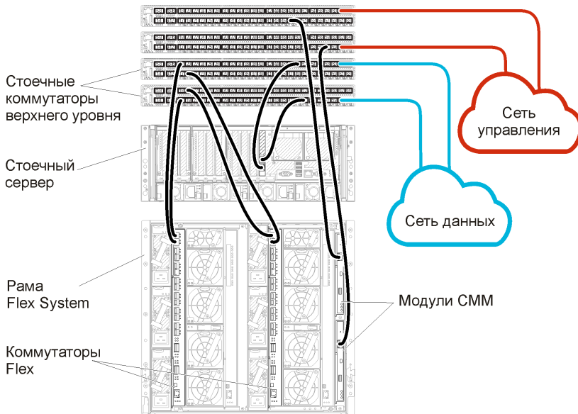
Рис. 15. Пример кабельных соединений для физически раздельных сетей данных и управления
