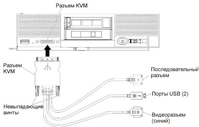
Рис. 22. Разводной консольный кабель и лицевая панель сервера
