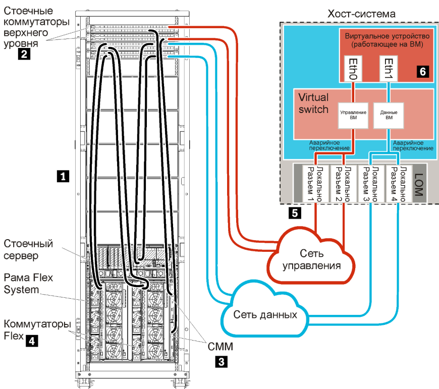
Рис. 13. Пример физически раздельных данных и топологии сети управления для виртуального устройства
