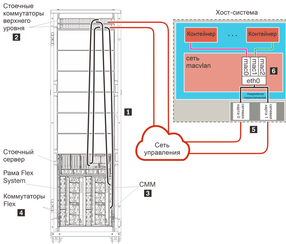
Рис. 26. Пример топологии сети только для управления для контейнеров
