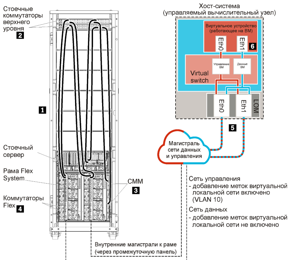
Рис. 17. Пример виртуально отдельных данных и топологии сети управления для виртуального устройства
