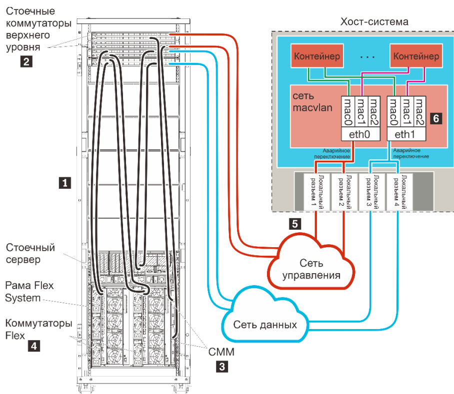
Рис. 14. Пример физически раздельных данных и топологии сети управления для контейнеров
