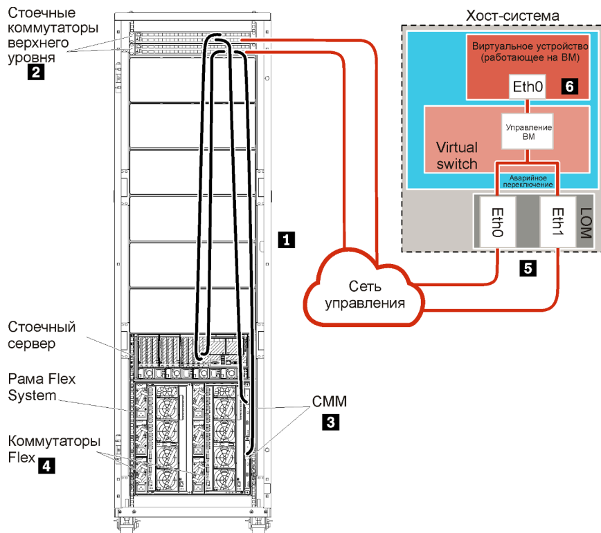
Рис. 25. Пример топологии сети только для управления для виртуального устройства
