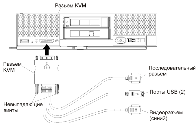
Рис. 21. Разводной консольный кабель и лицевая панель сервера
