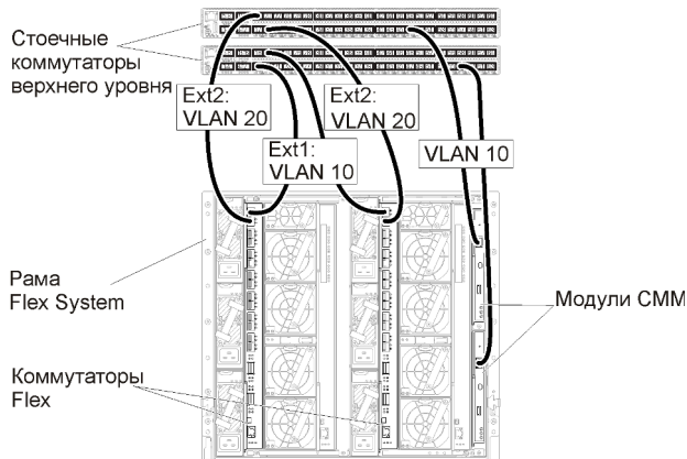
Рис. 20. Пример конфигурации для Коммутаторы Flex в виртуально разделенных сетях данных и управления (VMware ESXi), в которой добавление меток VLAN включено в обеих сетях
