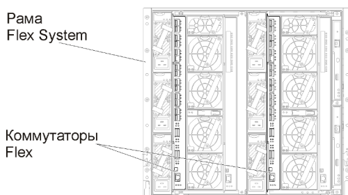
Рис. 26. Места установки Коммутатор Flex в раме
