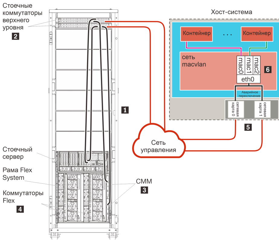
Рис. 24. Пример топологии сети только для управления для контейнеров
