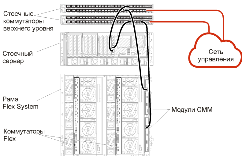
Рис. 25. Пример кабельных соединений для сети только для управления
