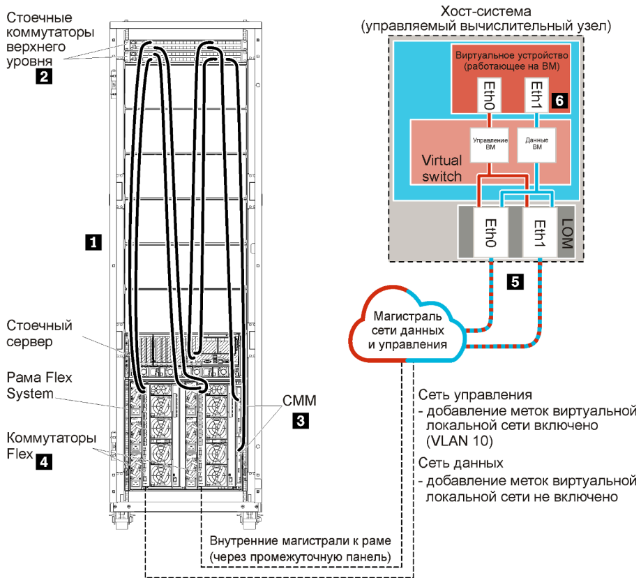
Рис. 16. Пример виртуально разделенных данных и топологии сети управления для виртуального устройства
