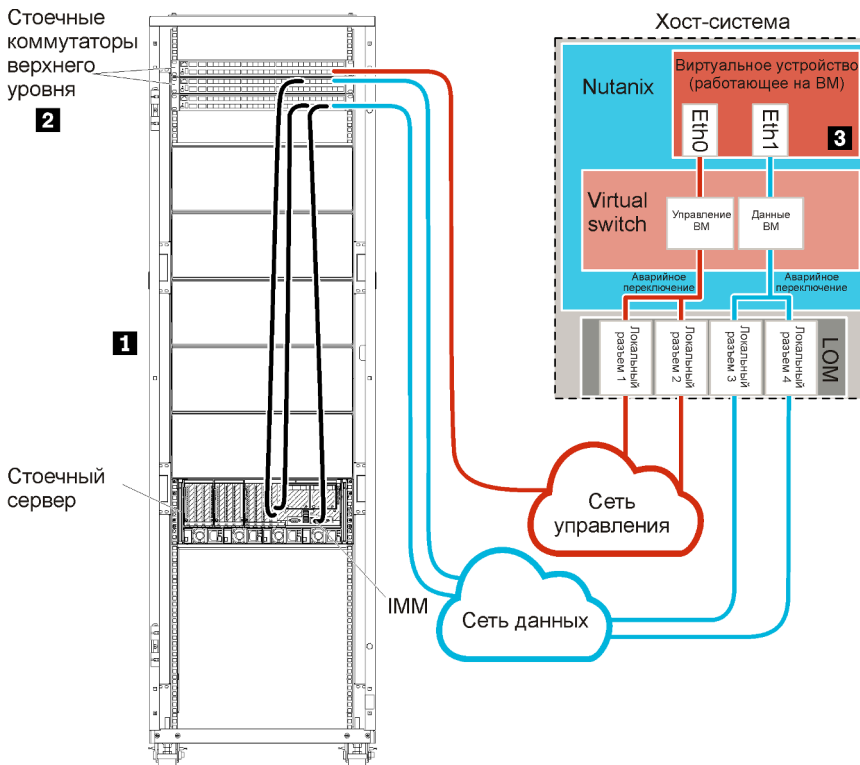
Рис. 10. Пример топологии сети: физическое разделение сети данных и сети управления (Nutanix AHV)
