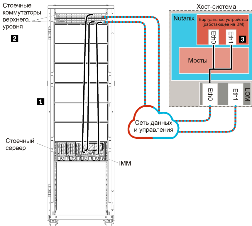
Рис. 8. Пример топологии единой сети данных и управления (Nutanix AHV)
