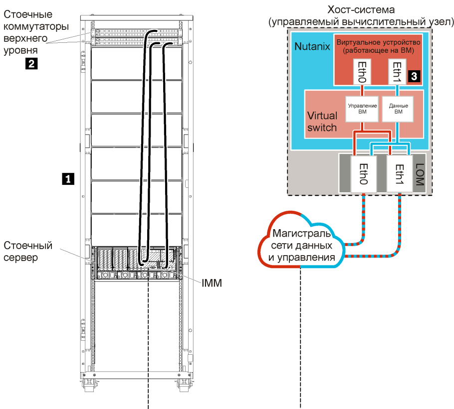
Рис. 12. Пример топологии сети: виртуальное разделение сети данных и сети управления (Nutanix AHV)
