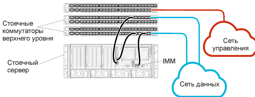
Рис. 11. Пример кабельных соединений для физически раздельных сетей данных и управления (VMware ESXi)
