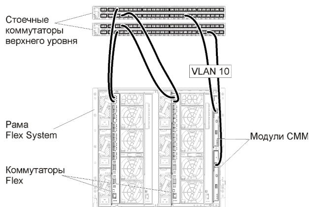
Рис. 14. Пример конфигурации для Коммутаторы Flex в виртуально разделенных сетях данных и управления (KVM), в которой добавление меток VLAN включено в сети управления
