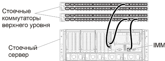
Рис. 13. Пример кабельных соединений для виртуально отдельных сетей данных и управления
