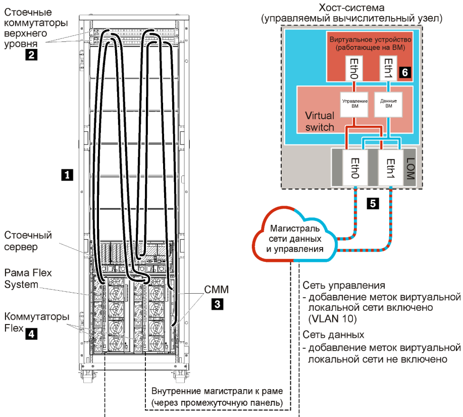
Рис. 16. Пример виртуально раздельных данных и топологии сети управления для виртуального устройства
