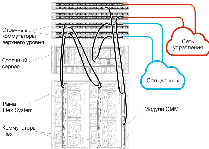
Рис. 14. Пример кабельных соединений для физически отдельных сетей данных и управления
