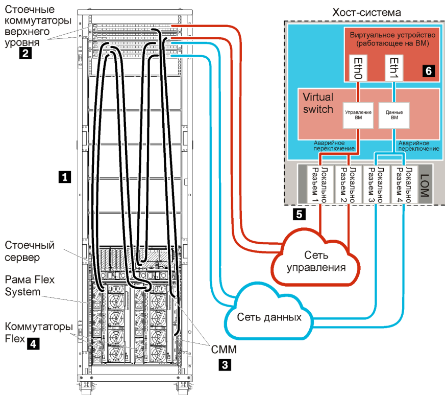
Рис. 12. Пример физически раздельных данных и топологии сети управления для виртуального устройства
