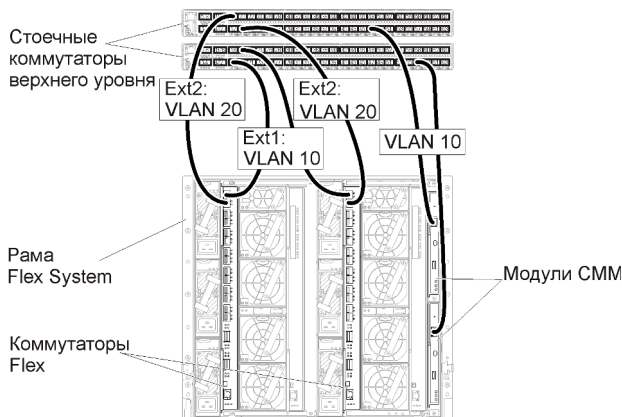
Рис. 20. Пример конфигурации для Коммутаторы Flex в виртуально разделенных сетях данных и управления (Red Hat KVM), в которой добавление меток VLAN включено в обеих сетях
