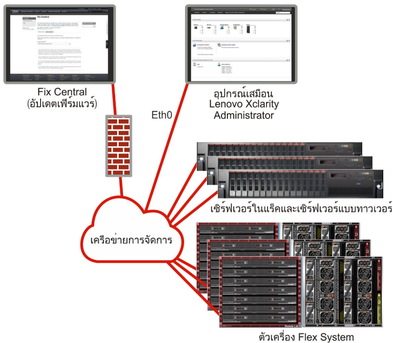
รูปภาพ 6. ตัวอย่างการนำมาใช้งานของเครือข่ายการจัดการอย่างเดียวที่ไม่มีการรองรับสำหรับการปรับใช้ระบบปฏิบัติการ
