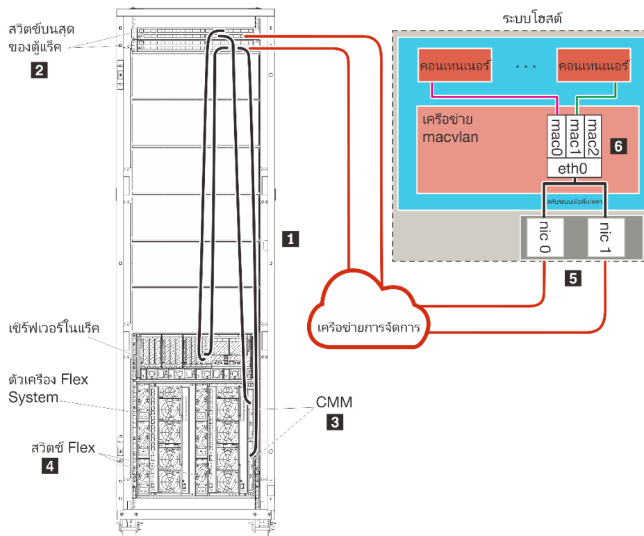
รูปภาพ 22. ตัวอย่างโทโพโลยีเครือข่ายการจัดการอย่างเดียสำหรับคอนเทนเนอร์
